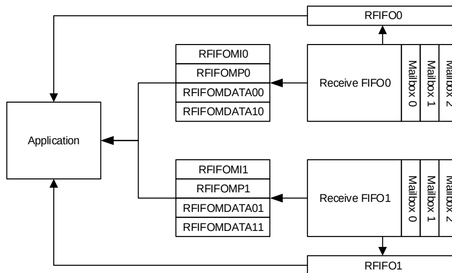
图 26-4. 接收寄存器
