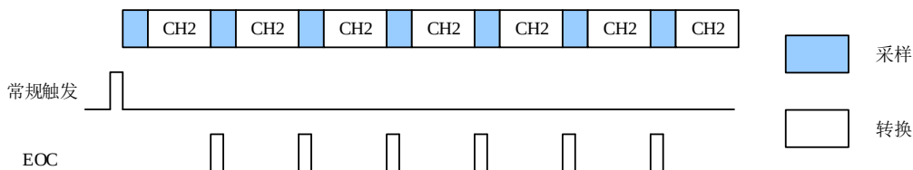
图 14-3. 连续运行模式
