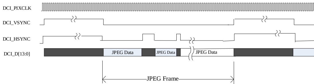
图 22-3. 硬件同步模式之 JPEG 格式
