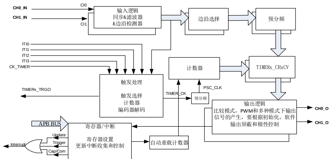
图 18-43. 通用定时器 L1 结构框图
