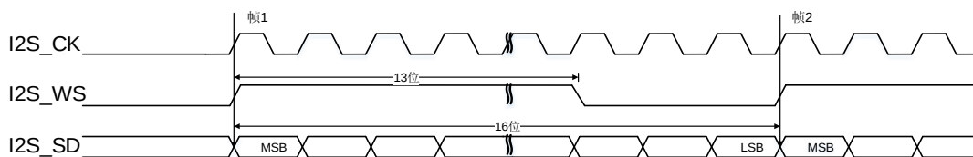
图 21-42. PCM 标准长帧同步模式时序图 (DTLEN=00, CHLEN=0, CKPL=0)
