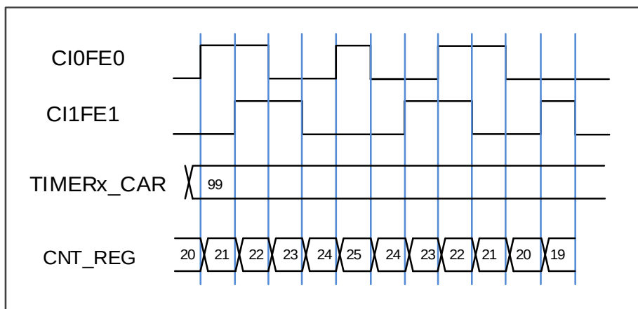
图 18-18. 在译码器模式 2 且 CI0FE0 极性不反相时计数器行为
