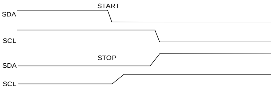
图 20-3. 起始和停止信号
