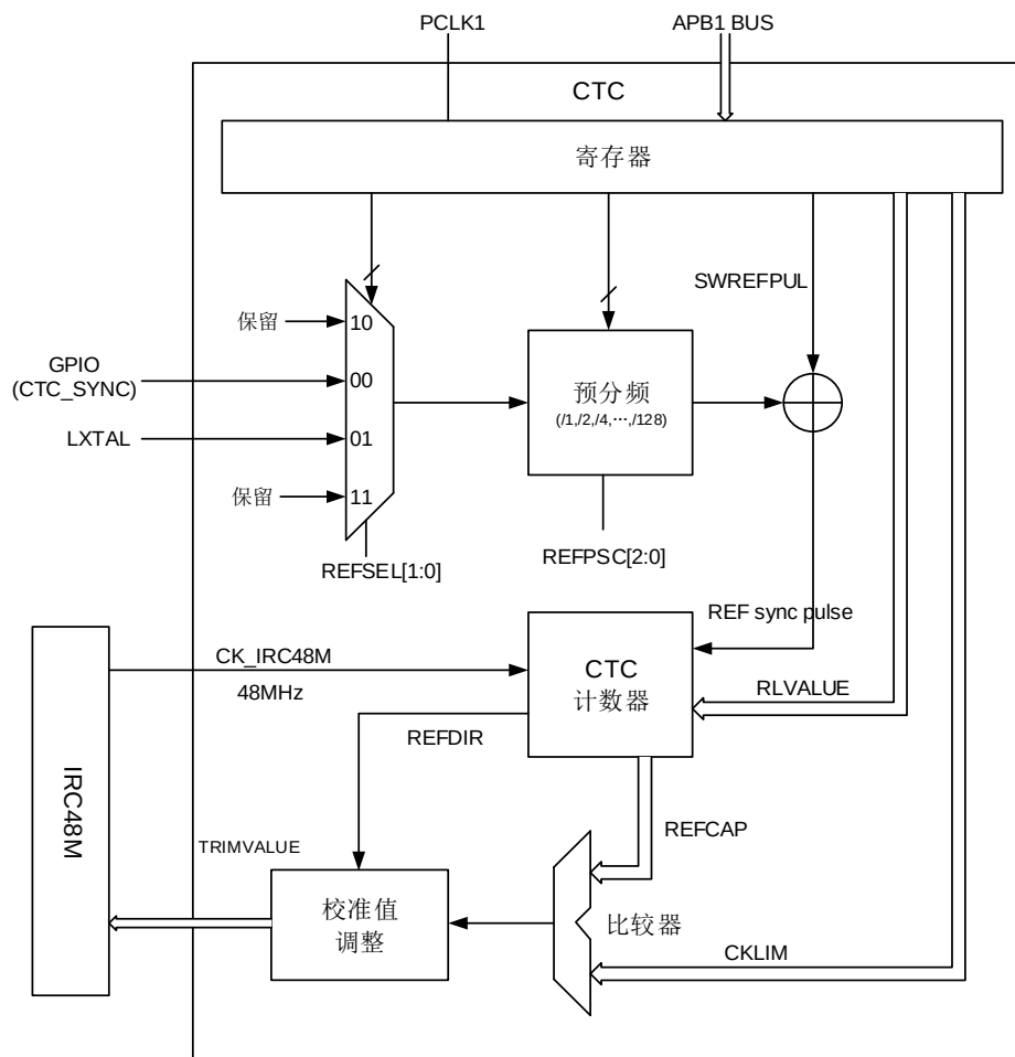
图5-1. CTC简介
