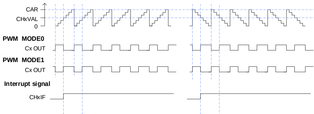
图 18-15. CAPWM 时序图
