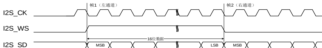
图 21-22. MSB 对齐标准时序图 (DTLEN=00, CHLEN=0, CKPL=0)
