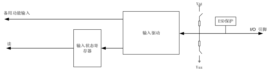
图 7-2. 输入配置的基本结构
