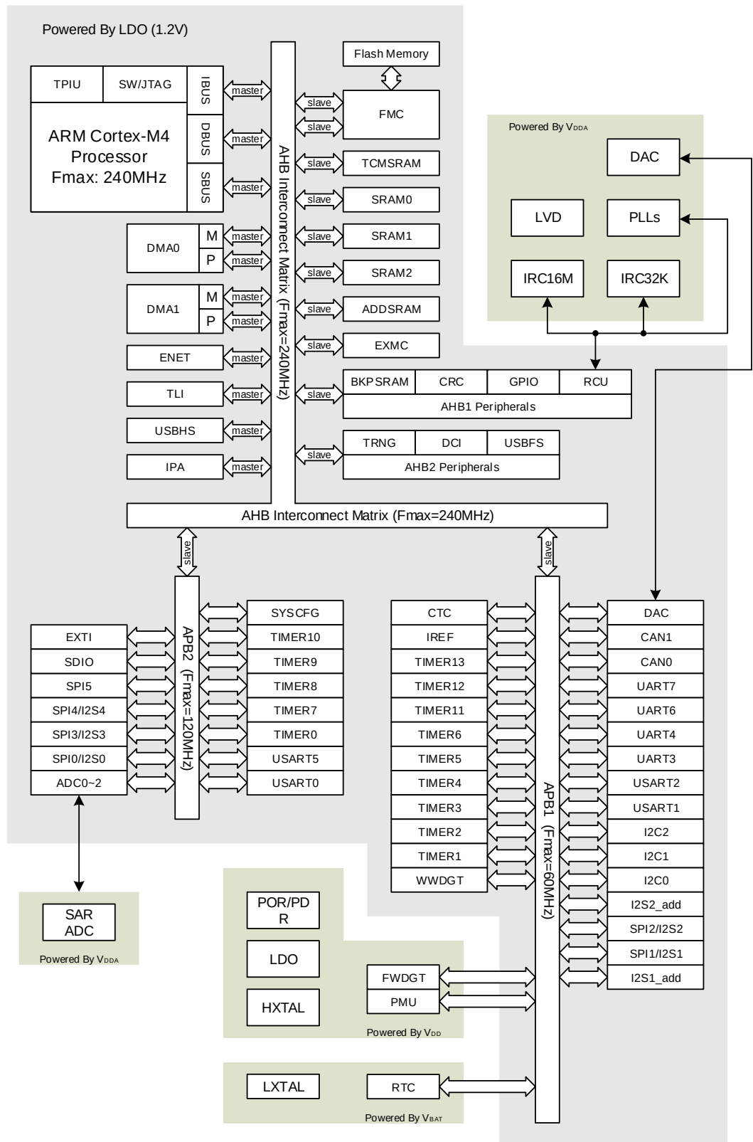
图 1-2. GD32F4xx 器件的系统架构示意图
