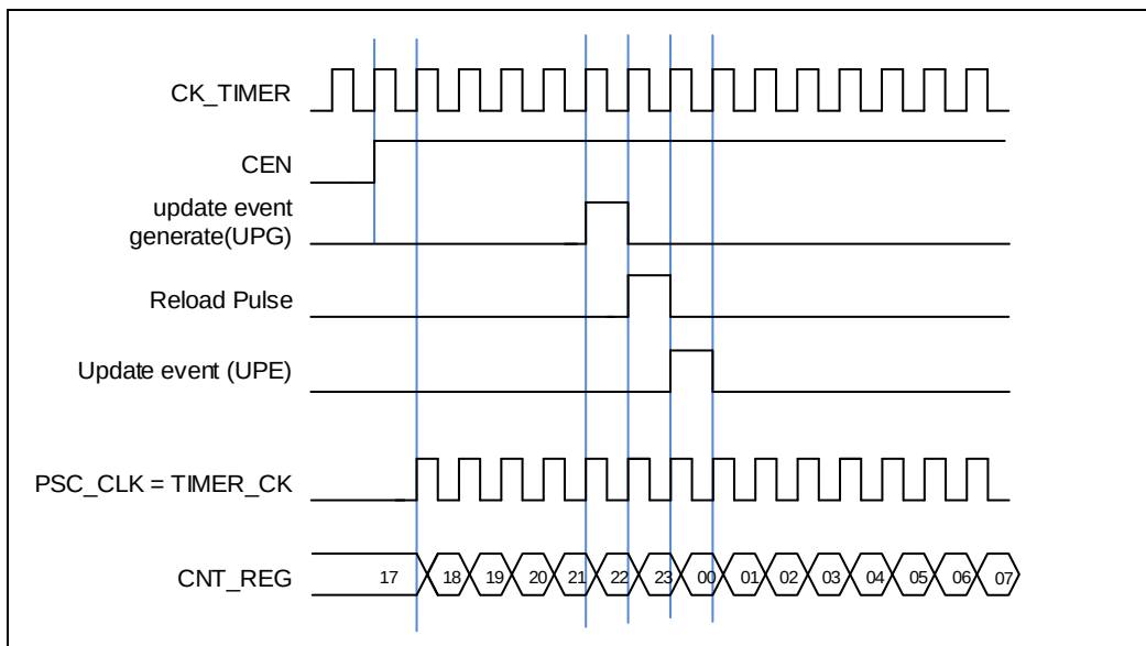
图 18-29. 内部时钟分频为 1 时，计数器的时序图
