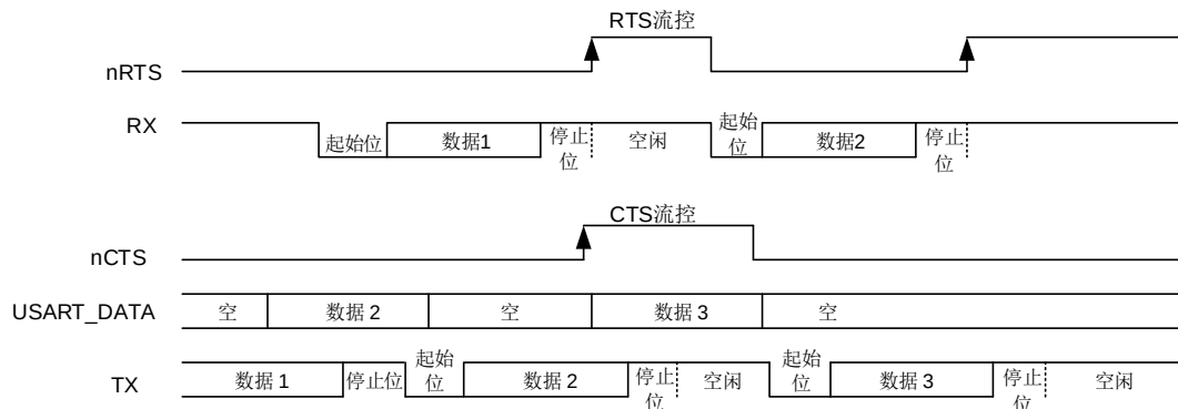
图 19-8. 硬件流控制
