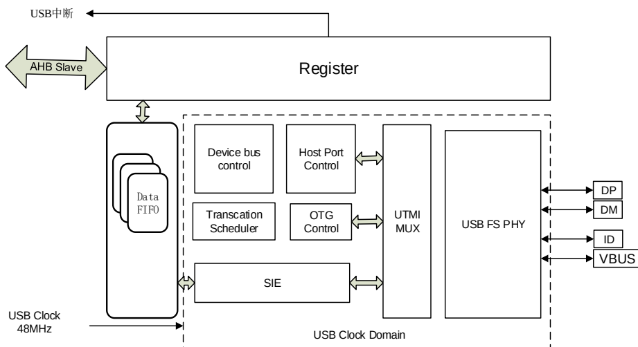
图 28-1. USBFS 结构框图
