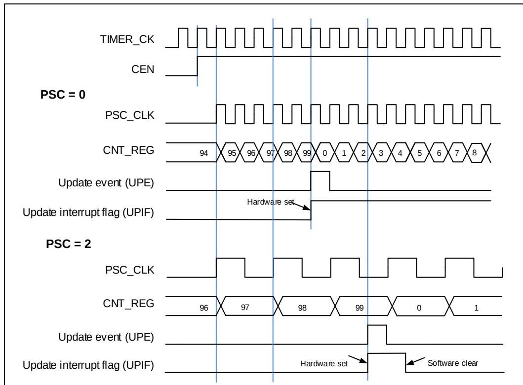
图 18-31. 向上计数时序图, PSC=0/2
