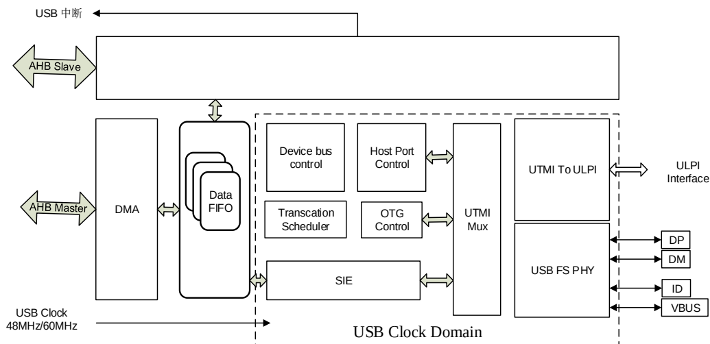
图 29-1. USBHS 结构框图
