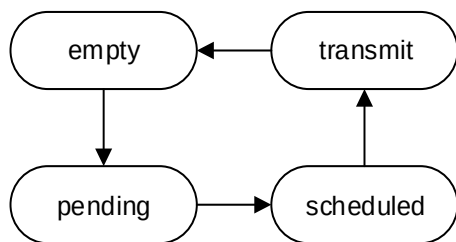
图 26-3. 发送邮箱状态转换
