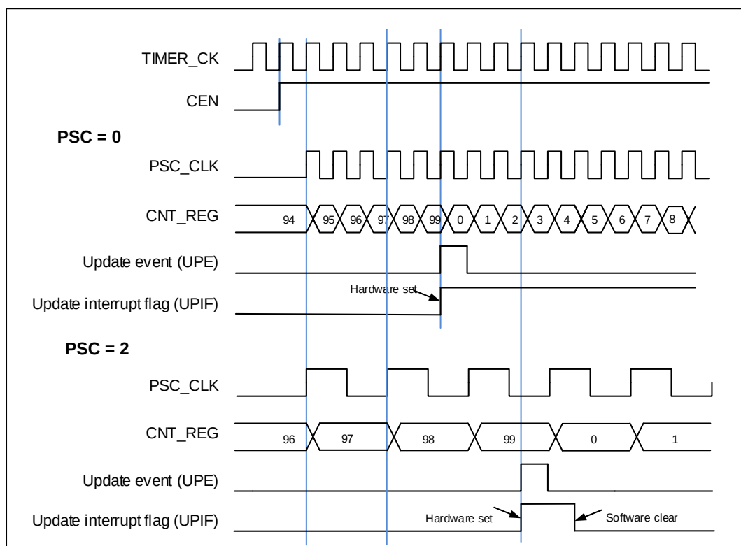
图 18-66. 向上计数时序图， PSC=0/2
