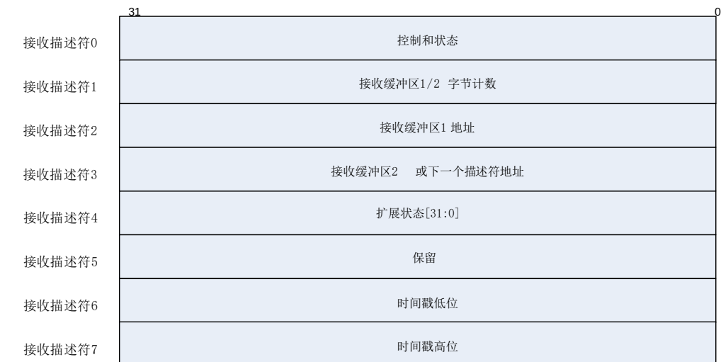
图 27-10. 增强接收描述符
