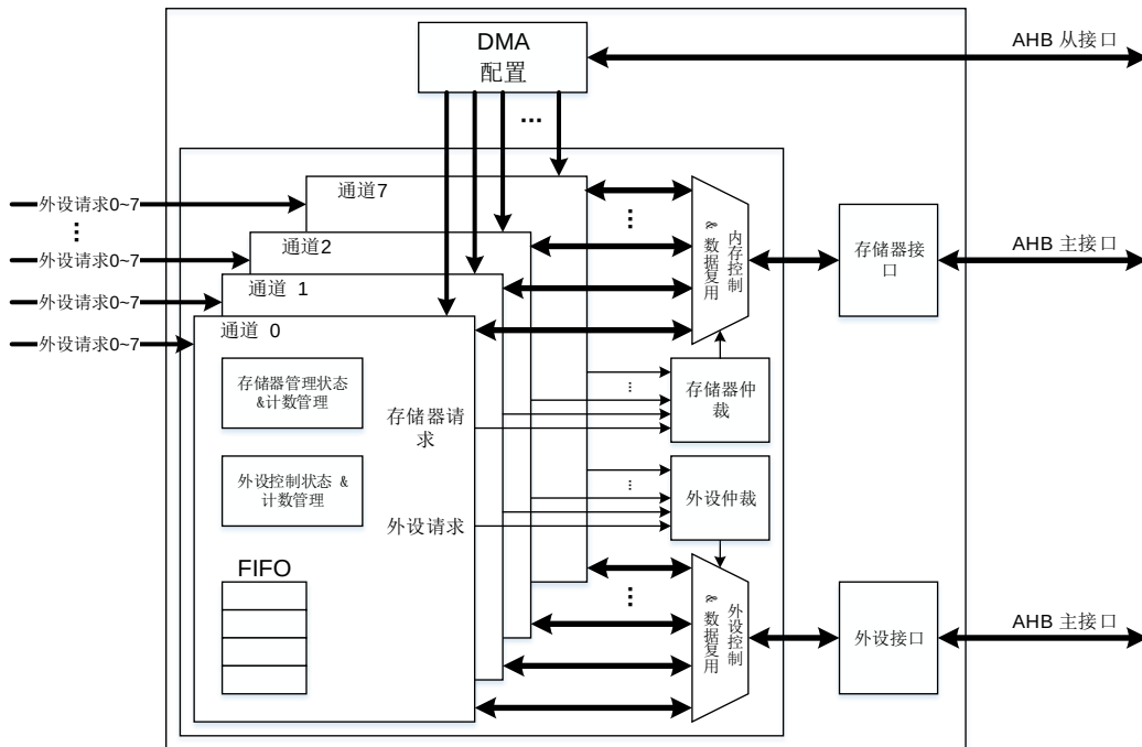
图 10-1. 系统架构
