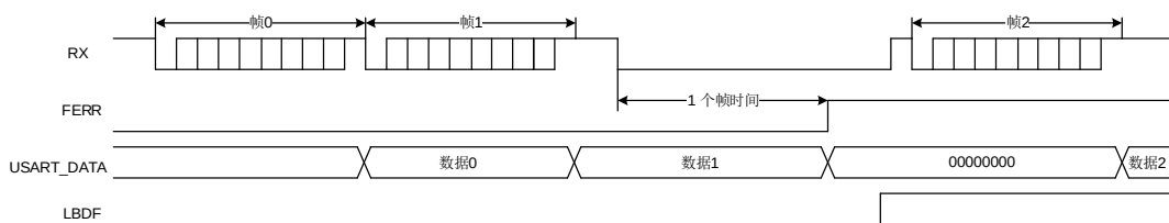
图 19-9. 空闲状态下检测断开帧
