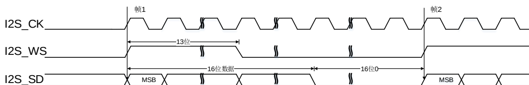
图 21-48. PCM 标准长帧同步模式时序图 (DTLEN=00, CHLEN=1, CKPL=0)
