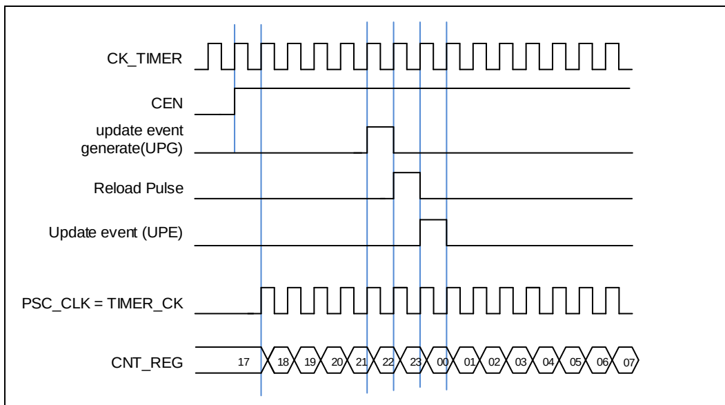
图 18-64. 内部时钟分频为 1 时，计数器的时序图
