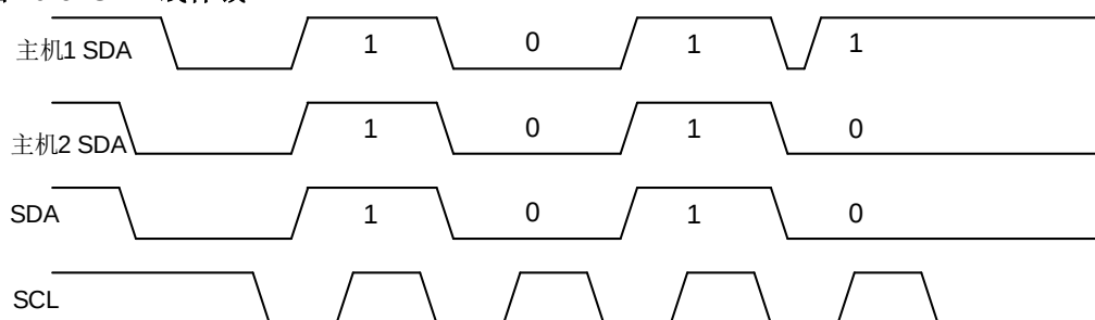
图 20-5. SDA 线仲裁
