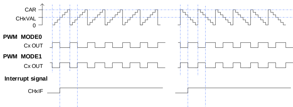
图 18-38. EAPWM 时序图
