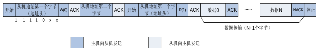
图 20-8. 10 位地址的 I2C 通讯流程（主机接收）
