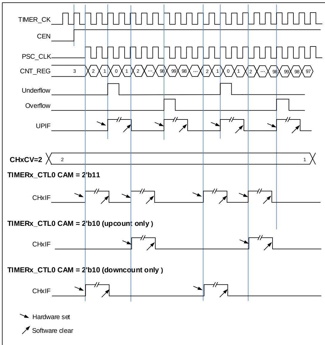
图 18-35. 中央计数模式计数器时序图
