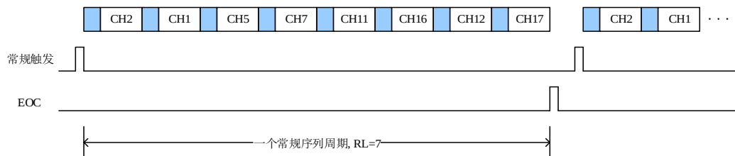
图 14-4. 扫描运行模式，且连续转换模式失能
