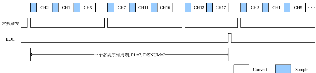
图 14-6. 中断转换模式
