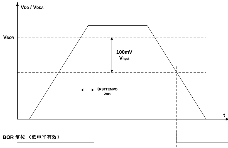
图3-3. BOR波形图
