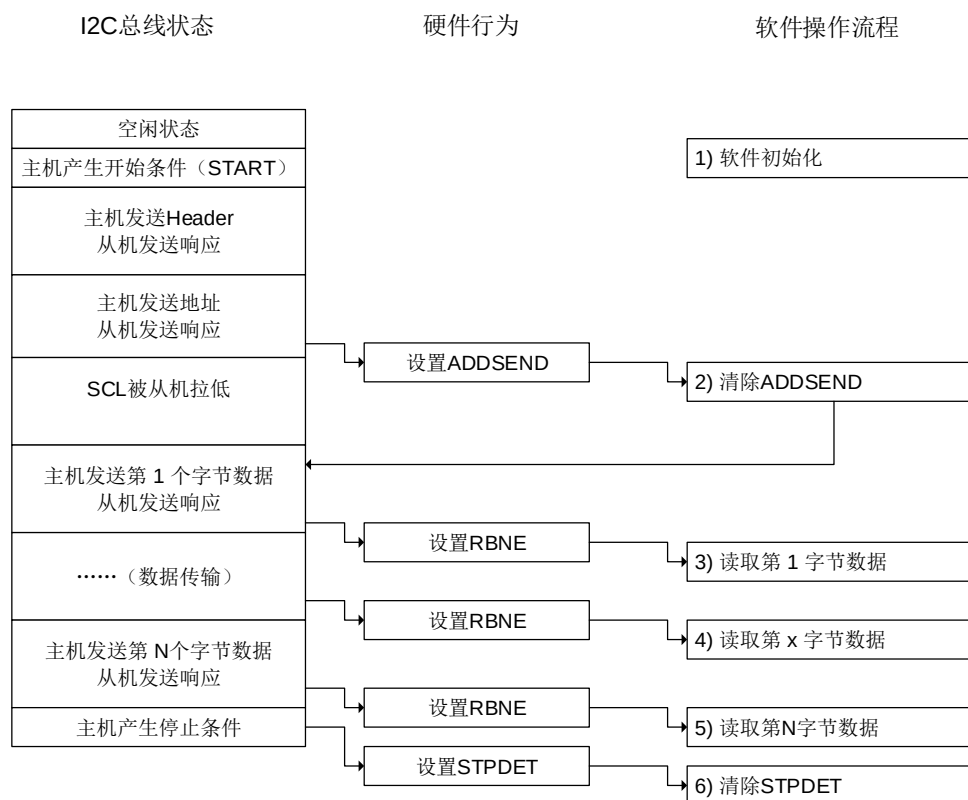
图 20-10. 从机接收模式（10 位地址模式）
