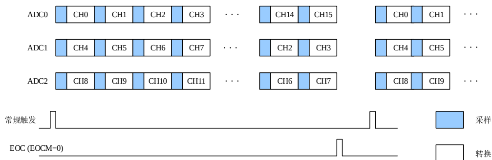
图 14-14. 基于 16 个通道的常规并行模式
