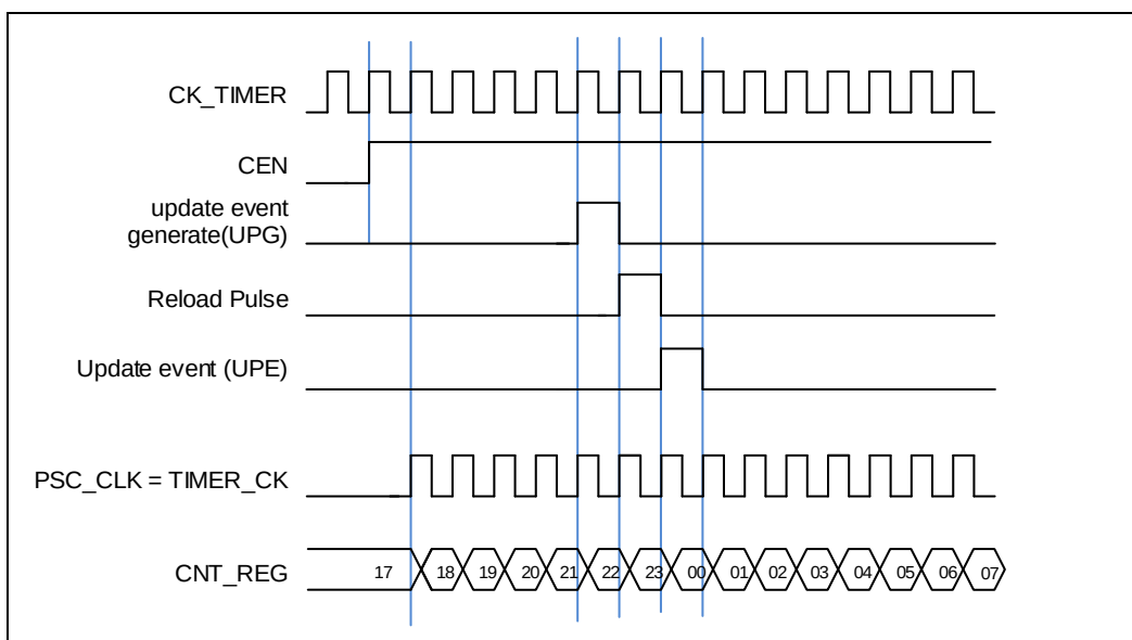
图 18-44. 内部时钟分频为 1 时，计数器的时序图
