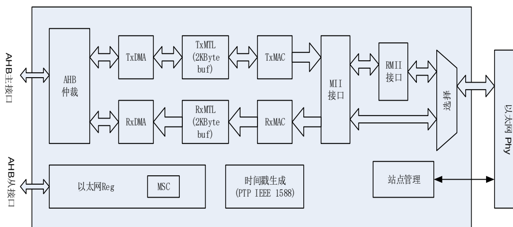
图 27-1. 以太网模块框图
