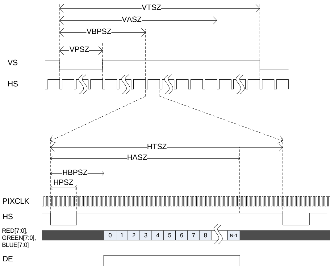
图 23-2. 显示时序图
