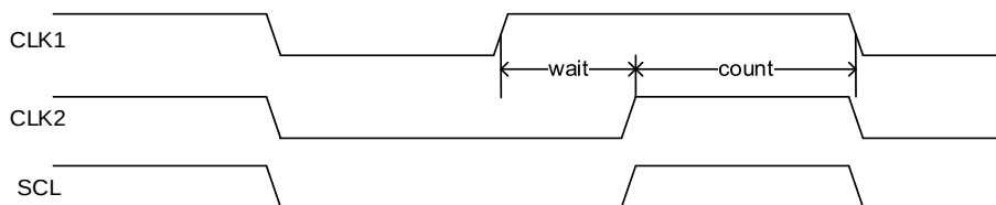
图 20-4. 时钟同步
