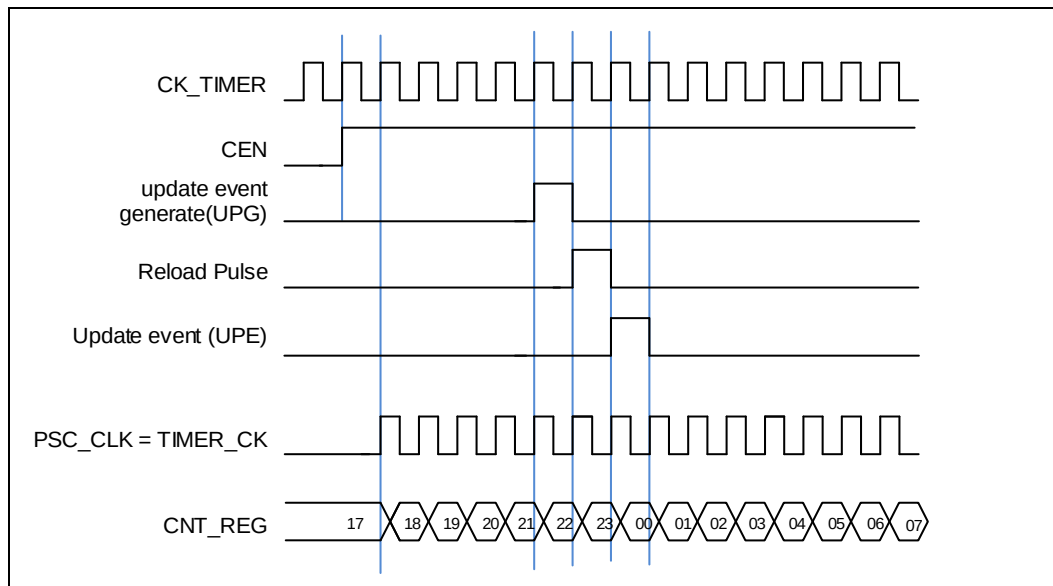
图 18-57. 内部时钟分频为 1 时，计数器的时序图
