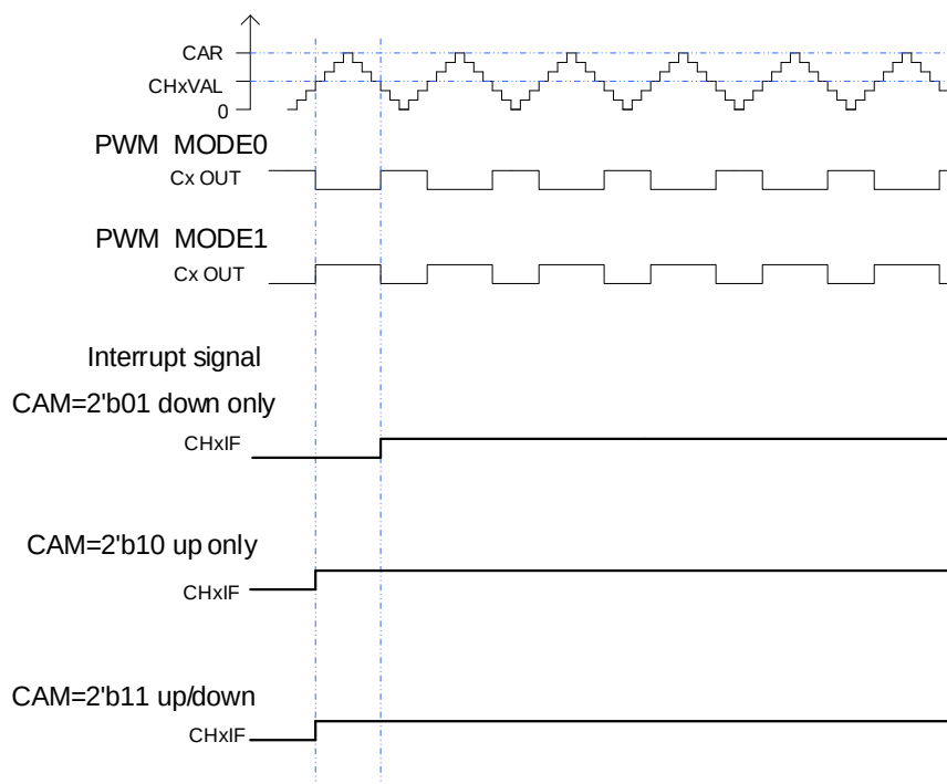
图 18-39. CAPWM 时序图
