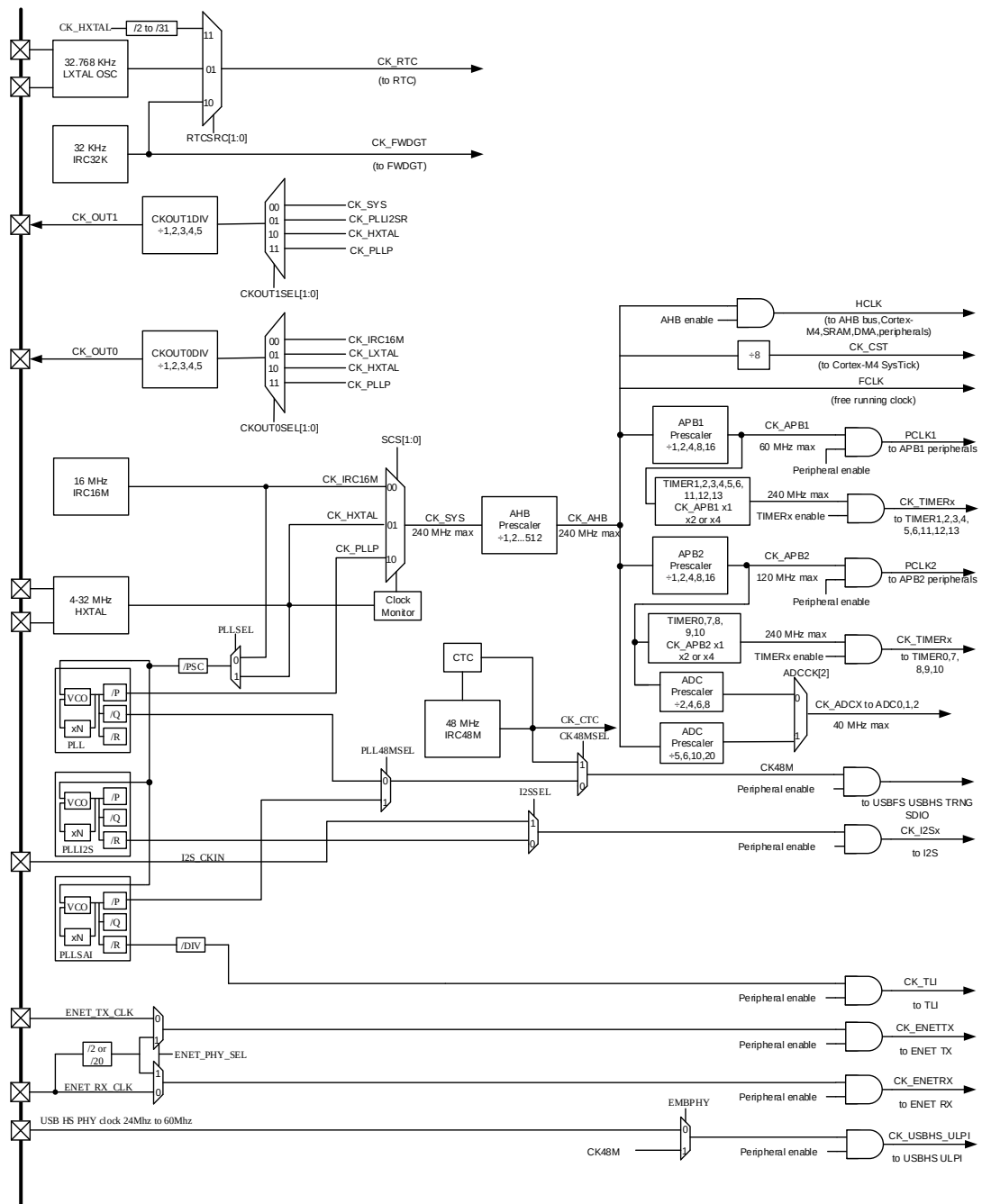
图4-2. 时钟树
