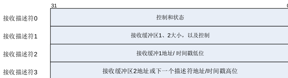
图 27-9. 常规接收描述符
