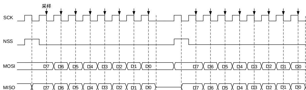
图 17-11. 主机 TI 模式在不连续发送时的时序图
