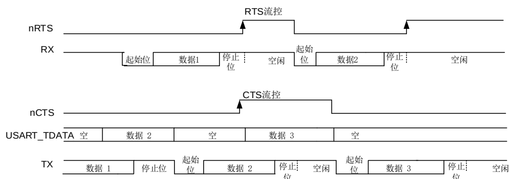
图 15-8. 硬件流控制
