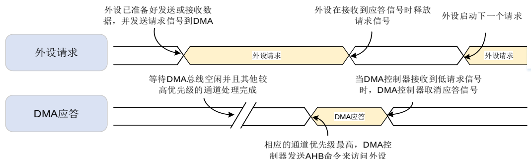
图 9-2. 握手机制
