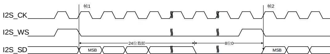
图 17-42. PCM 标准短帧同步模式时序图 (DTLEN=01, CHLEN=1, CKPL=0)
