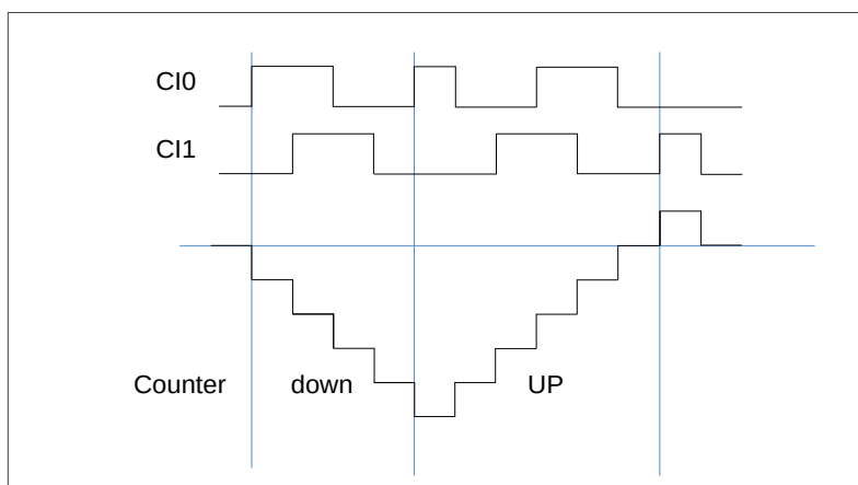
图 14-56. CI0FE0 极性反相的正交译码器接口模式下的例子
