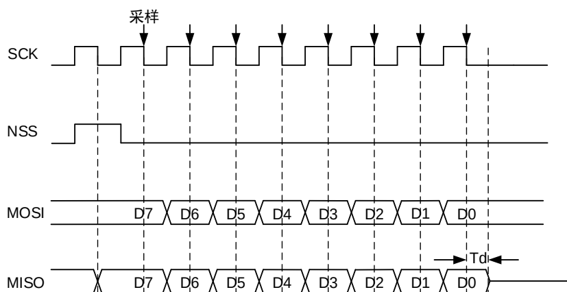
图 17-13. 从机 TI 模式时序图
