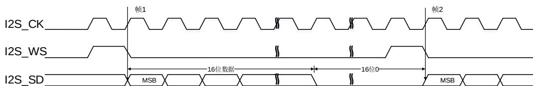
图 17-44. PCM 标准短帧同步模式时序图 (DTLEN=00, CHLEN=1, CKPL=0)
