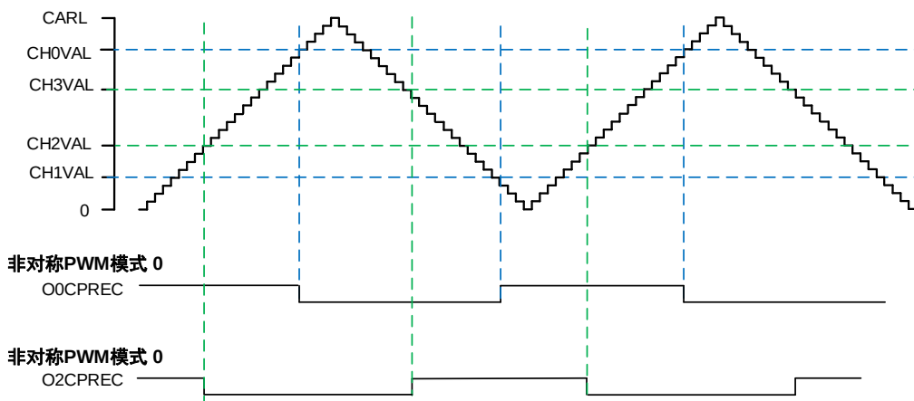
图 14-19. O0CPREC 和 O2CPREC 使用非对称 PWM 模式
