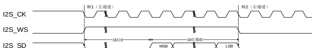
图 17-37. LSB 对齐标准时序图 (DTLEN=00, CHLEN=1, CKPL=1)
