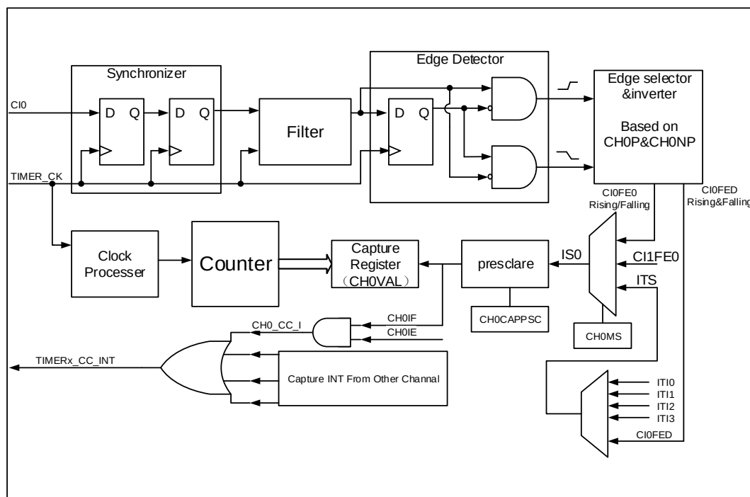
图 14-75. 输入捕获逻辑
