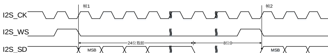
图 17-43. PCM 标准短帧同步模式时序图 (DTLEN=01, CHLEN=1, CKPL=1)
