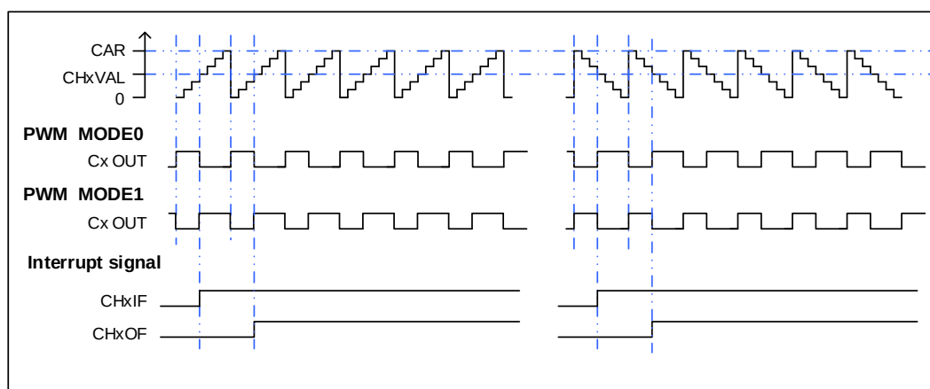
图 14-17. EAPWM 时序图
