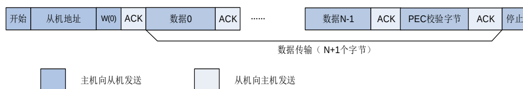
图 16-22. SMBus 主机发送器和从机接收器通信流程
