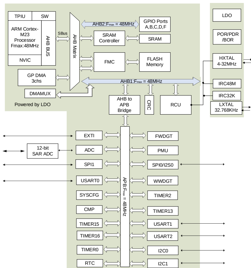
图 1-2. GD32C2x1 系列器件的系统架构示意图
