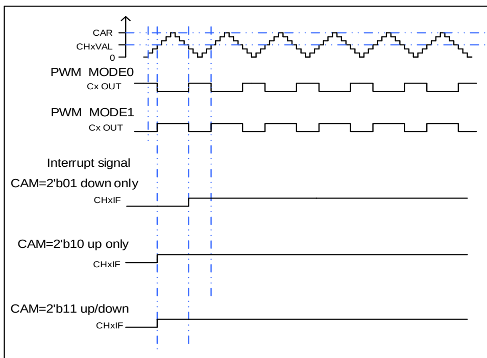
图 14-18. CAPWM 时序图
