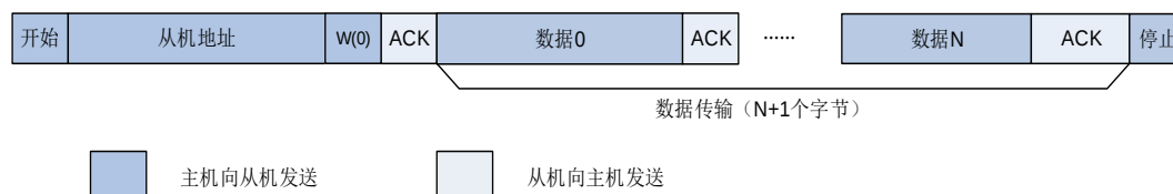
图 16-5. 7 位地址的 I2C 通讯流程（主机发送）
