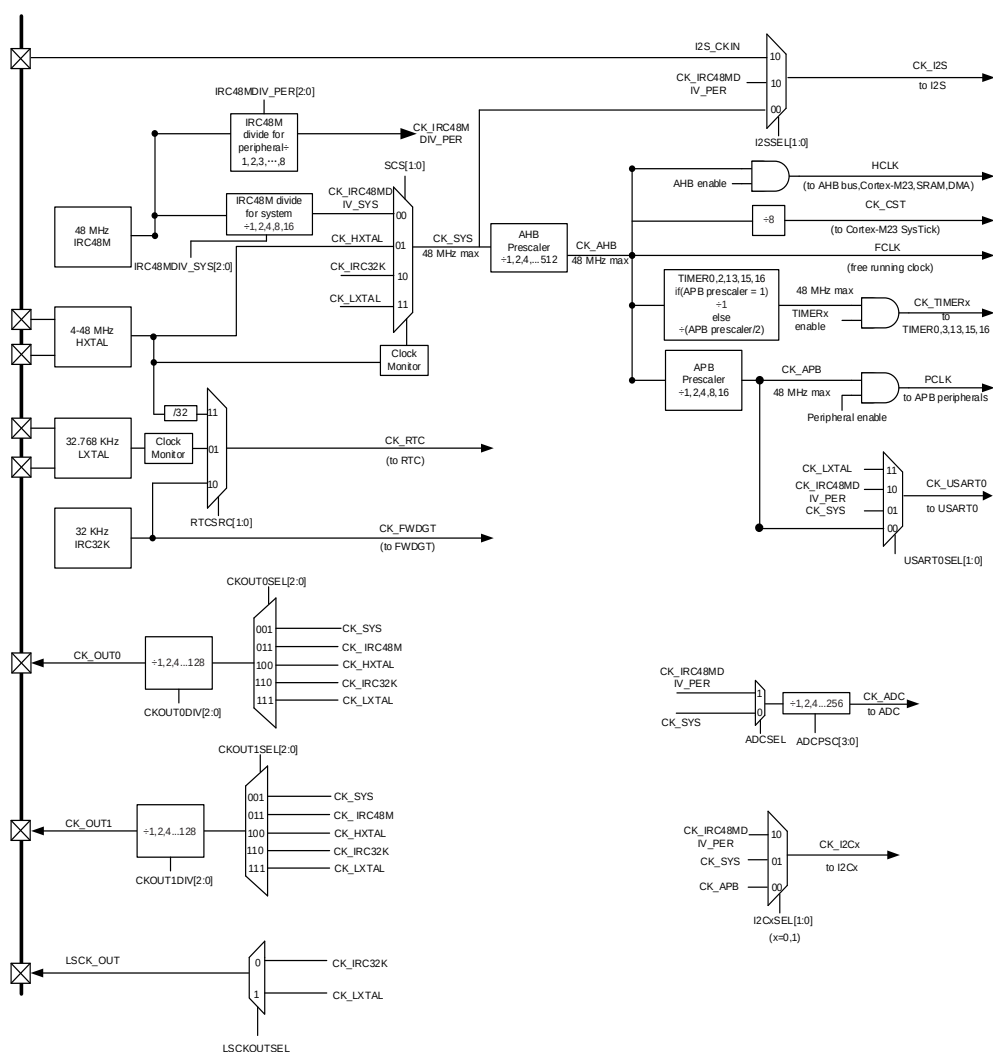
图 4-2. 时钟树
