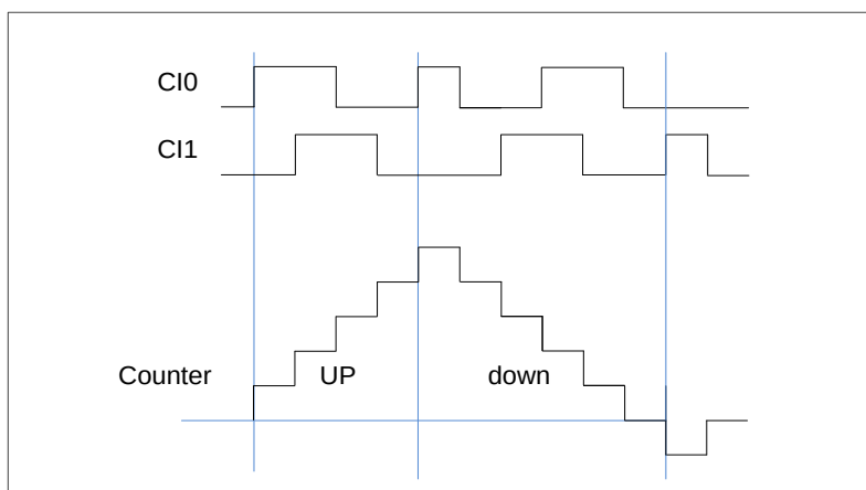
图 14-55. 正交译码器接口模式下计数器运行例子
