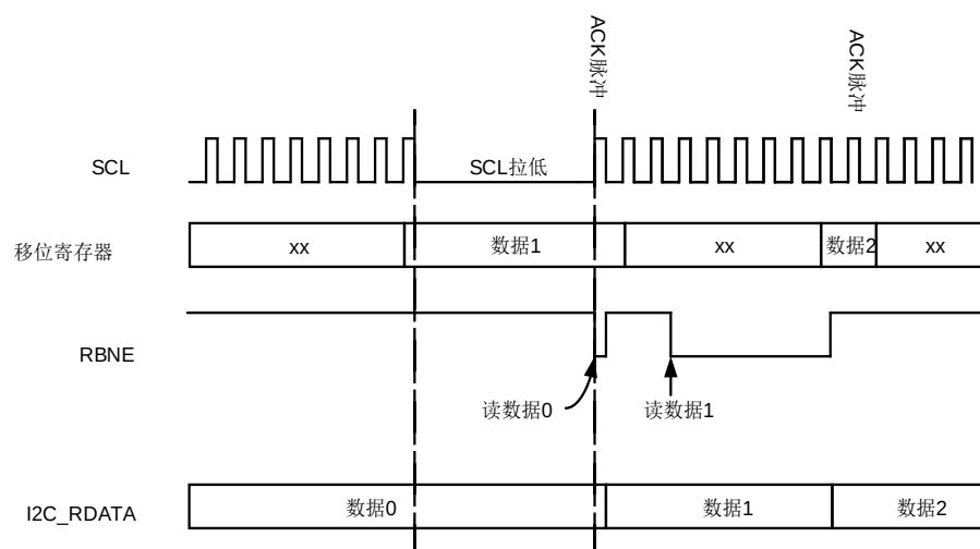
图 16-12. 数据接收
