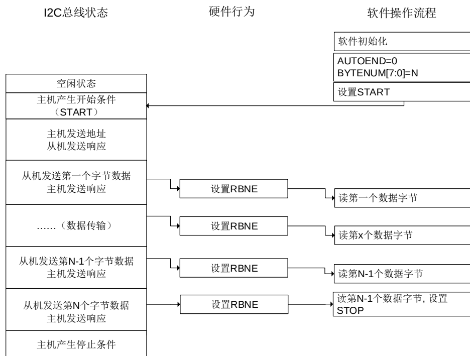
图 16-20. I2C 主机接收编程模型 ( N \leq 255 )
