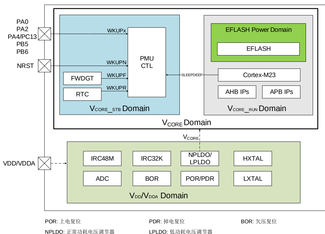
图 3-1. 电源域概览
