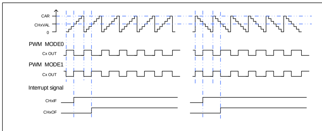
图 14-77. PWM 时序图
