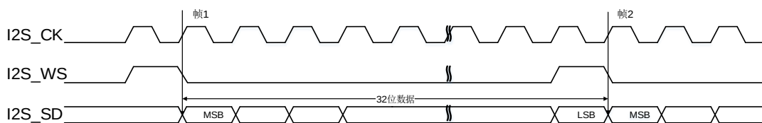
图 17-40. PCM 标准短帧同步模式时序图 (DTLEN=10, CHLEN=1, CKPL=0)
