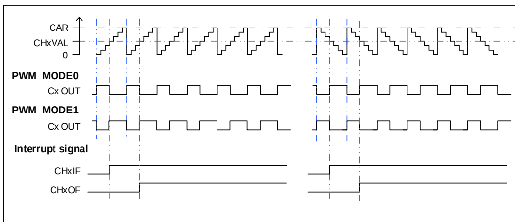
图 14-51. CAPWM 时序图
