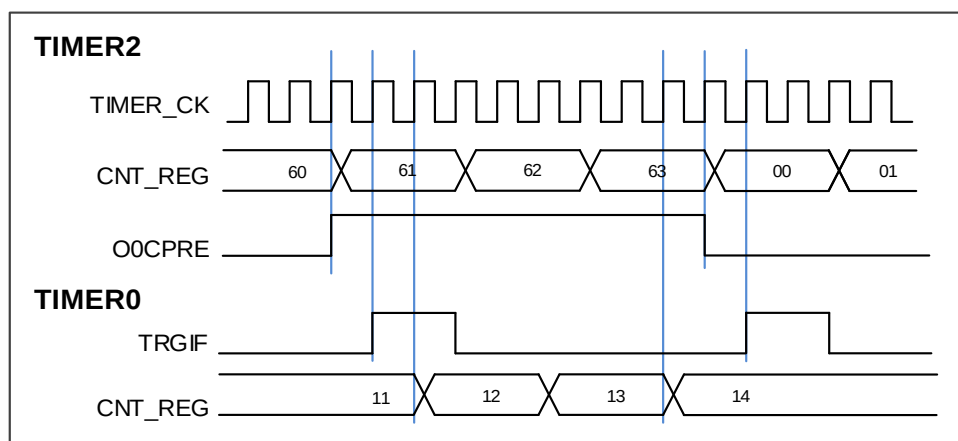
图 14-38. 用定时器 2 的 O0CPRE 信号控制定时器 0 的暂停模式
