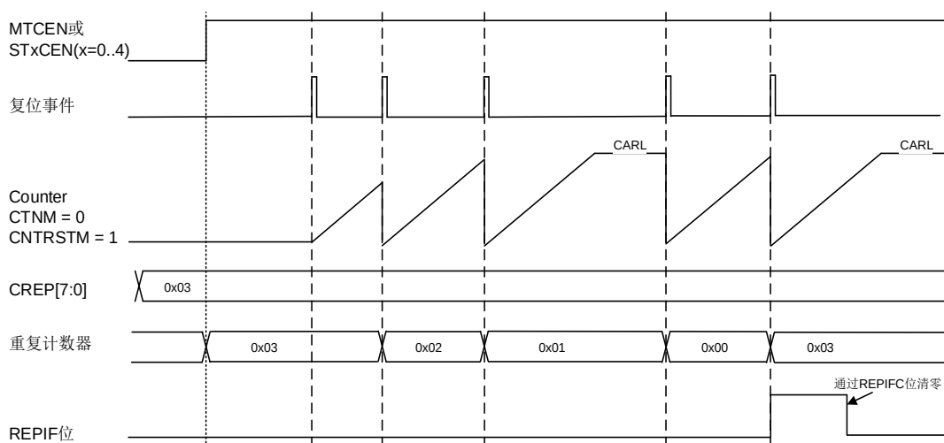
图 19-8. 单脉冲模式下, CNTRSTM = 1 时重复计数器的动作
