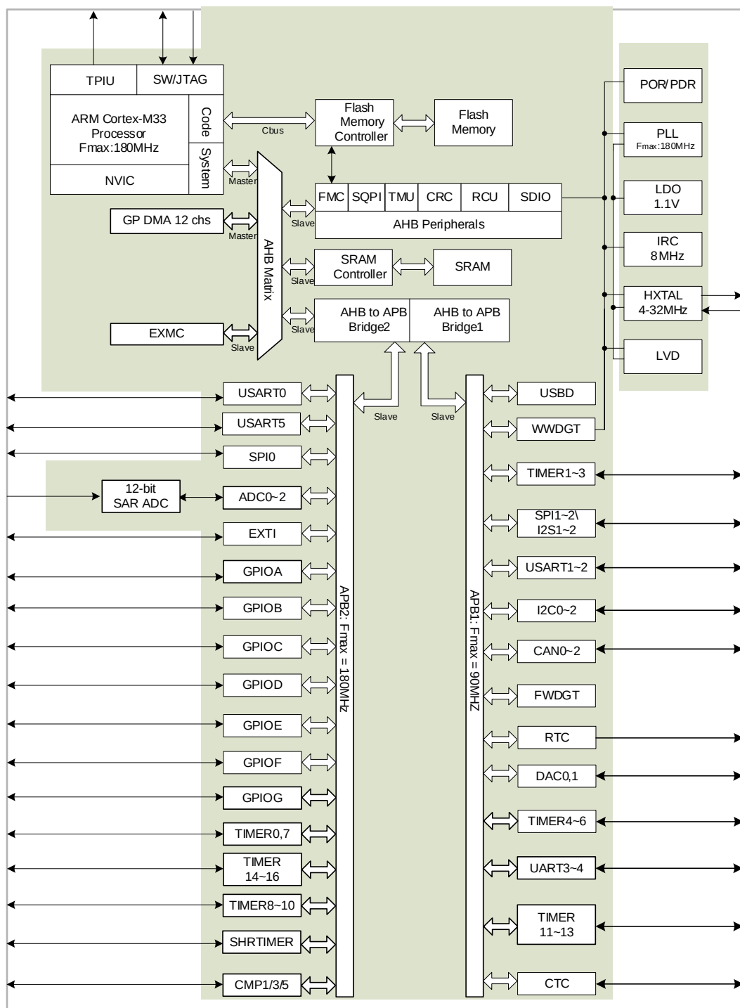
图 1-2. GD32E51x_HD 系列器件的系统架构示意图
