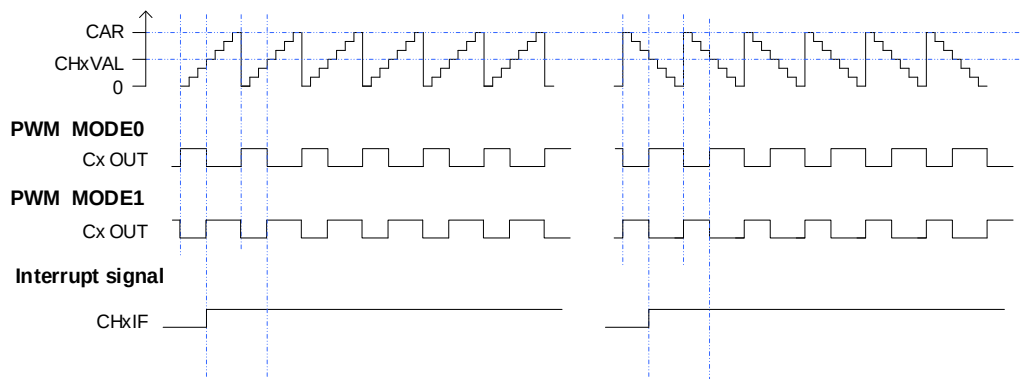
图 18-42. CAPWM 时序图
