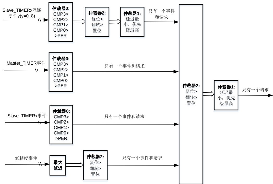
图 19-19. 每个 t_{SHRTIMER\_CK} 周期的仲裁机制过程
