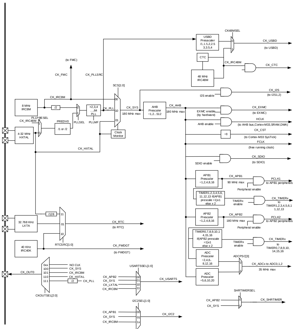
图 5-2. 时钟树
