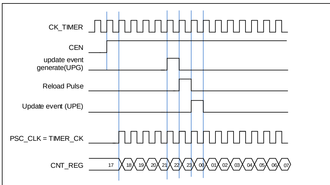
图 18-99. 内部时钟分频为 1 时，计数器的时序图
