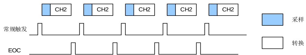
图 13-3. 单次运行模式
