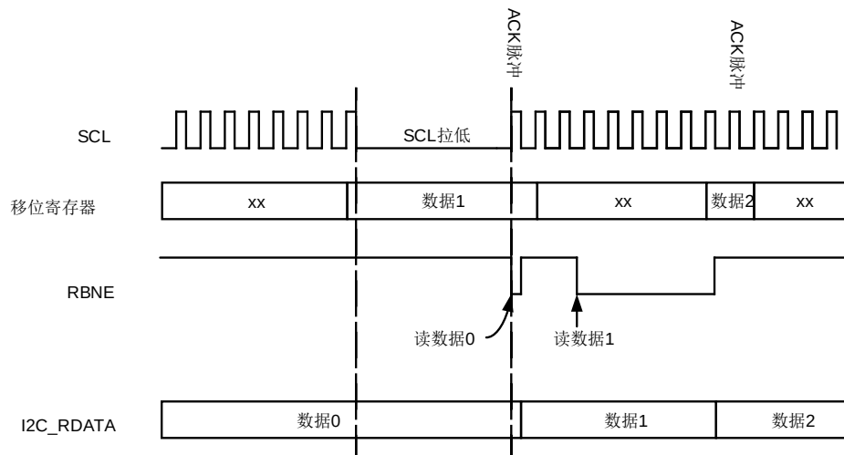
图 21-25. 数据接收
