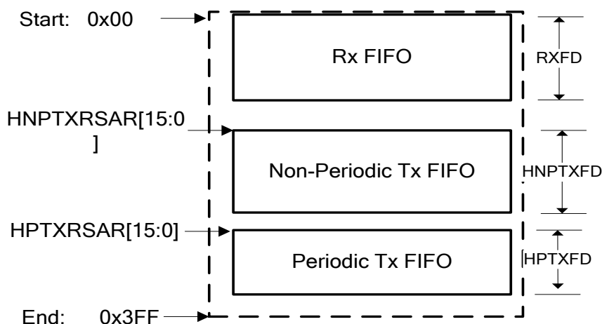
图 29-6. 主机模式 FIFO 空间
