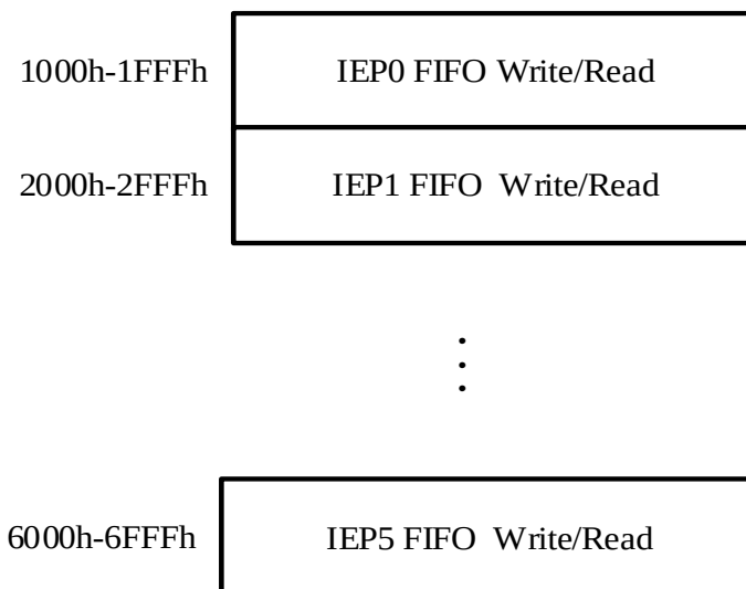
图 29-9. 设备模式 FIFO 访问寄存器映射表
