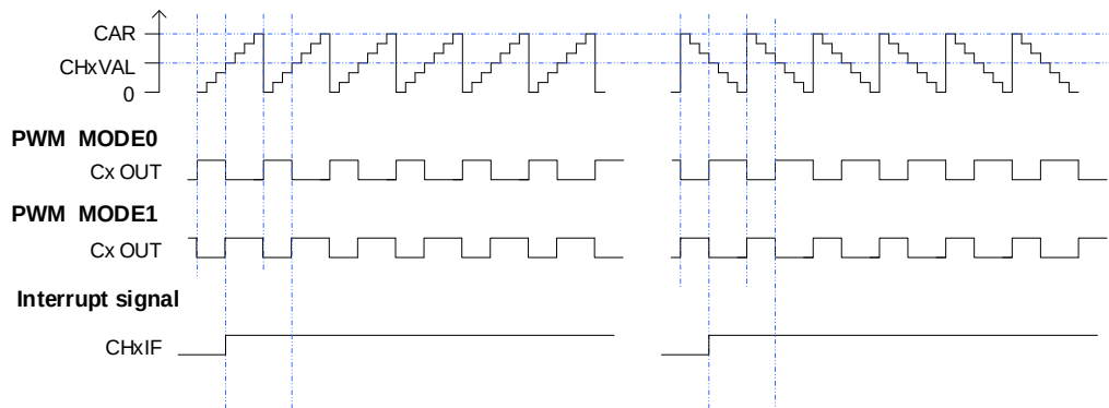
图 18-42. CAPWM 时序图
