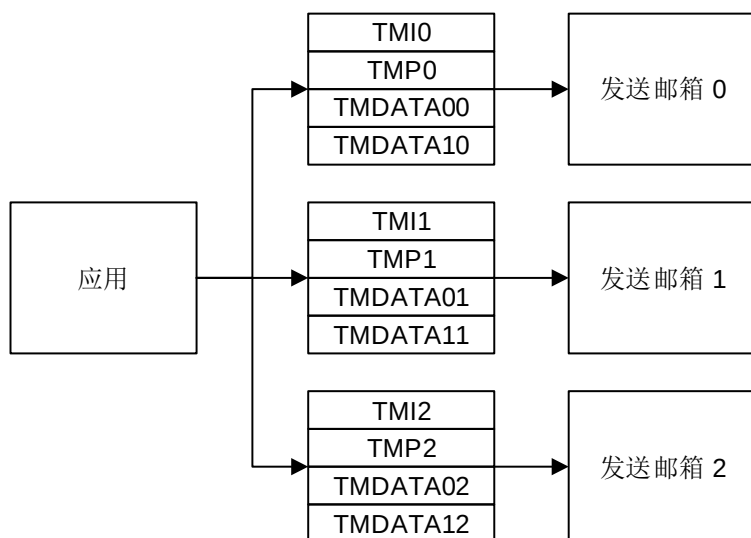
图 26-2. 发送寄存器
