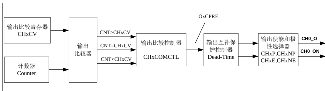
图 18-92. 通道输出比较原理（带有互补输出的通道，x=0）
