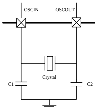
图 5-7. HXTAL 时钟源
