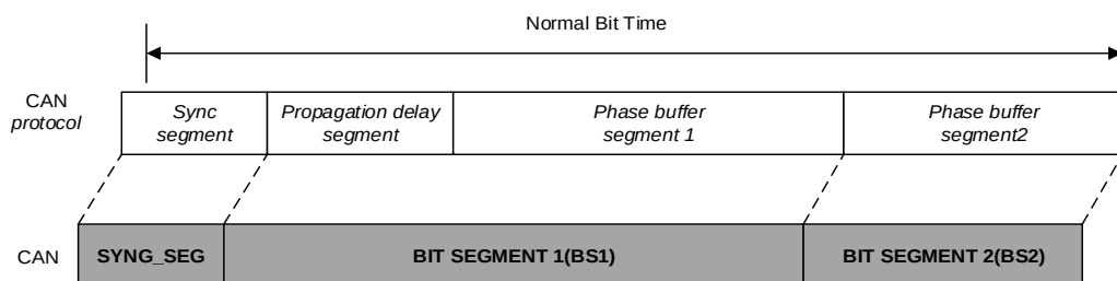
图 26-11. 位时序
