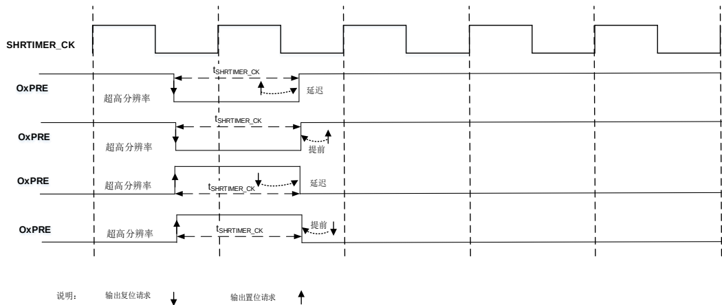
图 19-21. 脉冲宽度为 1 个 t_{SHRTIMER\_CK} 周期
