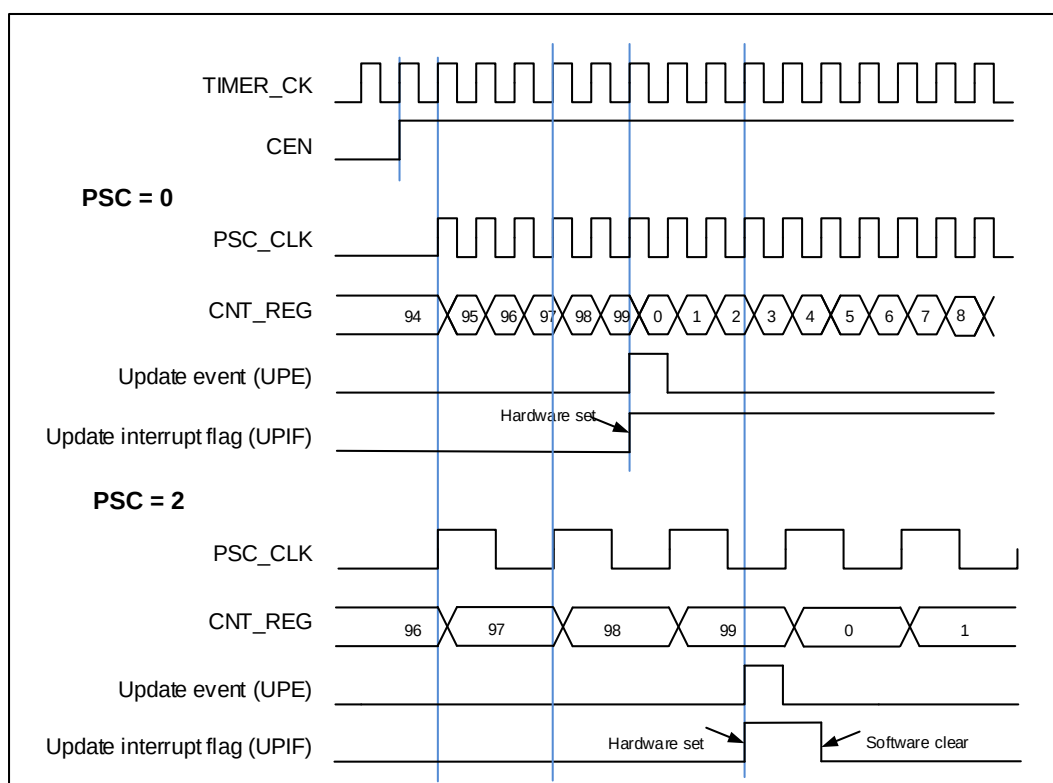
图 18-101. 向上计数时序图， PSC=0/2
