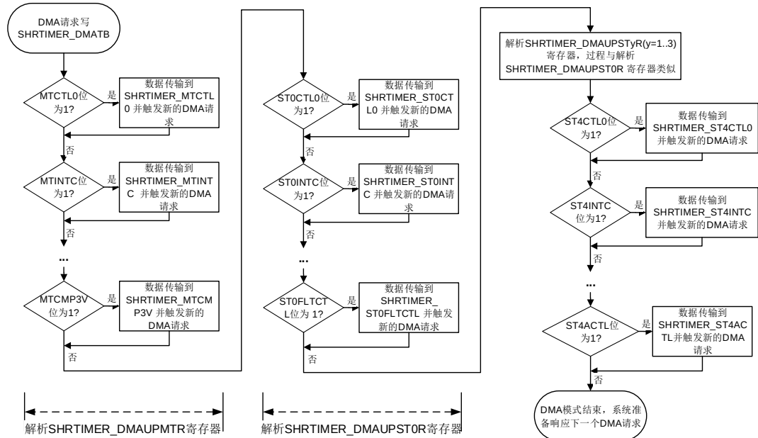
图 19-48. DMA 模式运行流程图
