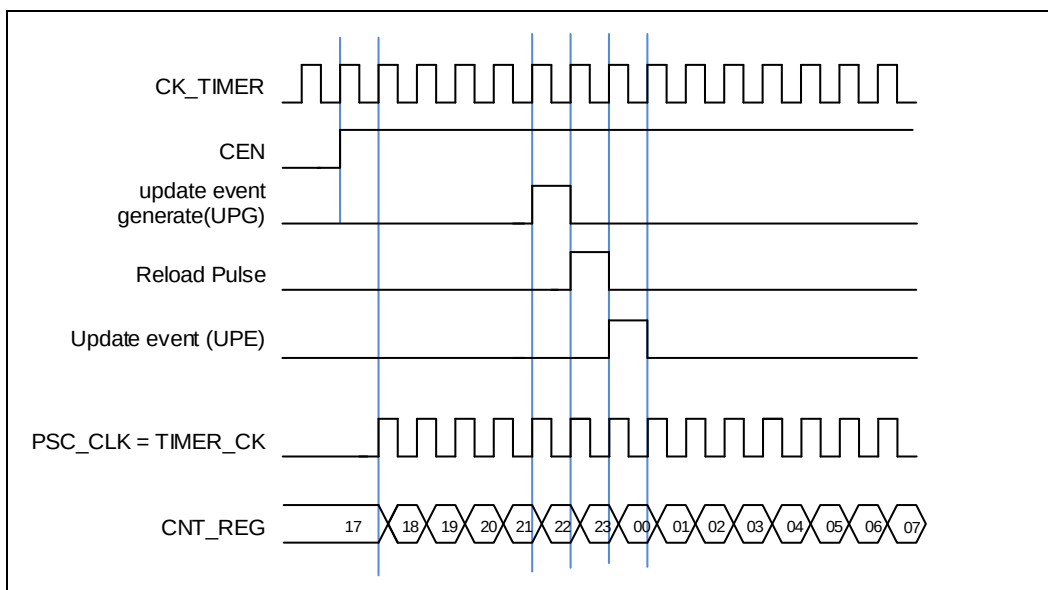
图 18-86. 内部时钟分频为 1 时，计数器的时序图
