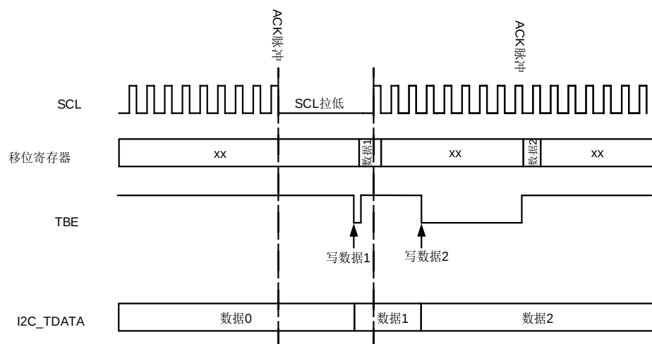
图 21-24. 数据发送
