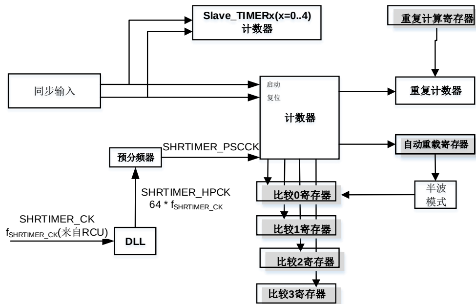
图 19-2. Master_TIMER 结构图
