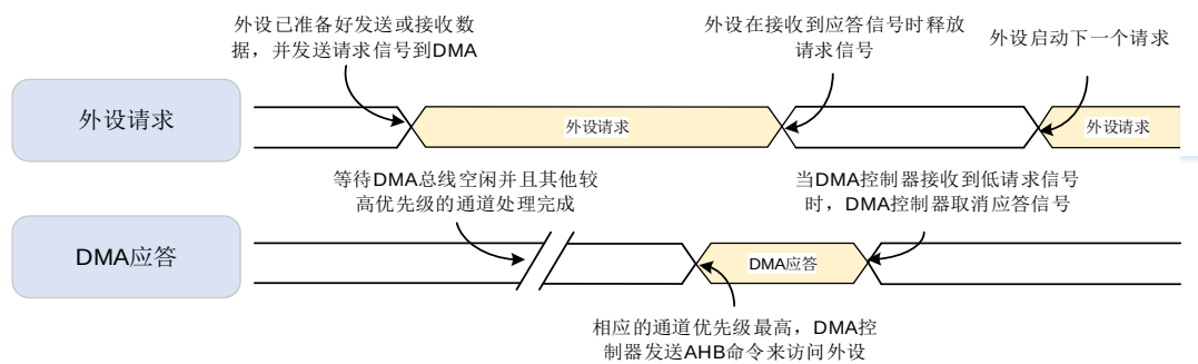
图 11-2. 握手机制
