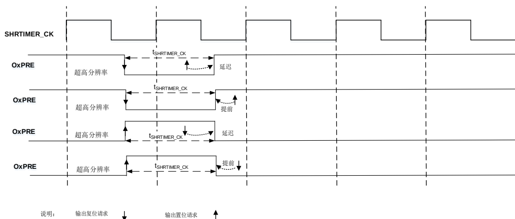
图 19-21. 脉冲宽度为 1 个 t_{SHRTIMER\_CK} 周期
