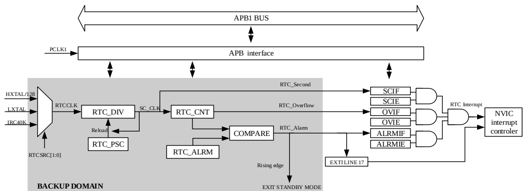
图 17-1. RTC 框图
