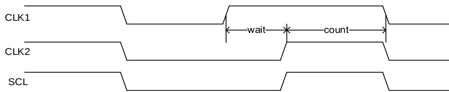
图 21-4. 时钟同步
