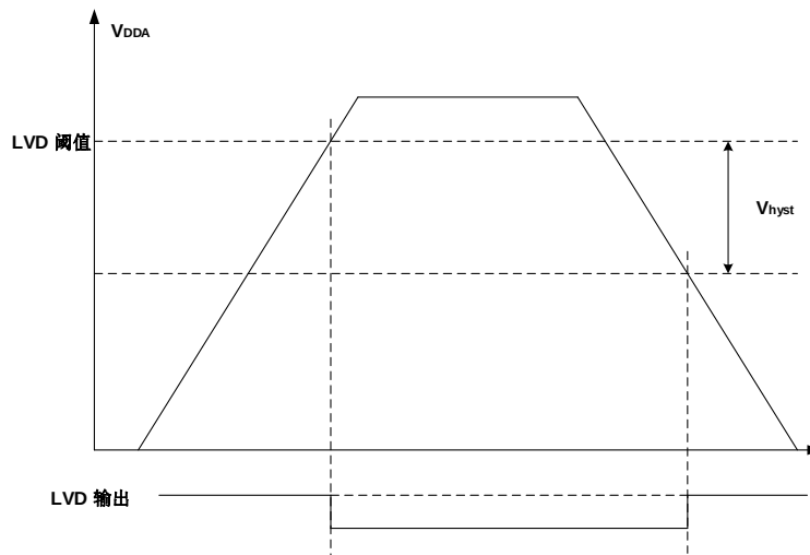
图 4-5. LVD 阈值波形图
