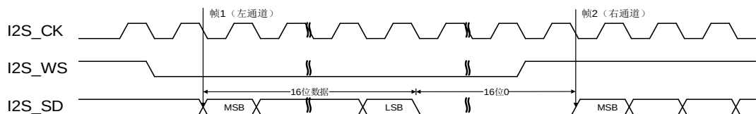
图 22-21. I2S 飞利浦标准时序图 (DTLEN=00, CHLEN=1, CKPL=0)
