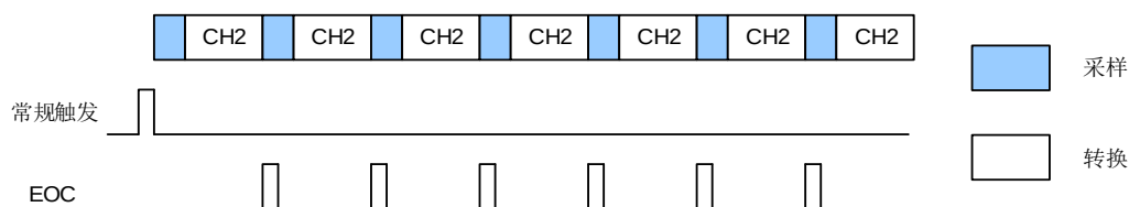
图 13-4. 连续运行模式
