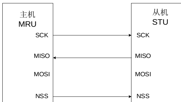
图 22-6. 典型的单工模式连接（主机：只发送，从机：接收）
