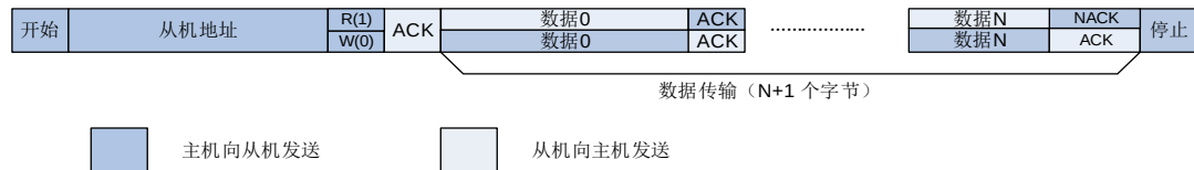
图 21-7. 10 位地址的 I2C 通讯流程（主机发送）
