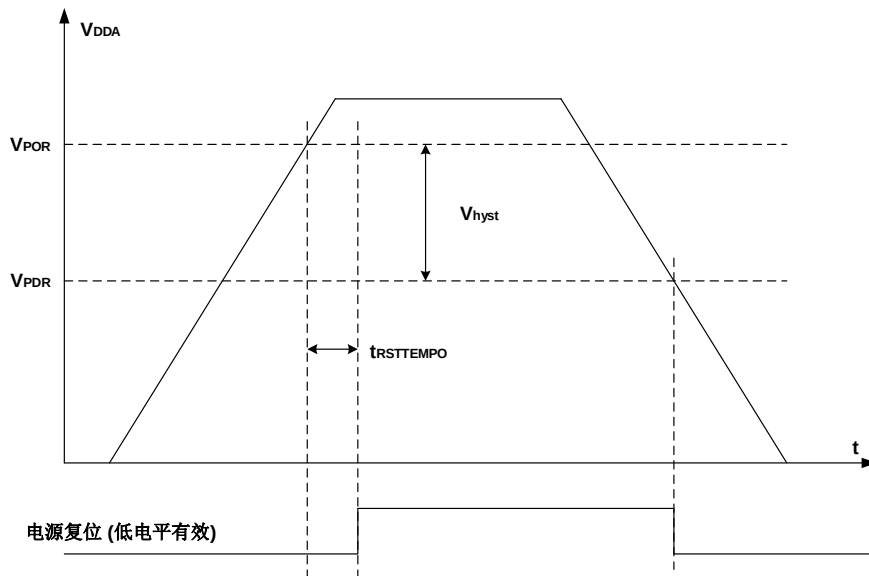
图 4-4. 上电/掉电复位波形图
