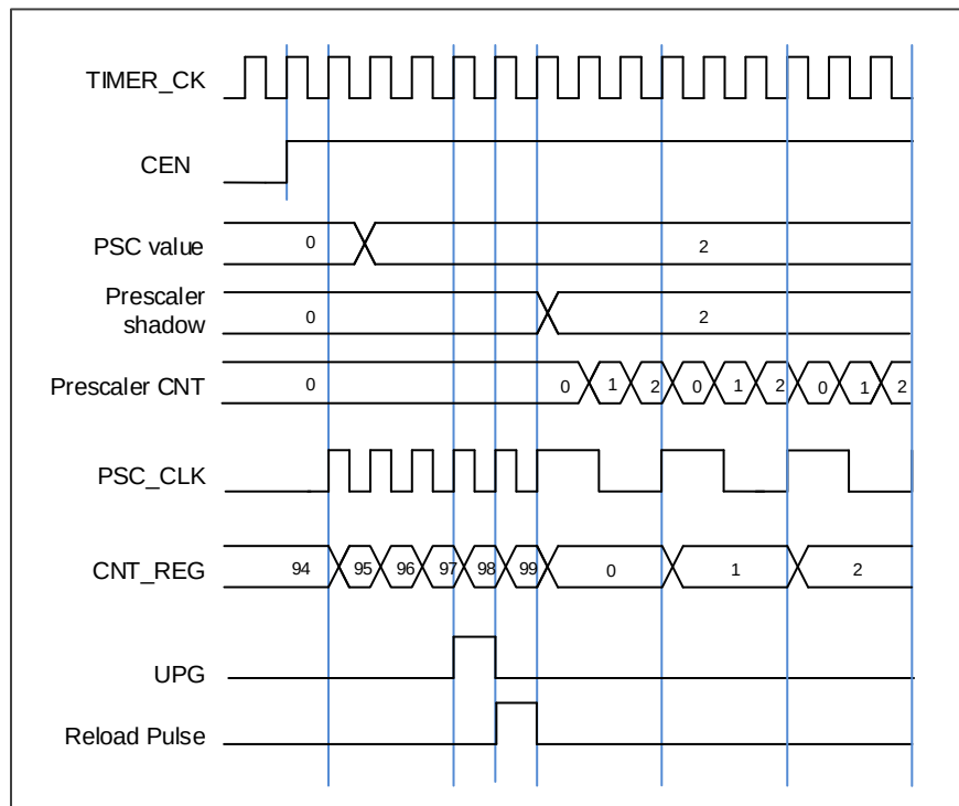
图 18-100. 当 PSC 数值从 0 变到 2 时，计数器的时序图
