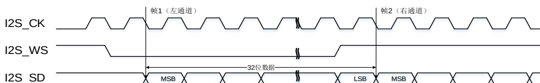
图 22-17. I2S 飞利浦标准时序图 (DTLEN=10, CHLEN=1, CKPL=0)
