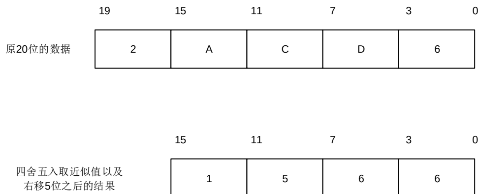
图 13-11. 右移 5 位和取整的数例
