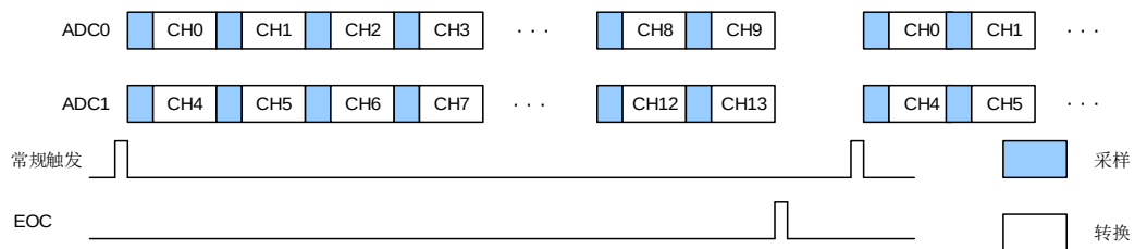
图 13-13. 基于 10 个通道的常规并行模式
