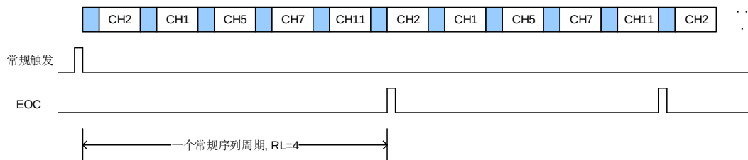
图 13-6. 扫描运行模式，连续运行模式使能
