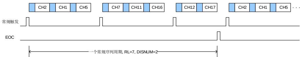
图 13-7. 间断运行模式
