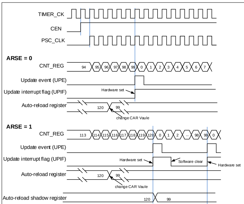
图 18-102. 向上计数时序图，在运行时改变 TIMERx_CAR 寄存器的值
