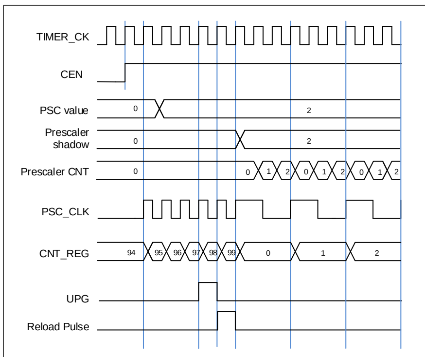
图 18-62. 当 PSC 数值从 0 变到 2 时，计数器的时序图
