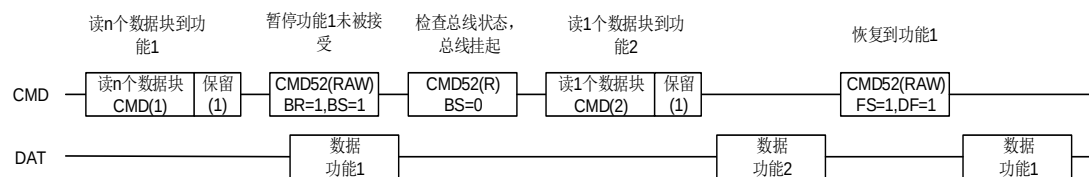
图 24-14. 在功能 1 的多块读周期期间插入功能 2 读周期
