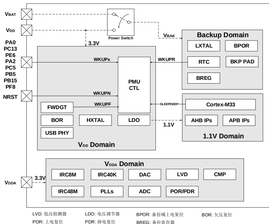
图 4-2. 1.1V 电源域概览
