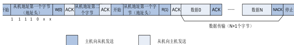
图 21-20. 10 位地址的 I2C 通讯流程（主机接收，HEAD10R=0）
