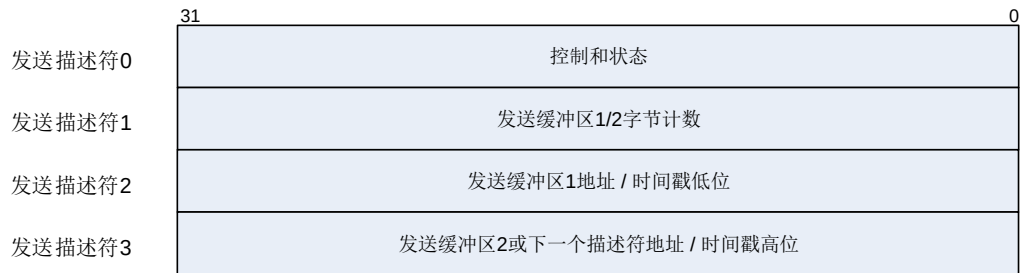
图 27-7. 常规发送描述符
