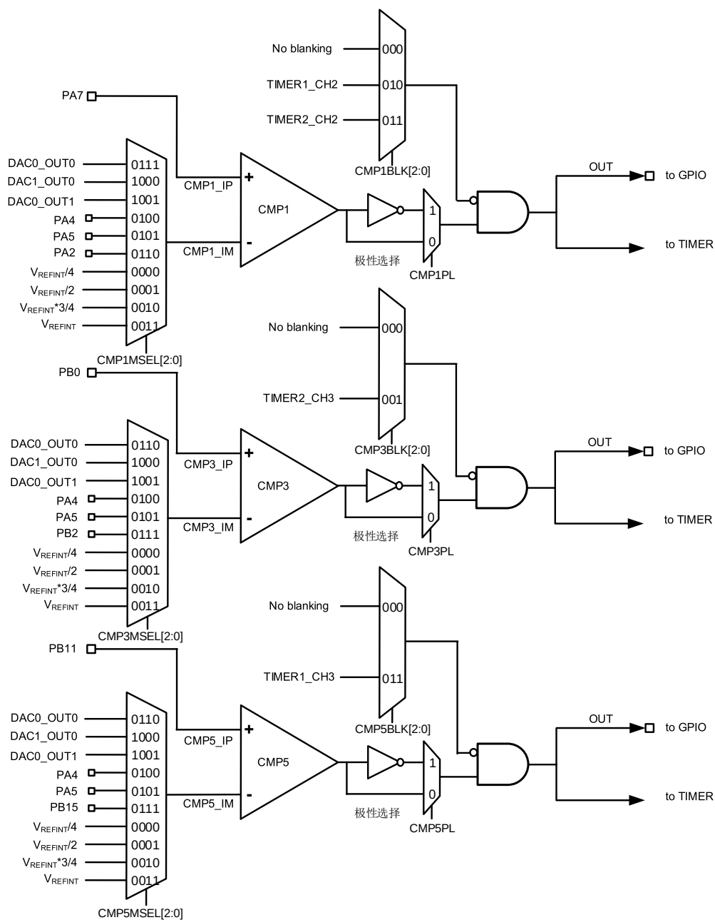
图 15-1. 比较器框图
