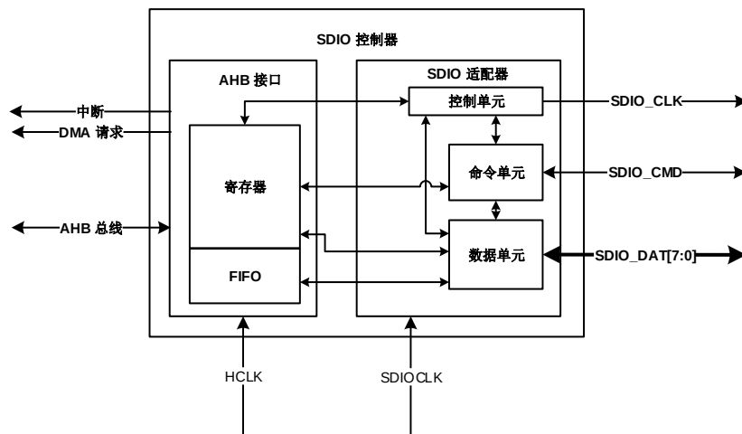
图 24-6. SDIO 框图
