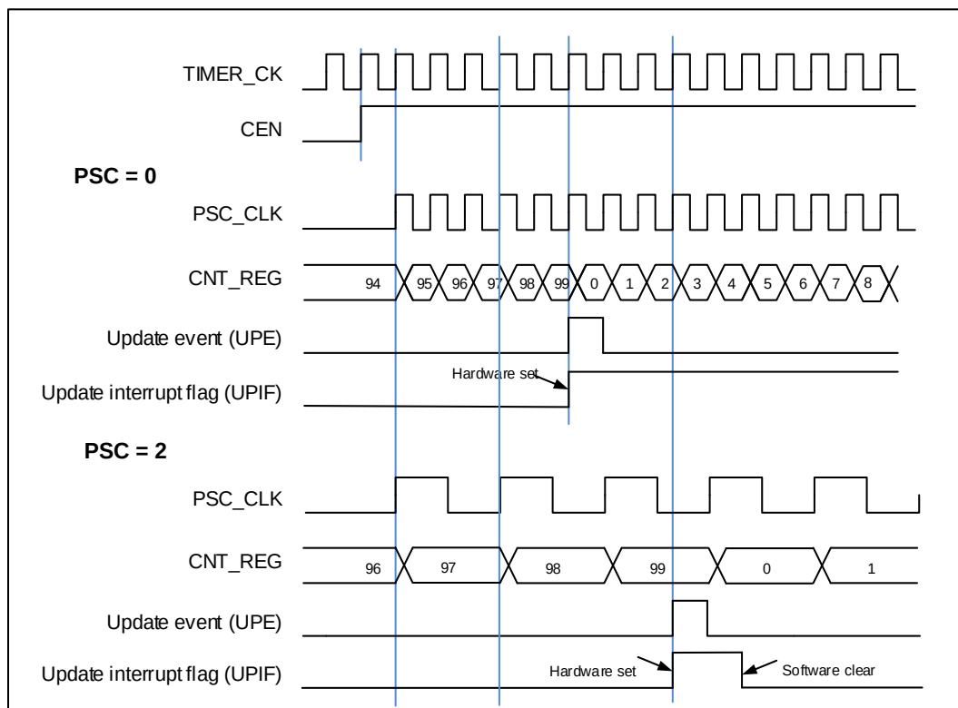
图 18-88. 向上计数时序图， \text{PSC}=0/2
