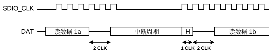
图 24-13. 使用 SDIO_DAT[2]信号线的读等待操作
