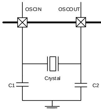
图 5-3. HXTAL 时钟源
