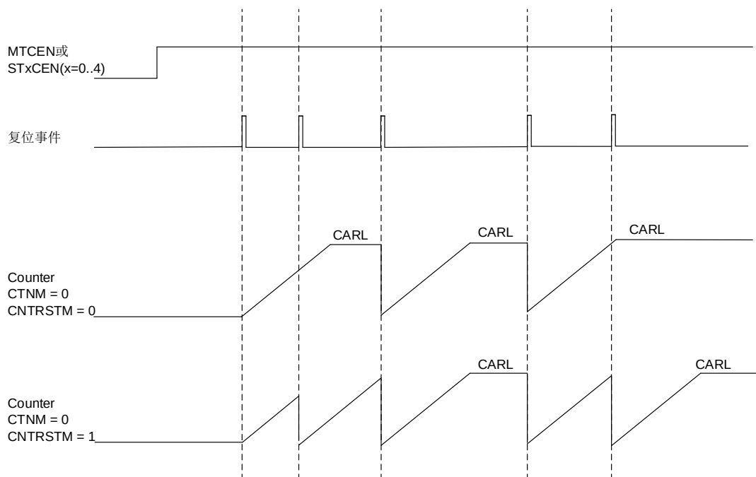
图 19-4. 单脉冲模式下计数器的动作
