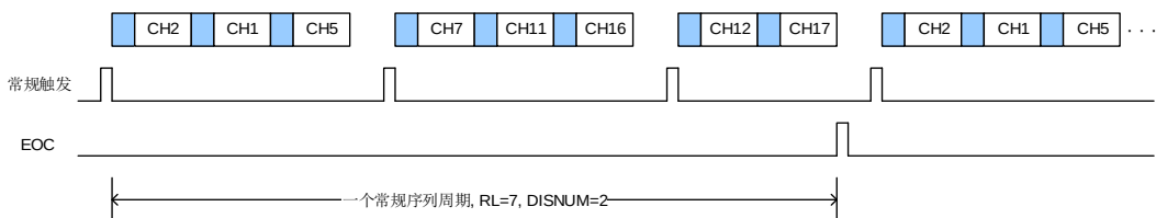
图 13-7. 间断运行模式
