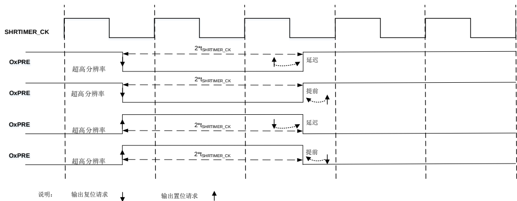
图 19-22. 脉冲宽度为 2 个 t_{SHRTIMER\_CK} 周期
