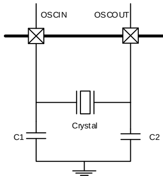
图 5-3. HXTAL 时钟源
