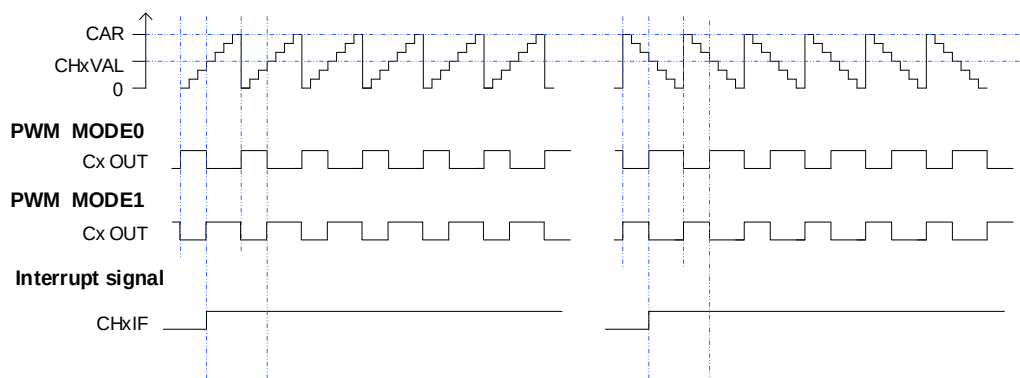
图 18-17. CAPWM 时序图
