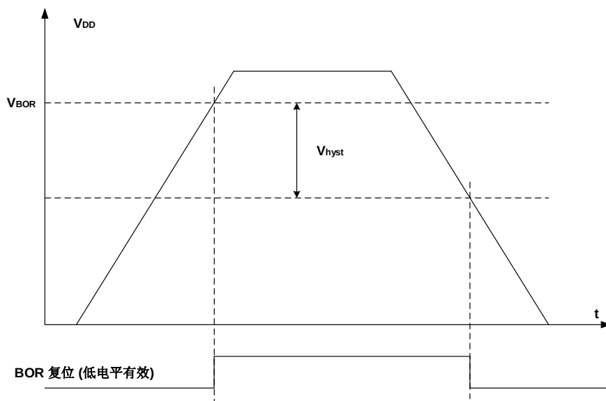
图 4-3. BOR 波形图
