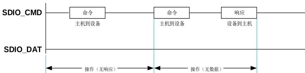
图 24-1. SDIO “无响应” 和 “无数据” 操作
