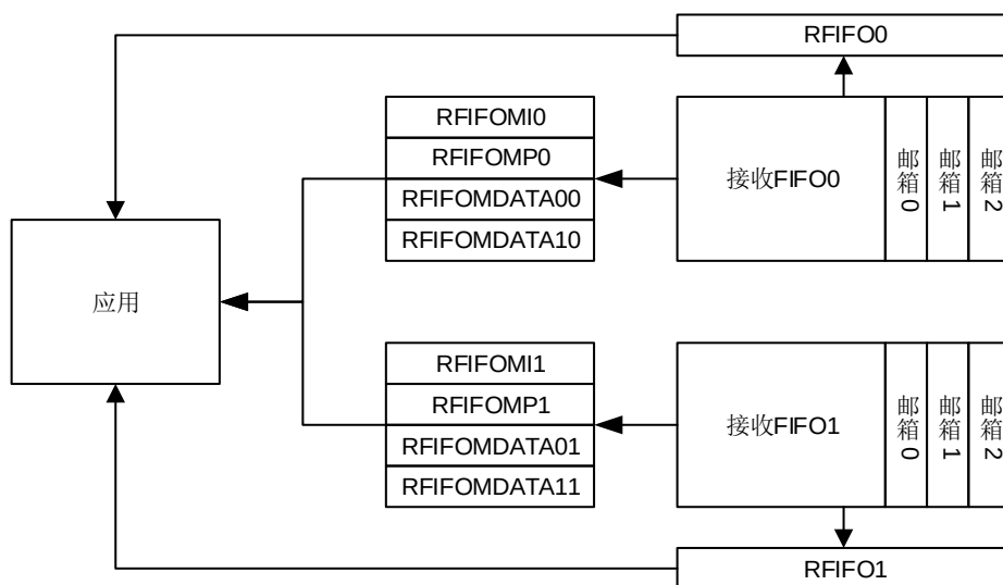
图 26-4. 接收寄存器
