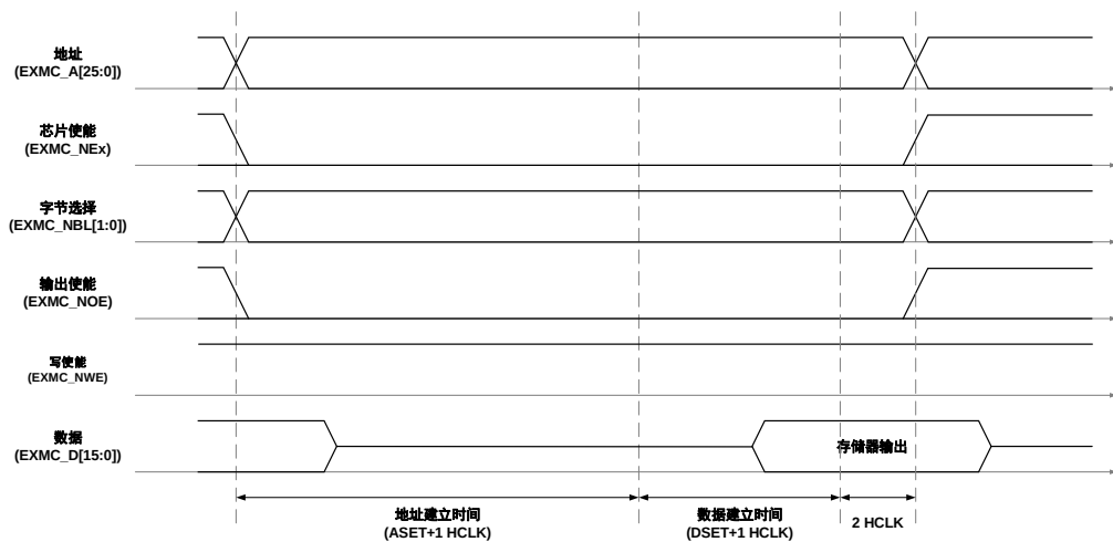
图 25-7. 模式 1 写时序
