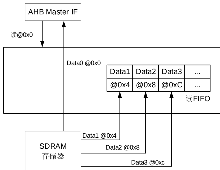
图 25-33. FIFO 未命中时的读访问（BRSTRD=1，CL=2，SDCLK=2，PIPED=2）
