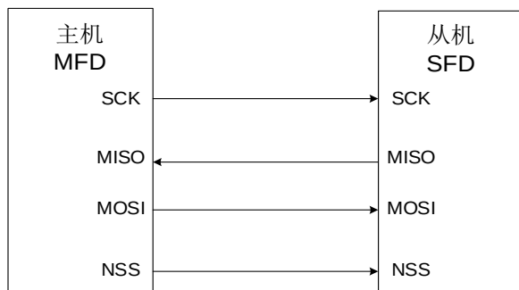
图 21-4. 典型的全双工模式连接
