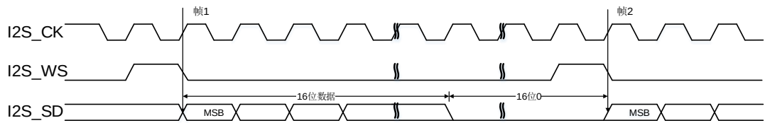
图 21-41. PCM 标准短帧同步模式时序图 (DTLEN=00, CHLEN=1, CKPL=1)
