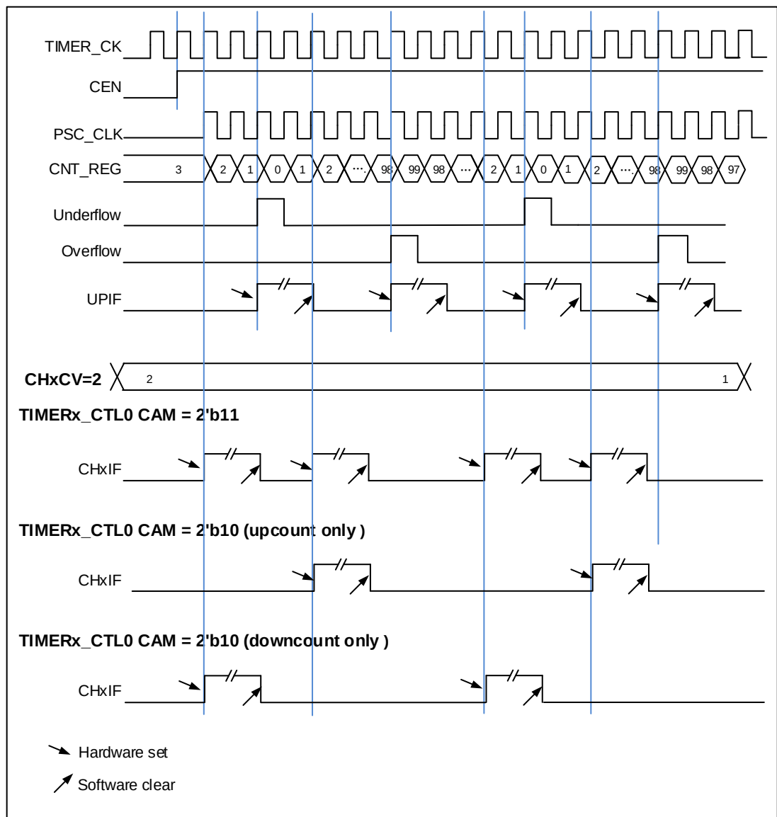
图 18-35. 中央计数模式计数器时序图
