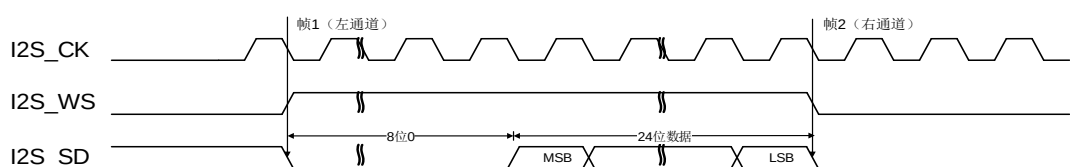
图 21-30. LSB 对齐标准时序图 (DTLEN=01, CHLEN=1, CKPL=0)
