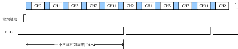
图 14-5. 扫描运行模式，连续运行模式使能
