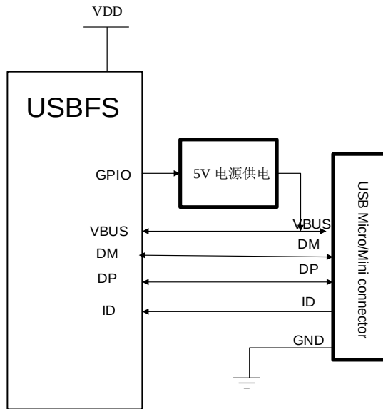
图 28-3. OTG 模式下连接示意图
