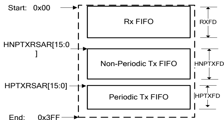
图 29-6. 主机模式 FIFO 空间
