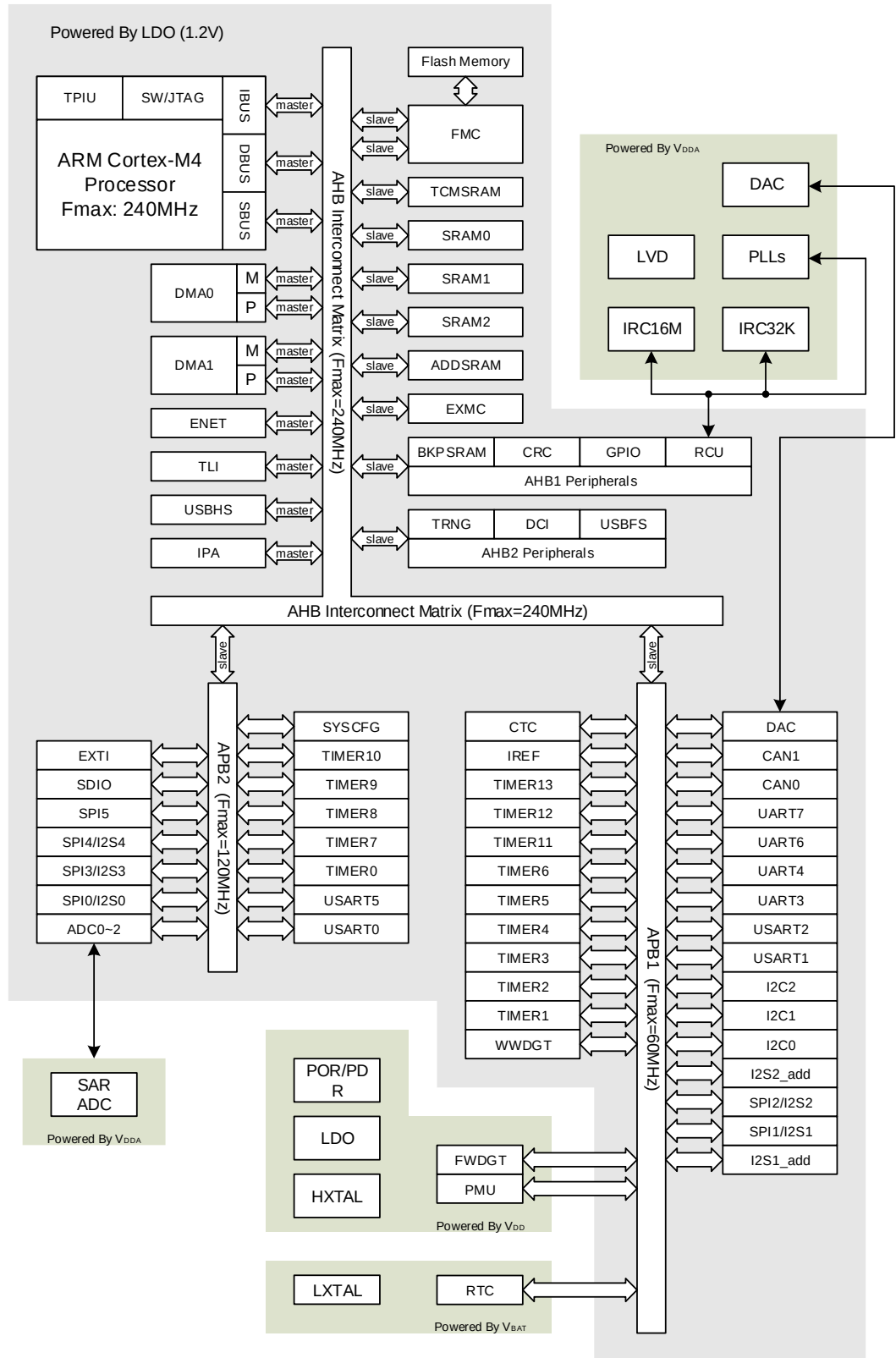
图 1-2. GD32A490xx 器件的系统架构示意图
