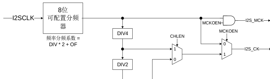
图 21-50. I2S 时钟生成结构框图
