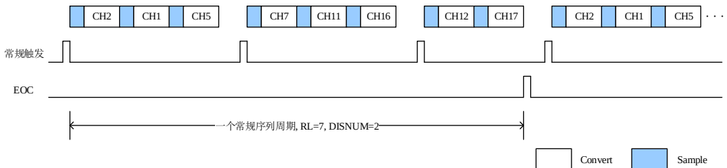
图 14-6. 间断转换模式
