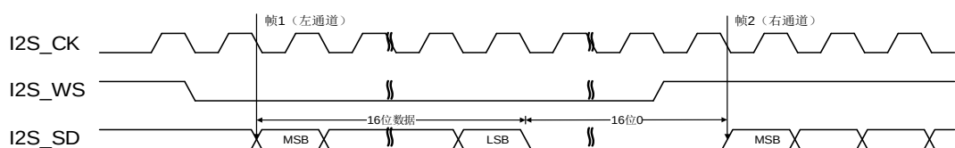
图 21-20. I2S 飞利浦标准时序图 (DTLEN=00, CHLEN=1, CKPL=0)
