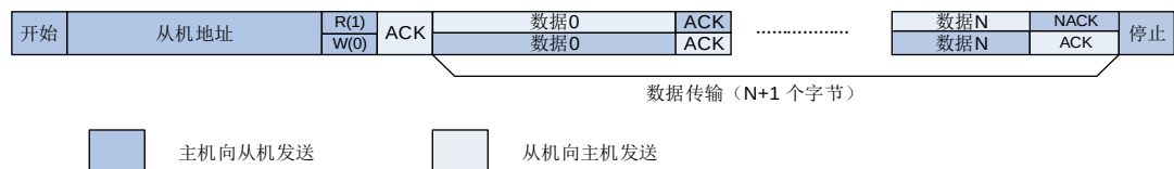
图 20-6. 7 位地址的 I2C 通讯流程
