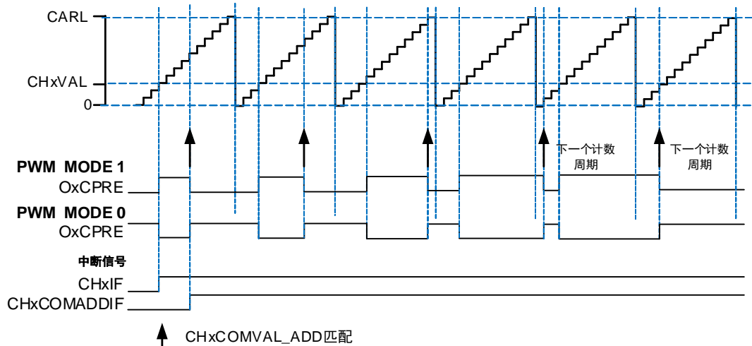
图 24-67. 通道 x 输出 PWM 占空比随着 CHxCOMVAL_ADD 值而改变
