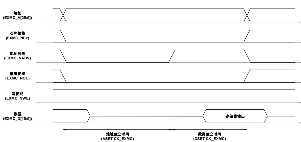
图 38-12. 模式 2 写时序
