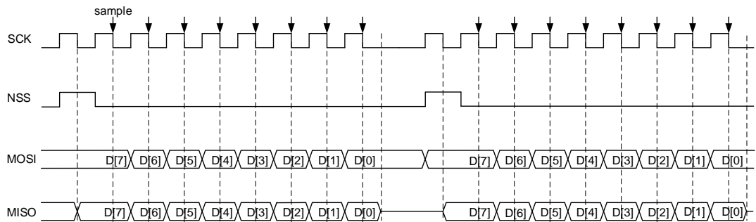
图 27-15. 主机 TI 模式在连续发送时的时序图
