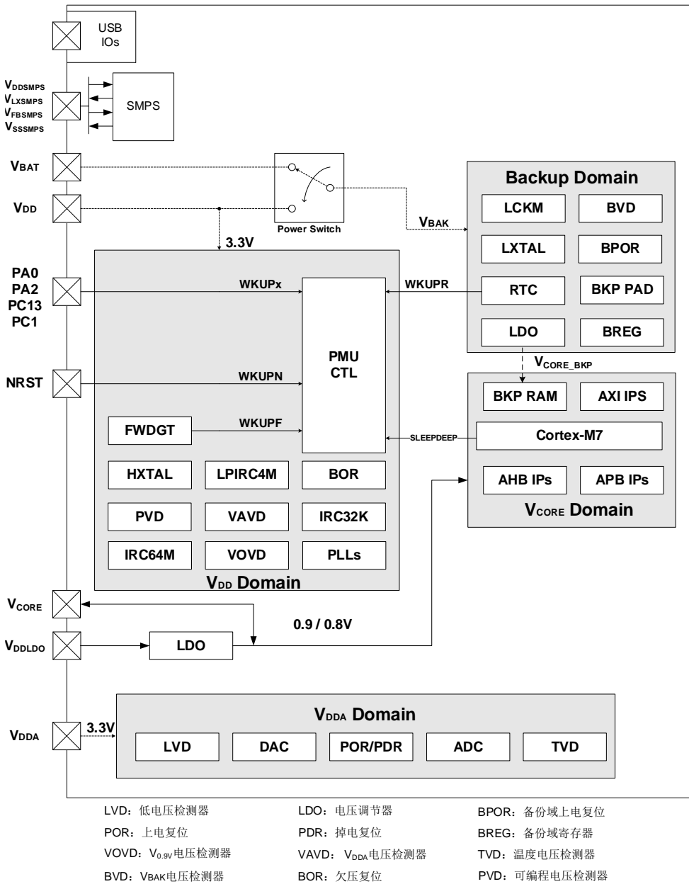
图5-1. 电源域概览
