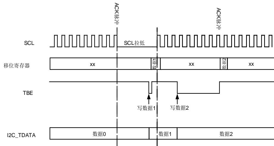
图 26-11. 数据发送
