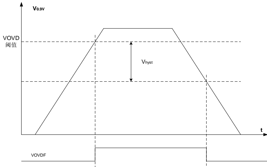
图 5-11. VOVD 波形
