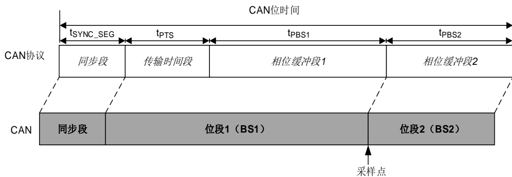
图 42-3. CAN 位时间
