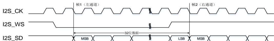
图 27-22. I2S 飞利浦标准时序图 (DTLEN = 10, CHLEN = 1, CKPL = 0)
