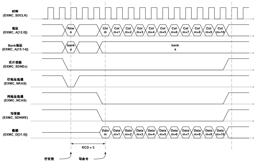
图 38-29. 突发写操作
