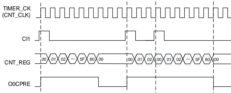
图 24-80. 可延时单脉冲模式（TIMERx_CHxCV=0x00, TIMERx_CAR=0x60）
