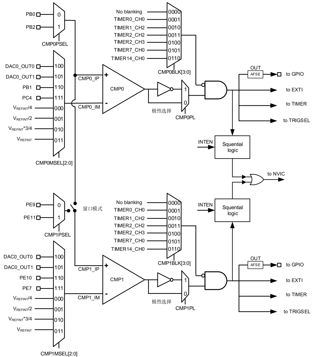
图 44-1. 比较器框图
