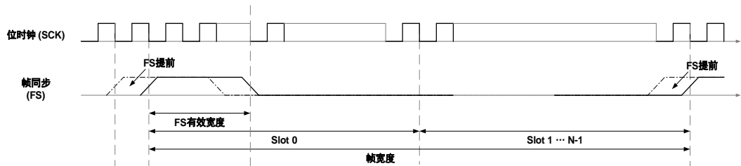
图 34-3. FS 有效宽度
