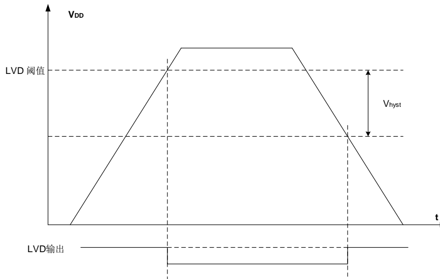
图 5-5. LVD 阈值波形图
