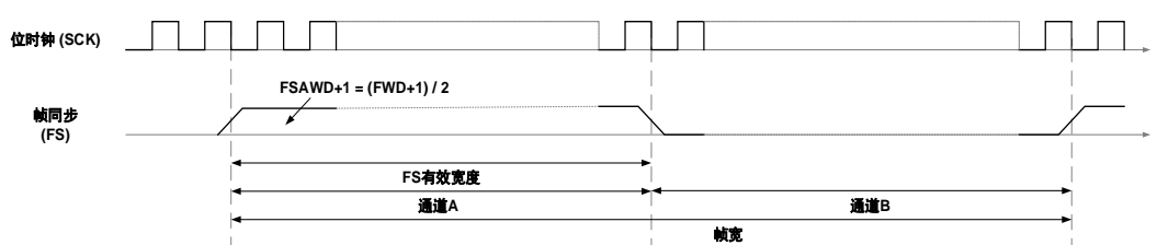
图 34-5. FS 功能
