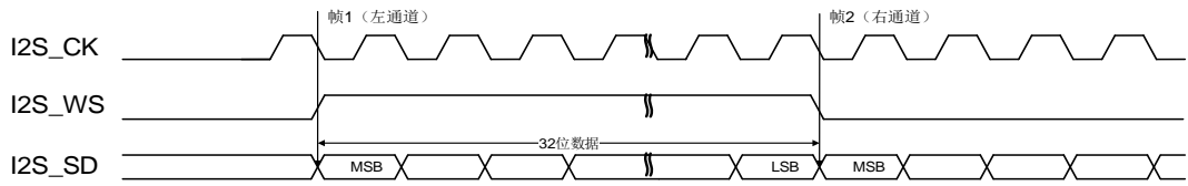
图 27-30. MSB 对齐标准时序图 (DTLEN = 10, CHLEN = 1, CKPL = 0)
