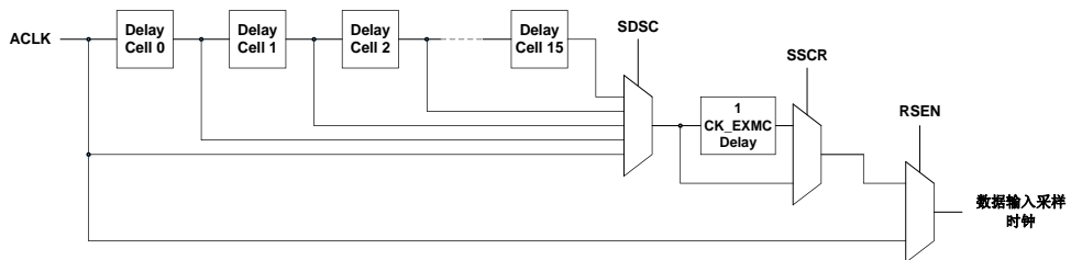
图 38-28. 数据采样时钟延迟模块
