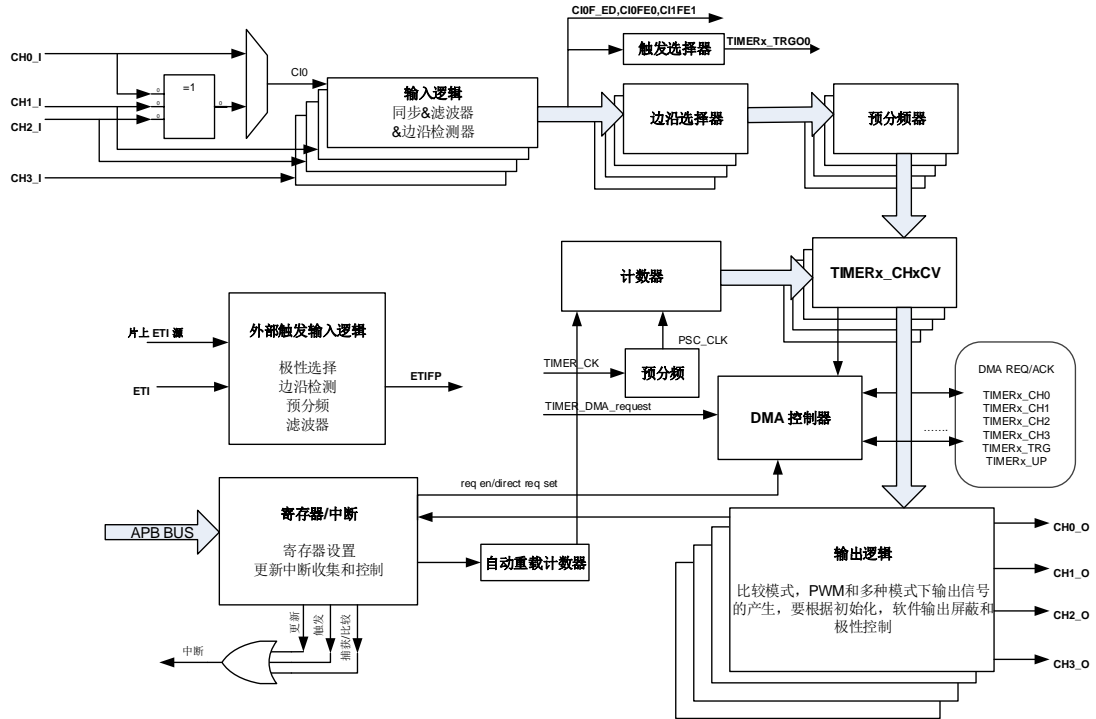
图 24-50. 通用定时器 L0 结构框图
