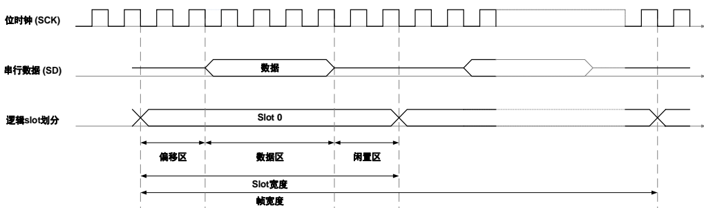
图 34-9. Slot 部分的规定
