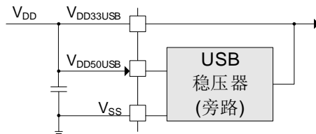
图 5-13. USB 稳压器旁路时连接示意图
