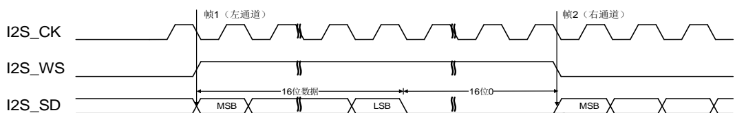
图 27-34. MSB 对齐标准时序图 (DTLEN = 00, CHLEN = 1, CKPL = 0)
