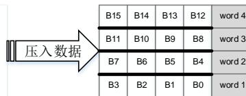
图 16-6. PWIDTH 为‘10’时，数据的打包/解包
