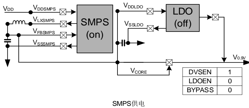
图 5-9. SMPS 供电 V CORE 电源域
