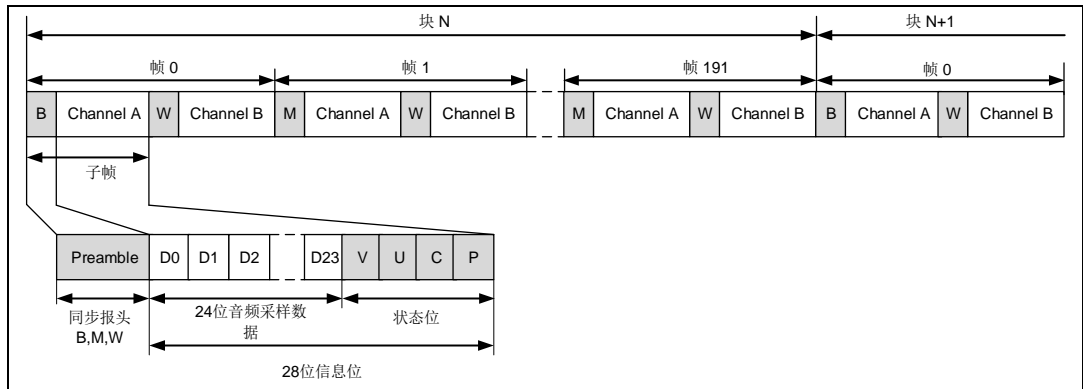
图 34-21. SPDIF 数据格式
