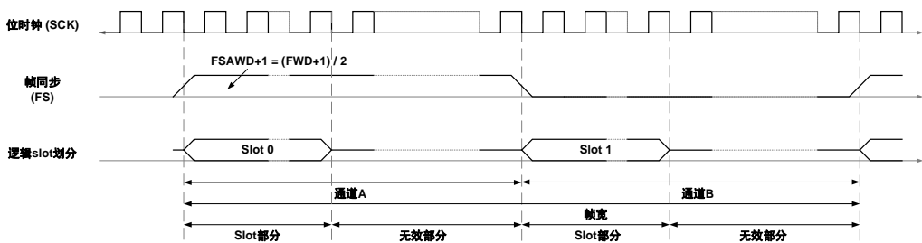
图 34-8. 当 FSFUNC=1 时, slot 分布
