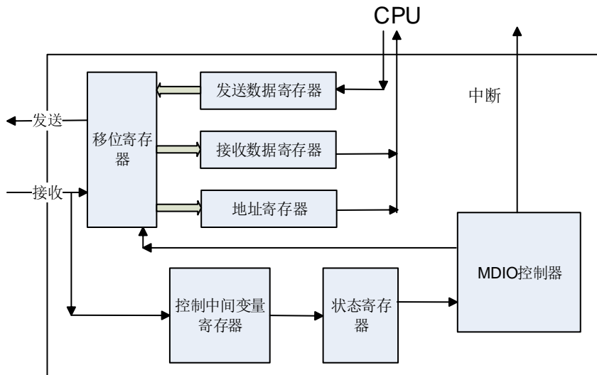
图37-2. MDIO框图
