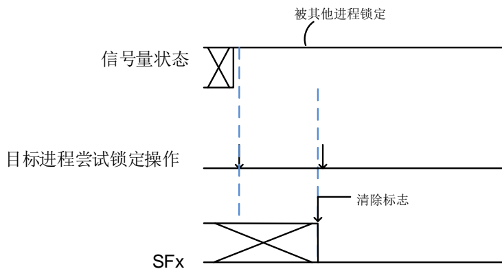
图 48-5. 第二次尝试锁定操作时失败
