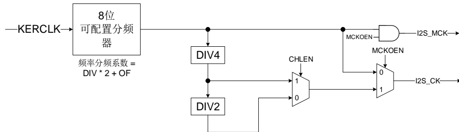
图 27-56. I2S 时钟生成结构框图
