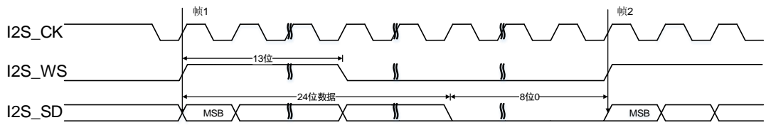
图 27-53. PCM 标准长帧同步模式时序图 (DTLEN = 01, CHLEN = 1, CKPL = 1)
