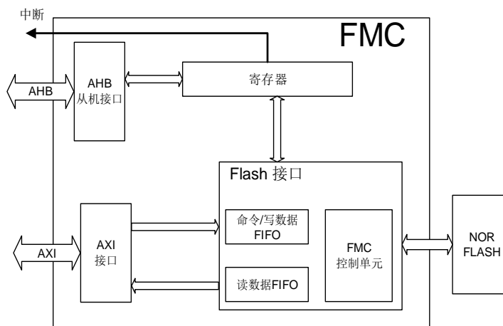
图 3-1. FMC 框图
