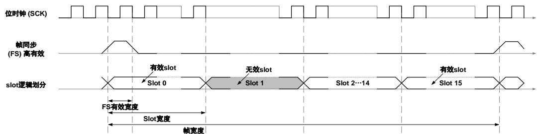
图 34-6. Slot 激活
