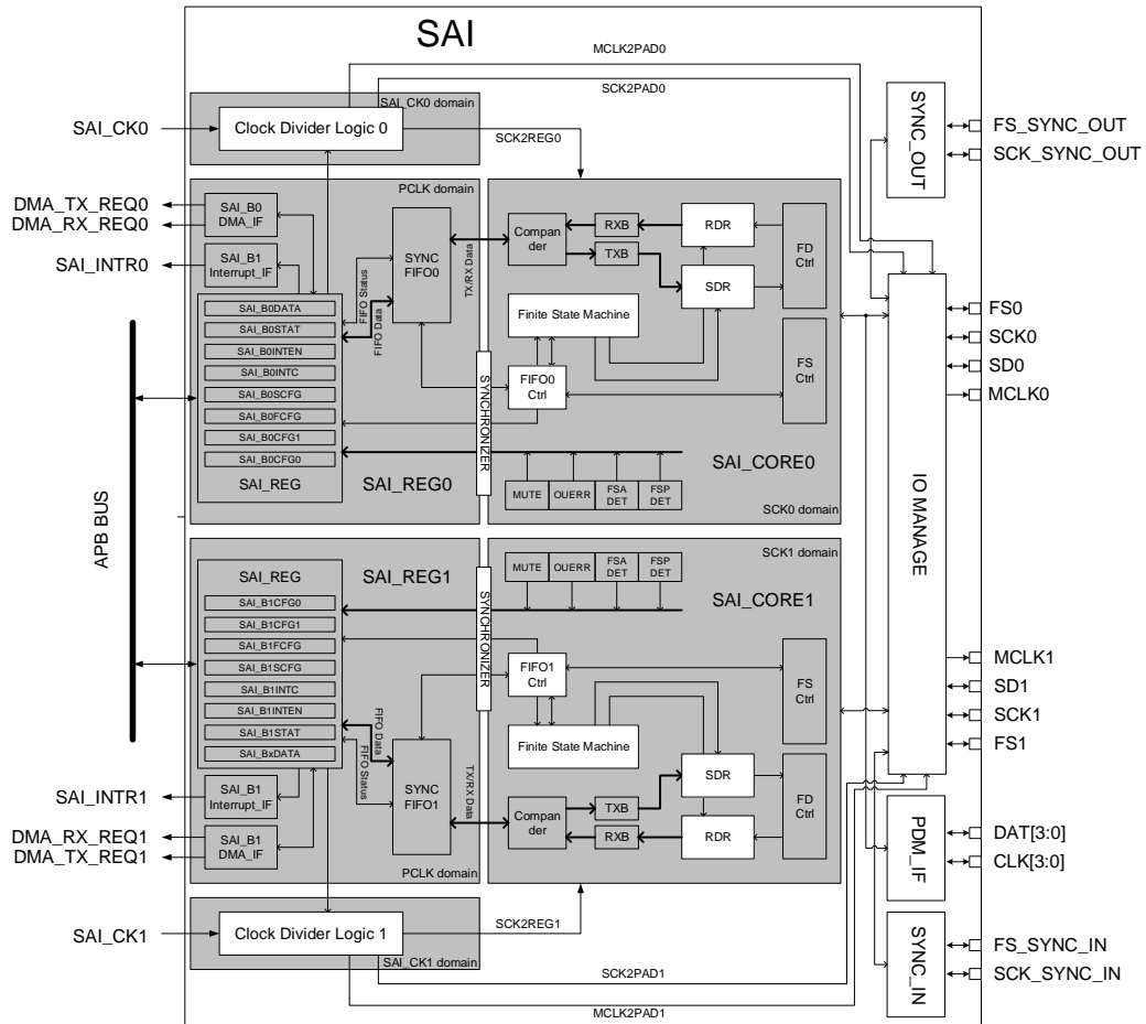
图 34-1. 模块框图
