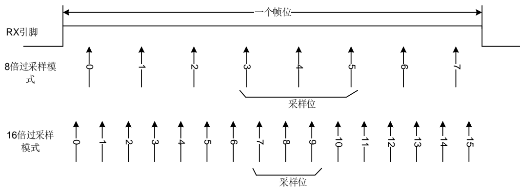
图 25-4. 过采样方式接收一个数据位（OSB = 0）
