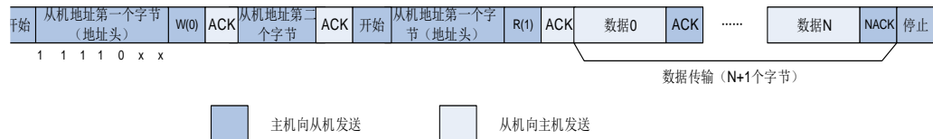
图 26-8. 10 位地址的 I2C 通讯流程（主机接收，HEAD10R = 1）
