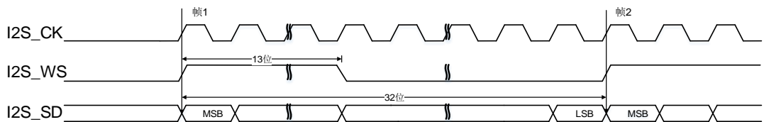
图 27-50. PCM 标准长帧同步模式时序图 (DTLEN = 10, CHLEN = 1, CKPL = 0)
