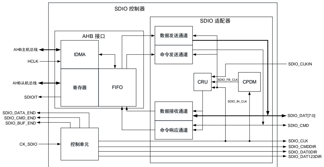
图 36-6. SDIO 框图
