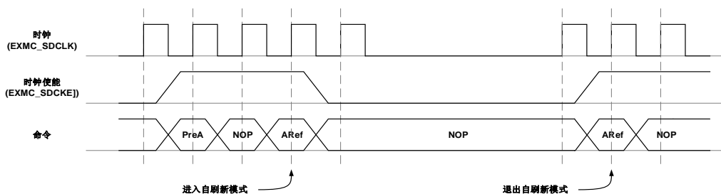
图 38-34. 自刷新模式进入和退出的处理
