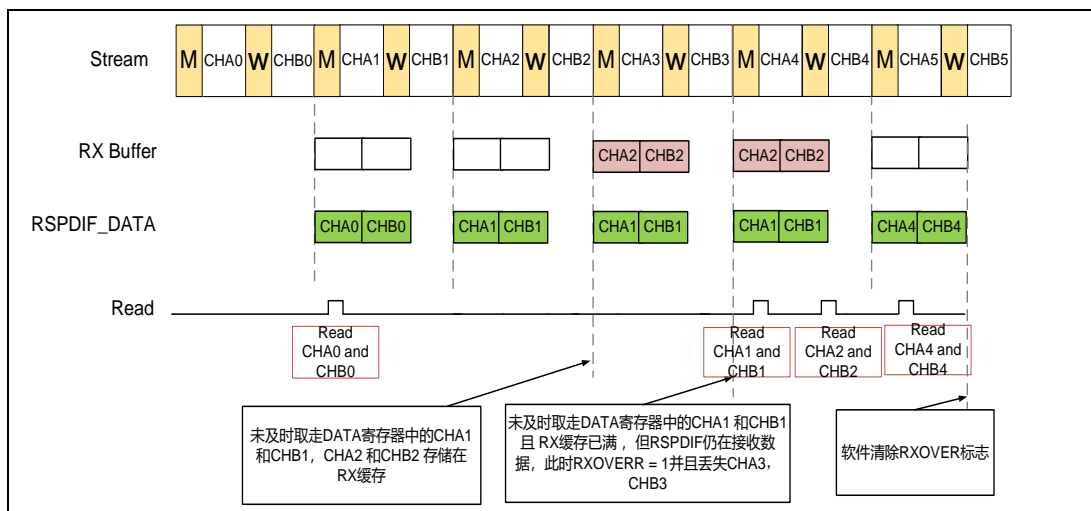
图 33-15. RSPDIF 上溢错误 (RXSTEOMEN = 1 且 RXDF[1:0] = 2'b10)
