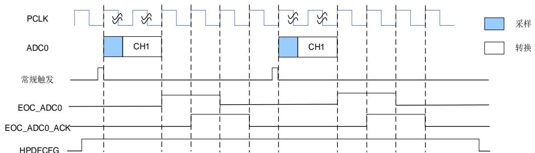
图 20-10. HPDF 与 ADC 模块握手信号示意图
