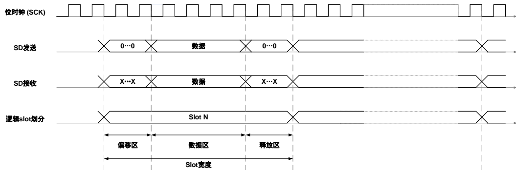
图 34-12. 数据配置
