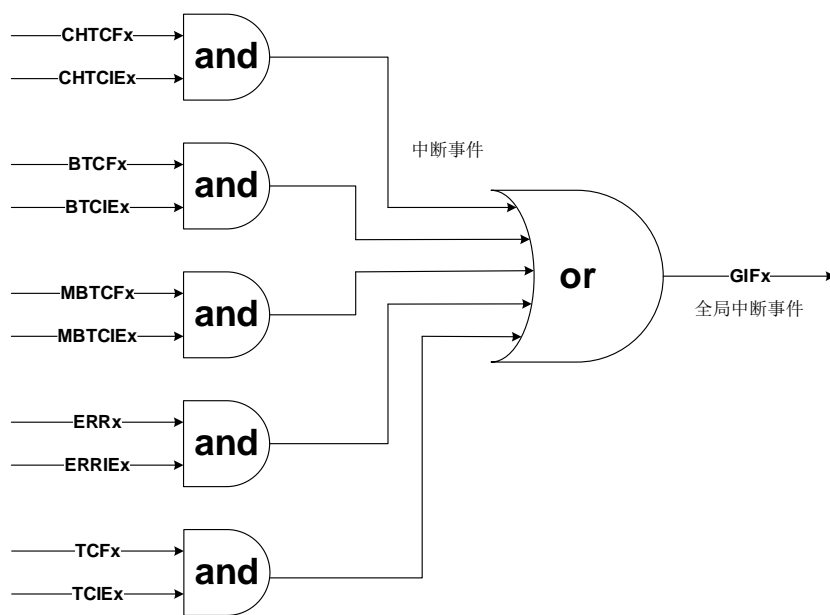
图 17-7. MDMA 中断逻辑图
