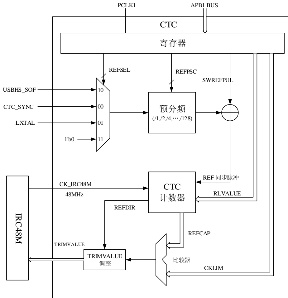
图 7-1. CTC 简介
