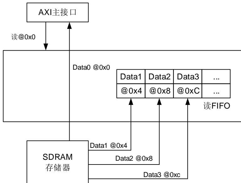
图 38-30. FIFO 未命中时的读访问 (BRSTRD=1, CL=2, SDCLK=2, PIPED=2)
