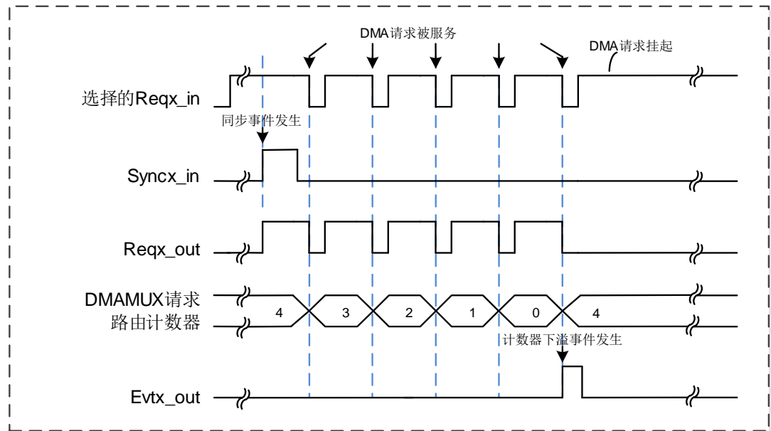
图 18-2. 同步模式
