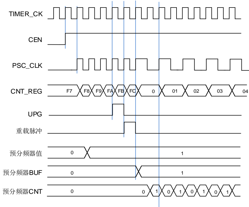
图 24-111. 当预分频器的参数从 1 变到 2 时, 计数器的时序图
