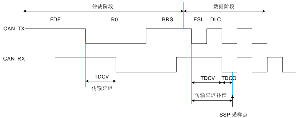
图 42-2. 传输延迟
