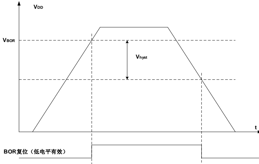
图5-4. BOR波形图
