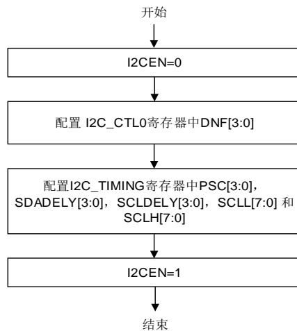
图 26-17. I2C 主机初始化
