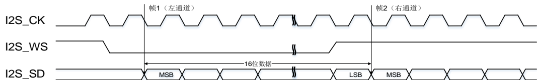
图 27-20. I2S 飞利浦标准时序图 (DTLEN = 00, CHLEN = 0, CKPL = 0)
