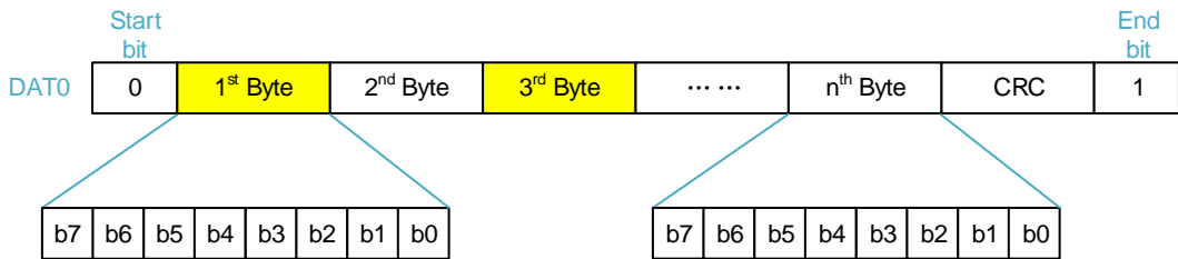
图 36-11. 1 位数据总线宽度
