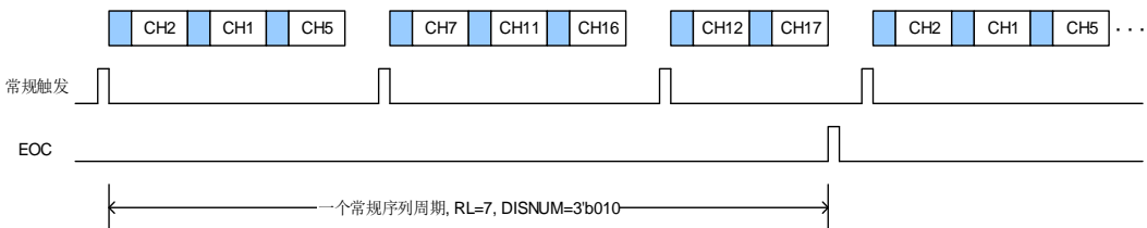
图 20-6. 间断运行模式
