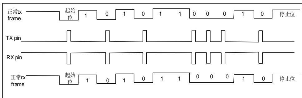
图 25-14. IrDA 数据调制
