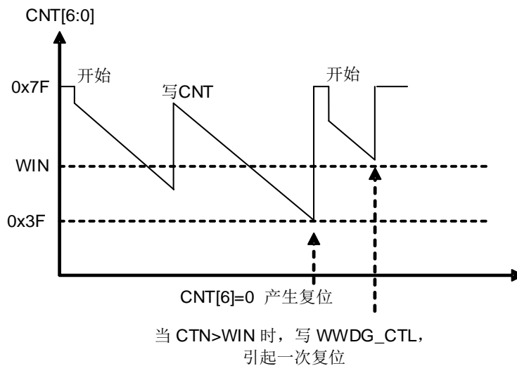
图 22-3. 窗口看门狗定时器时序图
