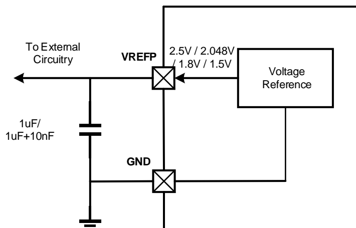
图 39-1. VREF 连接
