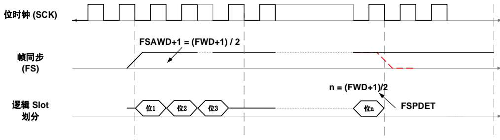
图34-25. 帧同步滞后检测示意图
