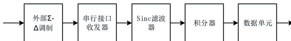
图 45-7. HPDF 模块外部输入数据处理流程
