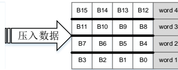
图 16-5. PWIDTH 为‘01’时，数据的打包/解包
