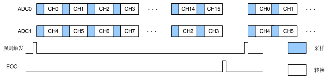
图 20-16. 基于 16 个通道的常规并行模式
