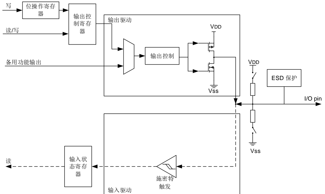
图 10-3. 输出配置
