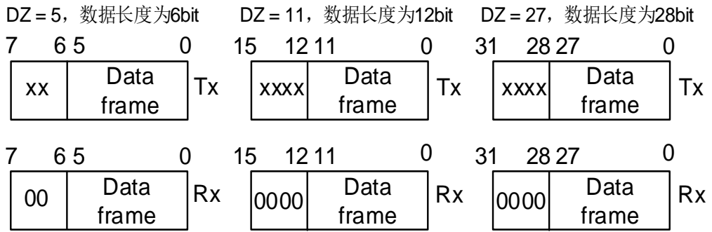
图 27-4. SPI 数据帧右对齐示意图
