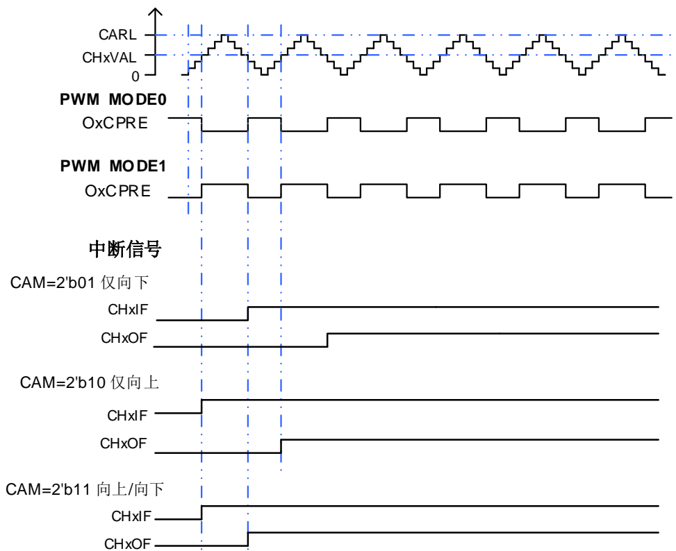
图 24-62. CAPWM 时序图
