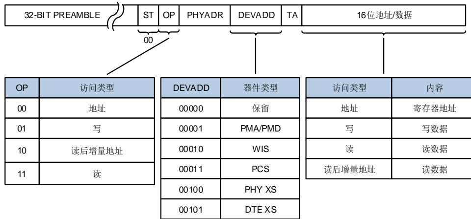
图37-3. MDIO帧格式
