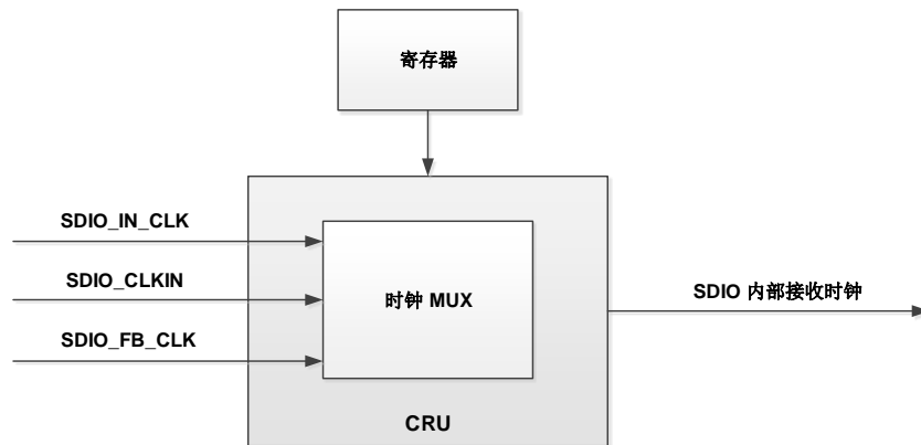
图 36-7. CRU 单元
