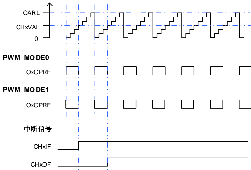
图 24-93. PWM 时序图
