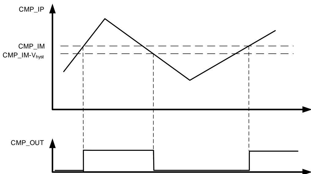
图 44-2. 比较器迟滞
