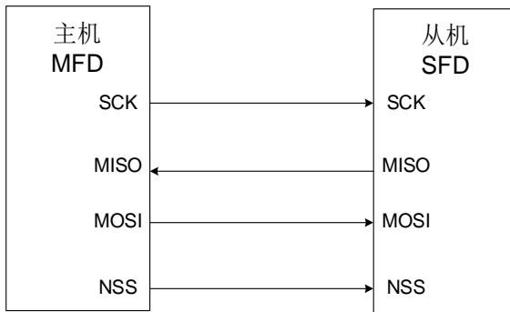
图 27-10. 典型的全双工模式连接
