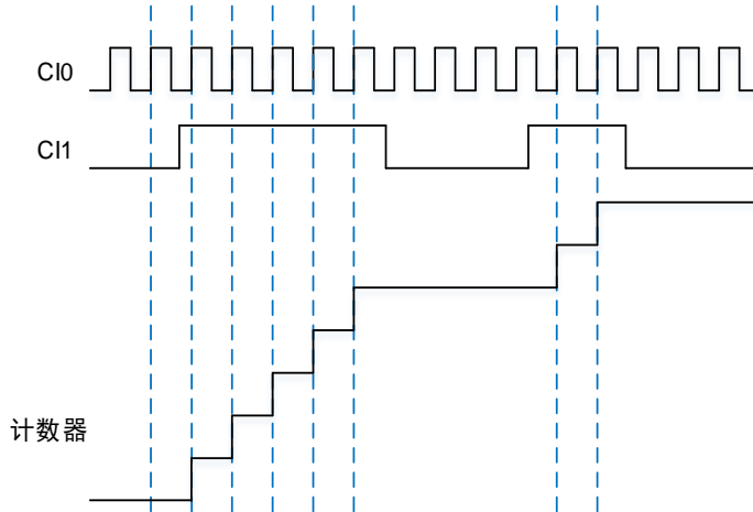
图 24-74. 非正交译码器模式 0 计数器运行实例 (CH1P=0)
