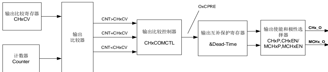
图 24-118. 输出比较逻辑 (当 MCHxMSEL = 2'11 时, x=0)
