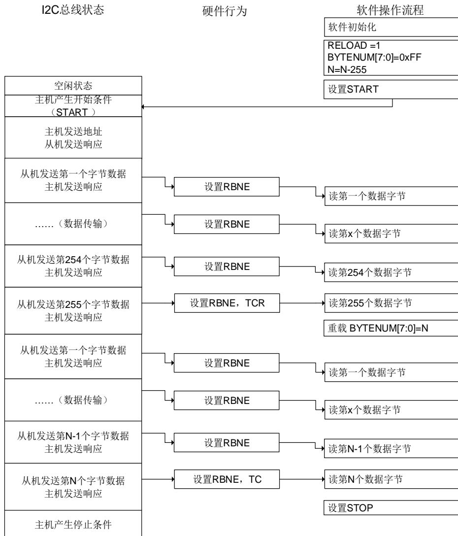
图 26-21. I2C 主机接收编程模型 (N>255)
