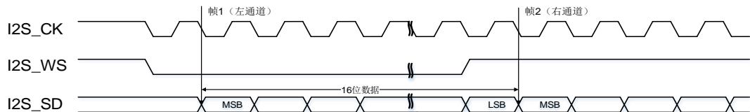
图 27-21. I2S 飞利浦标准时序图 (DTLEN = 00, CHLEN = 0, CKPL = 1)
