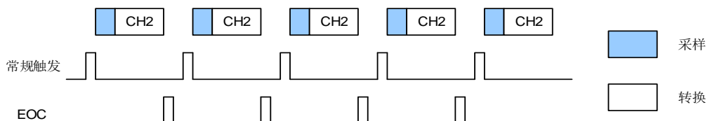
图 20-2. 单次运行模式
