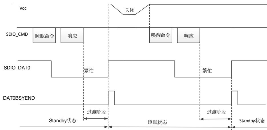
图 36-18. CMD5 时序
