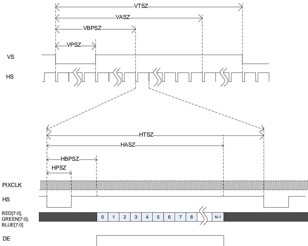
图 32-2. 显示时序图
