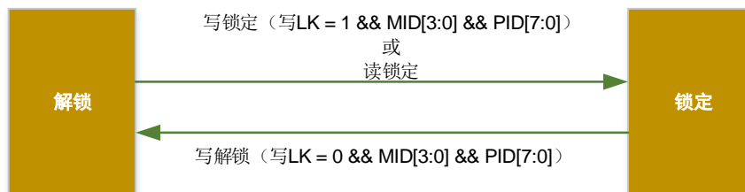
图 48-2. HWSEM 状态机
