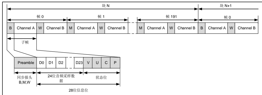
图 33-2. S/PDIF 块及子帧格式
