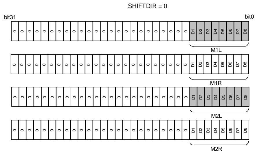
图 34-18. 双麦克风, 不同 slot 宽度下, BxDATA 寄存器数据格式
