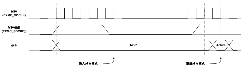
图 38-35. 掉电模式进入和退出的处理
