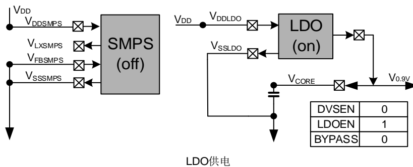
图 5-8. LDO 供电 V CORE 电源域
