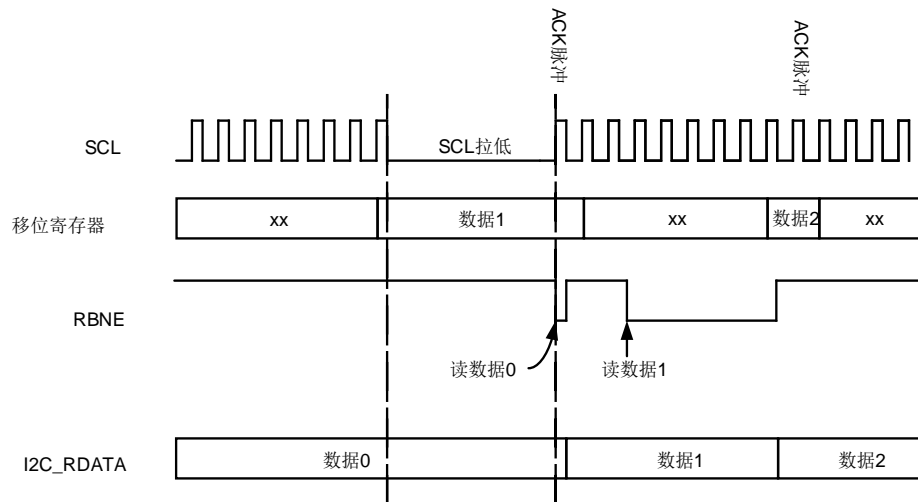
图 26-12. 数据接收
