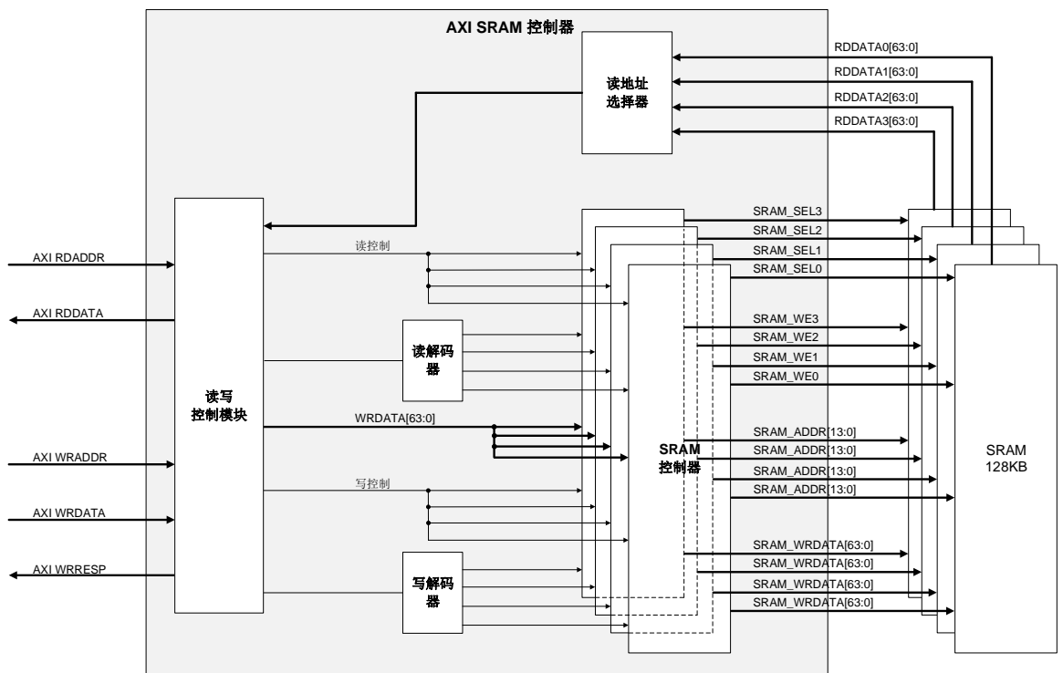
图 1-6. AXI SRAM 框图
