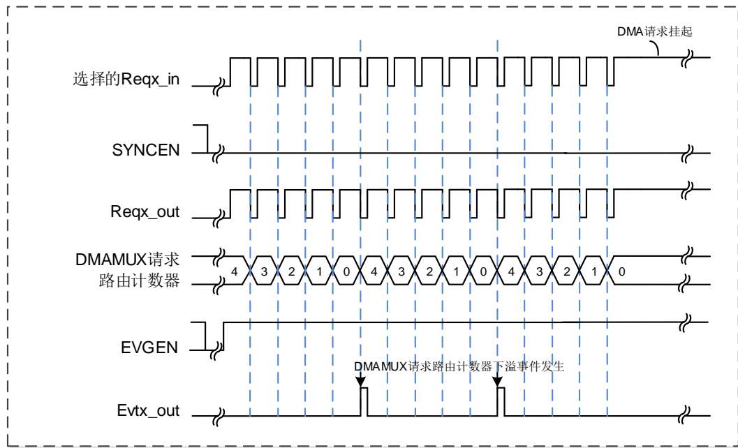
图 18-3. 通道事件输出
