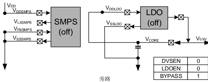
图 5-10.旁路
