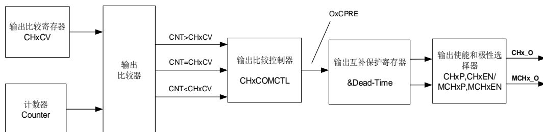
图 24-90. 输出比较逻辑（当 MCHxMSEL = 2'11 时, x=0）
