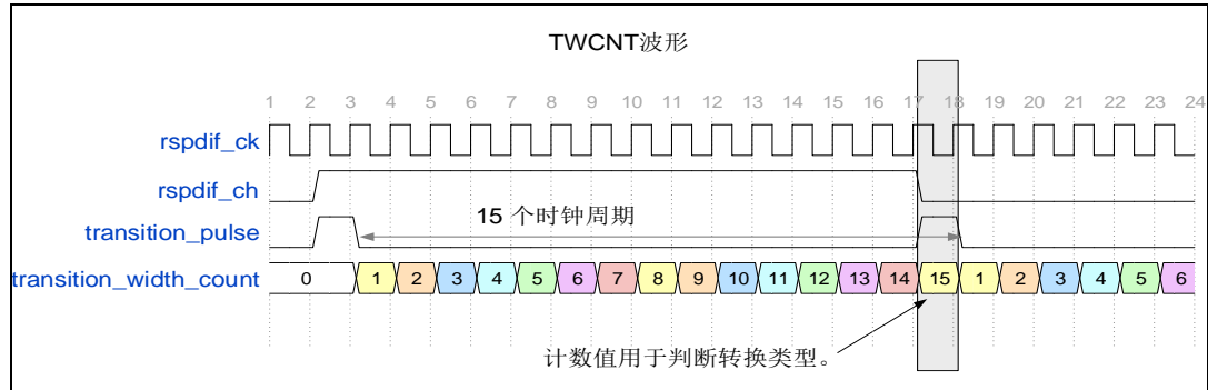
图 33-6. TWCNT 波形
