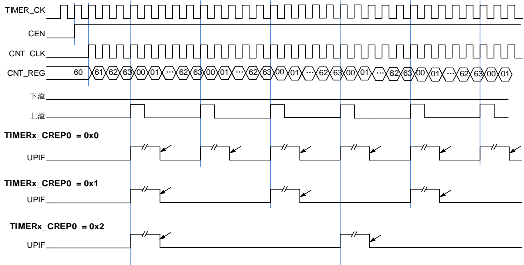
图 24-114. 在向上计数模式下计数器重复时序图
