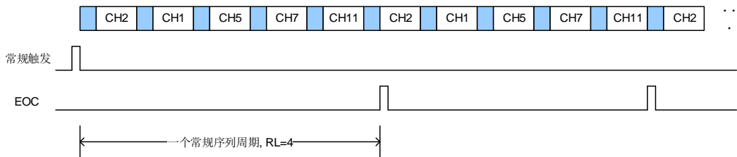
图 20-5. 扫描运行模式，连续运行模式使能
