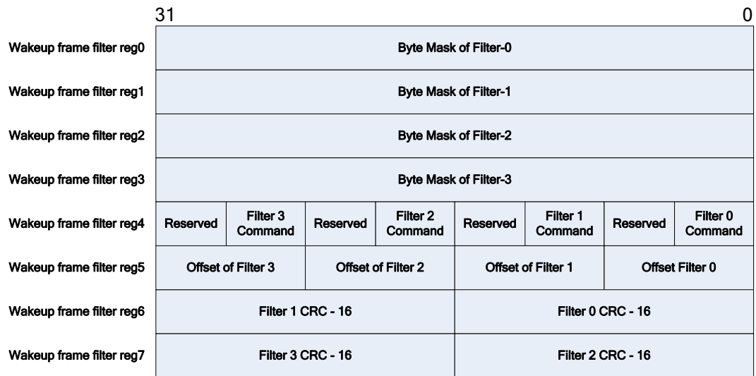
图 43-15. 远程唤醒帧过滤器寄存器
