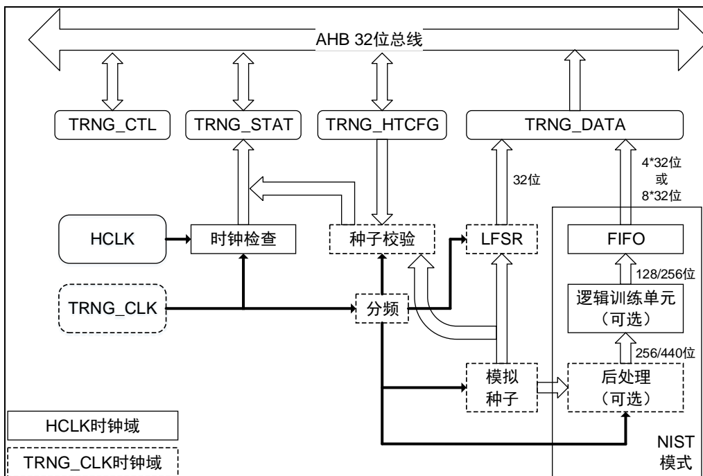
图 12-1. TRNG 模块框图
