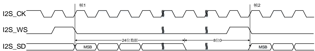
图 27-45. PCM 标准短帧同步模式时序图 (DTLEN = 01, CHLEN = 1, CKPL = 1)
