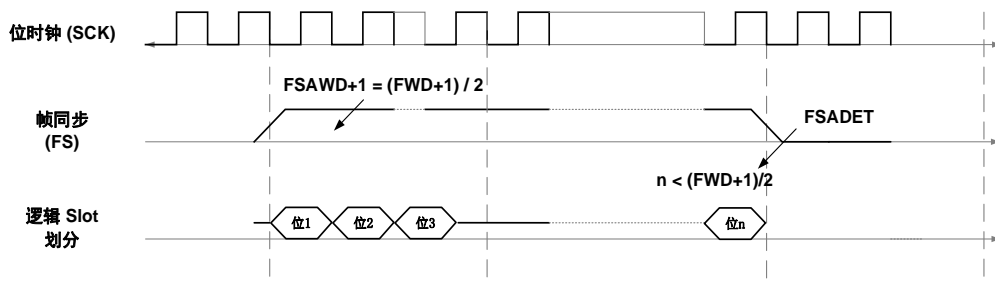
图34-24. 帧同步提前检测示意图
