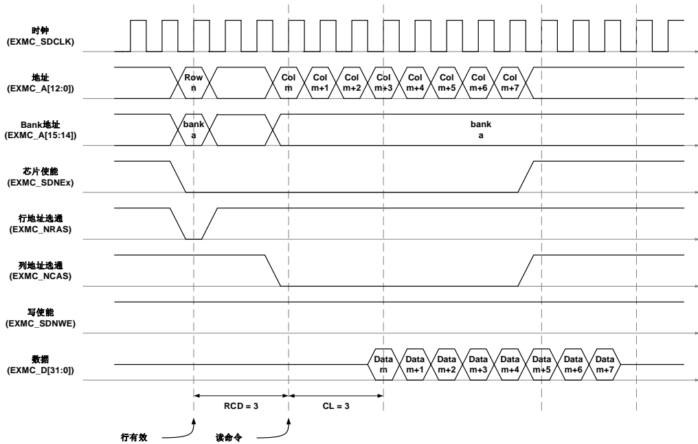
图 38-27. 突发读操作
