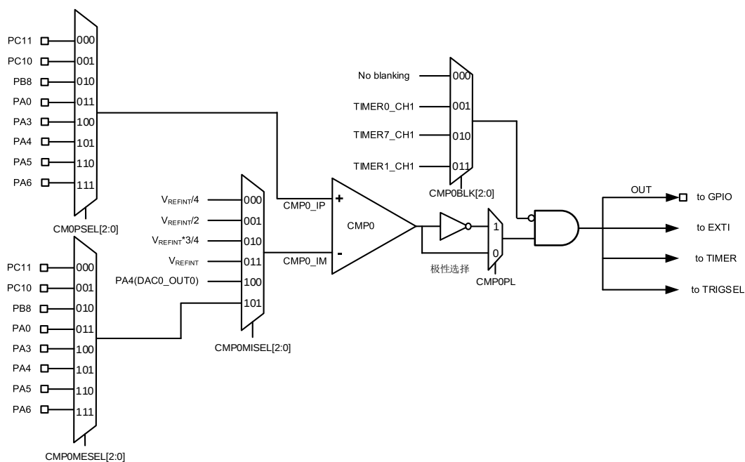
图 22-1. 比较器框图
