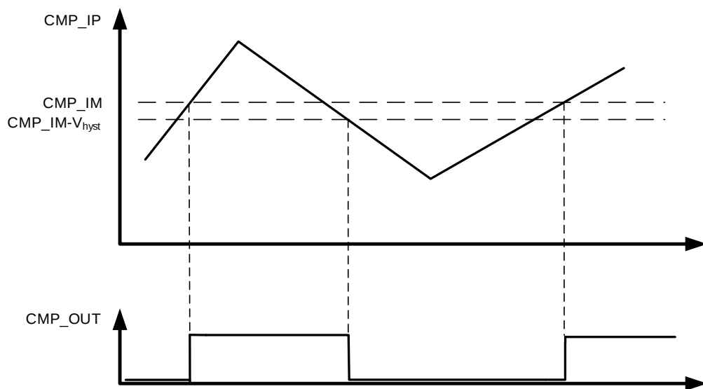
图 22-2. 比较器迟滞
