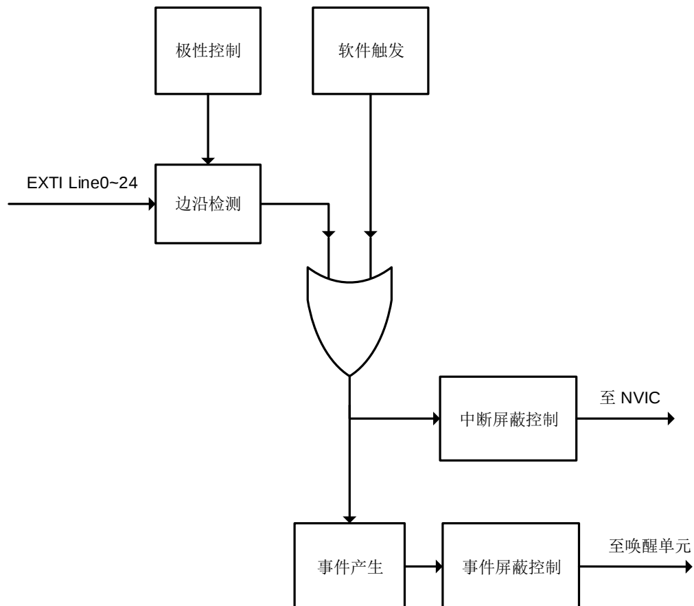
图 6-1. EXTI 框图
