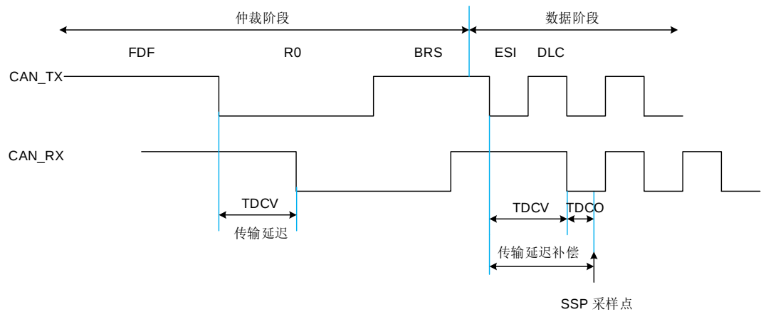
图 23-2. 传输延迟
