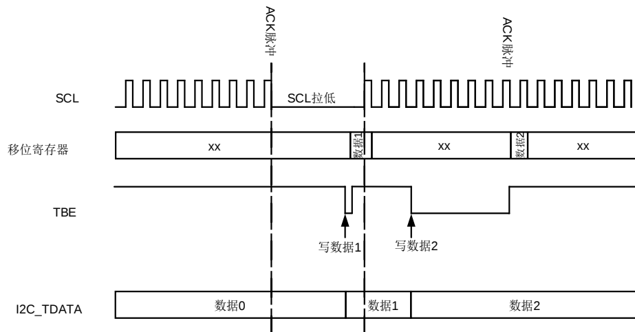
图 20-11. 数据发送
