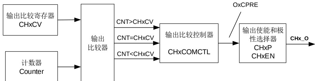
图 18-51. 输出比较原理 (x=0,1,2,3)
