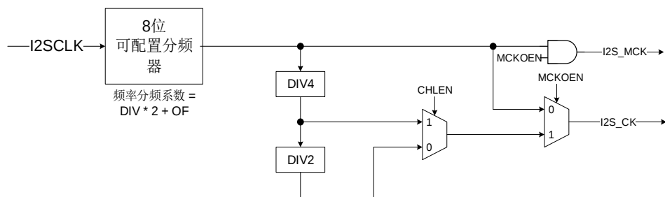
图 21-51. I2S 时钟生成结构框图
