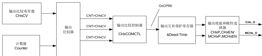
图 18-16. 输出比较原理（当 MCHxMSEL = 2'11 时互补输出, x=0,1,2,3 ）
