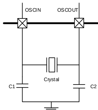
图5-3. HXTAL时钟源
