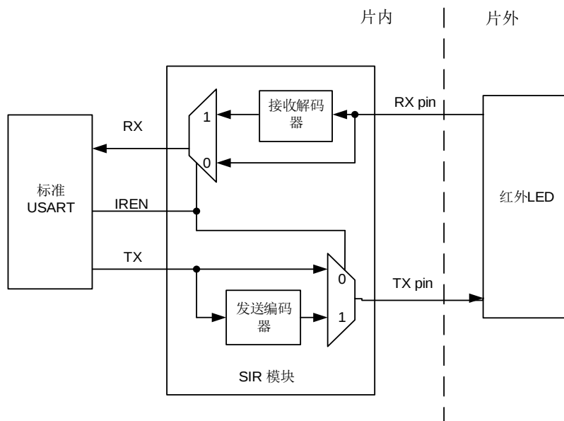
图 19-13. IrDA SIR ENDEC 模块
