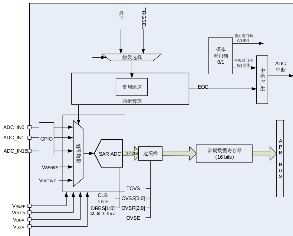
图 14-1. ADC 模块框图
