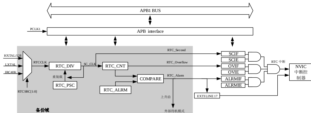
图 17-1. RTC 框图
