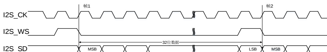
图 21-38. PCM 标准短帧同步模式时序图 (DTLEN=10, CHLEN=1, CKPL=1)
