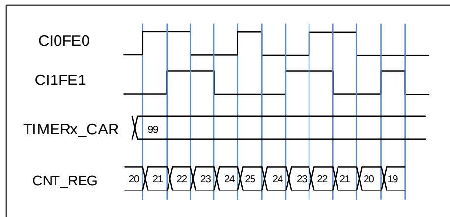
图 18-55. 在正交译码模式 2 且 CI0FE0 极性不反相时计数器行为
