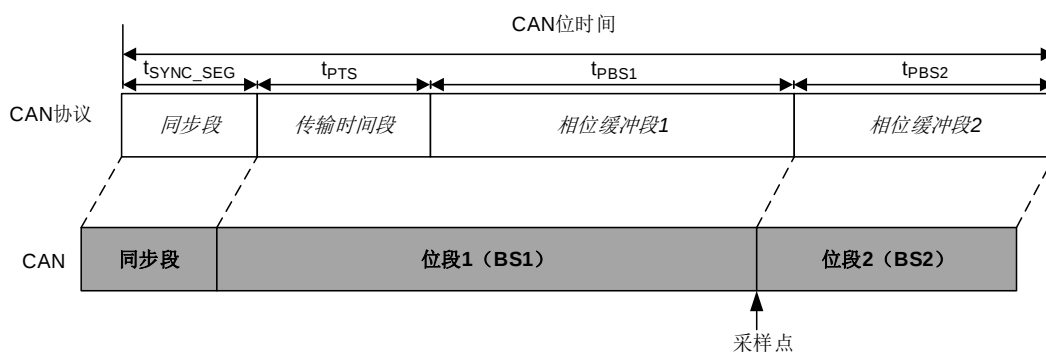
图 23-3. CAN 位时间
