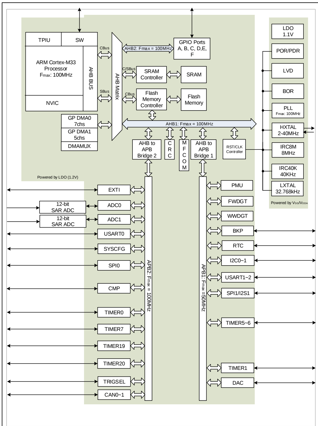
图 1-2. GD32A50x 系列器件的系统架构示意图
