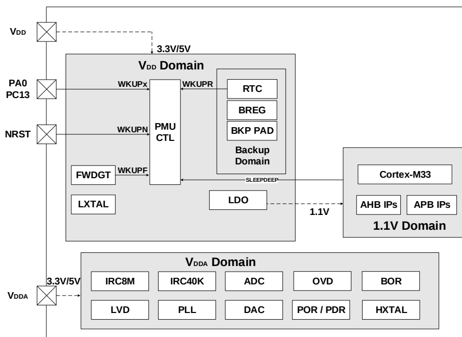
图3-1. 电源域概览
