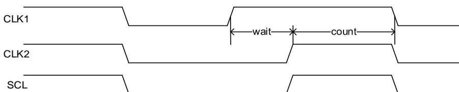
图 17-20. 时钟同步
