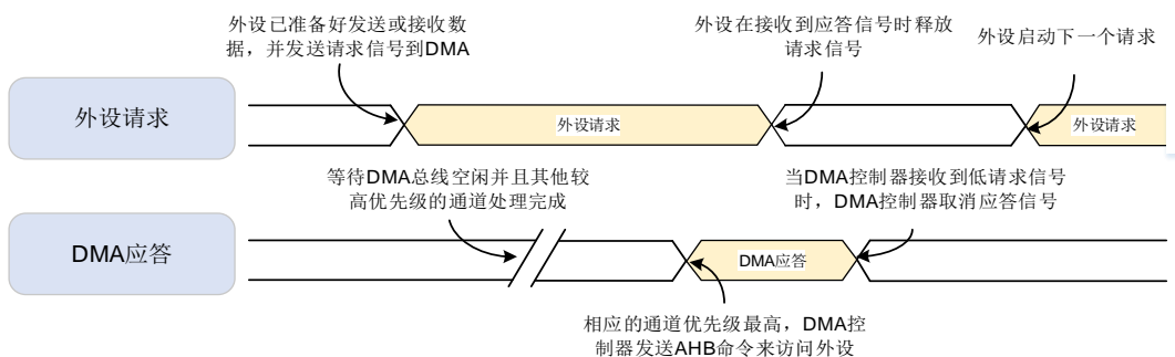
图 10-2. 握手机制
