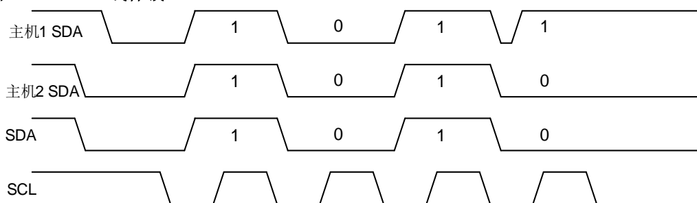
图 17-21. SDA 线仲裁
