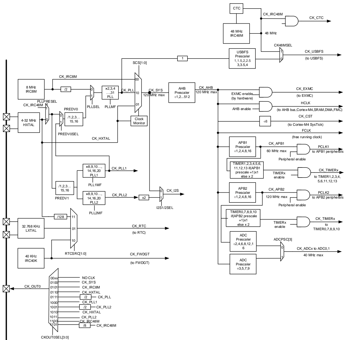
图5-2. 时钟树
