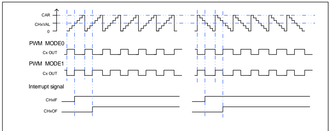
图 16-14. EAPWM 时序图
