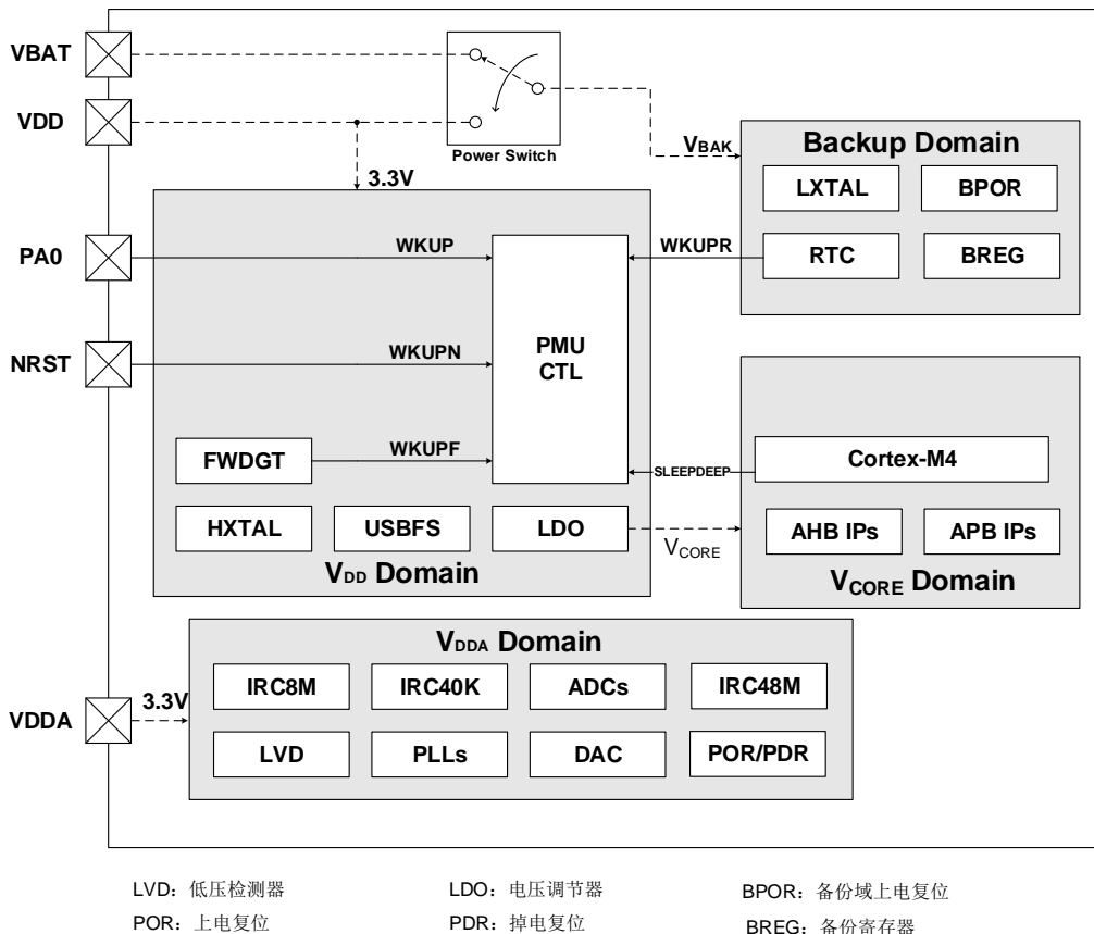
图3-1. 电源域概览
