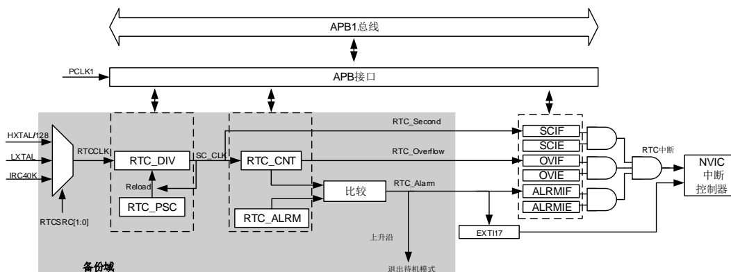
图 15-1. RTC 框图
