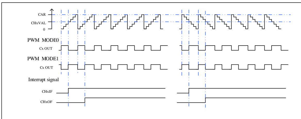
图 16-51. EAPWM 时序图
