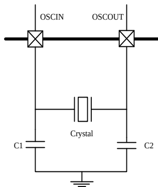
图5-3. HXTAL时钟源
