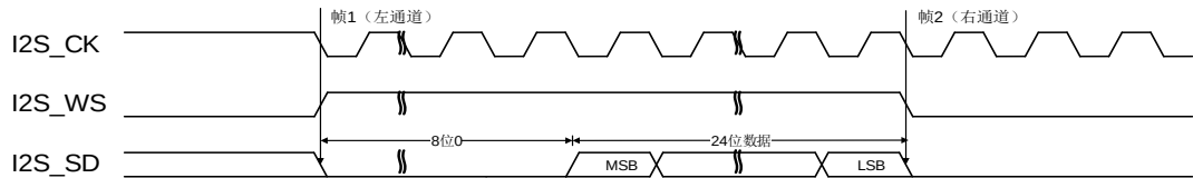
图 19-32. LSB 对齐标准时序图(DTLEN=01, CHLEN=1, CKPL=1)
