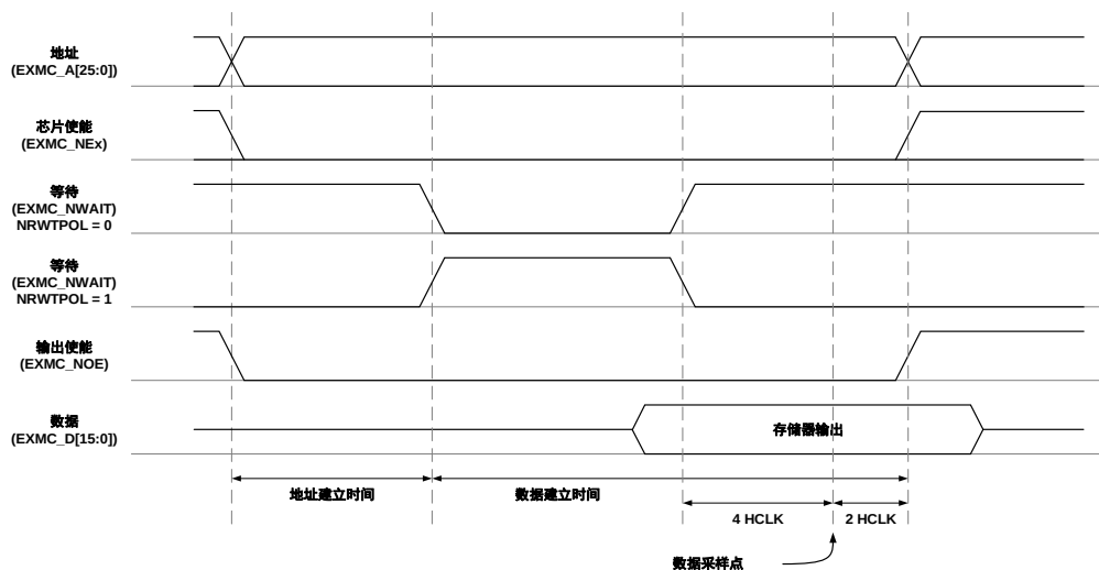
图 21-19. 异步等待有效时的读时序
