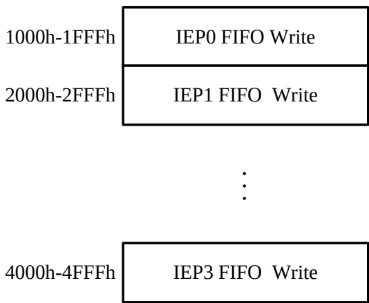
图 23-8. 设备模式 FIFO 访问寄存器映射表
