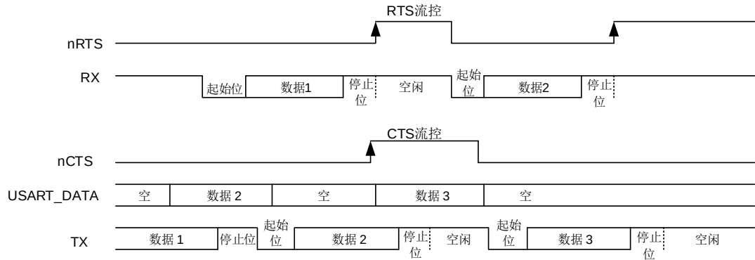
图 17-8. 硬件流控制
