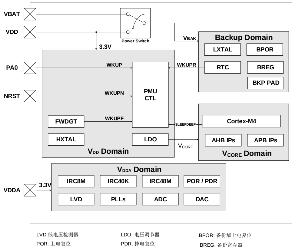
图3-1. 电源域概览
