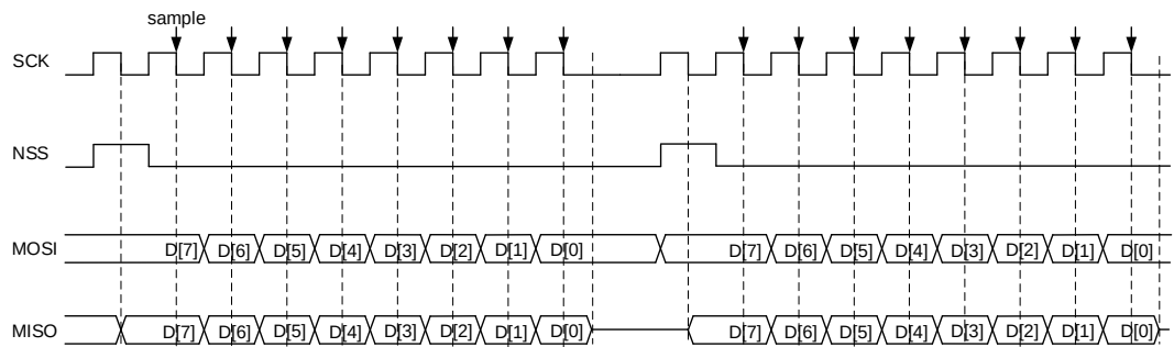
图 19-8. 主机 TI 模式在不连续发送时的时序图
