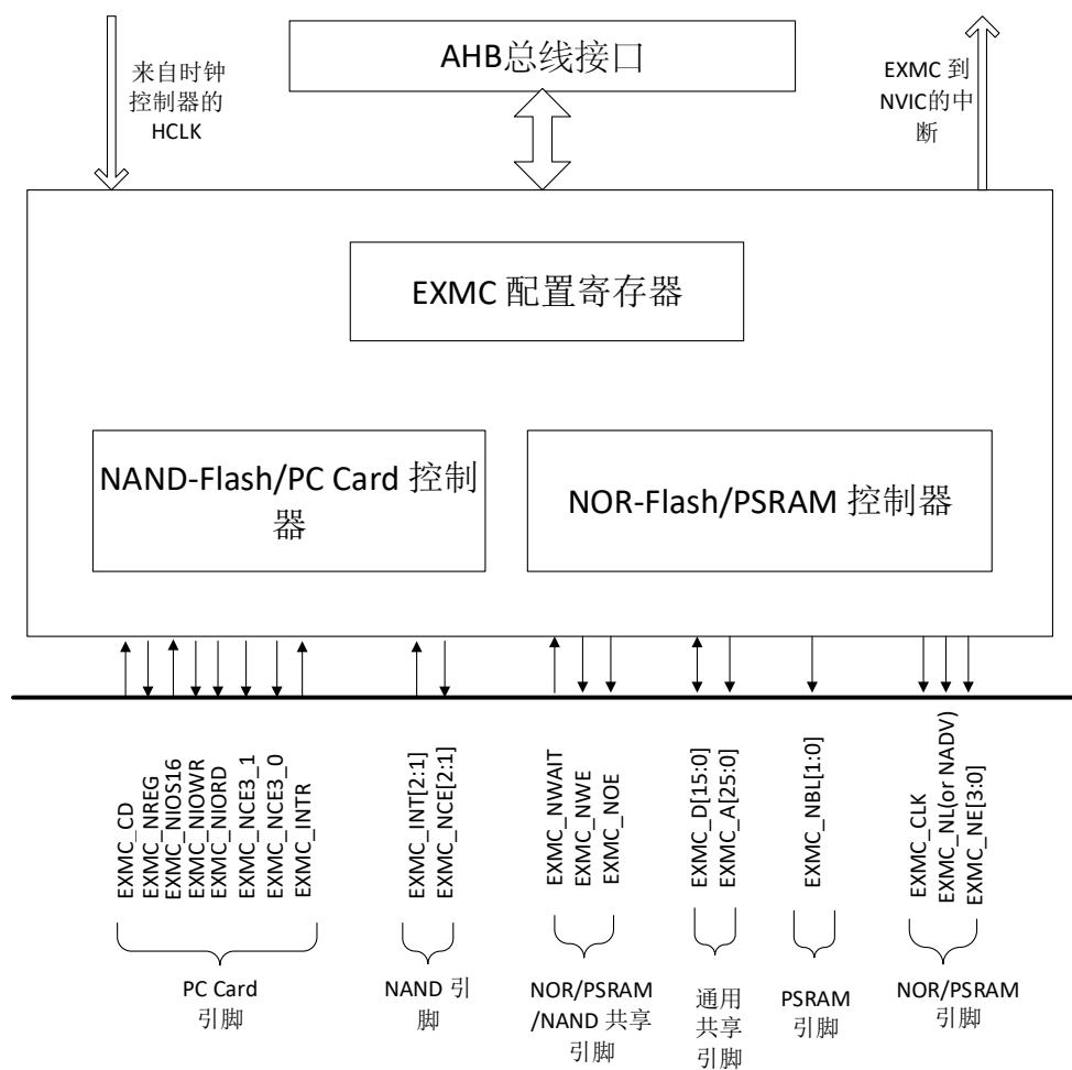
图 21-1. 系统架构
