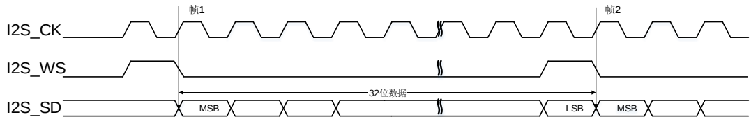
图 19-38. PCM 标准短帧同步模式时序图(DTLEN=10, CHLEN=1, CKPL=1)
