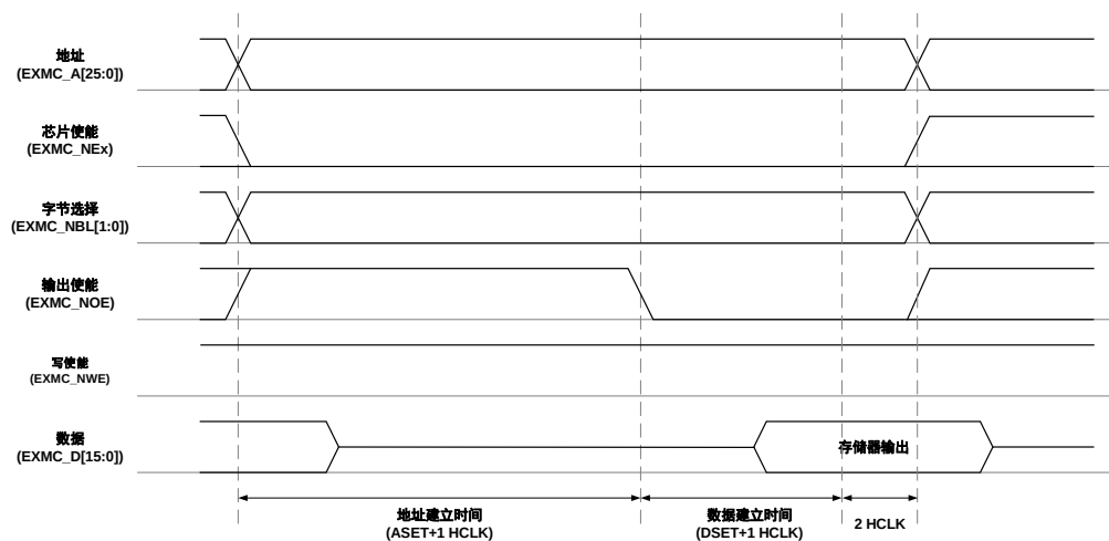
图 21-8. 模式 A 读时序
