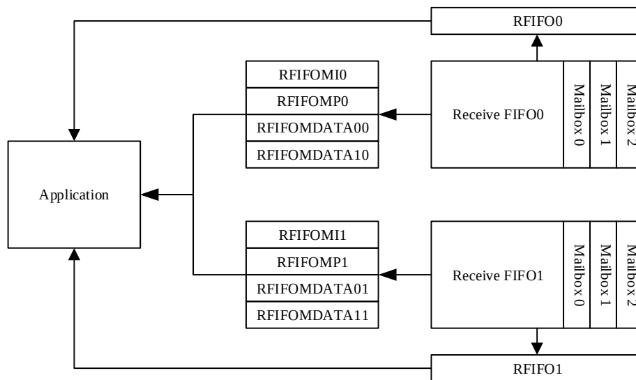
图 22-4. 接收寄存器
