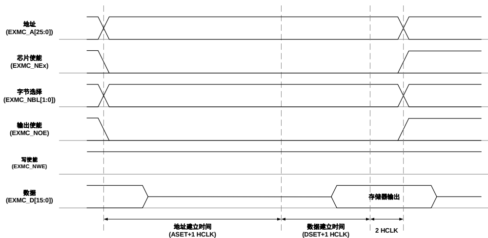
图 21-7. 模式 1 写时序
