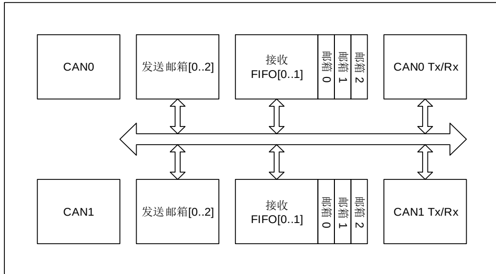
图 22-1. CAN 模块结构框图
