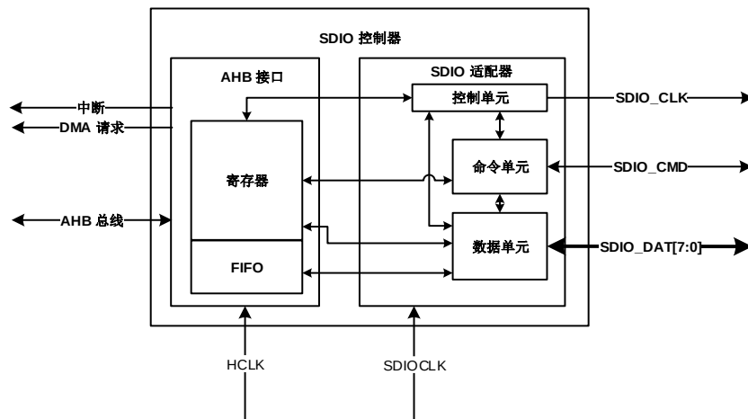
图 20-6. SDIO 框图
