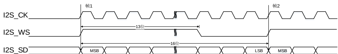
图 19-44. PCM 标准长帧同步模式时序图(DTLEN=00, CHLEN=0, CKPL=1)
