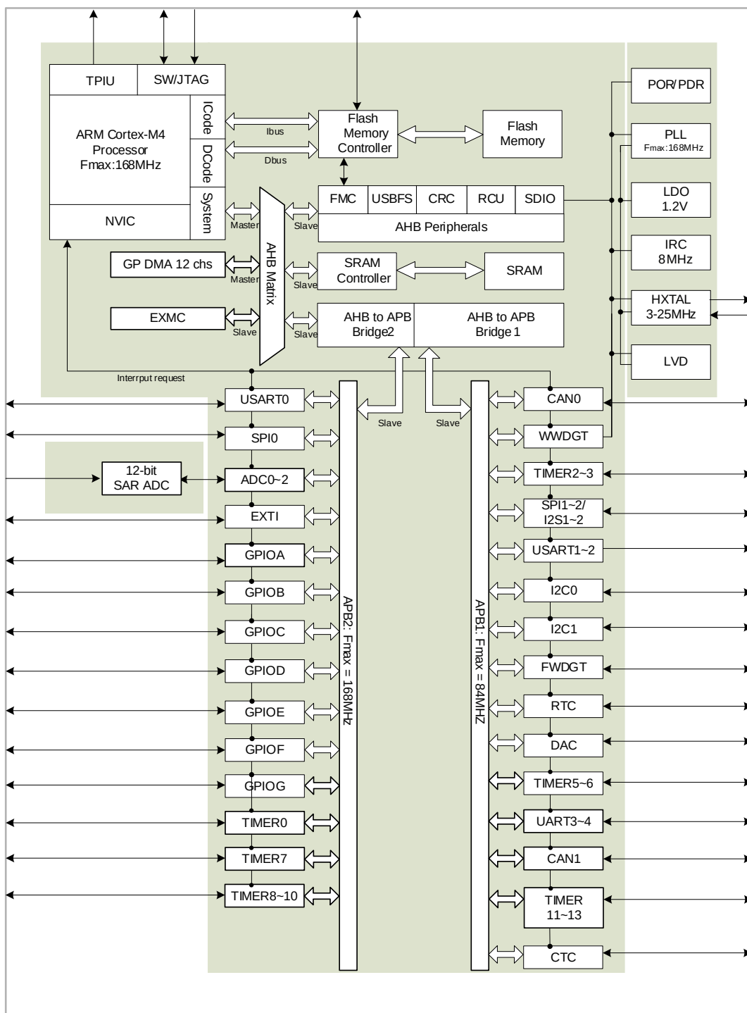
图 1-2. GD32F403xx 系列的系统架构
