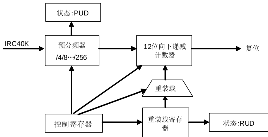
图 14-1. 独立看门狗定时器框图
