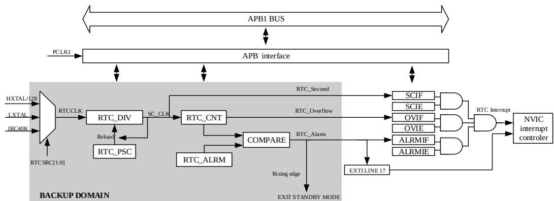
图 15-1. RTC 框图
