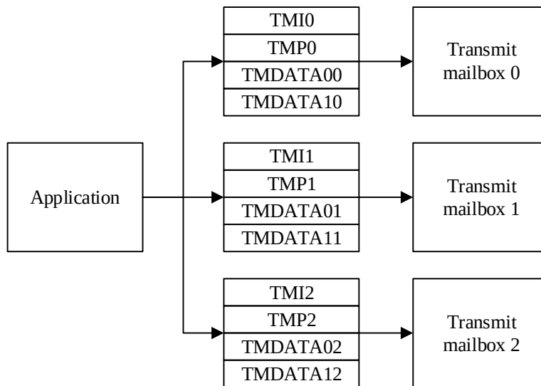
图 22-2. 发送寄存器
