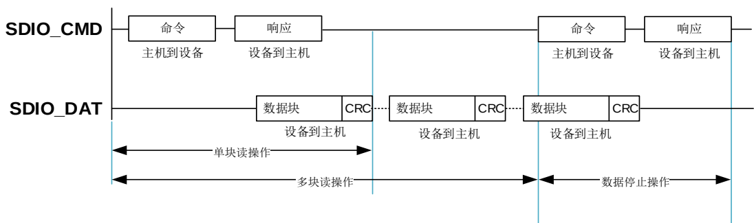
图 20-2. SDIO 多块读操作
