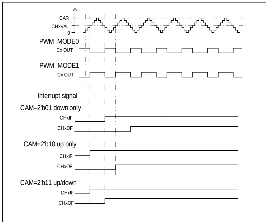
图 16-52. CAPWM 时序图
