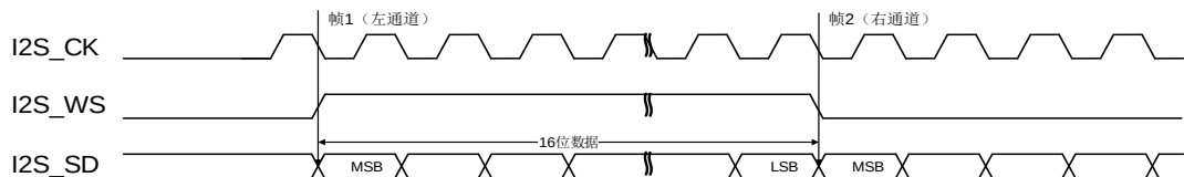
图 19-24. MSB 对齐标准时序图(DTLEN=00, CHLEN=0, CKPL=1)
