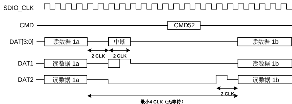
图 20-13. 使用 SDIO_DAT[2]信号线的读等待操作
