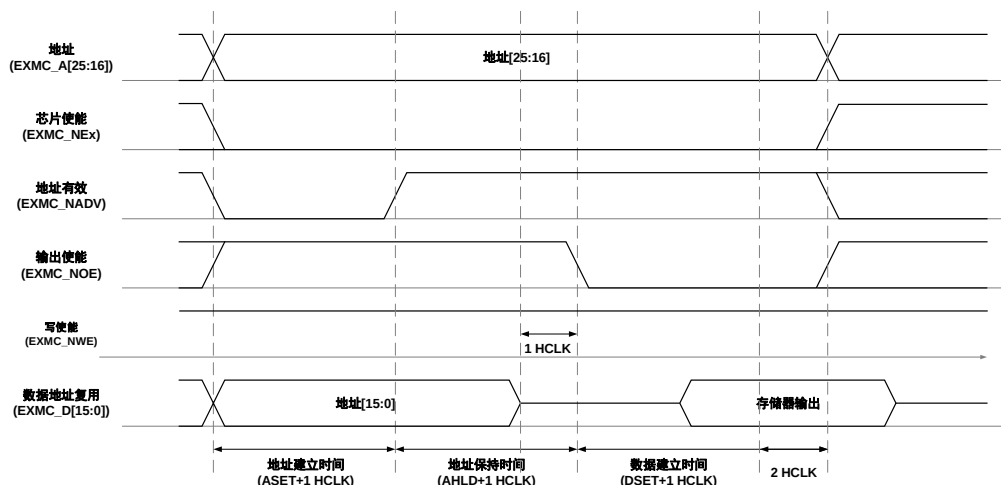
图 21-17. 复用模式读时序
