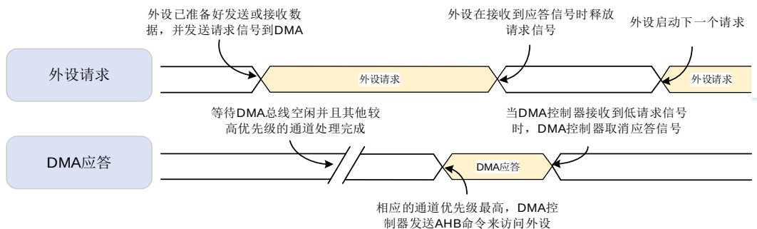
图 10-2. 握手机制
