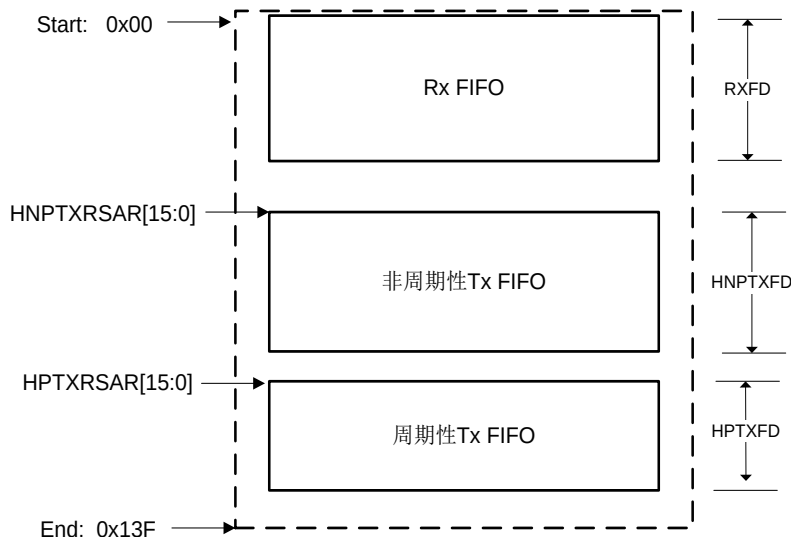
图 22-5. 主机模式 FIFO 空间
