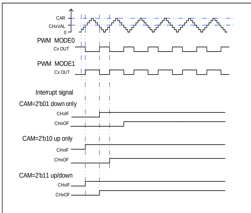
图 16-52. CAPWM 时序图
