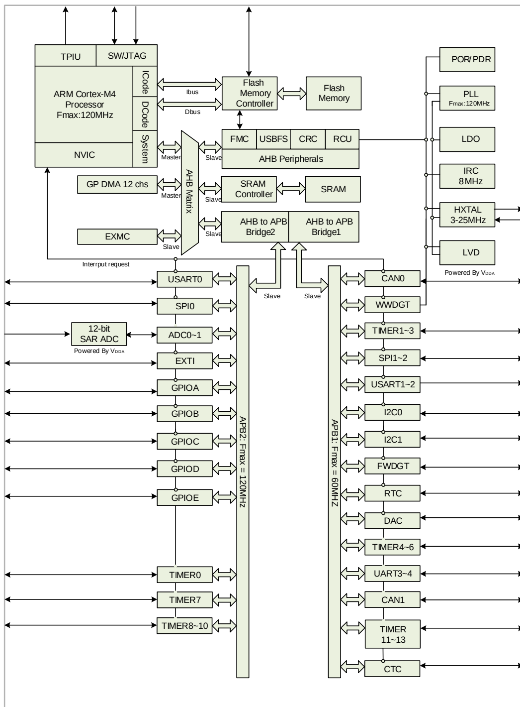
图 1-2. GD32C10x 器件的系统架构示意图
