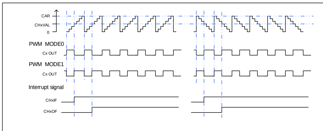
图 16-14. EAPWM 时序图
