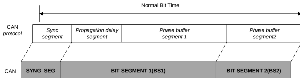
图 21-11. 位时序
