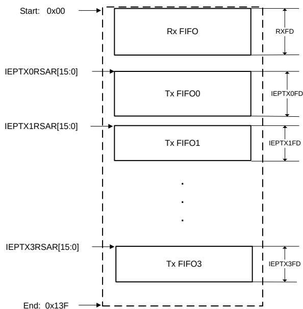
图 22-7. 设备模式 FIFO 空间
