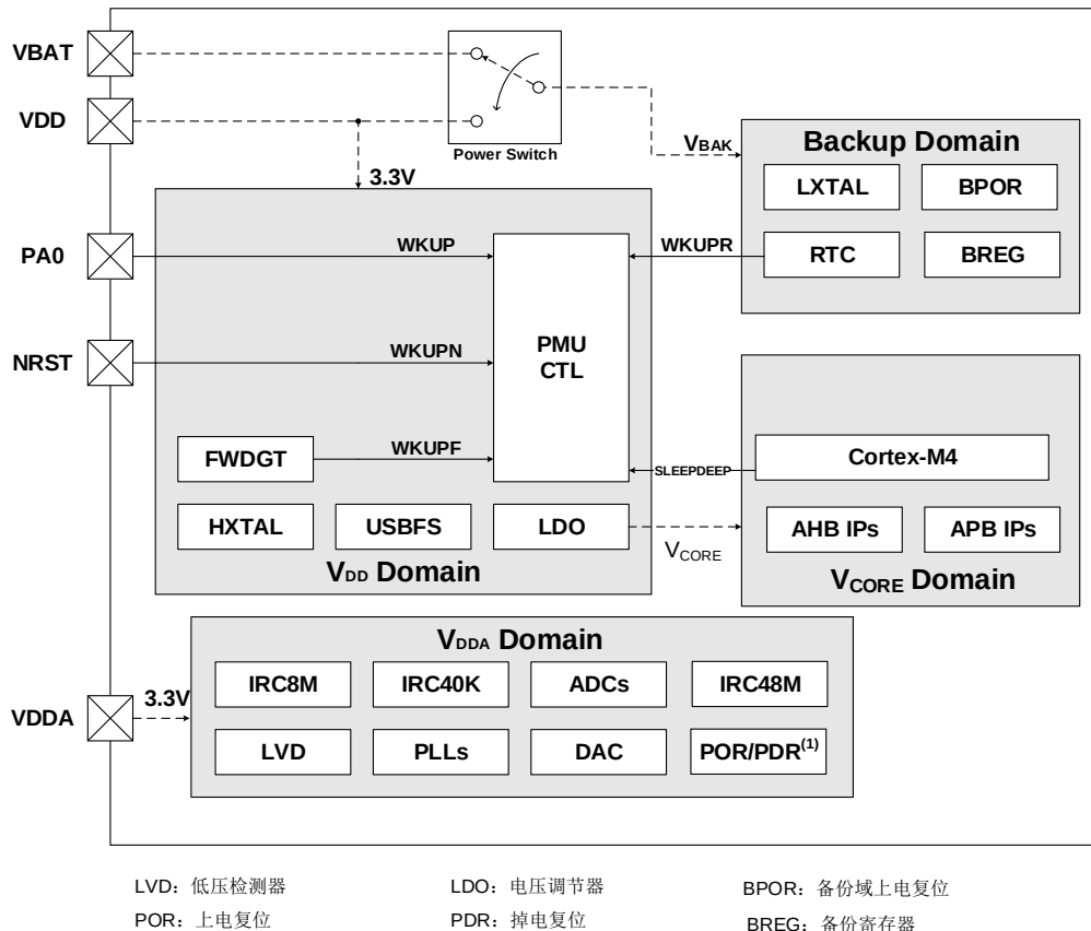
图3-1. 电源域概览
