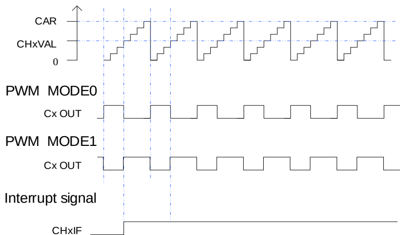
图 18-55. EAPWM 时序图
