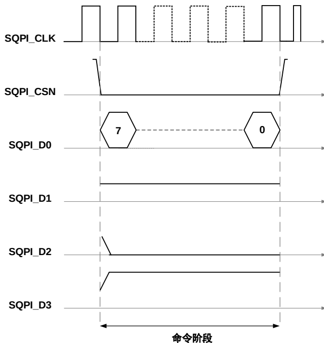
图 23-2. SQPI_SCMD 示例
