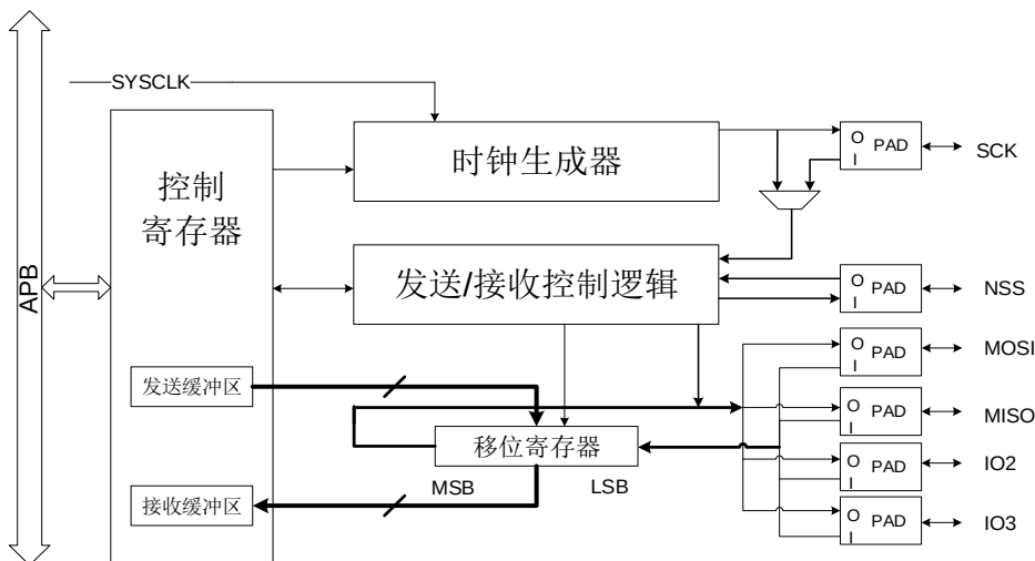
图 22-1. SPI 结构框图
