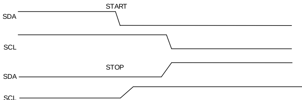
图 21-16. 开始和停止信号
