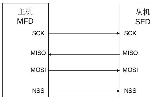
图 22-4. 典型的全双工模式连接
