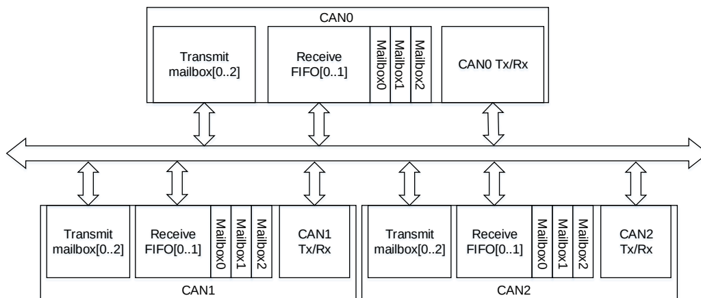
图 26-1. CAN 模块结构框图
