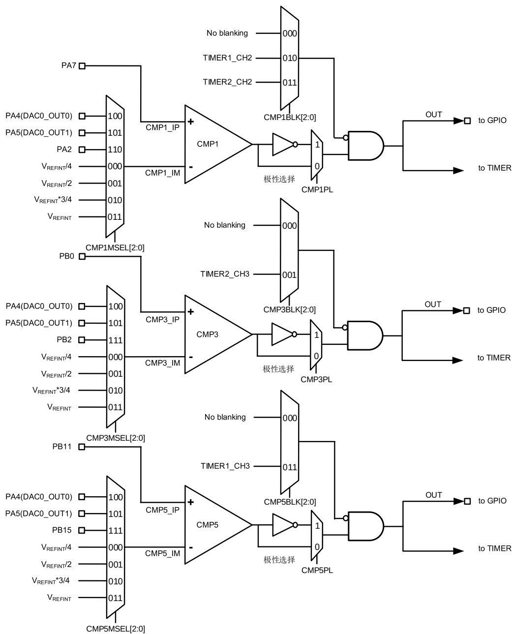
图 15-1.比较器框图
