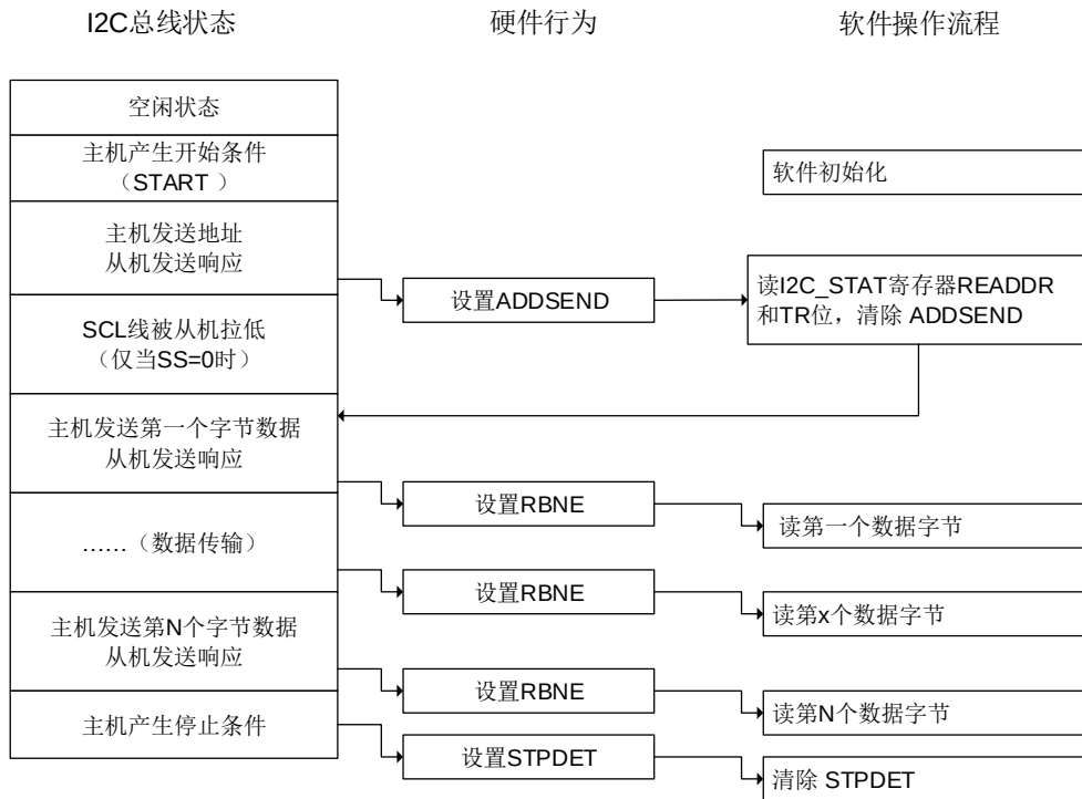
图 21-29. I2C 从机接收编程模型
