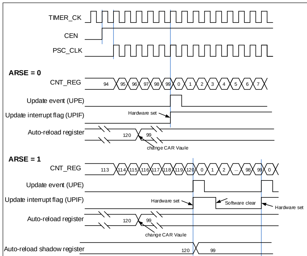
图 18-51. 向上计数时序图, 在运行时改变 TIMERx_CAR 寄存器的值
