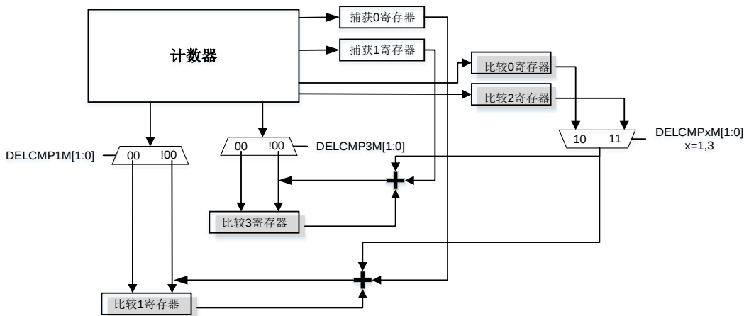
图 19-13. 比较延迟模式框图
