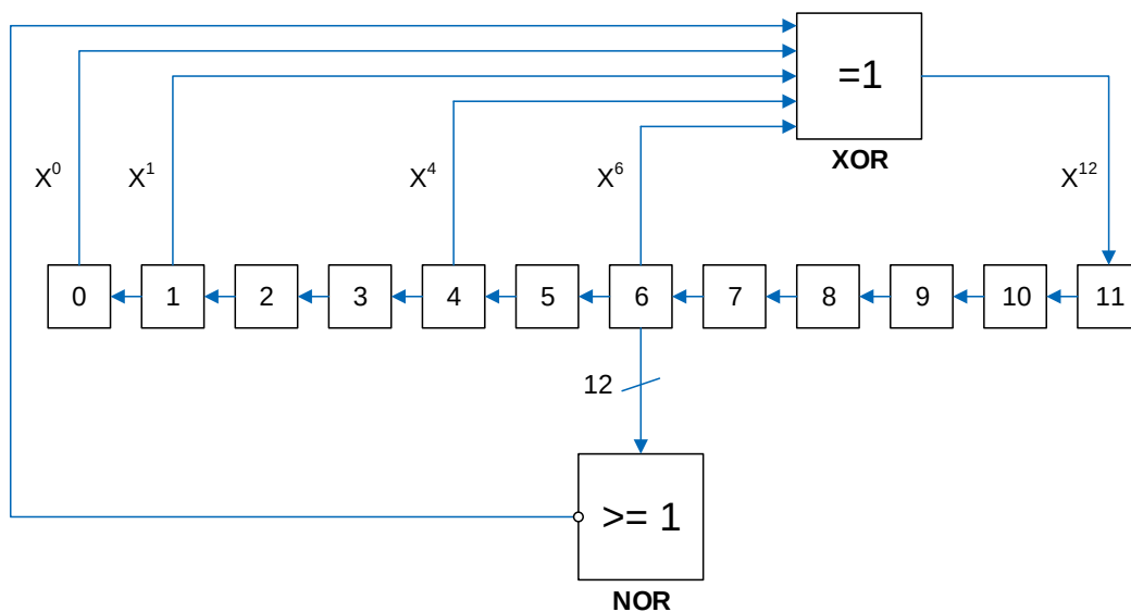
图 14-2. DAC LFSR 算法
