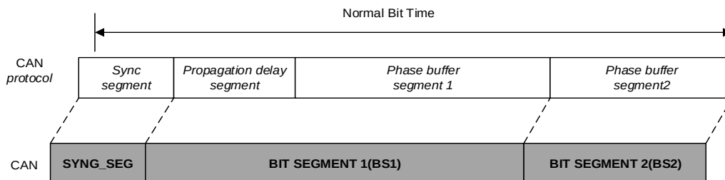
图 26-11. 位时序
