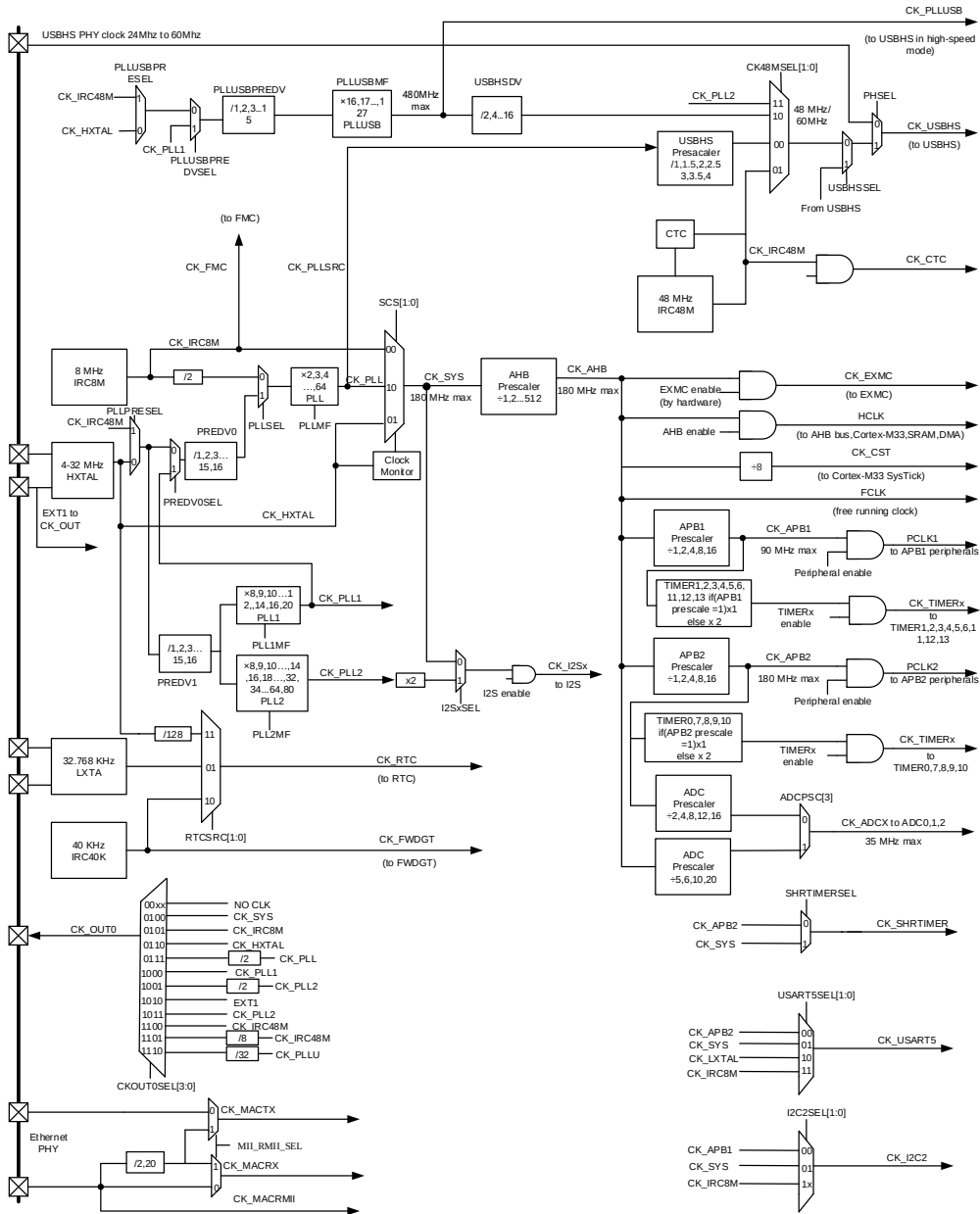
图5-6. 时钟树
