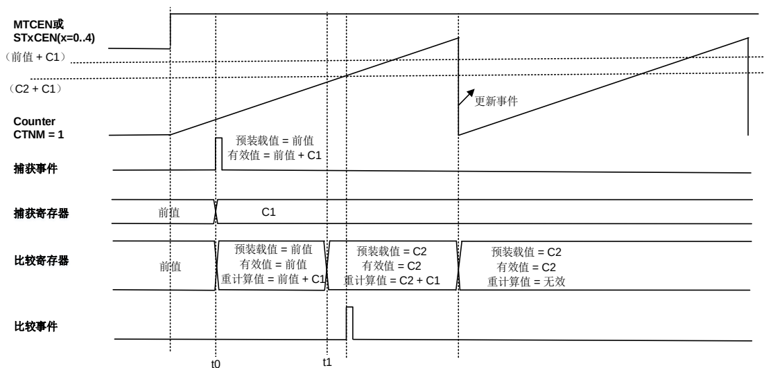
图 19-16. 比较延迟模式 (SHWEN=0)
