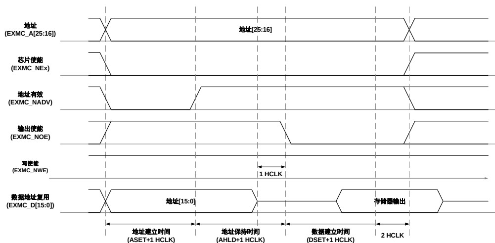
图 25-17. 复用模式读时序
