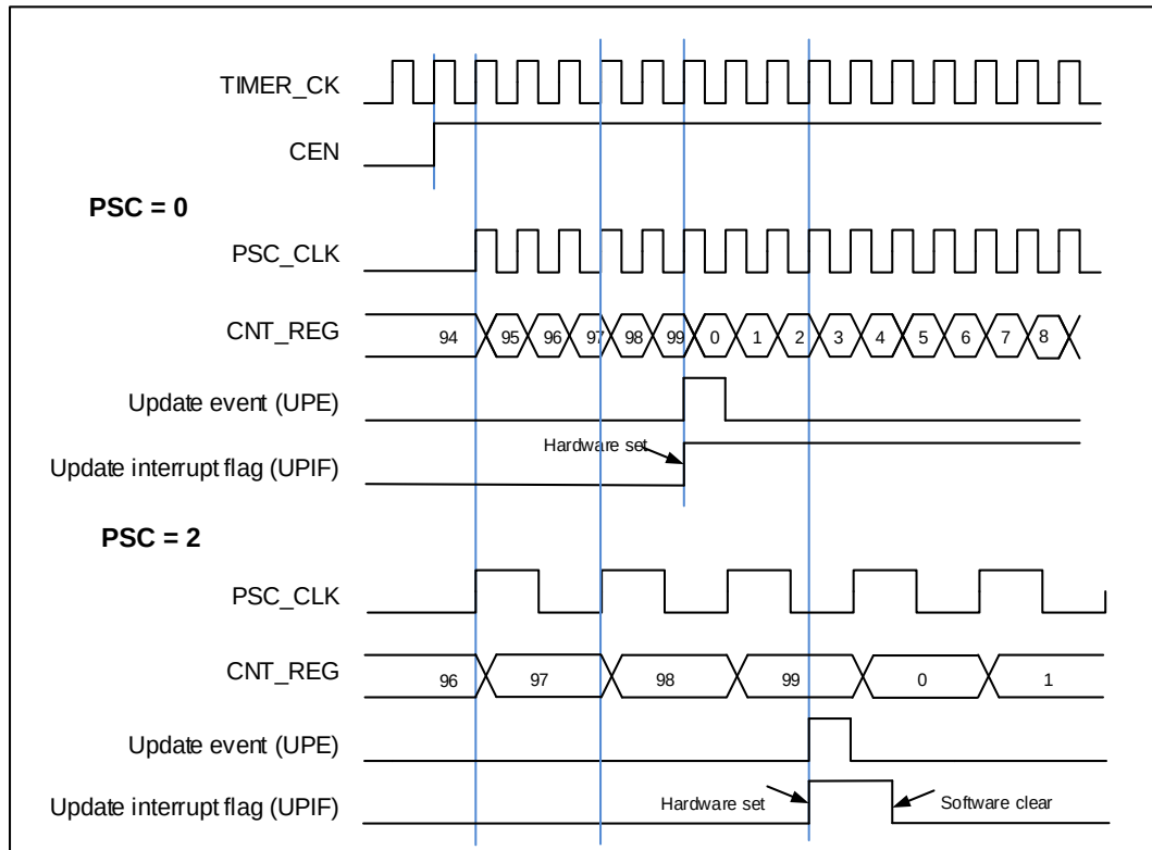
图 18-71. 向上计数时序图， PSC=0/2
