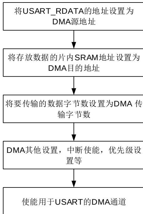
图 20-22. 采用 DMA 方式实现 USART 数据接收配置步骤
