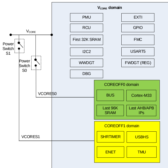
图 4-2. V CORE 电源域概览
