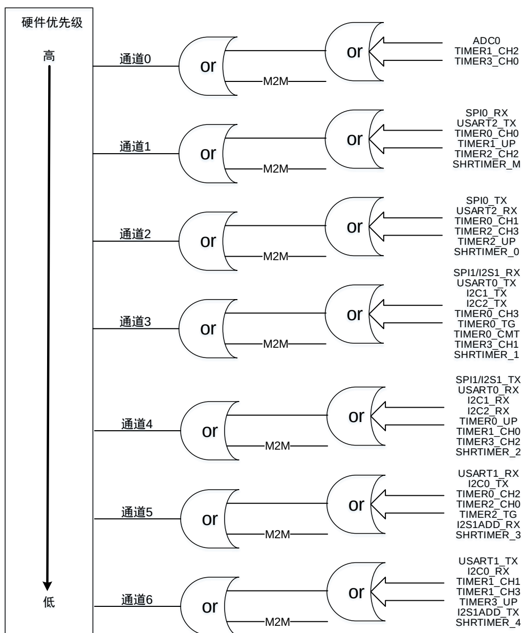
图 11-4. DMA0 请求映射
