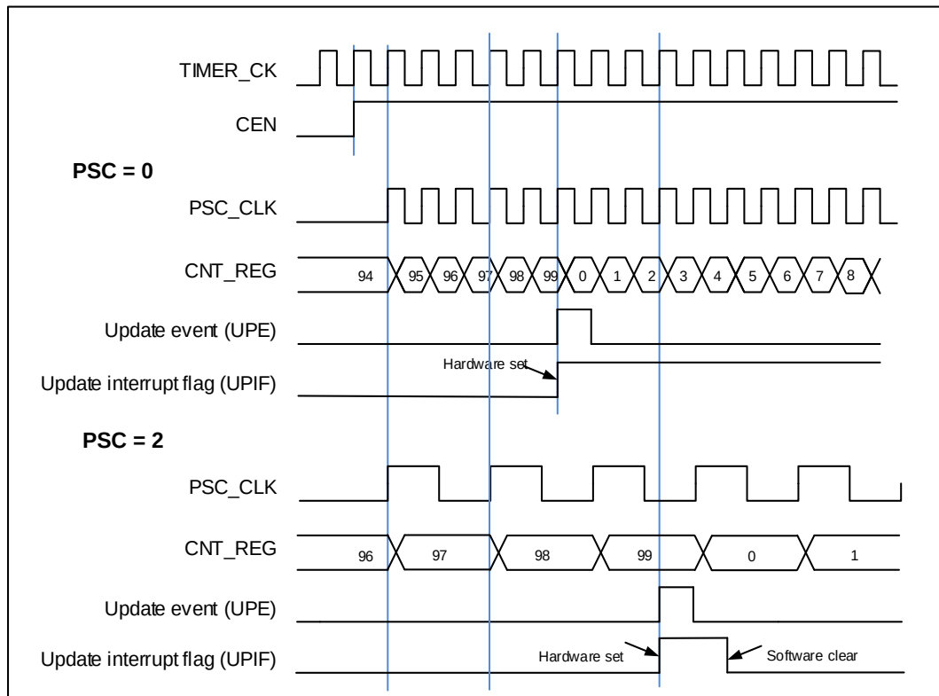
图 18-33. 向上计数时序图, PSC=0/2
