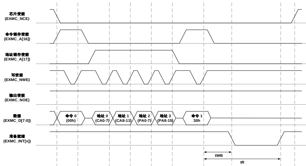
图 25-24. NCE 敏感 NAND Flash 访问时序
