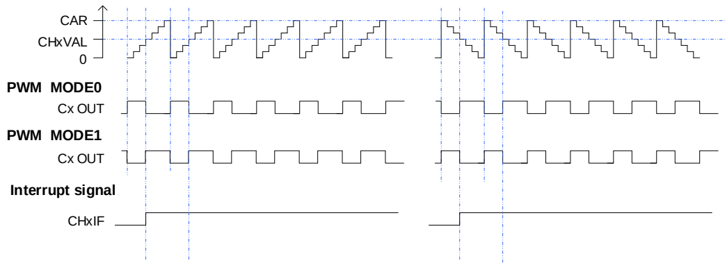
图 18-42. CAPWM 时序图
