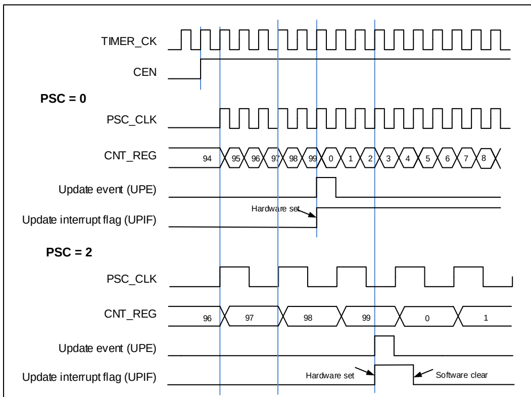
图 18-63. 向上计数时序图，PSC=0/2
