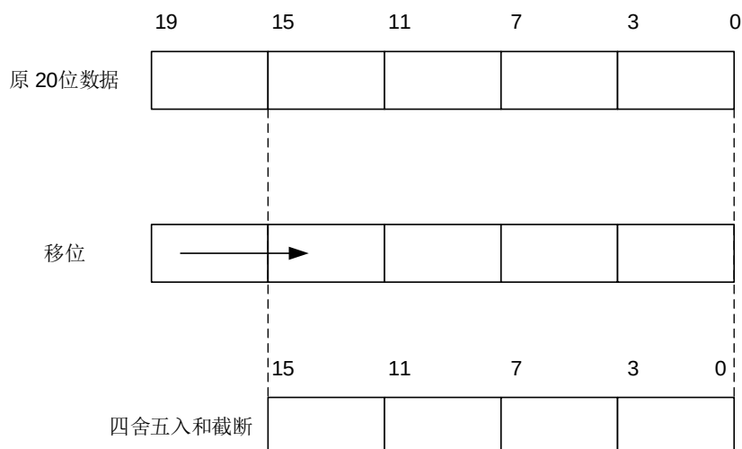
图 13-10. 20 位到 16 位的结果截断
