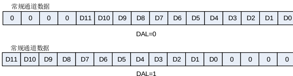
图 13-8. 12 位数据存储模式
