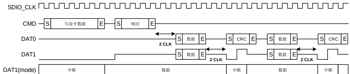
图 24-18. 4 位模式下多块写中断周期时序
