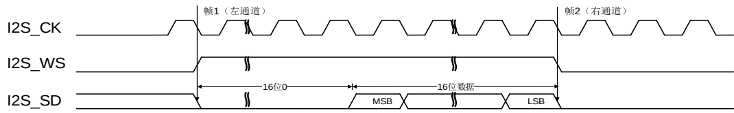
图 22-33. LSB 对齐标准时序图 (DTLEN=00, CHLEN=1, CKPL=0)
