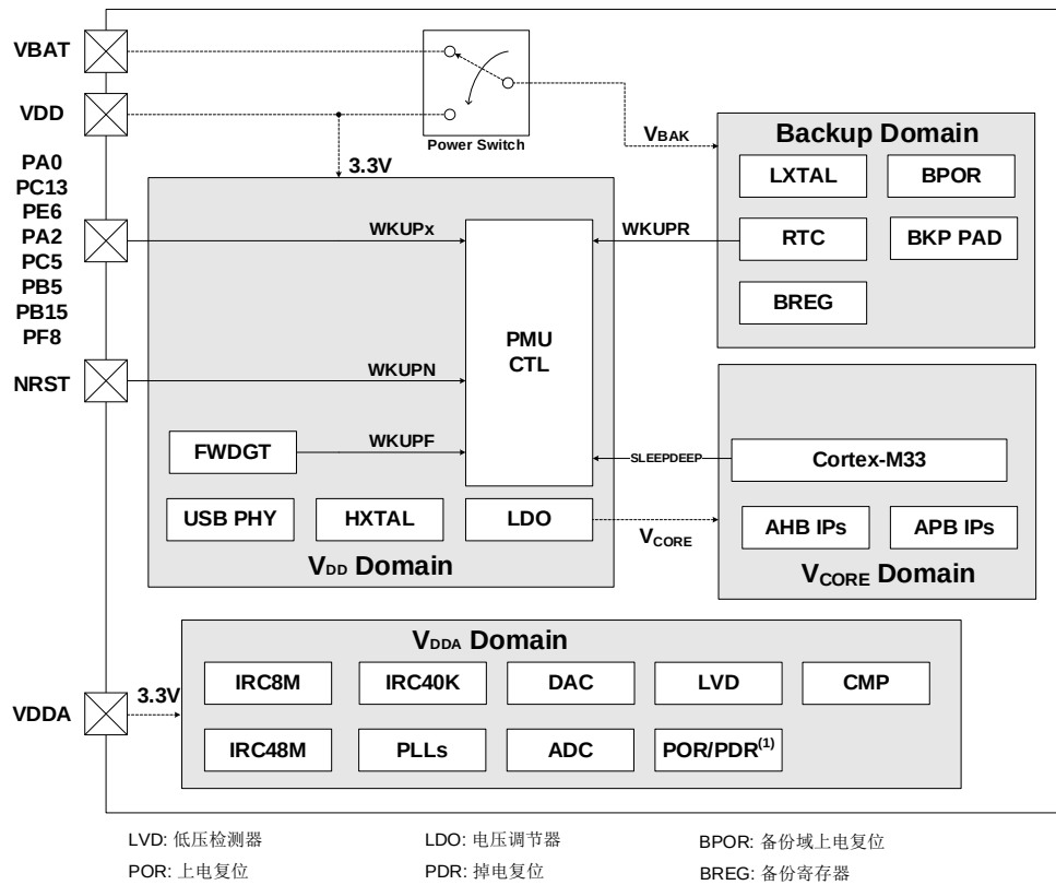
图4-1. 电源域概览
