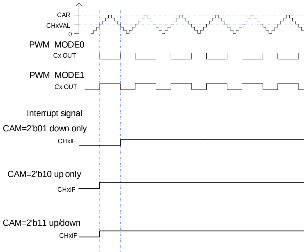
图 18-42. CAPWM 时序图
