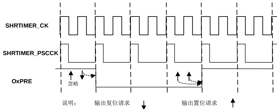
图 19-24. \text{CNTCKDIV}[3:0] = 4'b0110 时的 OxpRE 波形
