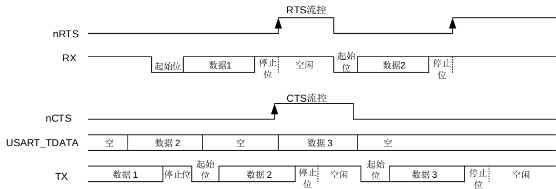
图 20-8. 硬件流控制
