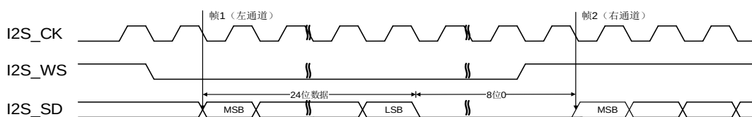
图 22-19. I2S 飞利浦标准时序图 (DTLEN=01, CHLEN=1, CKPL=0)
