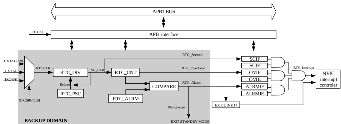
图 17-1. RTC 框图
