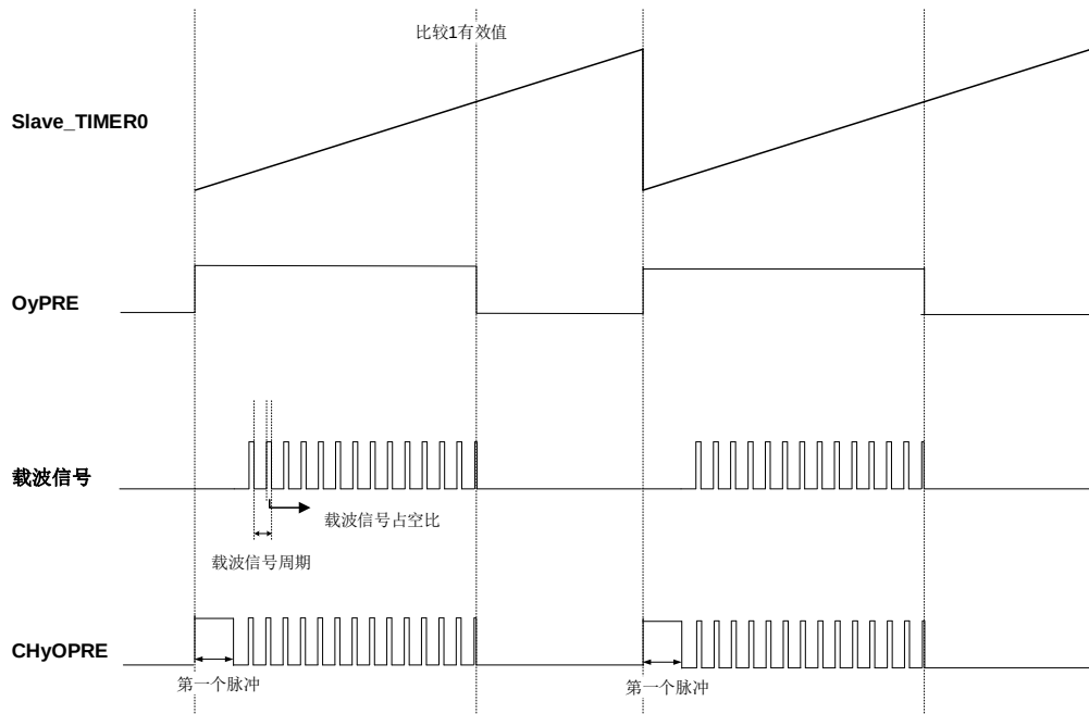
图 19-37. 载波模式使能时的 SHRTIMER 输出
