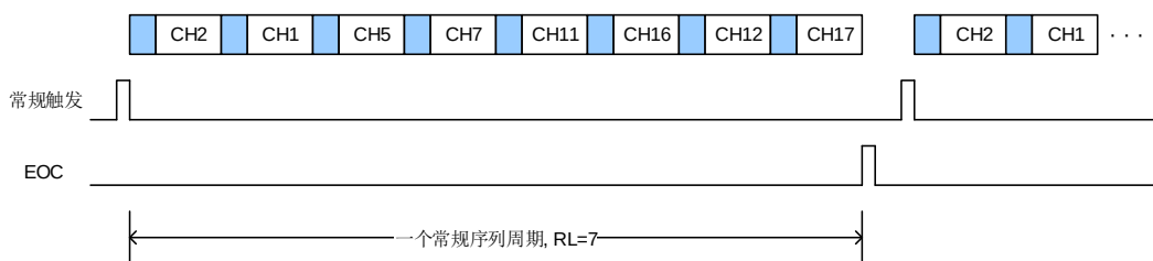
图 13-5. 扫描运行模式，且连续运行模式禁能
