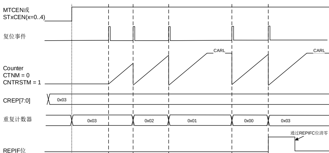
图 19-8. 单脉冲模式下，CNTSTM = 1 时重复计数器的动作
