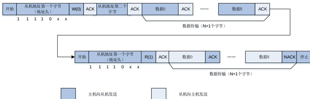
图 21-21. 10 位地址的 I2C 通讯流程（主机接收，HEAD10R=1）
