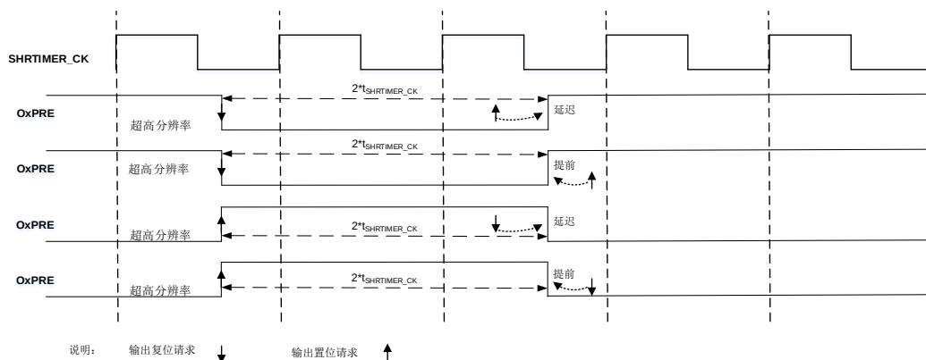
图 19-22. 脉冲宽度为 2 个 t_{\text{SHRTIMER\_CK}} 周期
