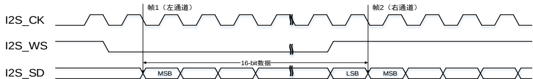
图 22-15. I2S 飞利浦标准时序图（DTLEN=00, CHLEN=0, CKPL=0）
