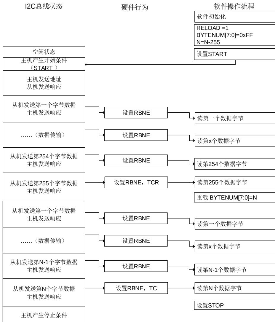
图 21-34. I2C 主机接收编程模型 (N&gt;255)
