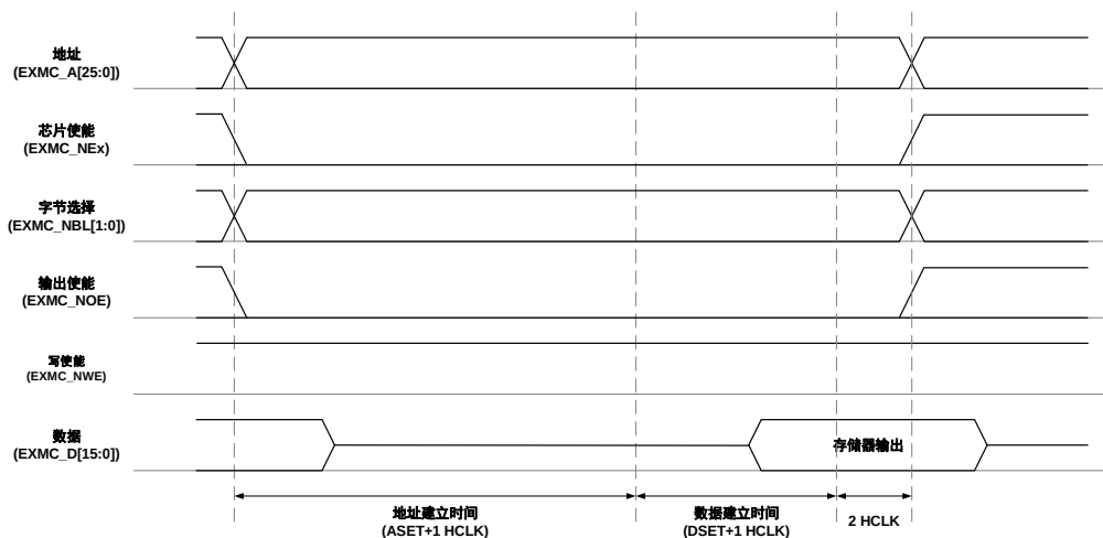
图 25-7. 模式 1 写时序
