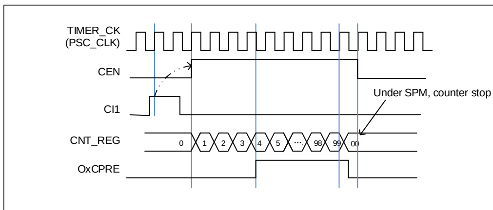
图 18-59. 单脉冲模式， TIMERx\_CHxCV = 4 TIMERx\_CAR=99
