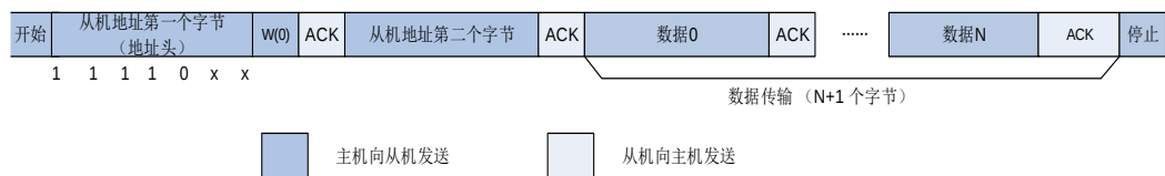
图 21-17. 10 位地址的 I2C 通讯流程（主机发送）
