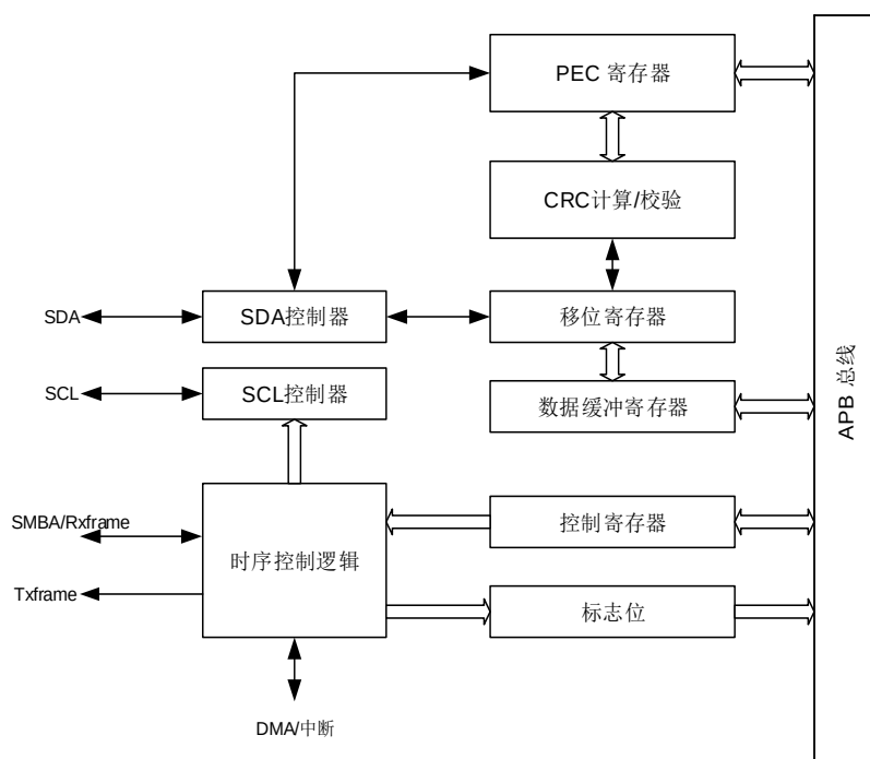
图 21-1. I2C 模块框图
