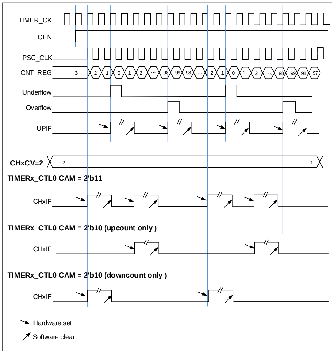
图 18-37. 中央计数模式计数器时序图
