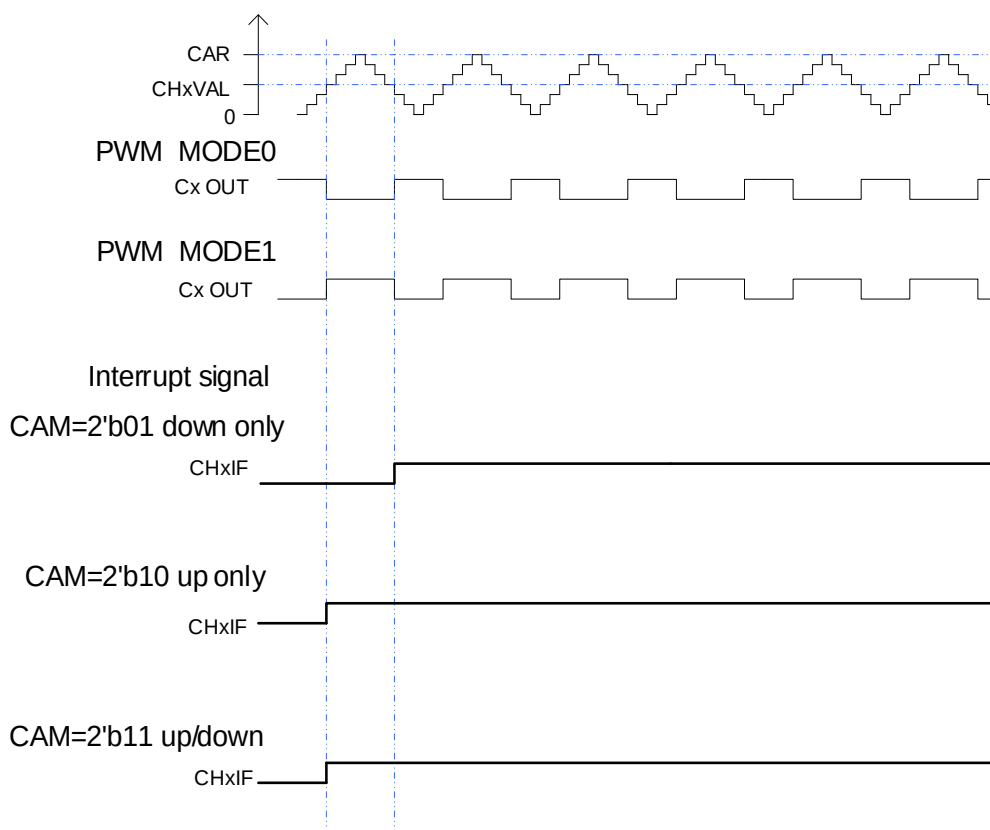
图 18-17. CAPWM 时序图
