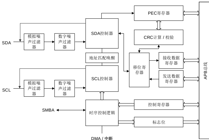
图 21-14. I2C 模块框图
