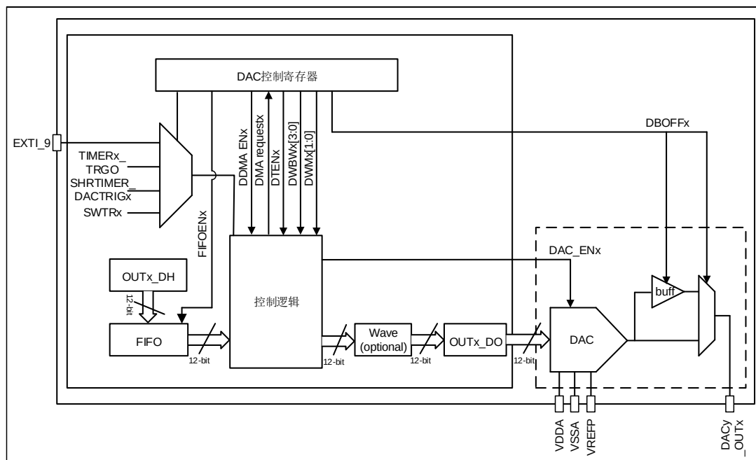
图 14-1. DAC 结构框图
