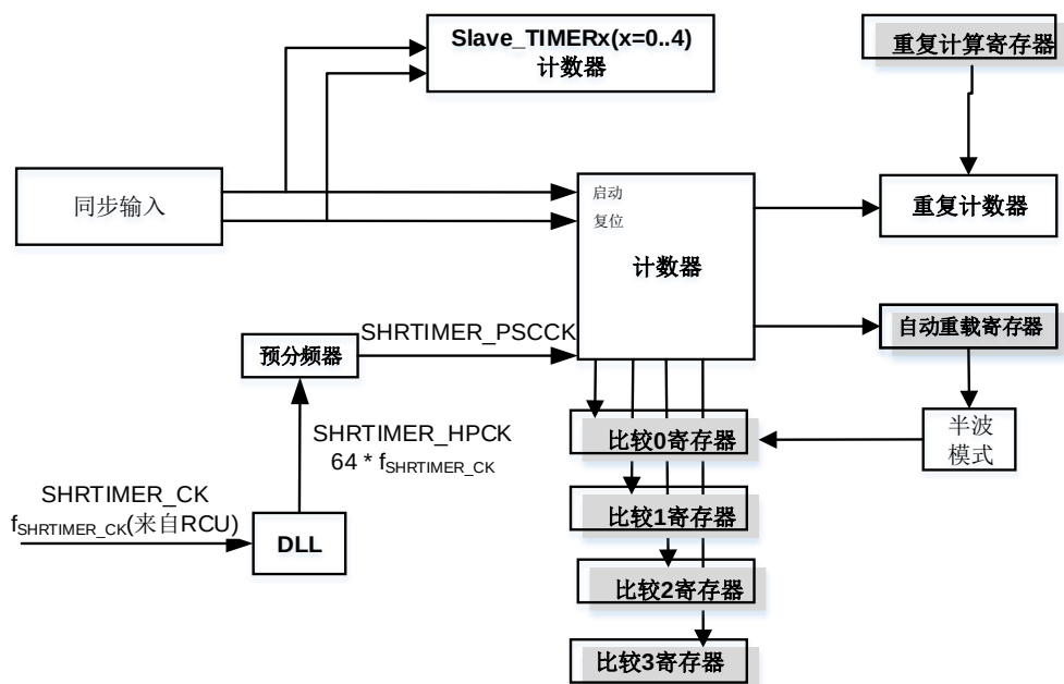
图 19-2. Master_TIMER 结构图
