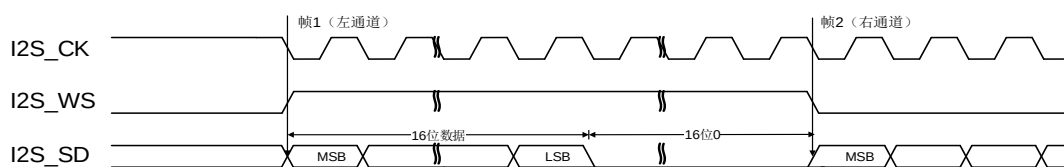
图 22-30. MSB 对齐标准时序图 (DTLEN=00, CHLEN=1, CKPL=1)
