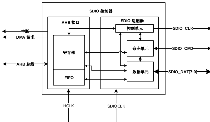
图 24-6. SDIO 框图
