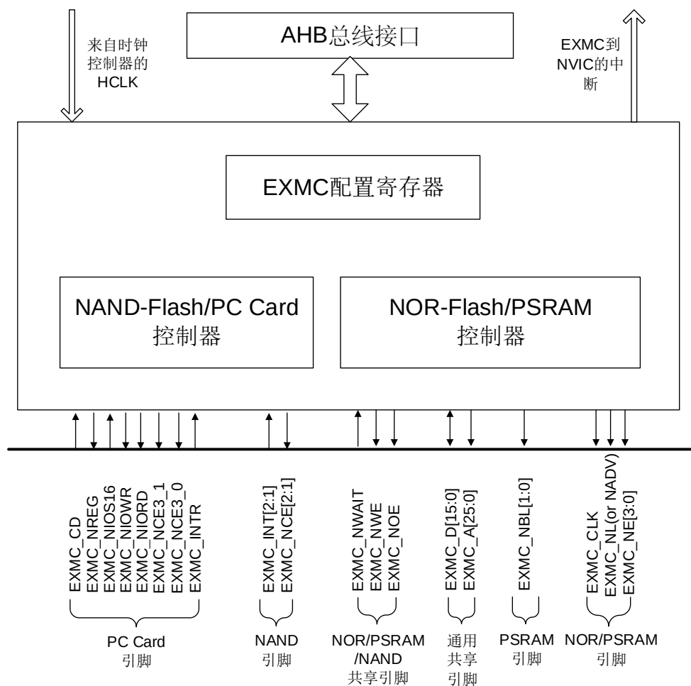
图 25-1. 系统架构
