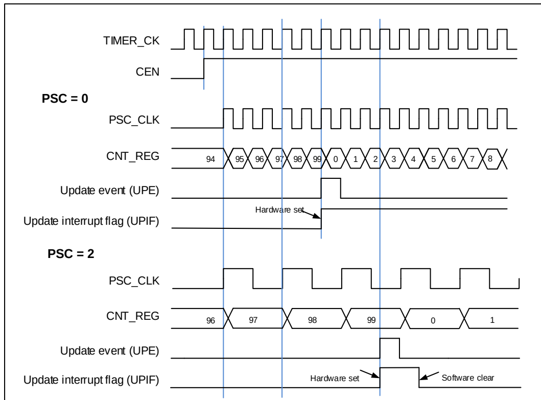
图 18-50. 向上计数时序图, PSC=0/2
