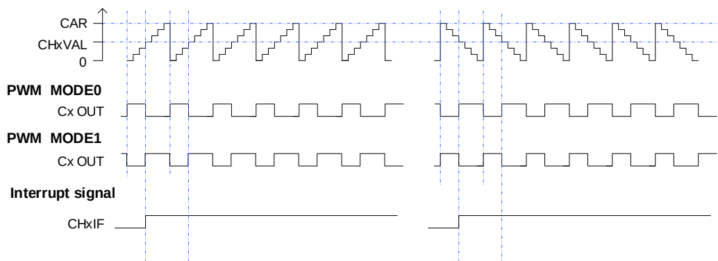
图 18-17. CAPWM 时序图
