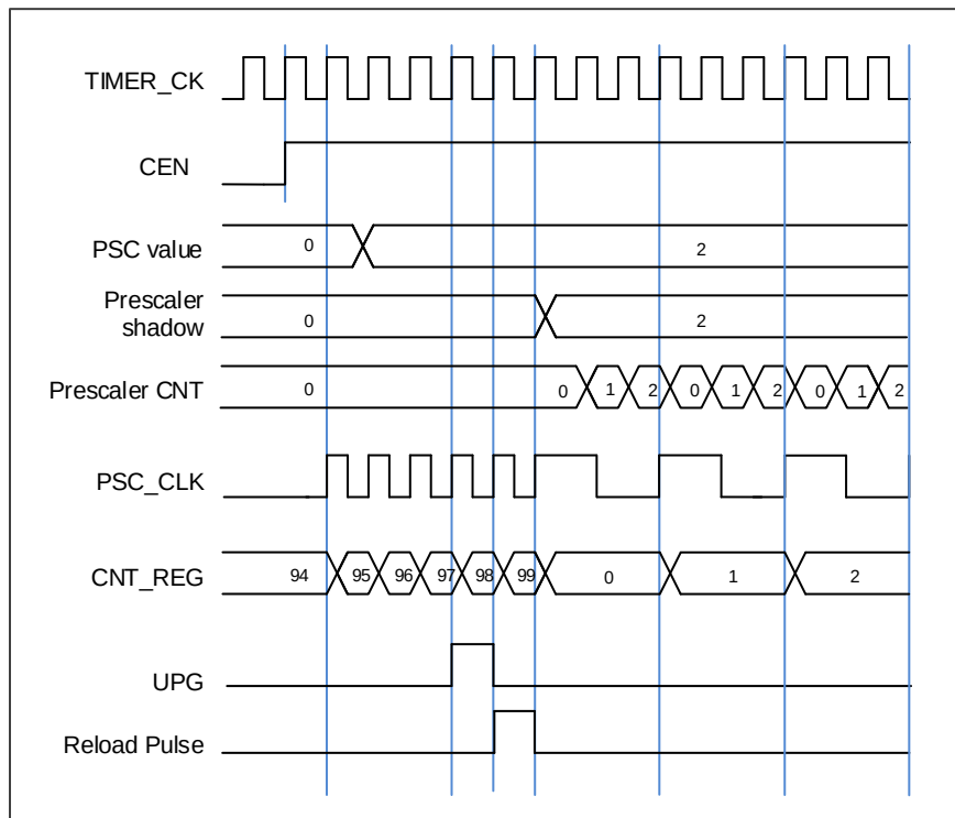
图 18-32. 当 PSC 数值从 0 变到 2 时，计数器的时序图
