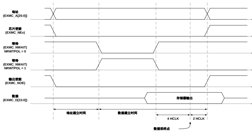
图 25-19. 异步等待有效时的读时序
