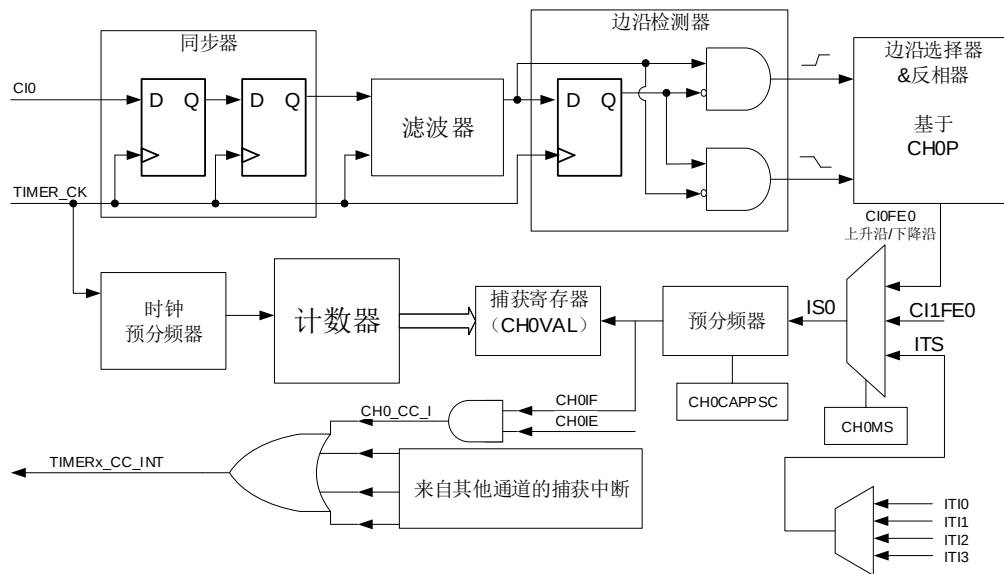
图 18-38. 通道输入捕获原理
