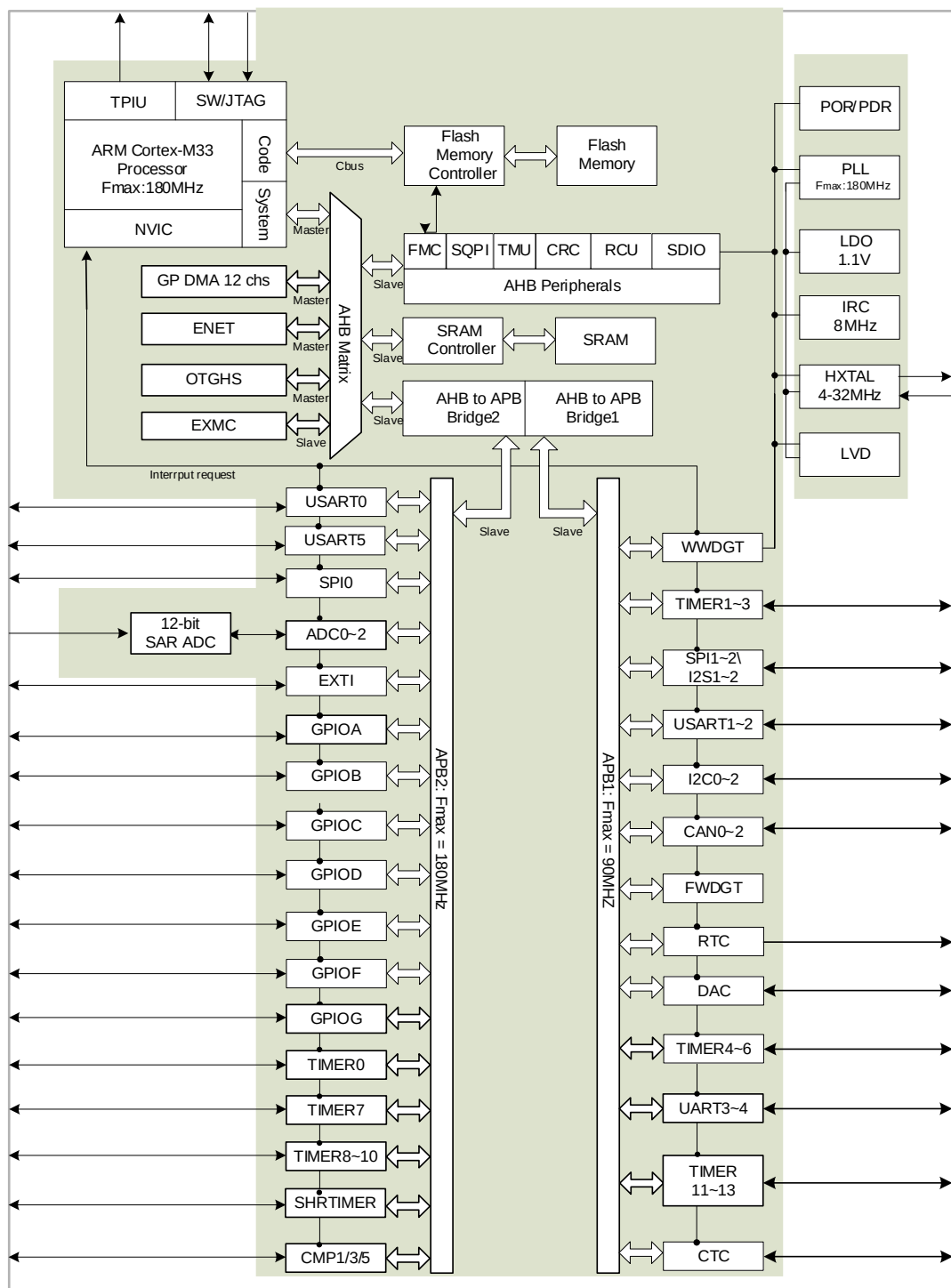
图 1-2. GD32E50x 系列器件的系统架构示意图
