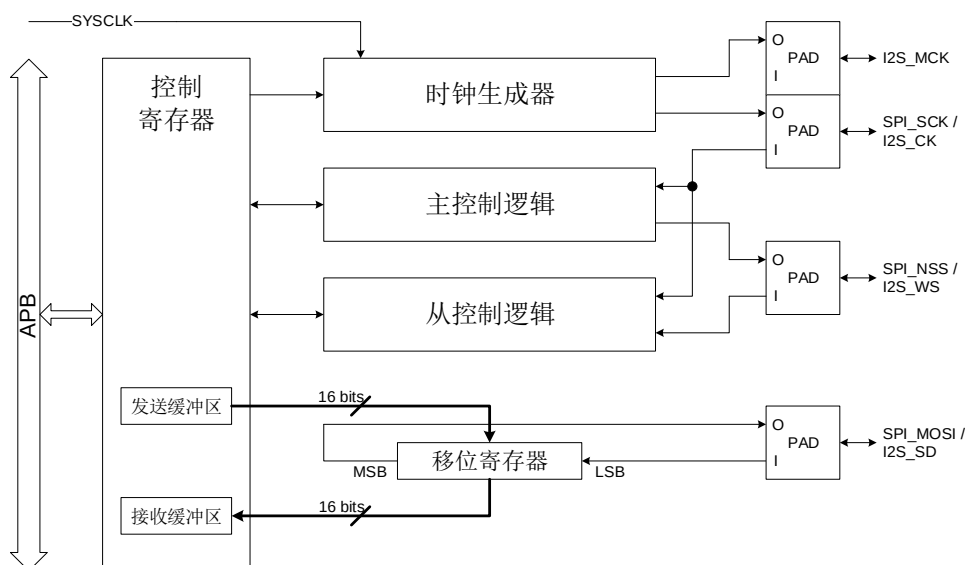
图 22-14. I2S 结构框图
