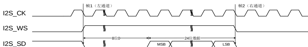
图 22-31. LSB 对齐标准时序图 (DTLEN=01, CHLEN=1, CKPL=0)
