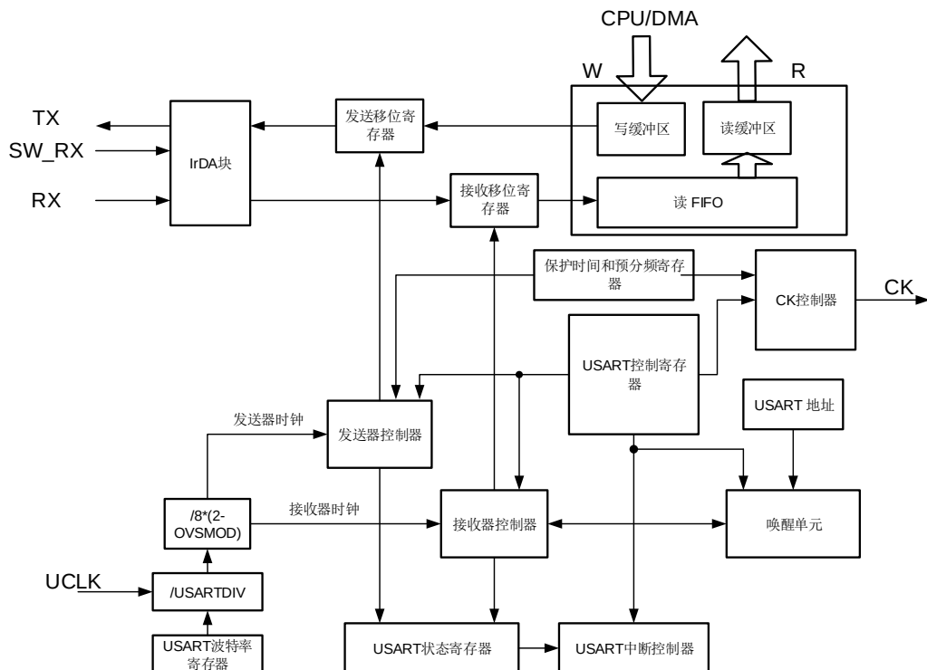
图 20-17. USART 模块内部框图
