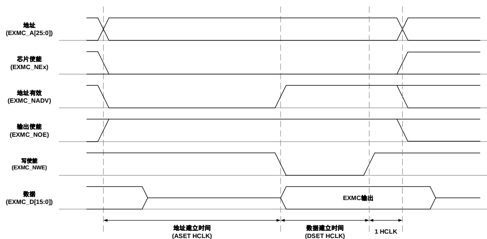
图 25-11. 模式 2 写时序
