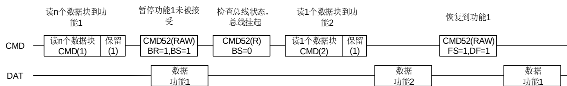
图 24-14. 在功能 1 的多块读周期期间插入功能 2 读周期
