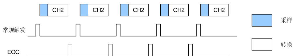
图 13-3. 单次运行模式
