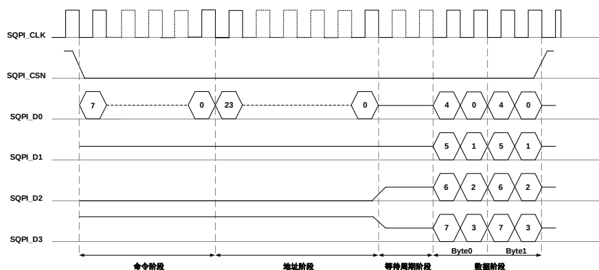
图 23-6. SQPI SSQ 模式时序
