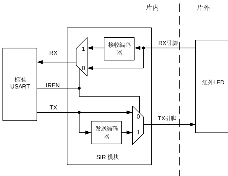
图 20-13. IrDA SIR ENDEC 模块
