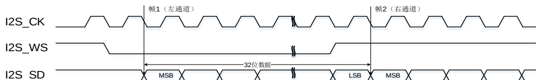
图 22-17. I2S 飞利浦标准时序图（DTLEN=10, CHLEN=1, CKPL=0）
