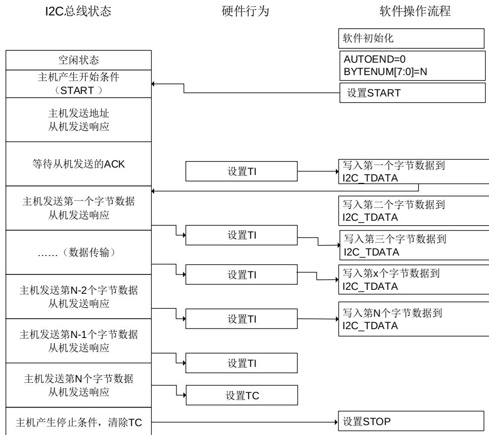
图 21-31. I2C 主机发送编程模型 ( N \leq 255 )
