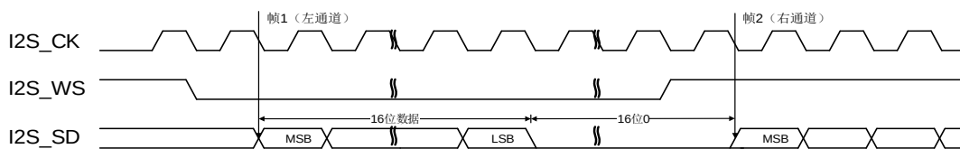
图 22-21. I2S 飞利浦标准时序图 (DTLEN=00, CHLEN=1, CKPL=0)
