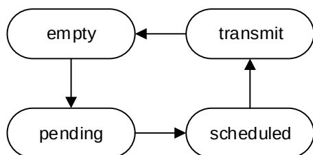
图 26-3. 发送邮箱状态转换
