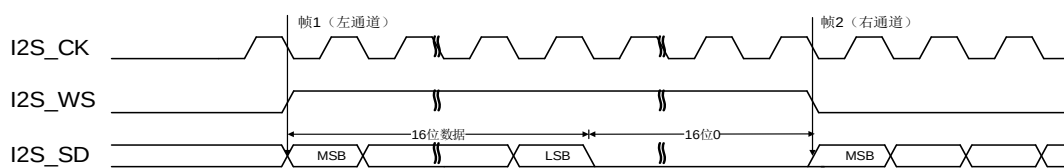
图 22-29. MSB 对齐标准时序图 (DTLEN=00, CHLEN=1, CKPL=0)
