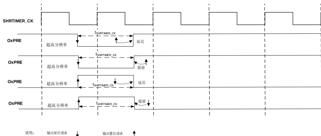
图 19-21. 脉冲宽度为 1 个 t_{SHRTMER\_CK} 周期
