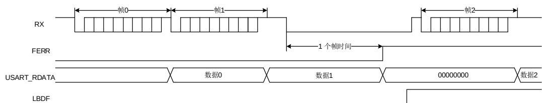
图 20-23. 空闲状态下检测断开帧
