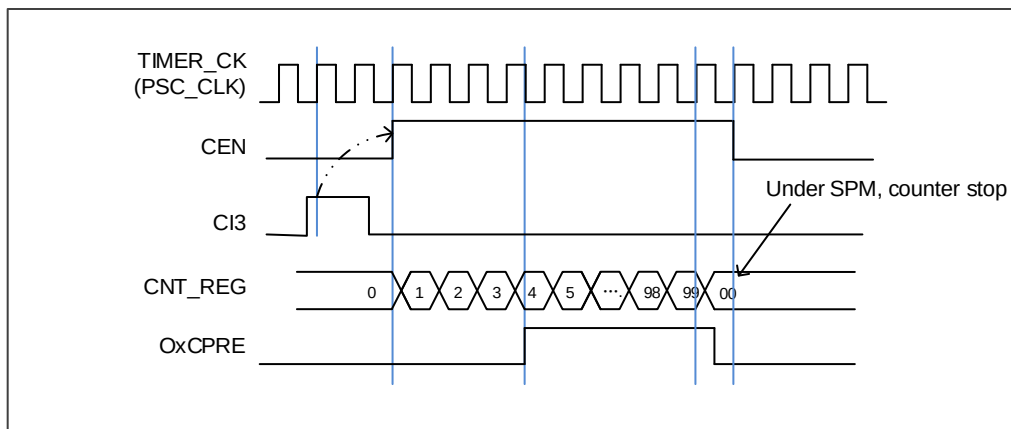
图 18-27. 单脉冲模式， TIMERx_CHxCV = 4 ， TIMERx_CAR=99
