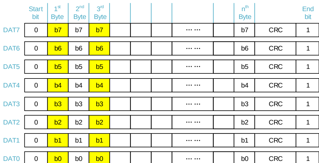
图 24-11. 8 位数据总线宽度
