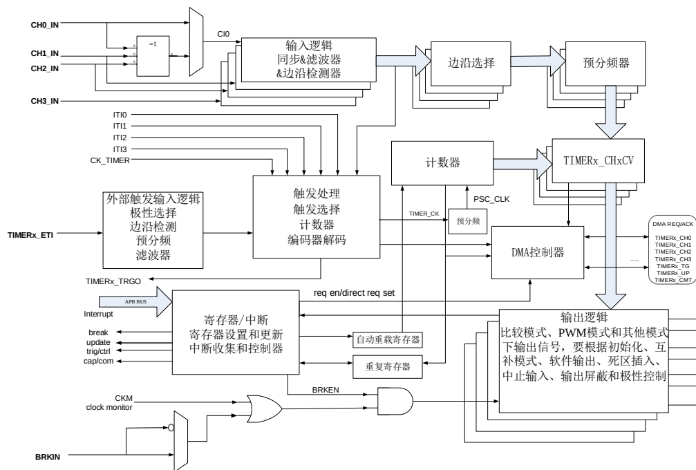
图 18-1. 高级定时器结构框图
