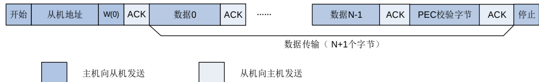
图 21-35. SMBus 主机发送器和从机接收器通信流程
