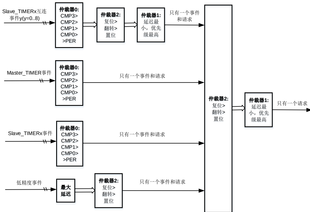
图 19-19. 每个 t_{SHRTIMER\_CK} 周期的仲裁机制过程
