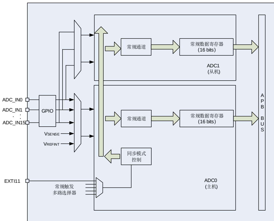
图 13-12. ADC 同步框图
