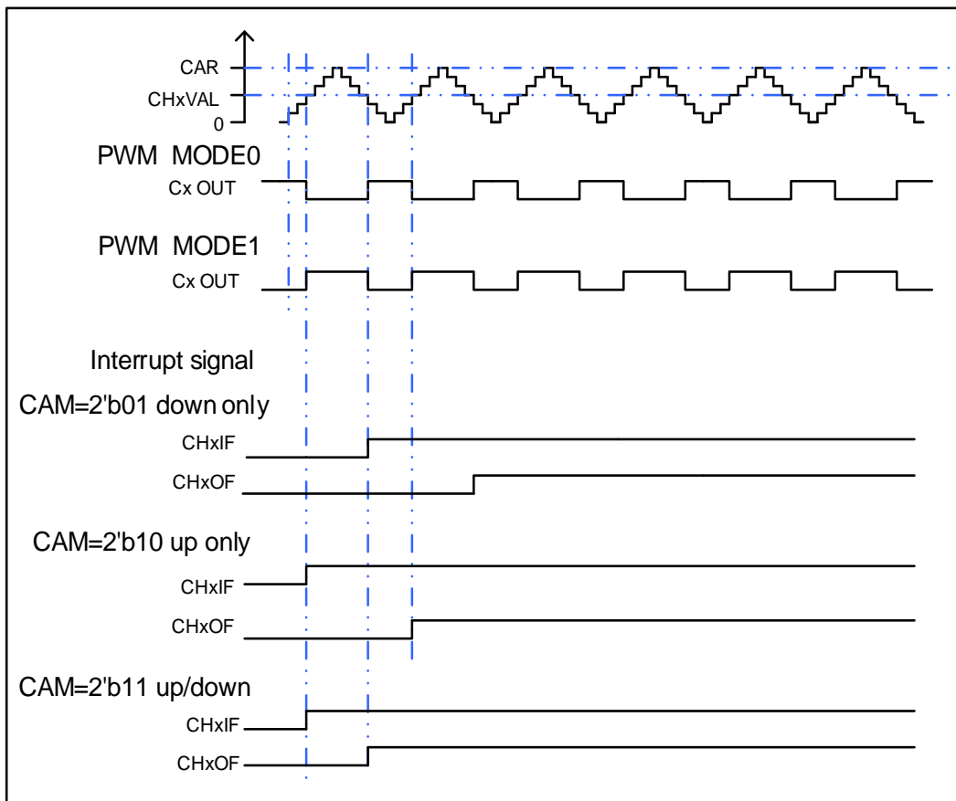
图 15-17. CAPWM 时序图
