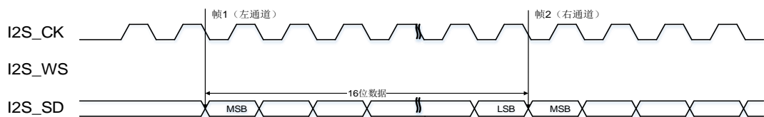
图 18-12. I2S 飞利浦标准时序图 (DTLEN=00, CHLEN=0, CKPL=0)
