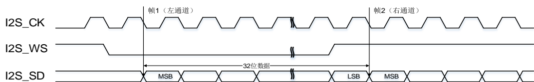
图 18-14. I2S 飞利浦标准时序图 (DTLEN=10, CHLEN=1, CKPL=0)
