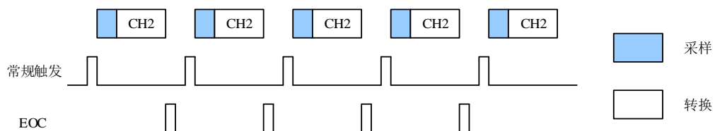
图 11-2. 单次运行模式
