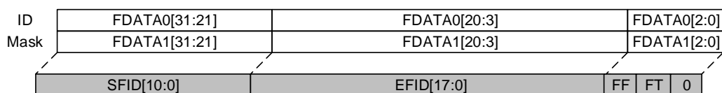
图 20-7. 32-bit 位宽掩码模式过滤器
