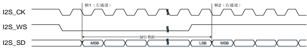
图 18-15. I2S 飞利浦标准时序图 (DTLEN=10, CHLEN=1, CKPL=1)
