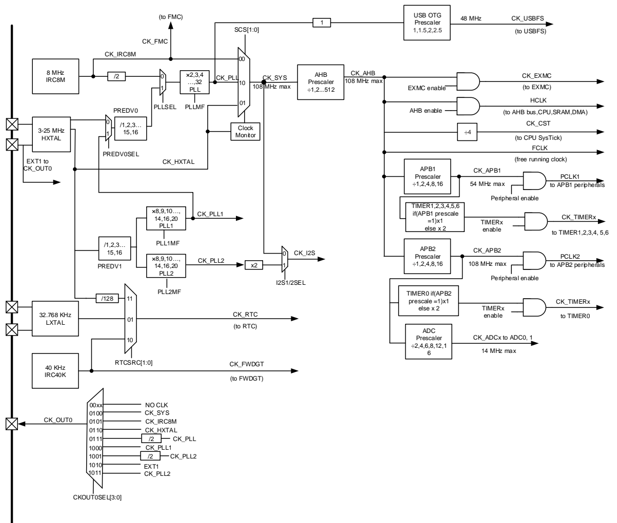
图5-2. 时钟树
