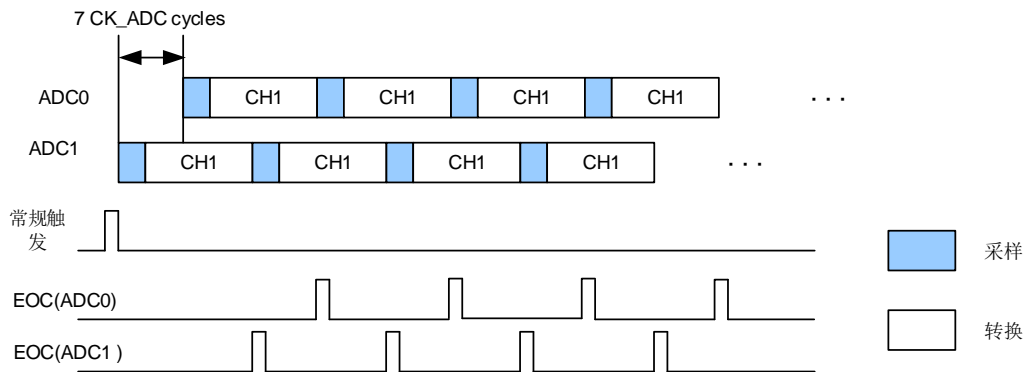
图 11-13. 常规序列上的快速交叉模式（两个 ADC 的 CTN=1）
