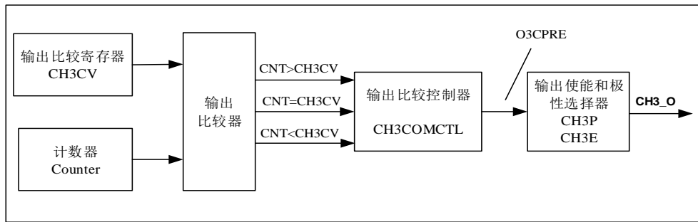
图 15-14. 输出比较原理
