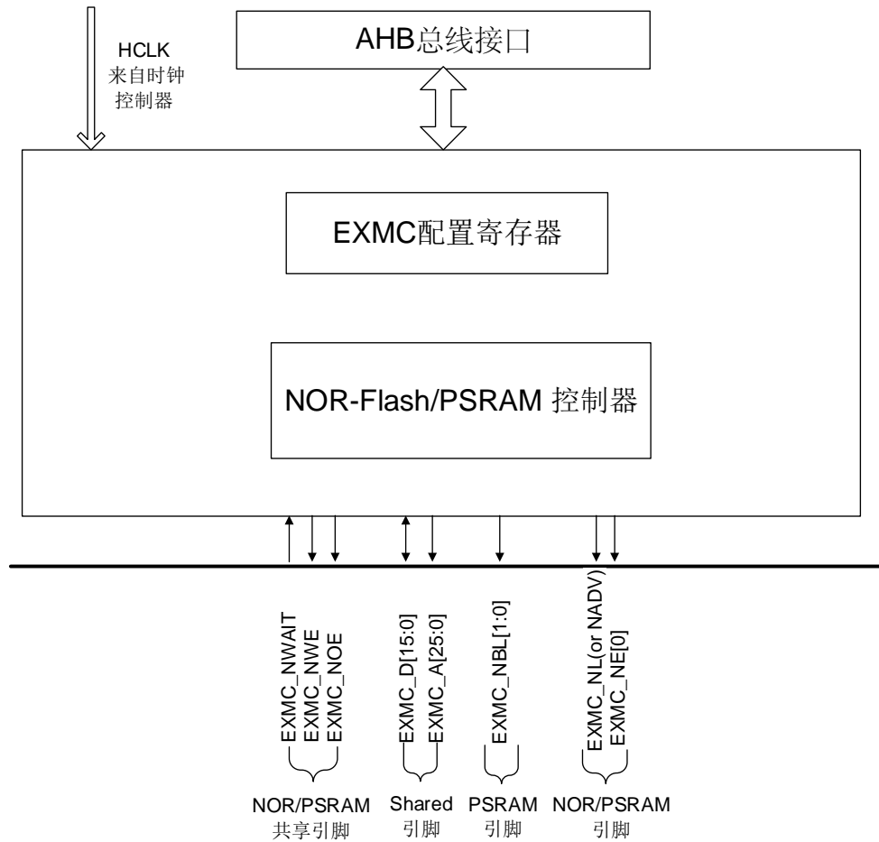
图 19-1. 系统架构
