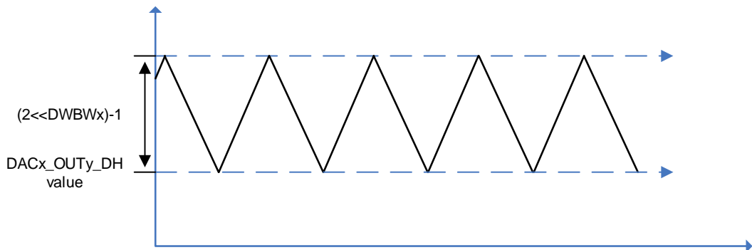
图 12-3. DAC 三角噪声模式生成的波形
