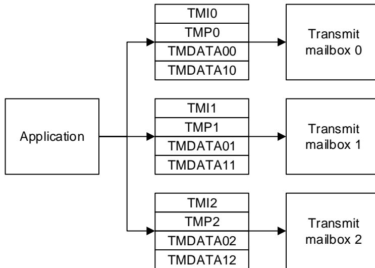
图 20-2. 发送寄存器
