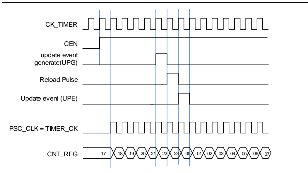
图 15-43. 内部时钟分频为 1 时，计数器的时序图
