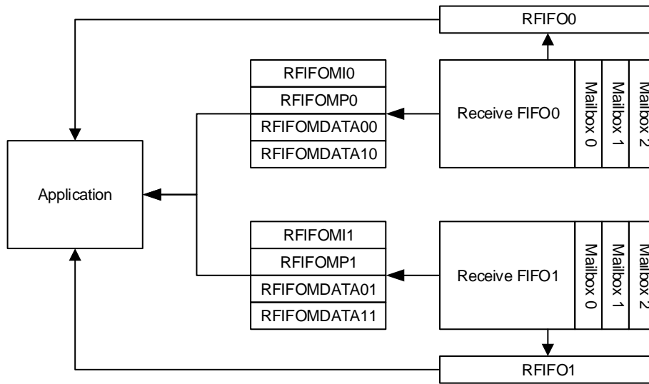
图 20-4. 接收寄存器
