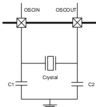
图5-3. HXTAL时钟源
