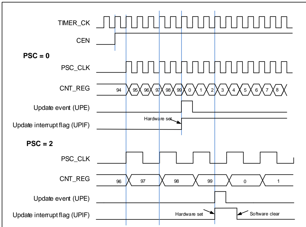
图 15-4. 向上计数时序图, PSC=0/2
