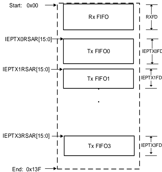
图 21-7. 设备模式 FIFO 空间
