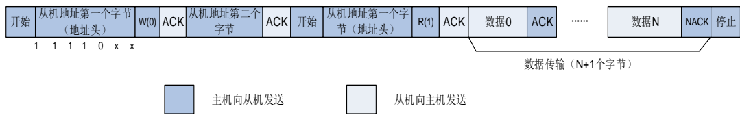
图 17-8. 10 位地址的 I2C 通讯流程（主机接收）
