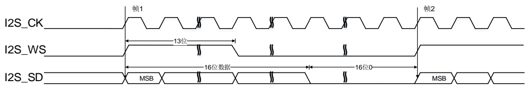
图 18-46. PCM 标准长帧同步模式时序图 (DTLEN=00, CHLEN=1, CKPL=0)
