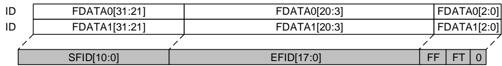
图 20-9. 32-bit 位宽列表模式过滤器
