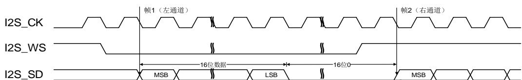
图 18-18. I2S 飞利浦标准时序图 (DTLEN=00, CHLEN=1, CKPL=0)
