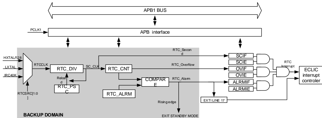
图 14-1. RTC 框图
