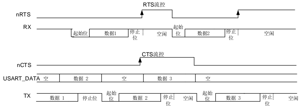
图 16-8. 硬件流控制
