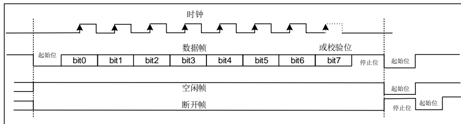
图 16-2. USART 字符帧（8 数据位和 1 停止位）
