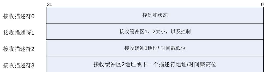
图 27-8. 接收描述符
