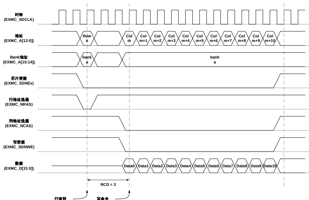
图 25-32. 突发写操作
