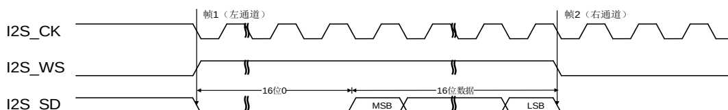
图 21-30. LSB 对齐标准时序图 (DTLEN=00, CHLEN=1, CKPL=1)
