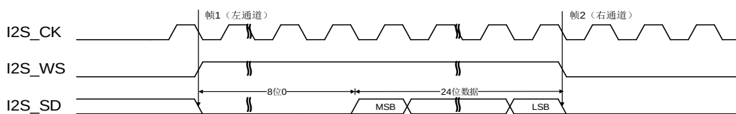
图 21-27. LSB 对齐标准时序图 (DTLEN=01, CHLEN=1, CKPL=0)
