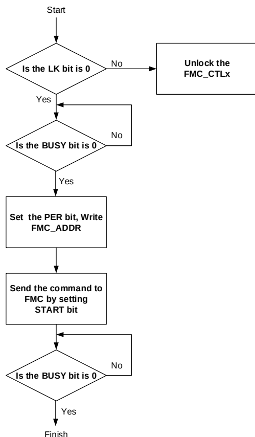
图 2-1. 页擦除操作流程
