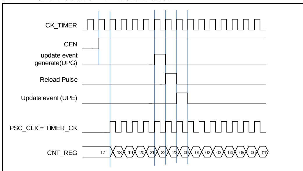
图 18-66. 内部时钟分频为 1 时，计数器的时序图
