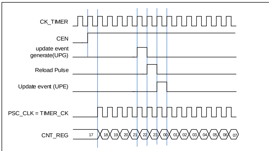
图 18-49. 内部时钟分频为 1 时，计数器的时序图
