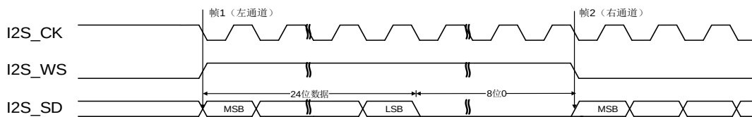
图 21-24. MSB 对齐标准时序图 (DTLEN=01, CHLEN=1, CKPL=1)
