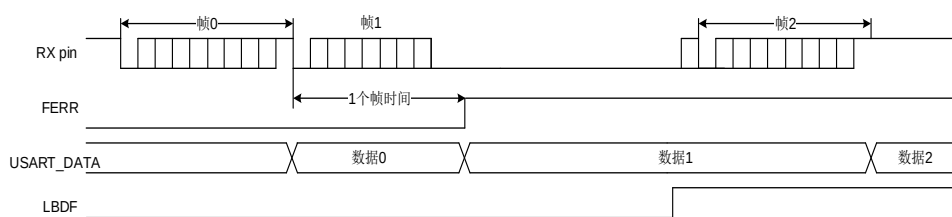
图 19-10. 数据传输过程中检测断开帧
