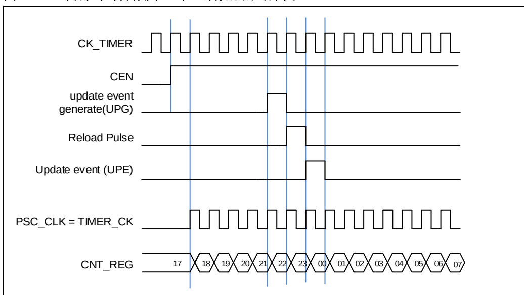
图 18-32. 内部时钟分频为 1 时，计数器的时序图
