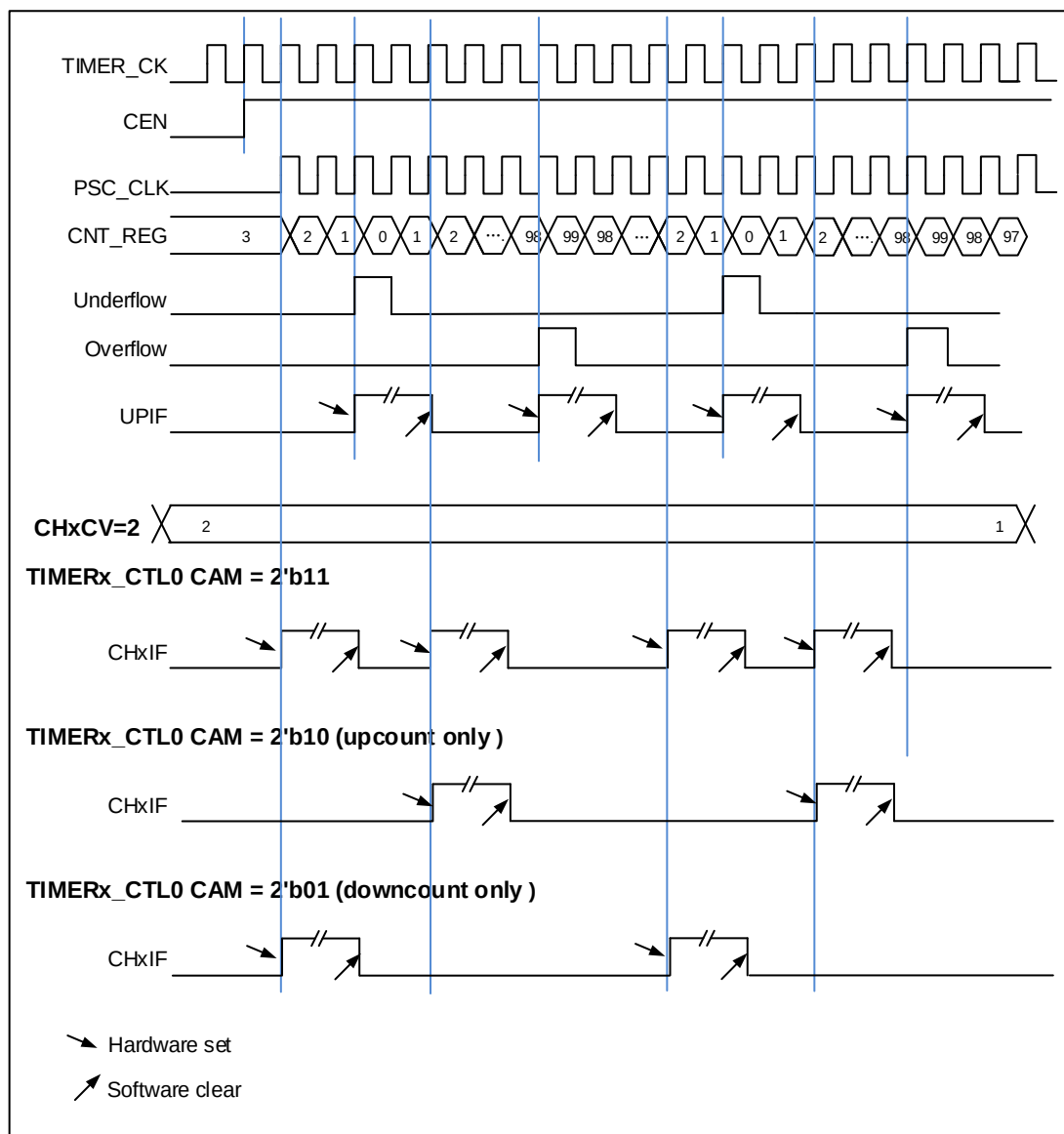
图 18-8. 中央对齐计数模式计数器时序图
