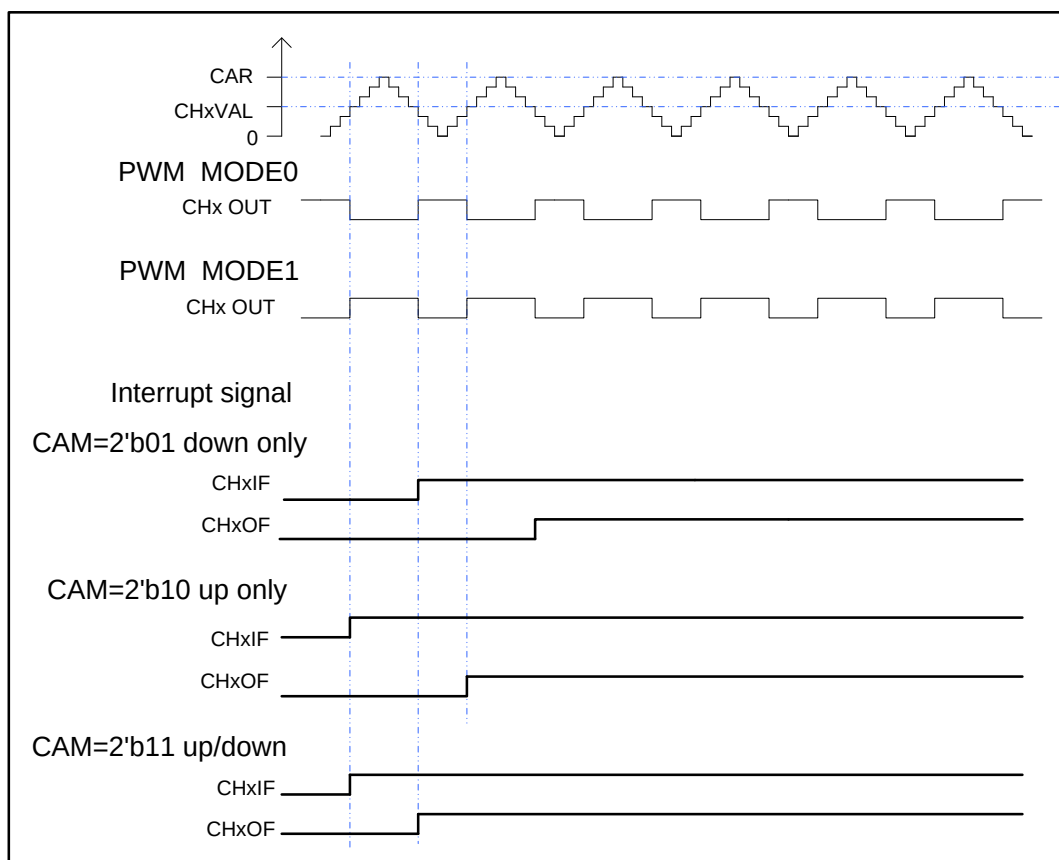
图 18-60. CAPWM 时序图
