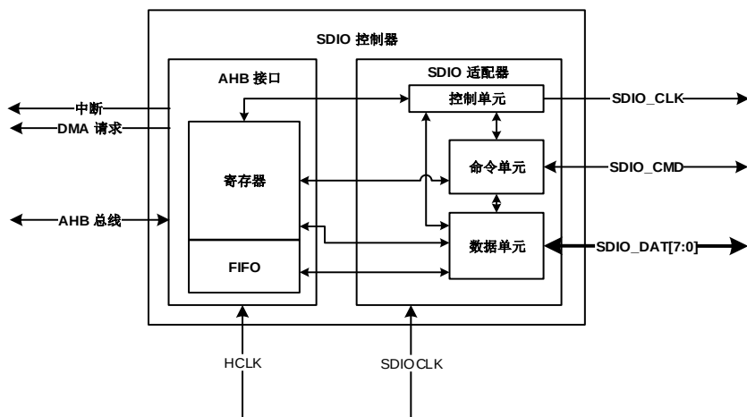
图 24-6. SDIO 框图
