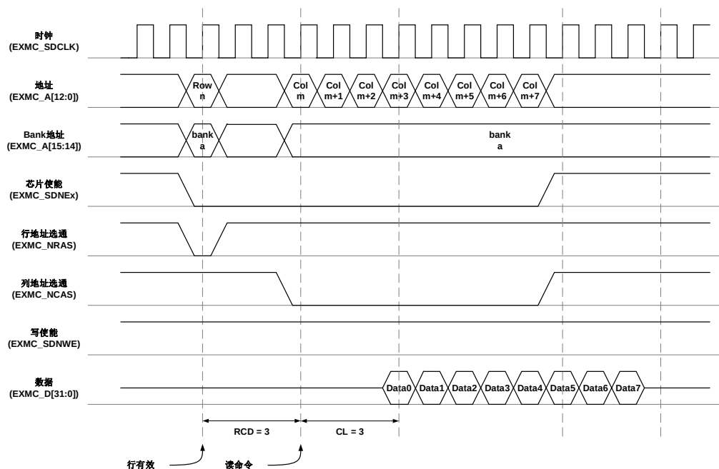
图 25-30. 突发读操作
