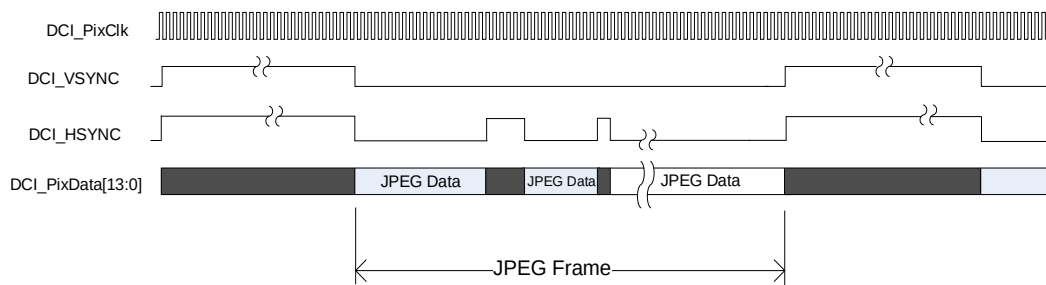
图 22-3. 硬件同步模式之 JPEG 子模式
