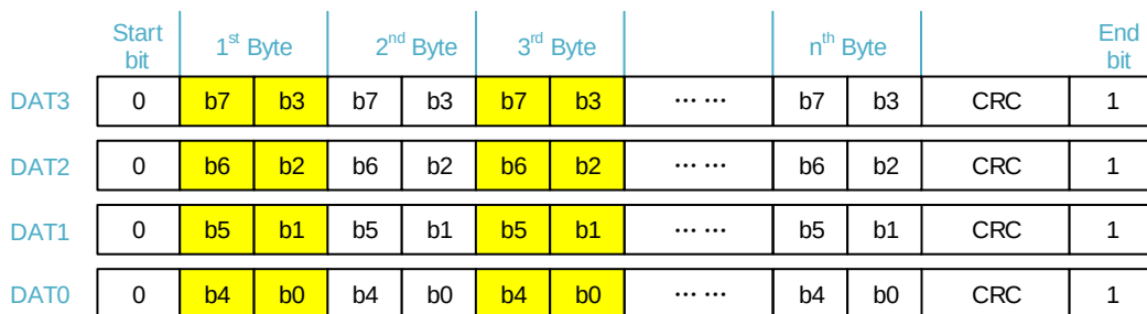
图 24-10. 4 位数据总线宽度
