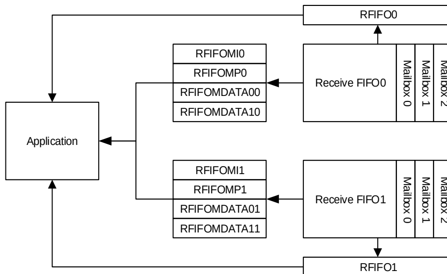
图 26-4. 接收寄存器
