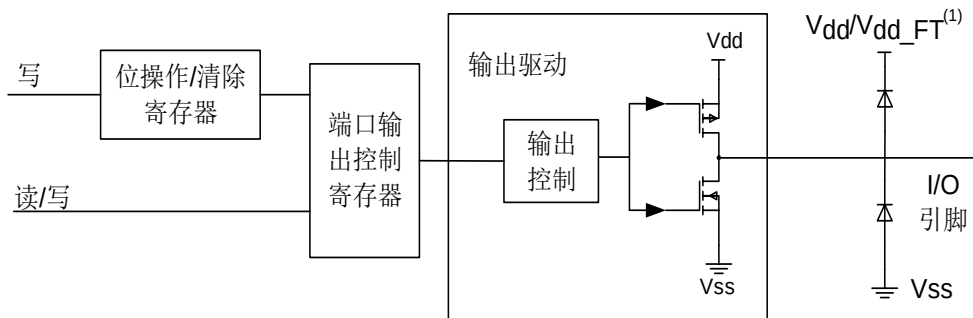
图 7-3. 输出配置
