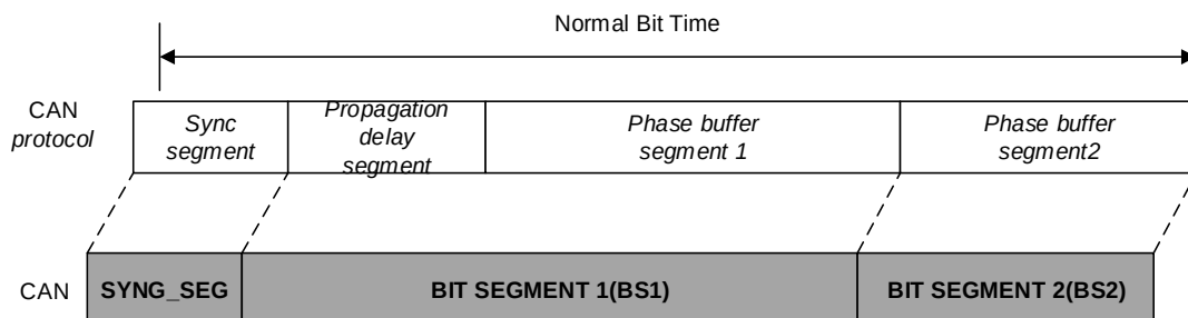
图 26-11. 位时序
