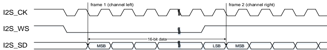
Figure 18-9. I2S Philips standard timing diagram (DTLEN=00, CHLEN=0, CKPL=1)
