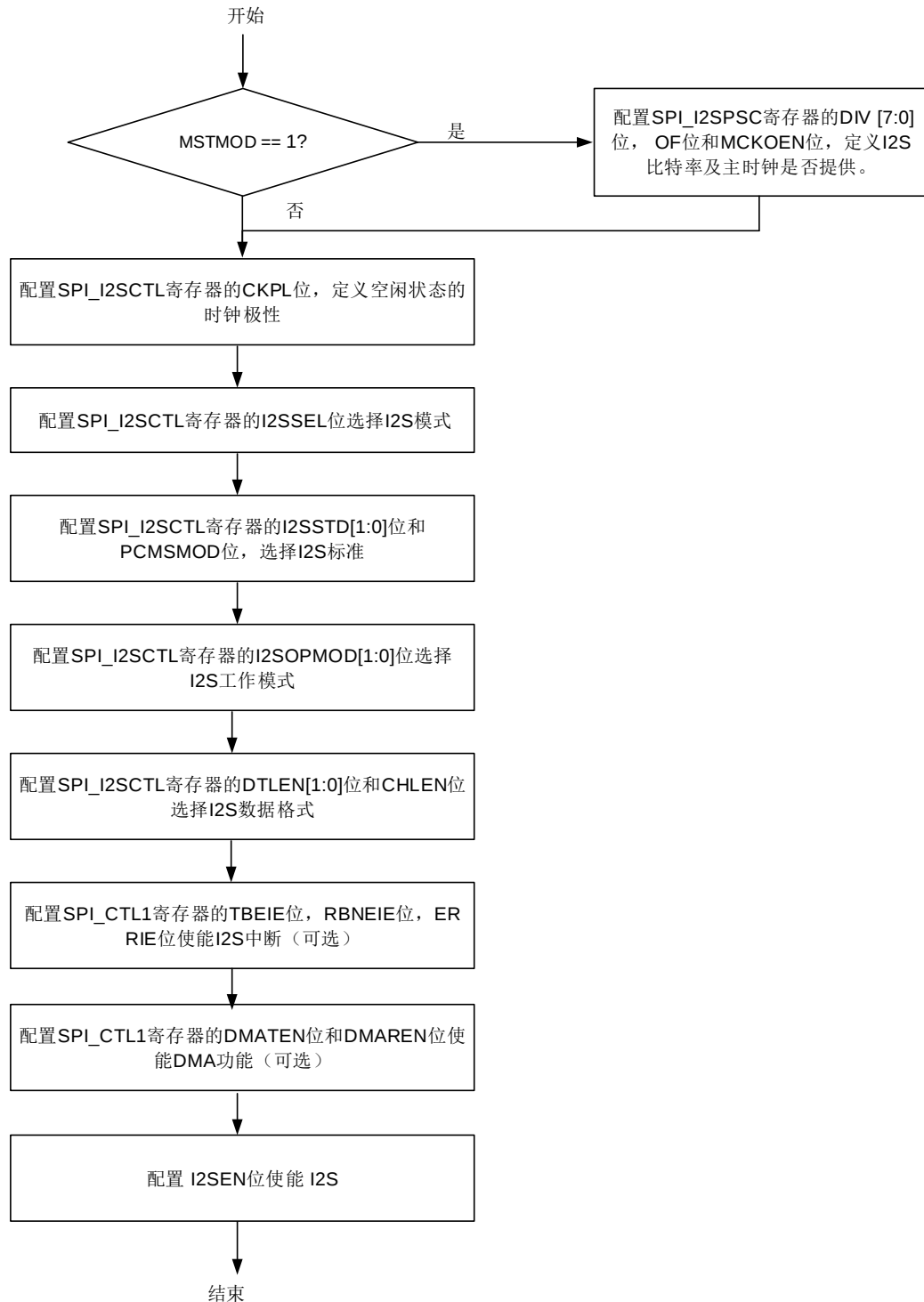
图 21-51. I2S 初始化流程
