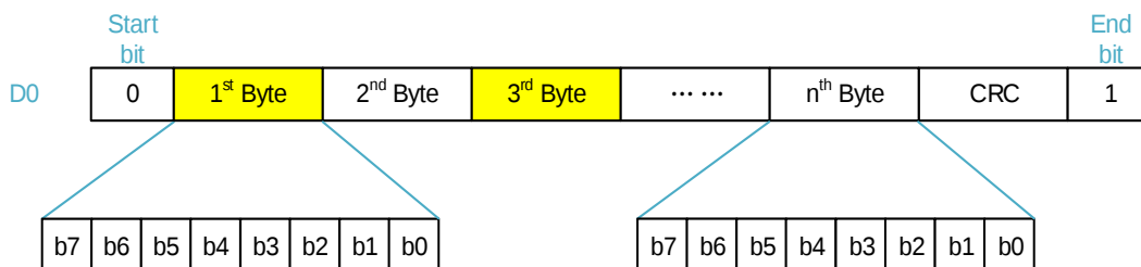
图 24-9. 1 位数据总线宽度
