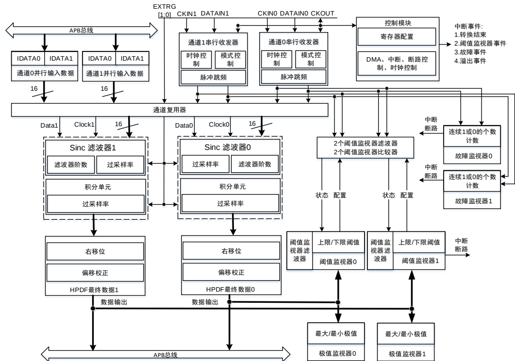
图 31-1. HPDF 结构框图
