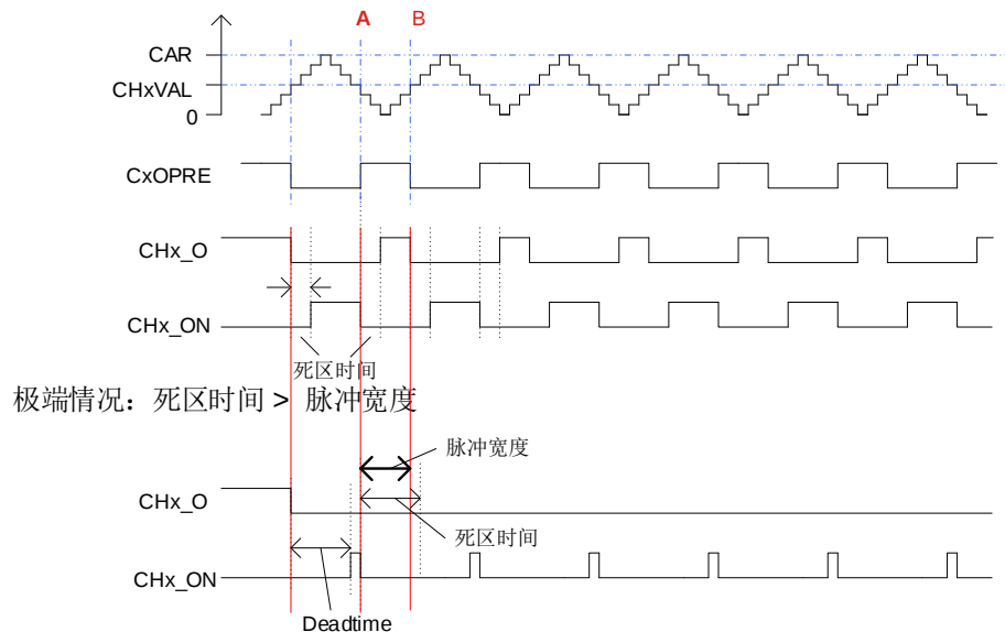
图 18-77. 带死区时间的互补输出
