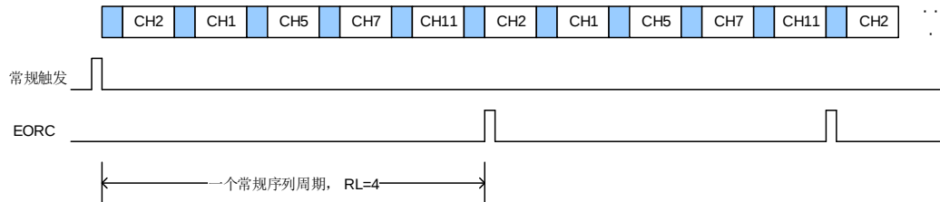
图 15-14. 扫描转换模式，连续转换模式使能
