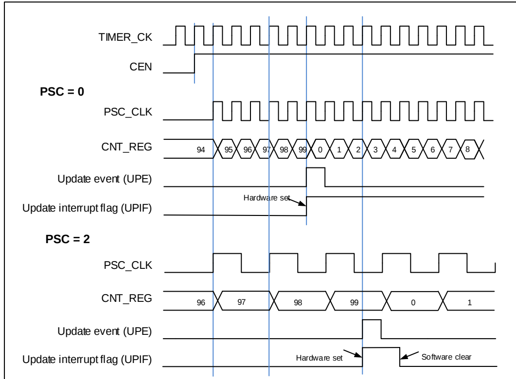
图 18-6. 向上计数时序图, PSC=0/2
