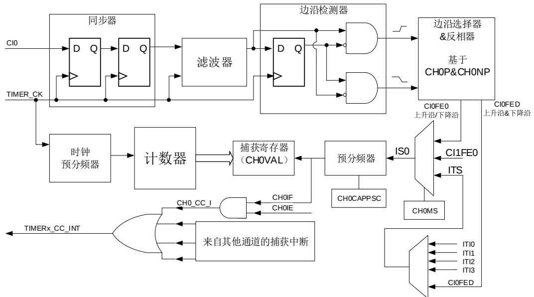
图 18-55. 通道输入捕获原理
