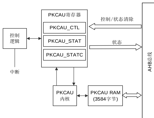
图 30-1. PKCAU 模块框图
