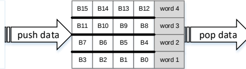
图 14-5. PWIDTH 为‘2b01’时，数据的打包/解包
