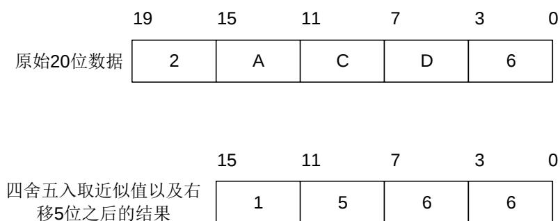
图 15-9. 右移 5 位和取整的数例
