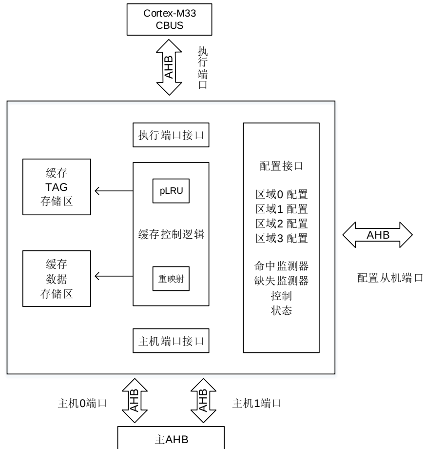
图 4-1. ICACHE 结构框图
