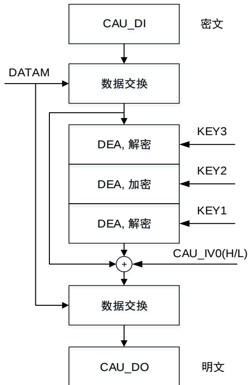
图 28-7. DES / TDES CBC 解密
