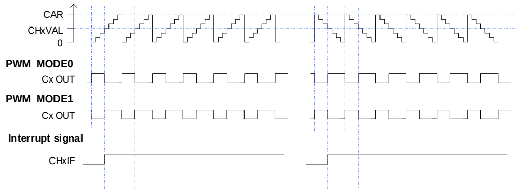
图 18-19. CAPWM 时序图
