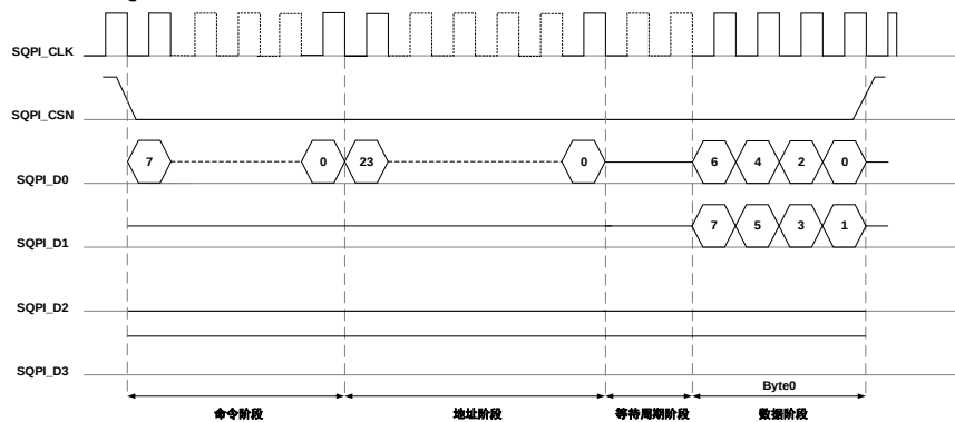
图 22-10. SQPI SDD 模式时序
