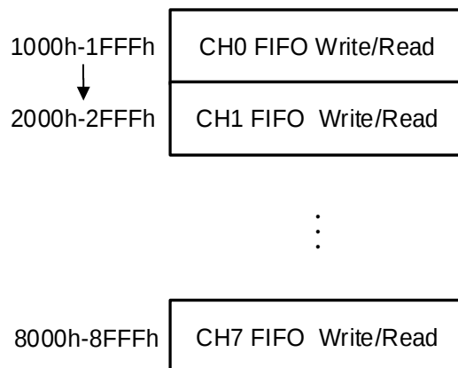
图 25-6. 主机模式 FIFO 访问寄存器映射表
