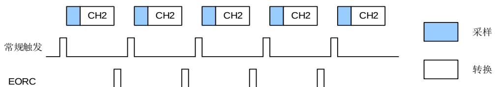
图 15-11. 单次运行模式
