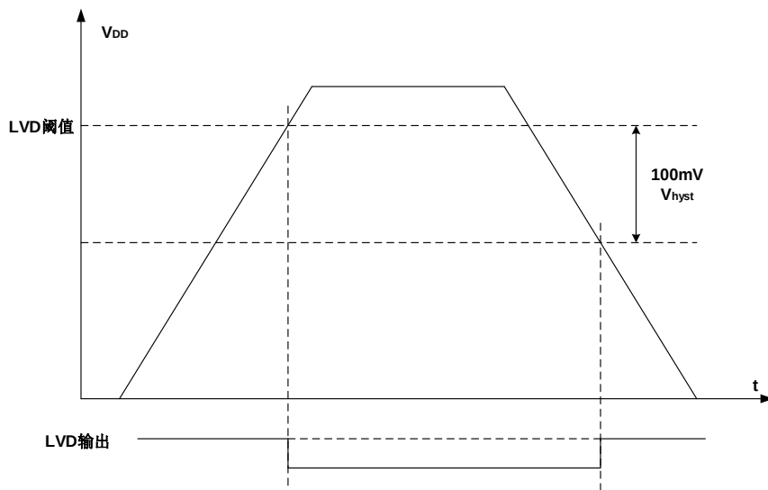
图 5-6. LVD 阈值波形图
