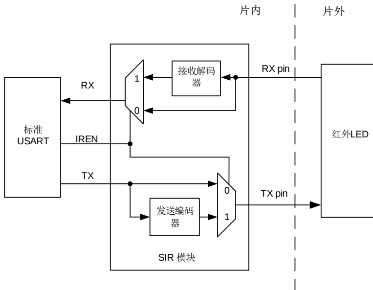
图 19-13. IrDA SIR ENDEC 模块
