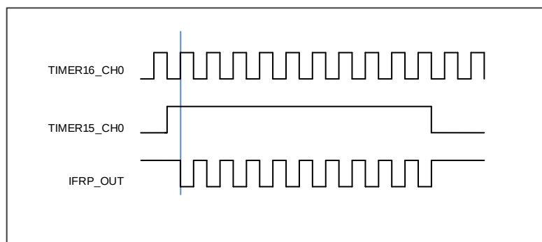
图 32-1. IFRP 输出时序图 1
