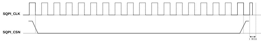
图 22-4. SQPI_CLK 示例
