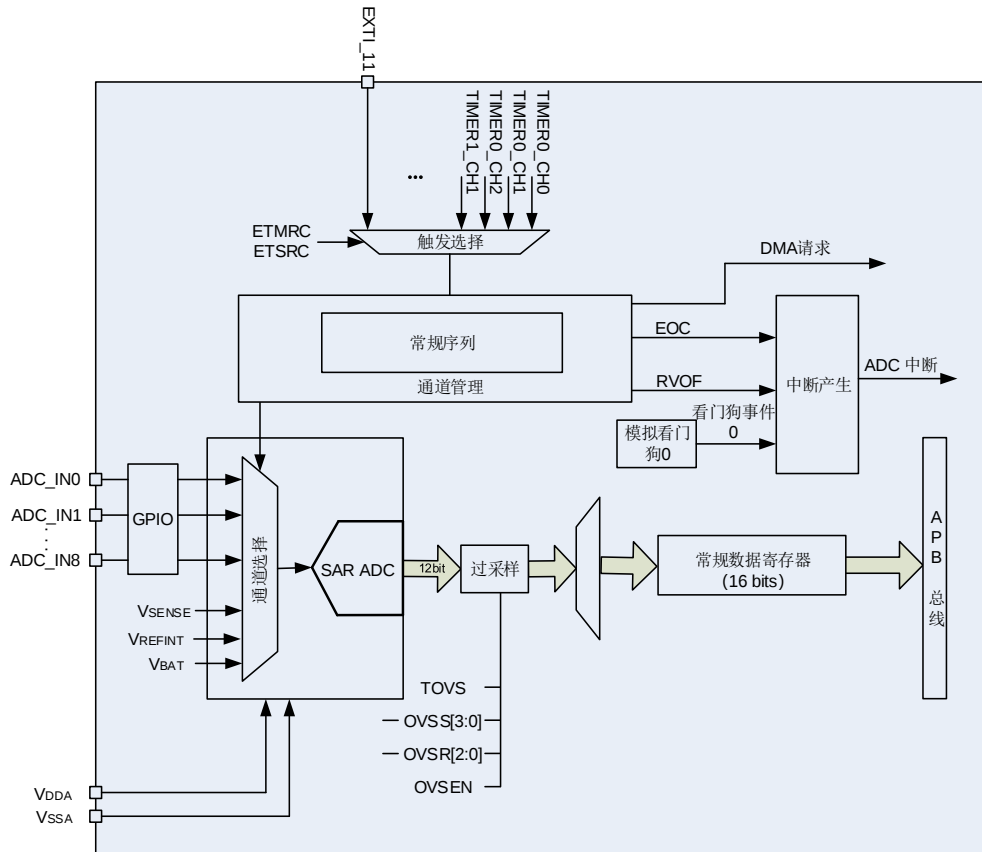
图 15-1. ADC 模块框图
