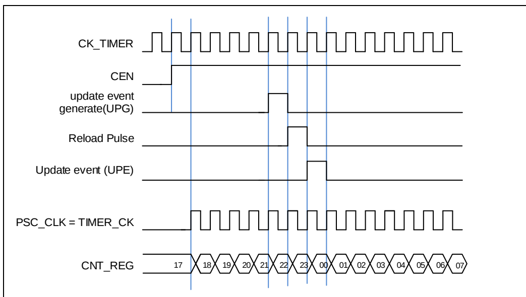
图 18-48. 内部时钟分频为 1 时，计数器的时序图（仅适用于 GD32F5HCxx 系列）
