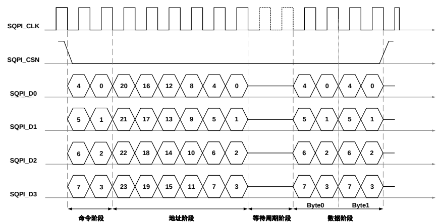
图 22-8. SQPI QQQ 模式时序(QPI)
