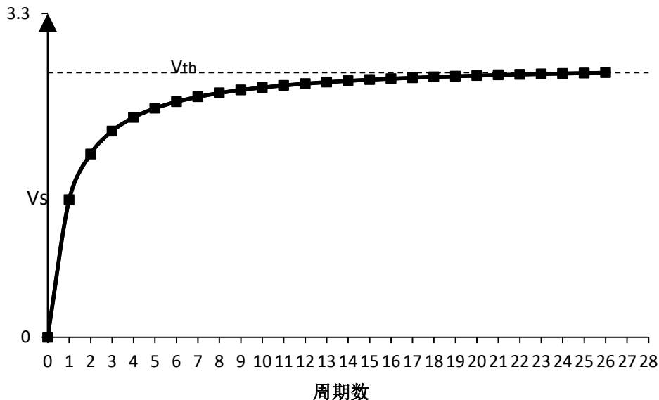
图 27-3. 电荷序列转移期间的采样引脚的电压
