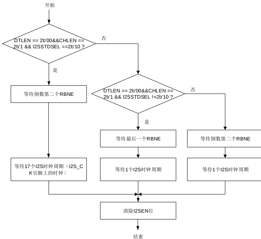
图 21-52. I2S 主机接收禁能流程
