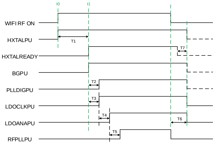
图 5-7. RF 时序
