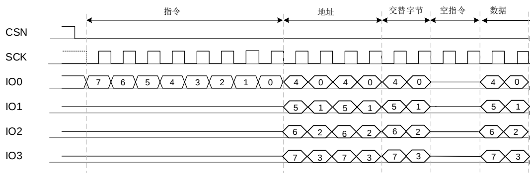
图 23-2. QSPI 命令格式
