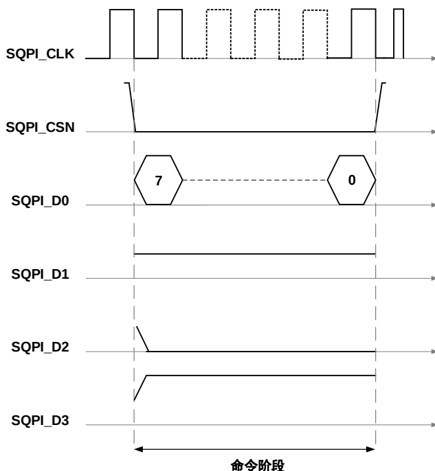
图 22-2. SQPI 特殊命令
