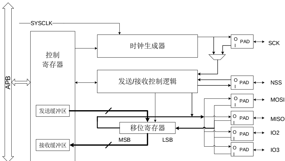
图 21-1. SPI 结构框图
