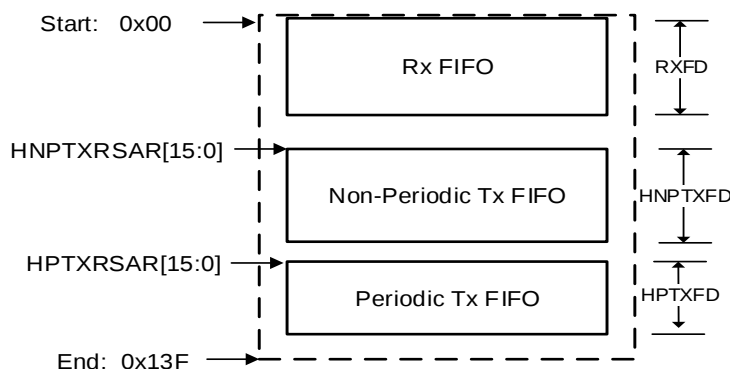
图 25-5. 主机模式 FIFO 空间
