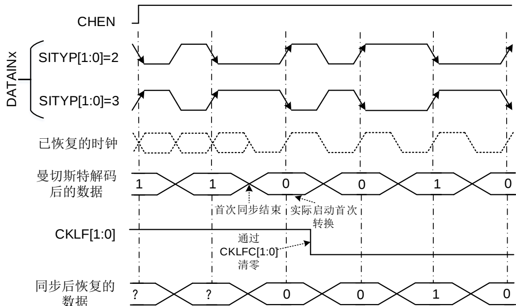
图 31-4. 曼切斯特同步时序图
