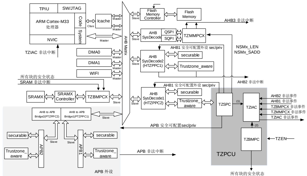
图 10-1. TZPCU 框图
