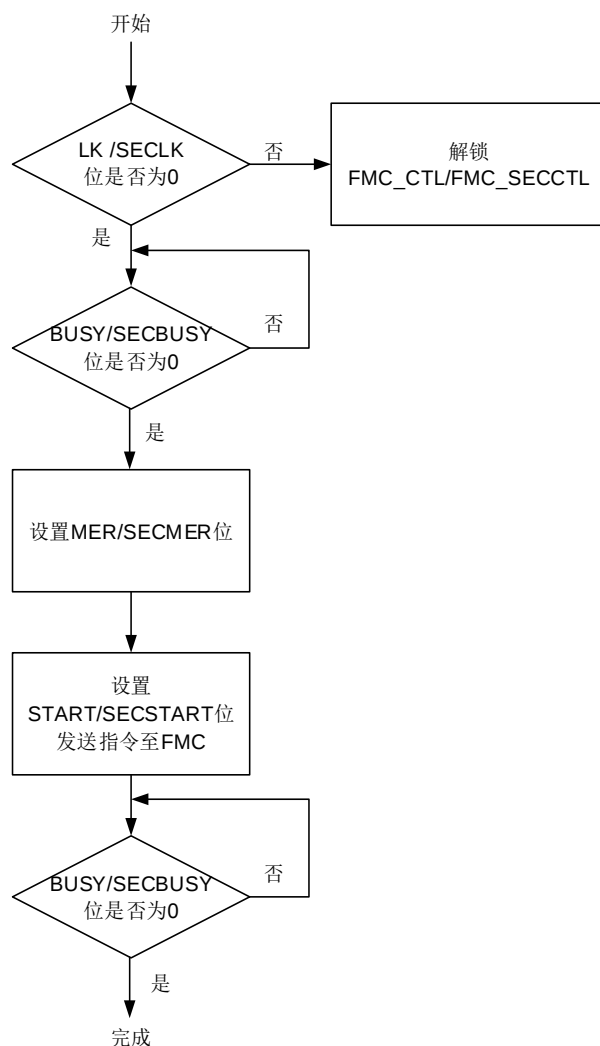
图 2-3. 整片擦除操作流程
