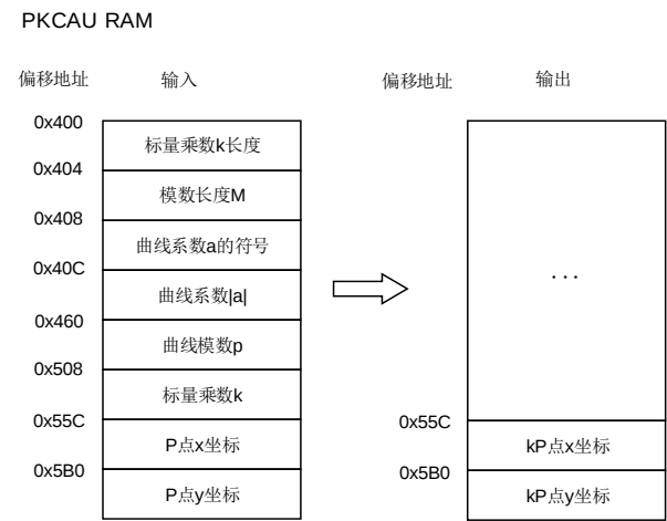
图 30-20. 普通模式 ECC 标量乘法
