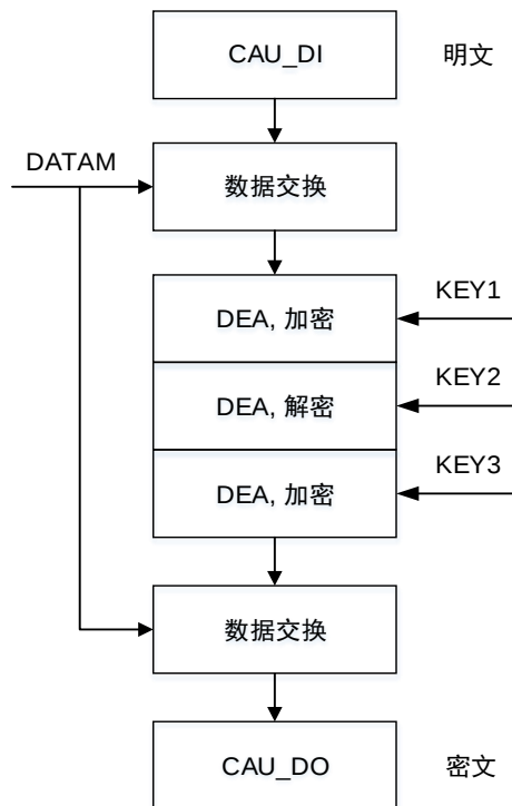
图 28-4. DES / TDES ECB 加密
