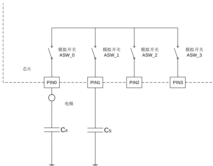
图 27-2. 通道引脚与采样引脚的框图
