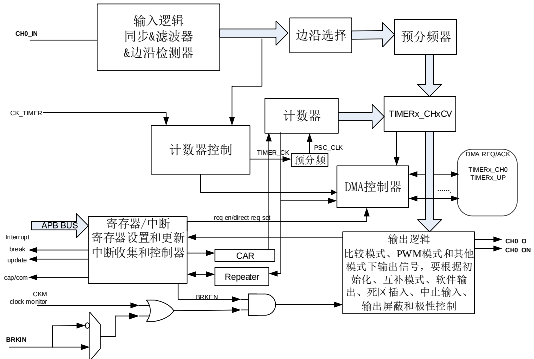
图 18-67. 通用定时器 L4 结构框图
