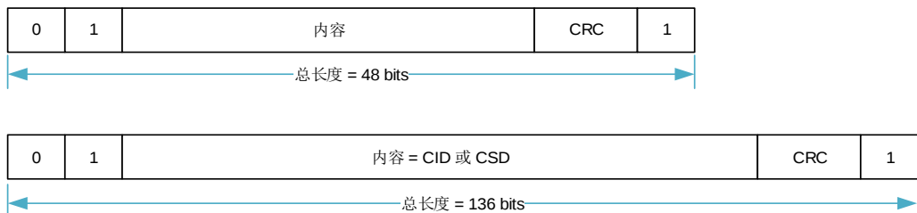
图 24-8. 响应令牌格式
