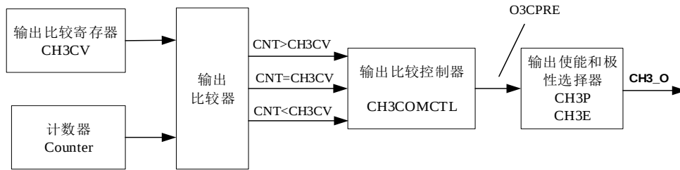
图 18-16. 通道输出比较原理
