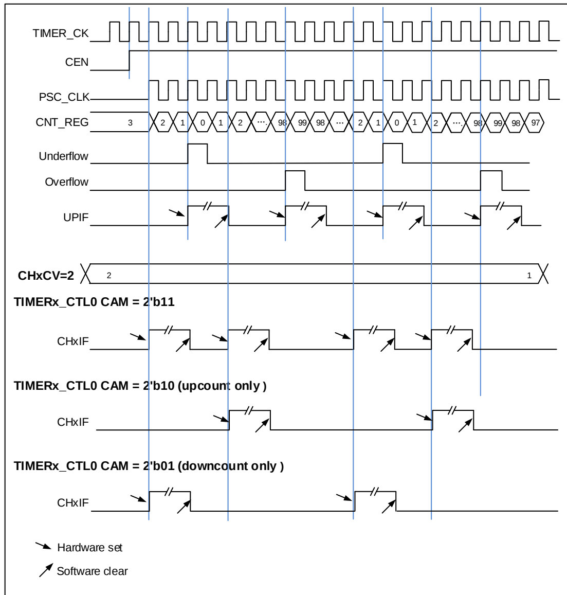
图 18-10. 中央计数模式计数器时序图
