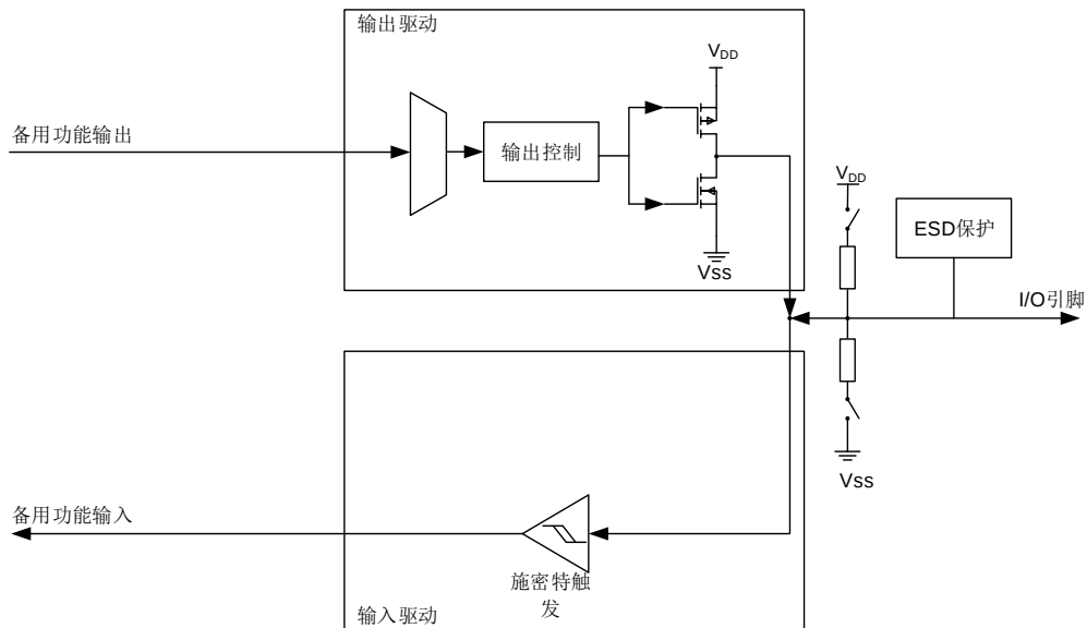
图 9-5. 备用功能配置的基本结构
