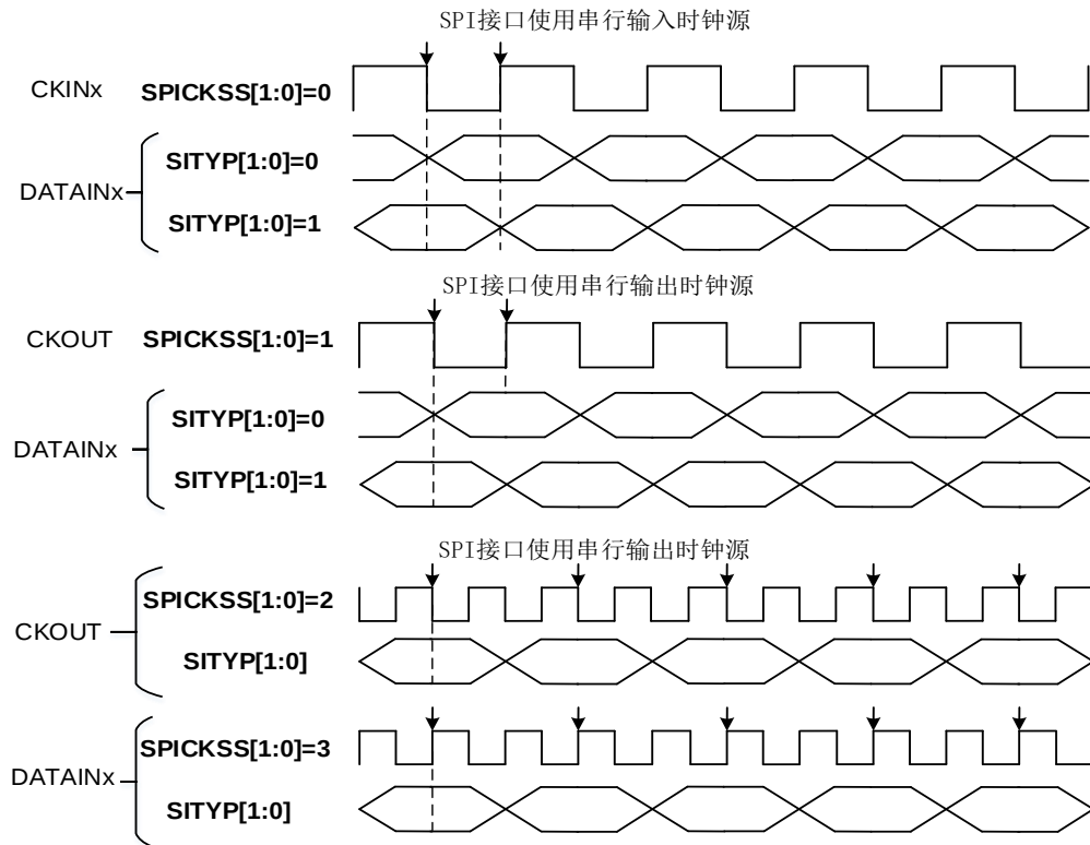
图 31-2. SPI 数据传输时序图
