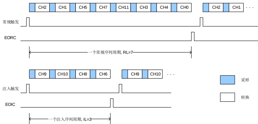
图 15-13. 扫描运行模式，且连续转换模式禁能
