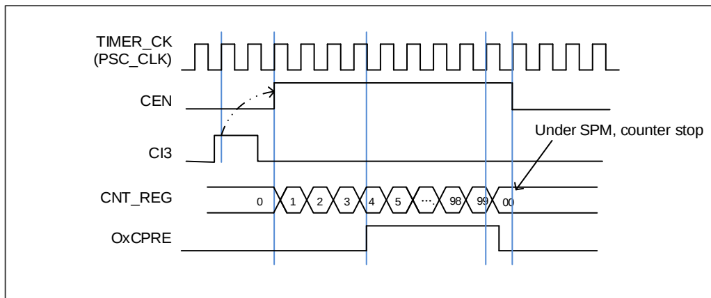
图 18-66. 单脉冲模式，TIMERx_CHxCV = 4 TIMERx_CAR=99
