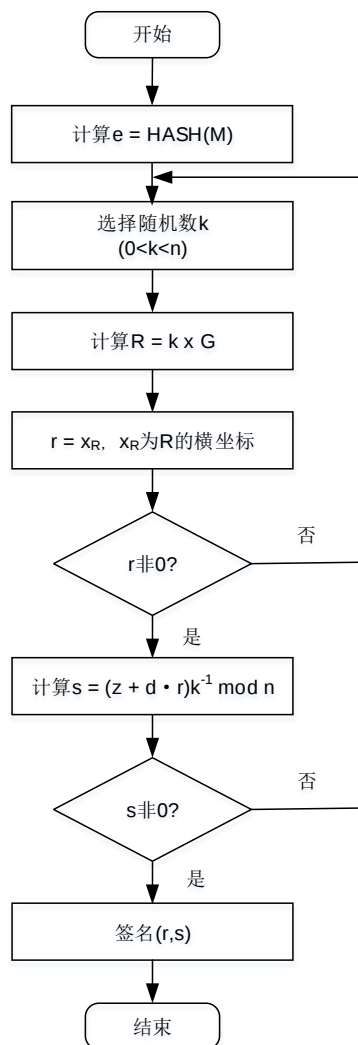
图 30-3. ECDSA 签名流程图
