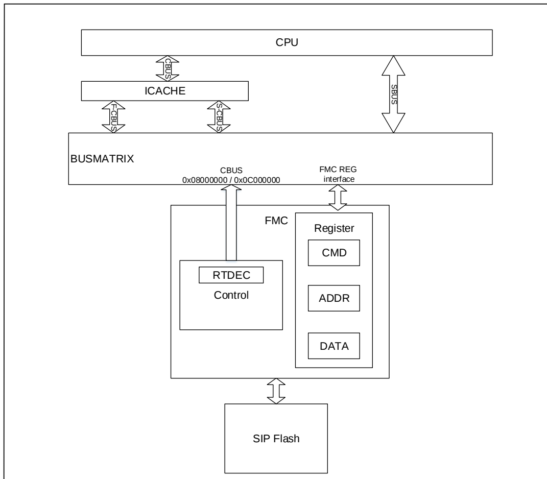
图 2-1. GD32W51x_F5HC FMC 总线
