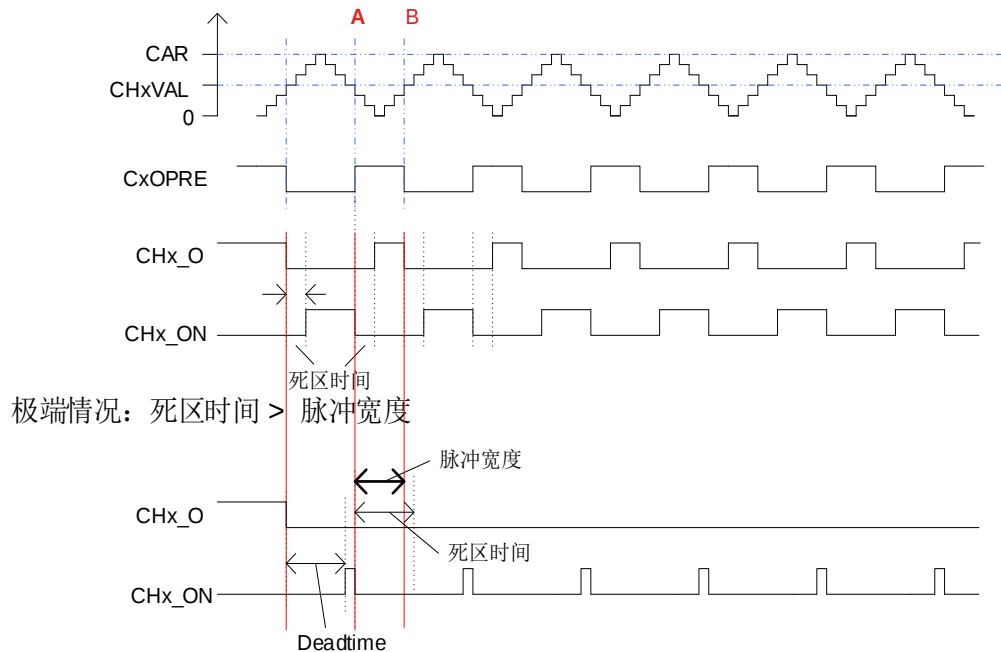
图 18-20. 带死区时间的互补输出
