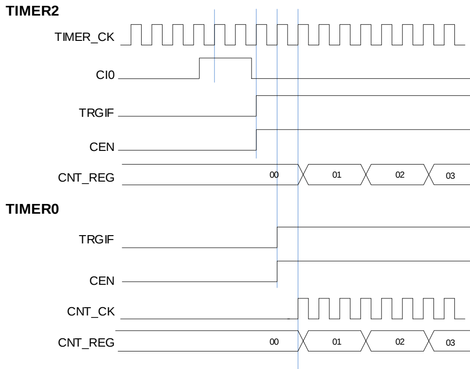
图 18-38. 用定时器 2 的 CI0 信号来触发定时器 0 和定时器 2（仅适用于 GD32W515xx 系列）
