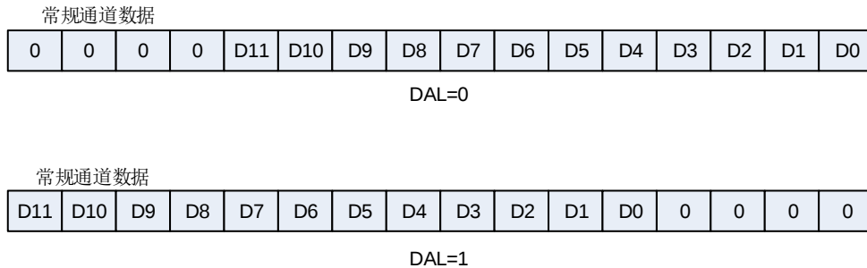
图 15-7. 12 位数据存储
