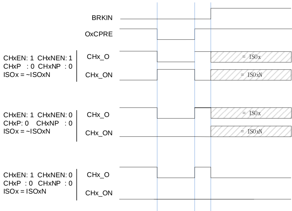
图 18-78. 通道响应中止输入（高电平有效）时，输出信号的行为
