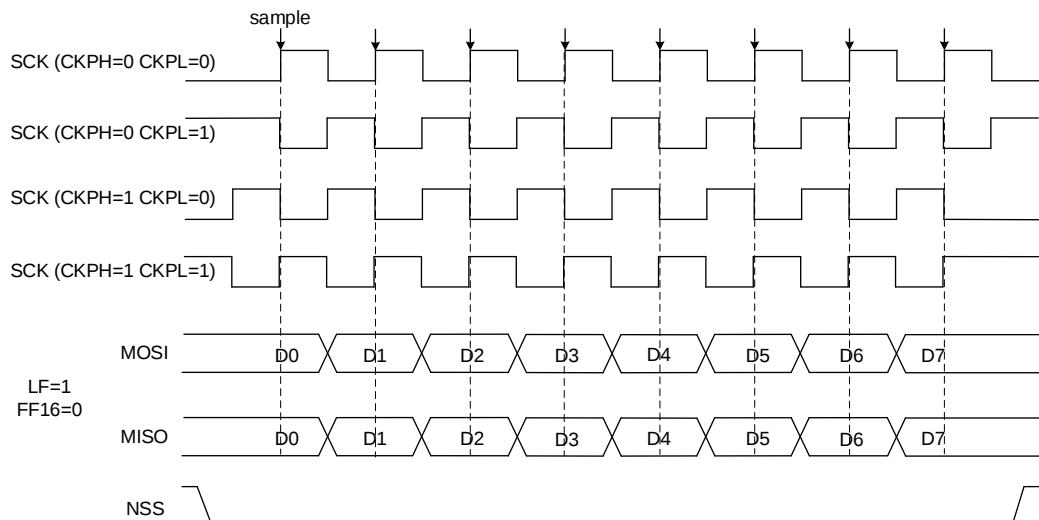
图 21-2. 常规模式下的 SPI 时序图
