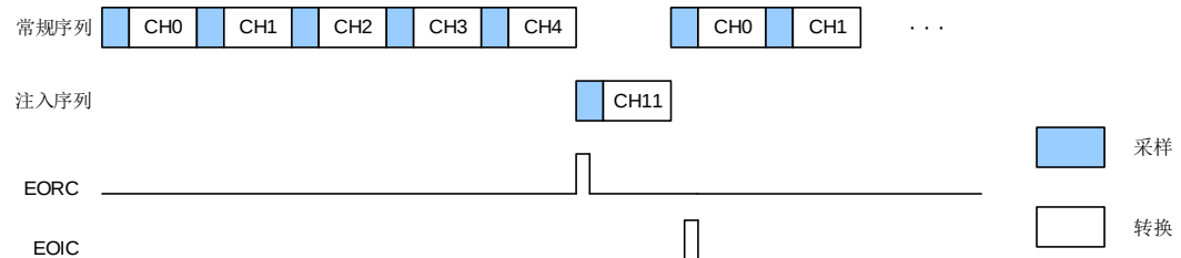
图 15-16. 自动注入，CNT=1
