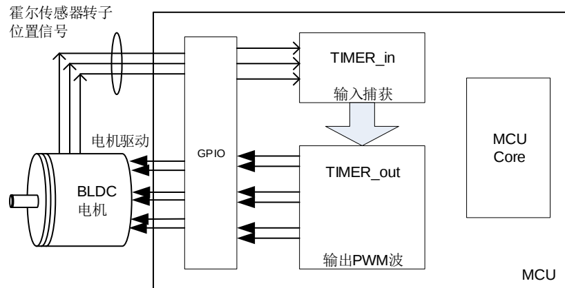
图 18-24. 霍尔传感器用在 BLDC 电机控制中
