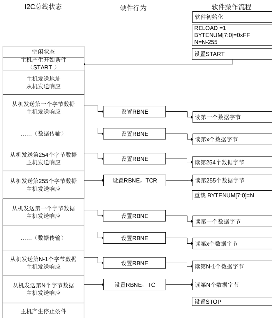
图 20-21. I2C 主机接收编程模型 (N&gt;255)
