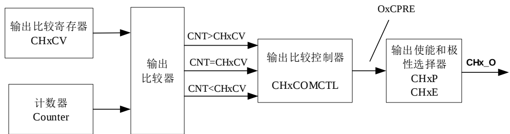
图 18-56. 通道输出比较原理 (x=0,1,2,3)
