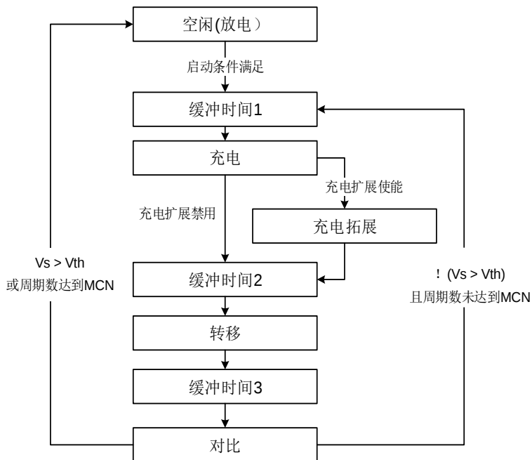
图 27-4. 电荷转移序列的有限状态机的状态转移图
