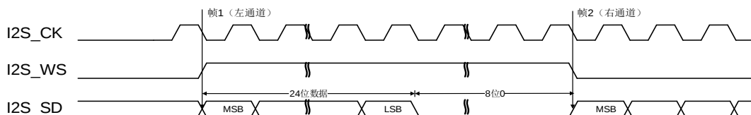
图 21-26. MSB 对齐标准时序图 (DTLEN=01, CHLEN=1, CKPL=0)
