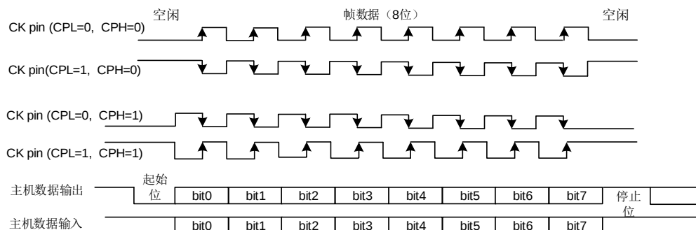
图 19-12. 8-bit 格式的 USART 同步通信波形（CLEN=1）
