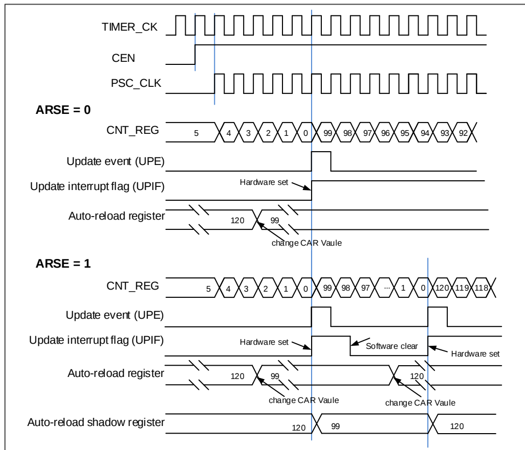
图 18-53. 向下计数时序图, 在运行时改变 TIMERx_CAR 寄存器值
