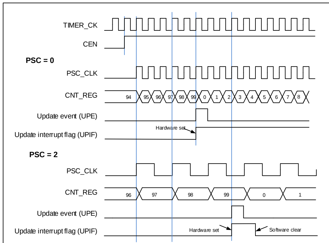
图 18-83. 向上计数时序图，PSC=0/2
