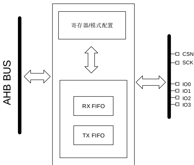
图 23-1. QSPI 结构框图
