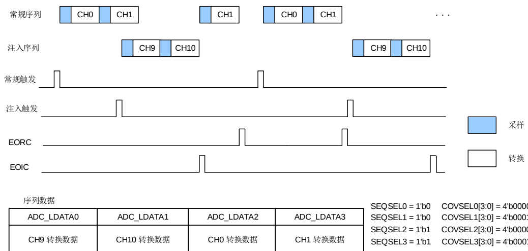
图 15-19. ADC_LDATAB x 读取序列数据
