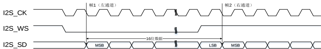
图 21-15. I2S 飞利浦标准时序图 (DTLEN=00, CHLEN=0, CKPL=1)
