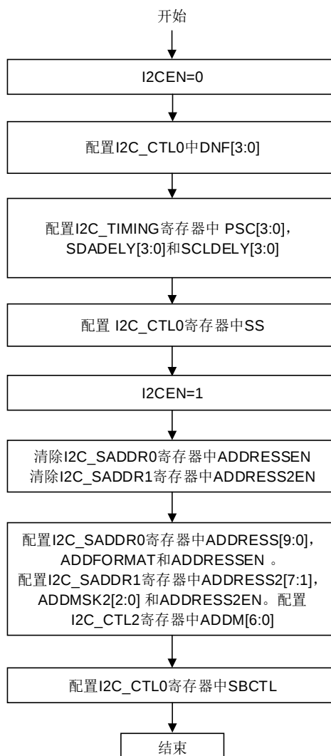
图 20-13. I2C 从机初始化
