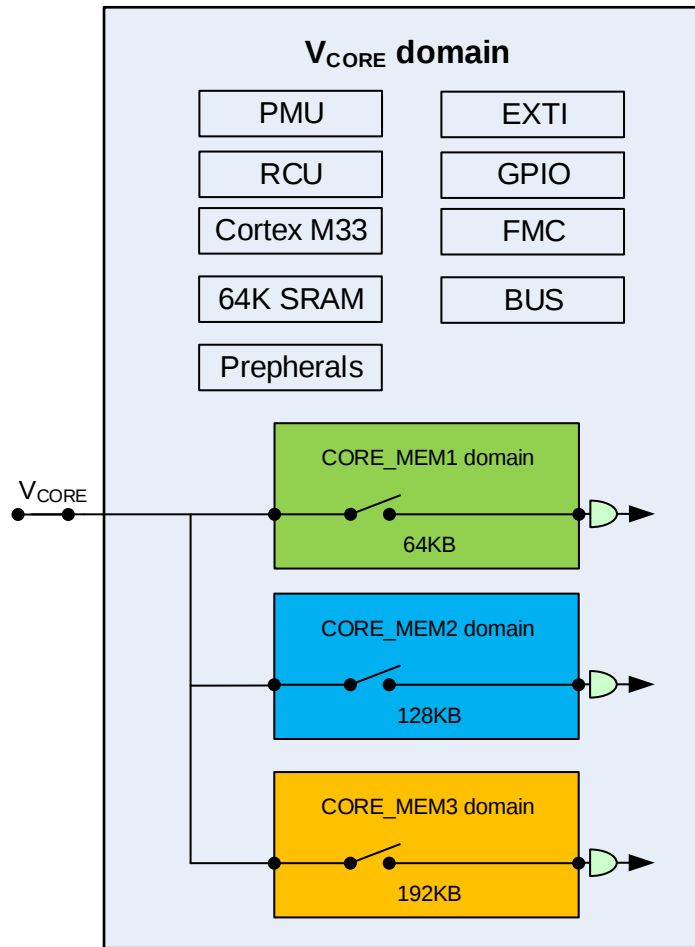
图 5-4. V CORE 电源域概览（适用于 GD32F5HCxx 系列）
