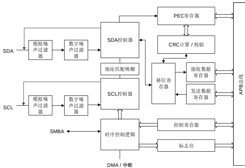
图 20-1. I2C 模块框图
