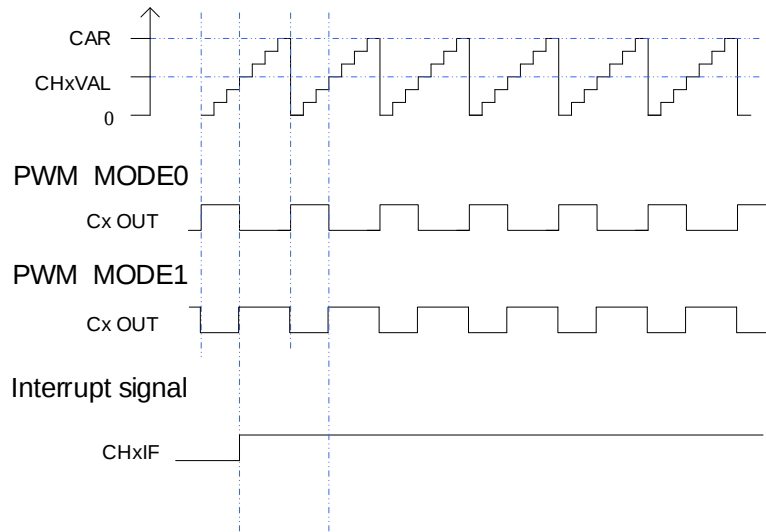
图 18-76. PWM 时序图
