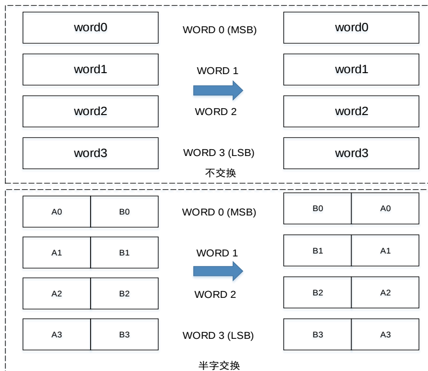
图 29-1. DATAM 不交换/半字交换
