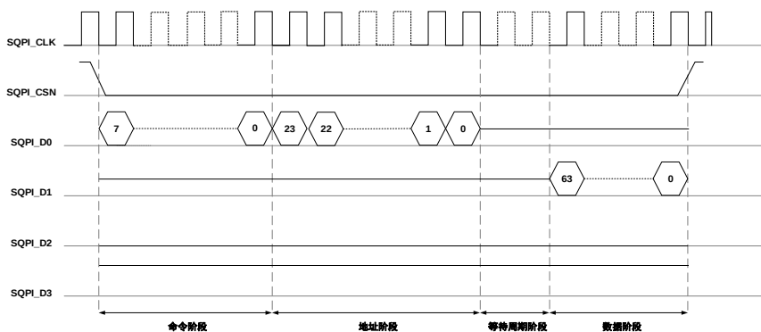
图 22-3. SQPI 读 ID (IDLEN=00)
