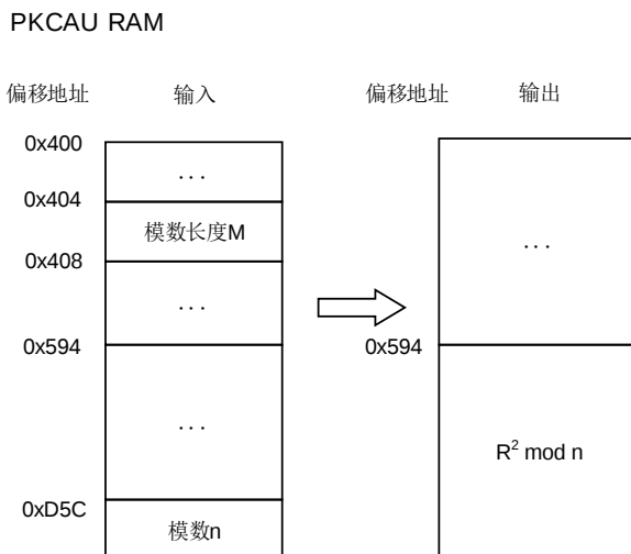
图 30-12. 蒙哥马利参数计算
