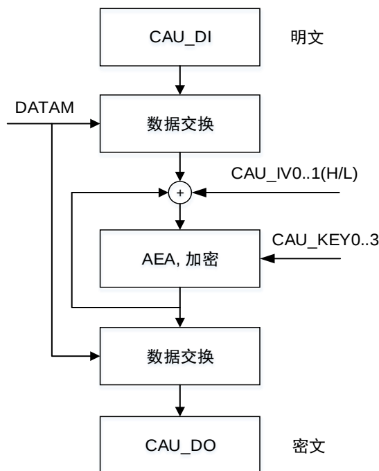
图 28-10. AES CBC 加密
