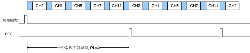
图 15-5. 扫描运行模式，连续运行模式使能
