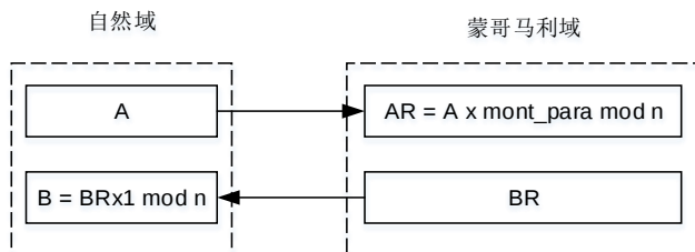
图 30-13. 蒙哥马利域和自然域之间的相互映射
