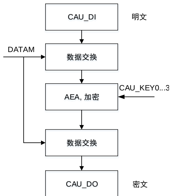
图 28-8. AES ECB 加密
