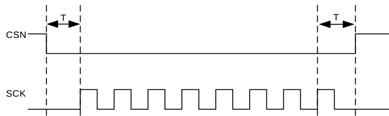
图 23-3. CSN 和 SCK 的行为
