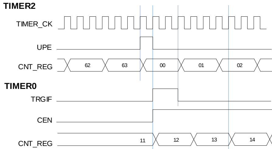
图 18-41. 用定时器 2 的更新事件来触发定时器 0（仅适用于 GD32F5HCxx 系列）
