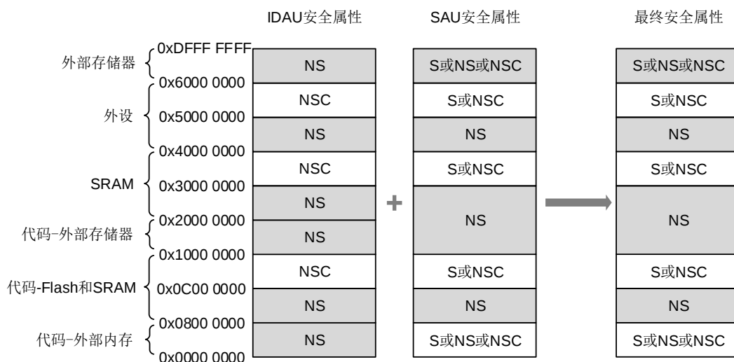
图 1-4. 内存映射安全属性与 SAU 配置区域的示例
