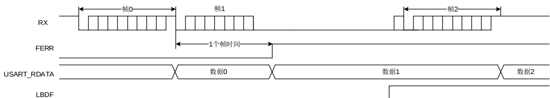
图 19-10. 数据传输过程中检测断开帧
