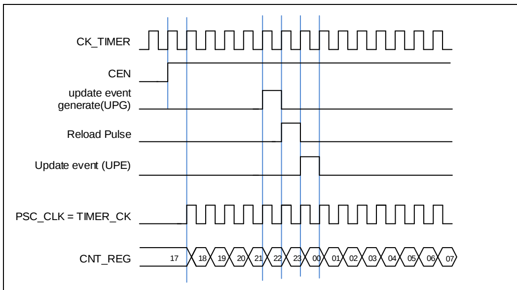
图 18-47. 内部时钟分频为 1 时，计数器的时序图（仅适用于 GD32W515xx 系列）
