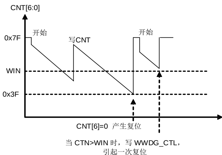
图 16-3. 窗口看门狗定时器时序图
