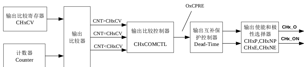
图 18-15. 通道输出比较原理（带有互补输出的通道， x=0,1,2 ）
