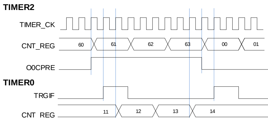
图 18-37. 用定时器 2 的 O0CPRE 信号控制定时器 0 的暂停模式（仅适用于 GD32W515xx 系列）
