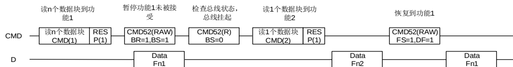
图 24-14. 在功能 1 的多块读周期期间插入功能 2 读周期
