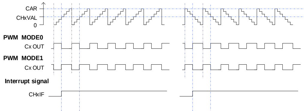
图 18-59. CAPWM 时序图
