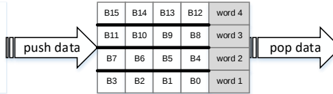
图 14-4. PWIDTH 为‘2b00’时，数据的打包/解包
