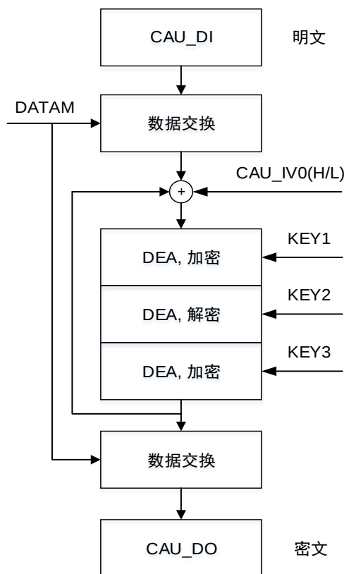
图 28-6. DES / TDES CBC 加密
