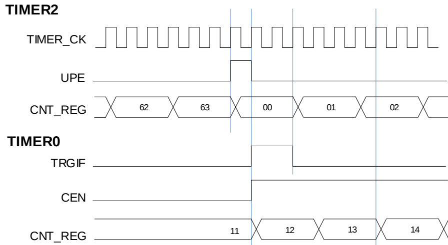
图 18-35. 用定时器 2 的更新事件来触发定时器 0（仅适用于 GD32W515xx 系列）
