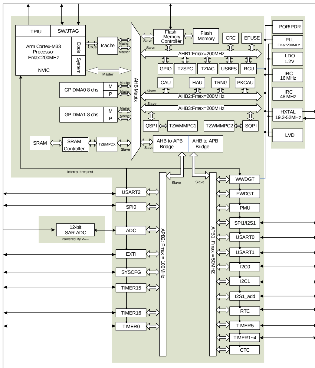
图 1-2. GD32F5HCxx 系列器件的系统架构示意图
