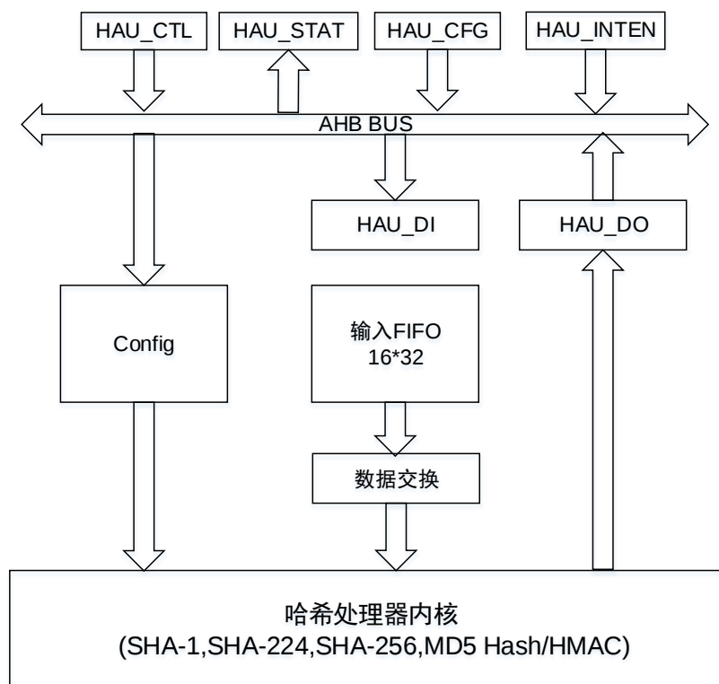
图 29-3. HAU 结构框图
