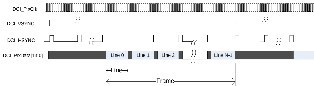
图 26-2. 硬件同步模式
