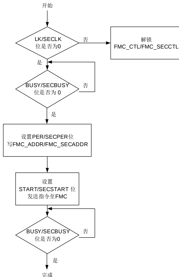
图 2-2. 页擦除操作流程
