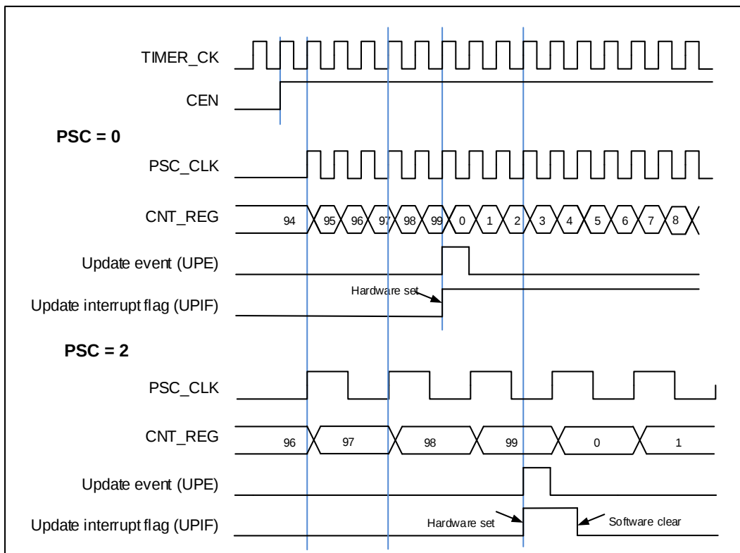
图 18-70. 向上计数时序图，PSC=0/2
