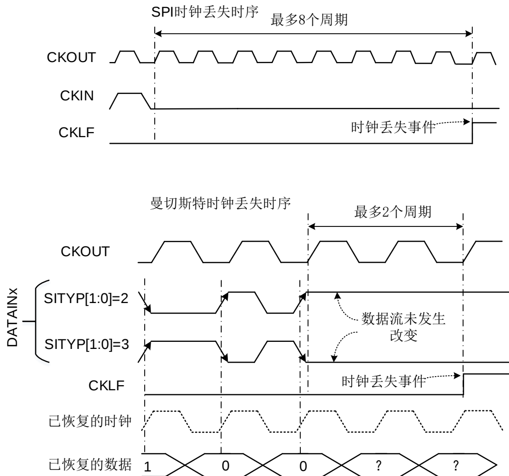
图 31-5. 时钟丢失检测时序图
