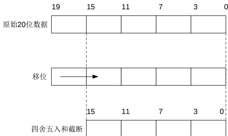
图 15-8. 20 位到 16 位的结果截断
