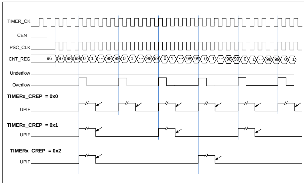
图 18-72. 在向上计数模式下计数器重复时序图
