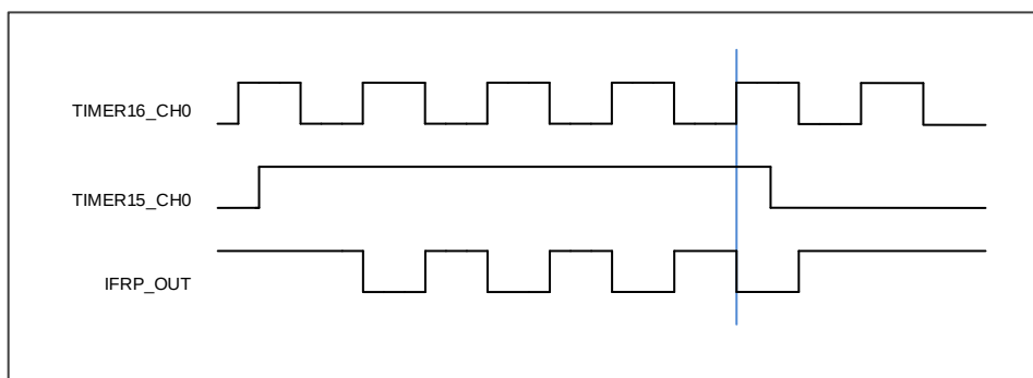
图 32-3. IFRP 输出时序图 2
