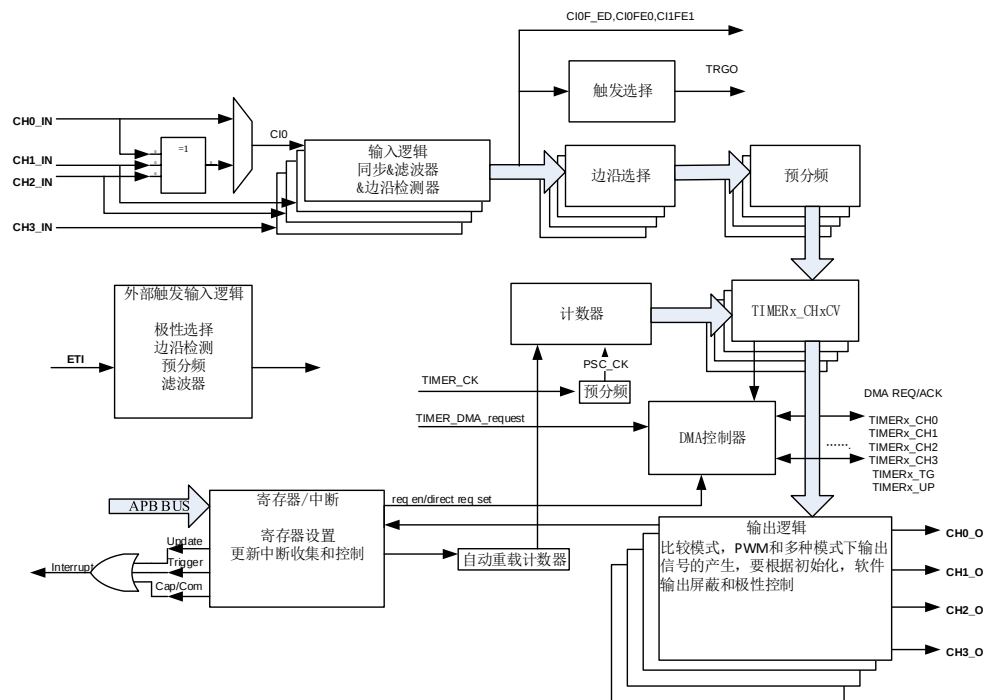
图 18-46. 通用定时器 L0 结构框图（仅适用于 GD32F5HCxx 系列）
