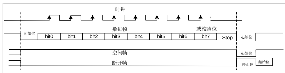
图 19-2. USART 字符帧 (8 数据位和 1 停止位)
