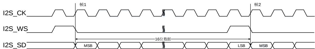
图 21-34. PCM 标准短帧同步模式时序图 (DTLEN=00, CHLEN=0, CKPL=0)
