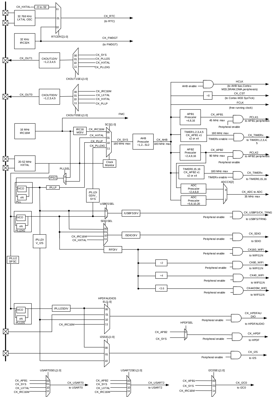
图 6-2. 时钟树 (适用于 GD32W515xx 系列)
