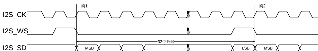
图 21-37. PCM 标准短帧同步模式时序图 (DTLEN=10, CHLEN=1, CKPL=1)
