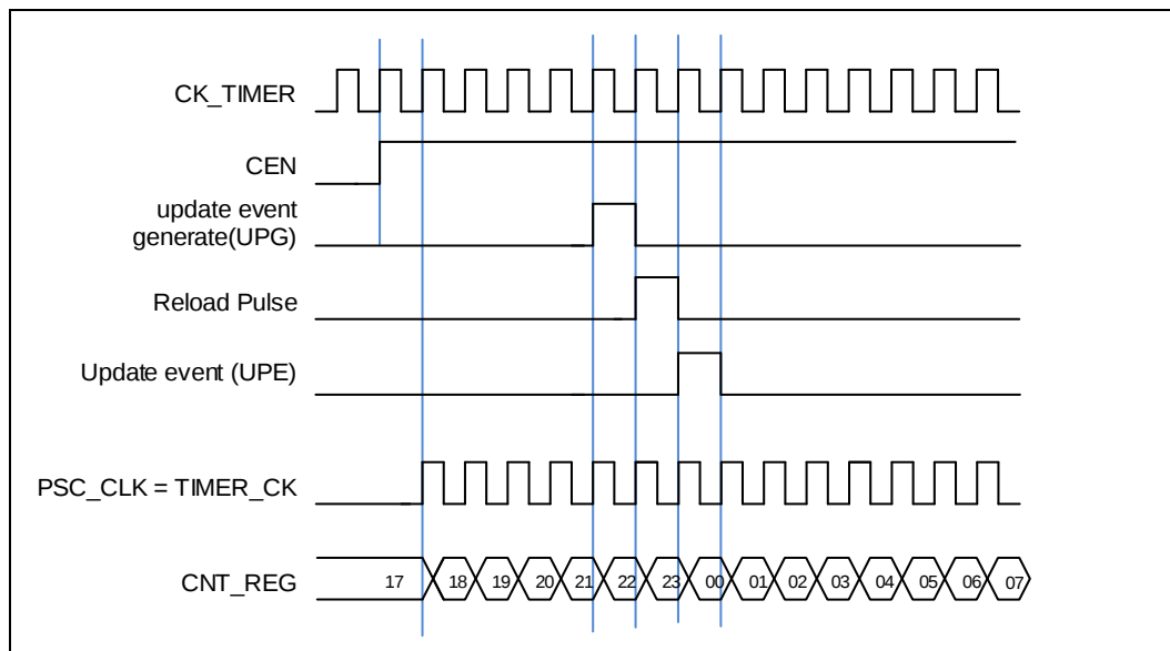
图 18-3. 内部时钟分频为 1 时，计数器的时序图（仅适用于 GD32W515xx 系列）
