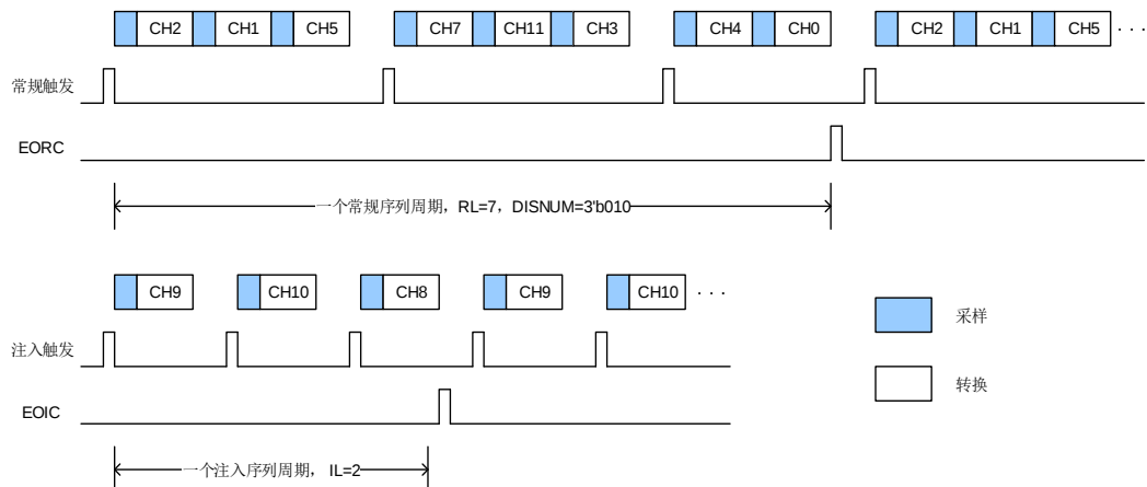
图 15-15. 中断运行模式
