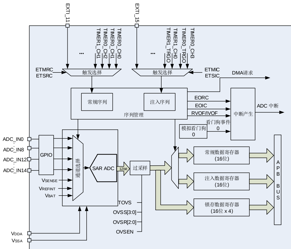
图 15-10. ADC 模块框图
