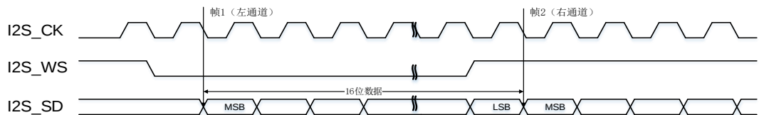
图 21-14. I2S 飞利浦标准时序图 (DTLEN=00, CHLEN=0, CKPL=0)
