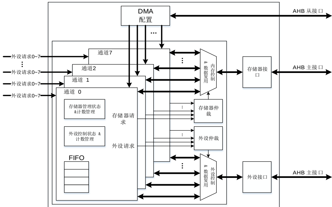
图 14-1. 系统架构
