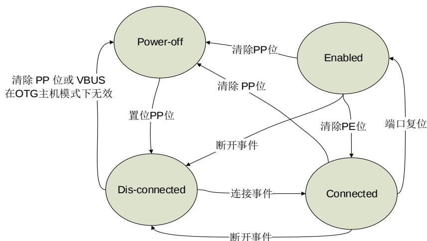
图 25-4. 主机端口状态转移图
