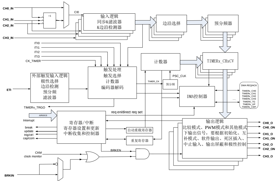
图 18-1. 高级定时器结构框图（仅适用于 GD32W515xx 系列）
