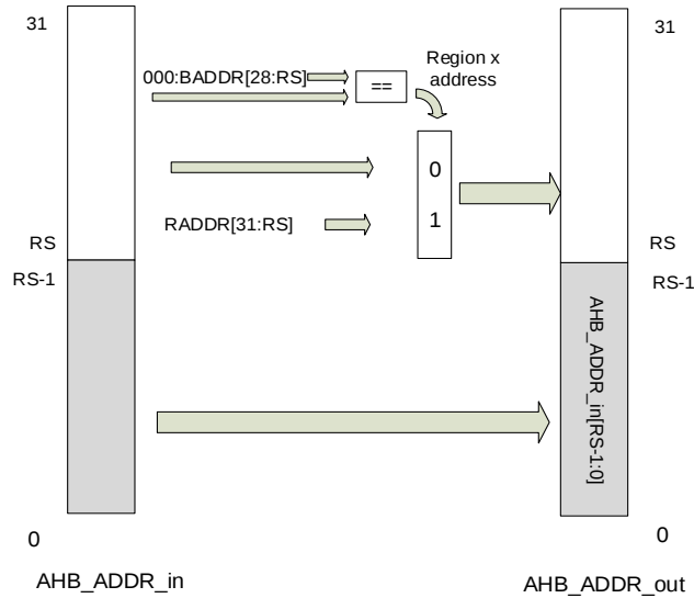
图 4-2. ICACHE 重映射区域大小
