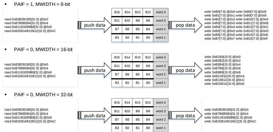
图 14-6. PWIDTH 为‘2b10’时，数据的打包/解包
