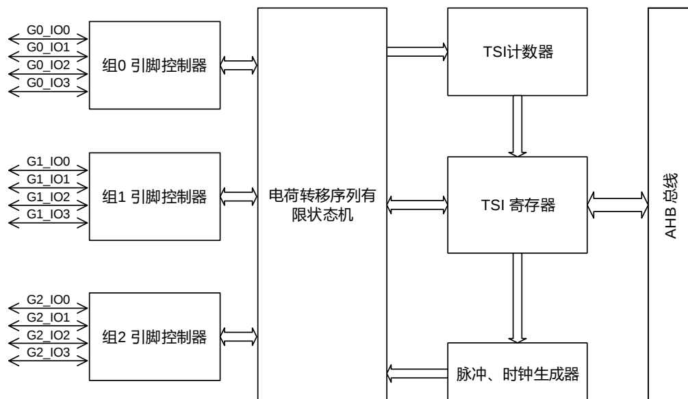
图 27-1. TSI 模块框图
