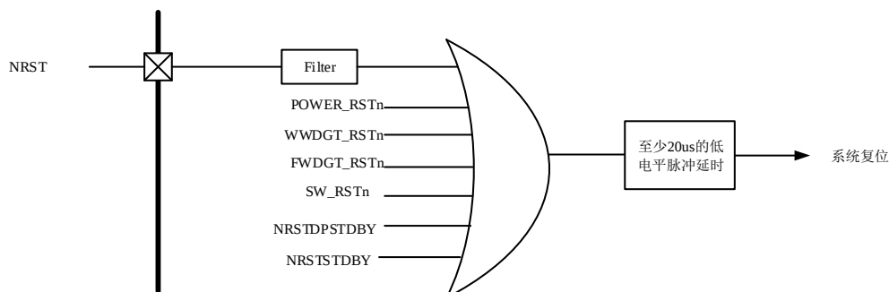
图 6-1.系统复位电路
