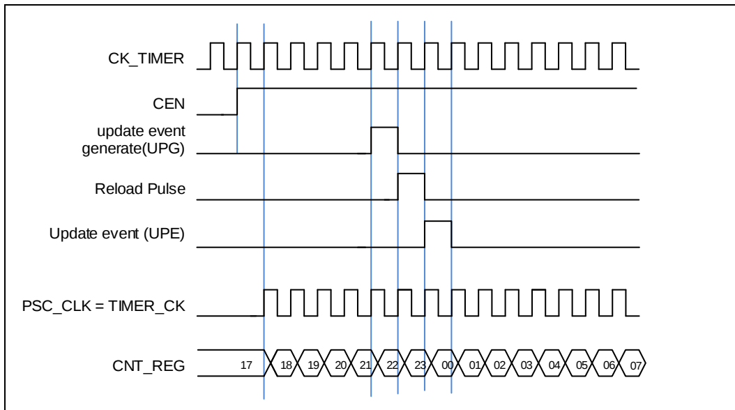
图 18-68. 内部时钟分频为 1 时，计数器的时序图
