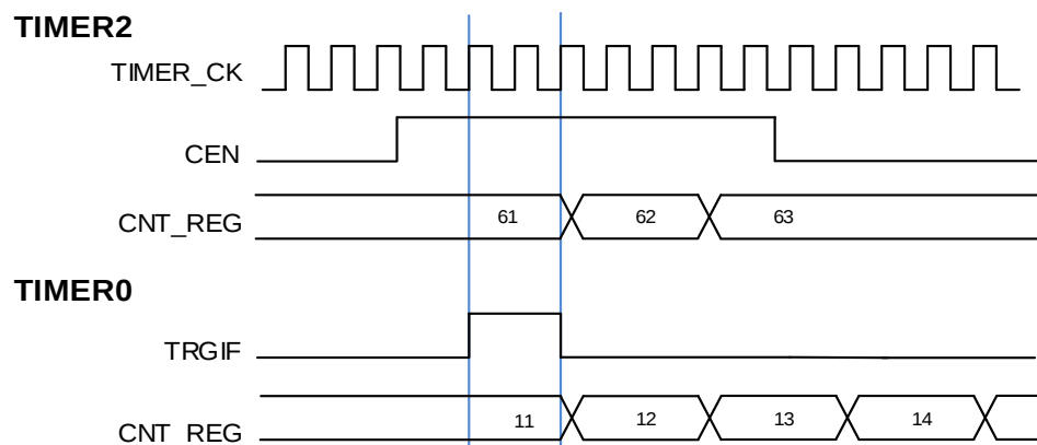
图 18-34. 用定时器 2 的使能信号触发定时器 0（仅适用于 GD32W515xx 系列）
