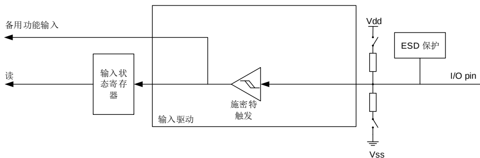
图 9-2. 输入配置的基本结构
