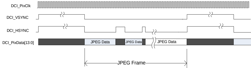
图 26-3. 硬件同步模式之 JPEG 格式
