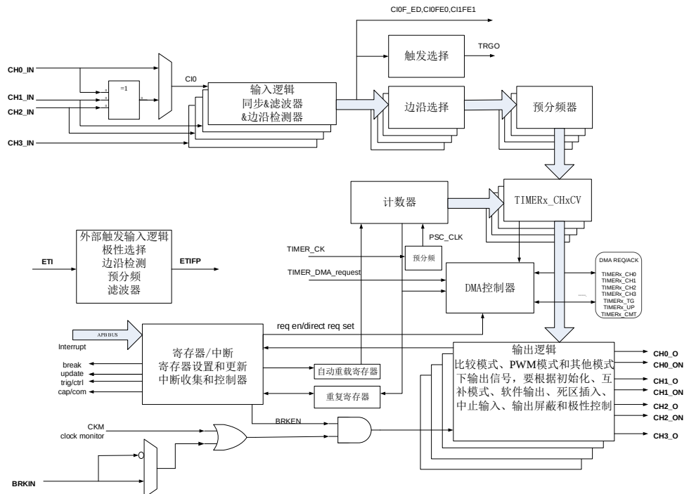
图 18-2. 高级定时器结构框图（仅适用于 GD32F5HCxx 系列）
