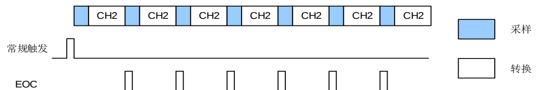
图 15-3. 连续运行模式
