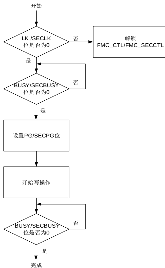
图 2-4. 字编程操作流程
