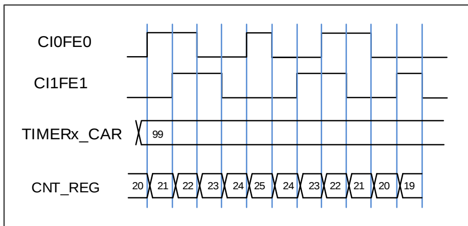
图 18-23.在编码器模式 2 且 CI0FE0 极性反相时计数器行为
