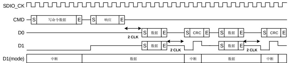
图 24-18. 4 位模式下多块写中断周期时序
