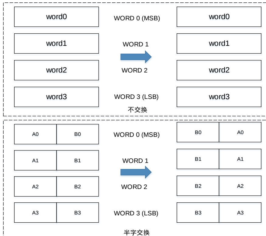
图 28-1. DATAM 不交换/半字交换
