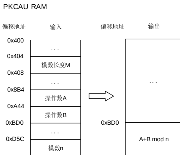
图 30-10. 模加法
