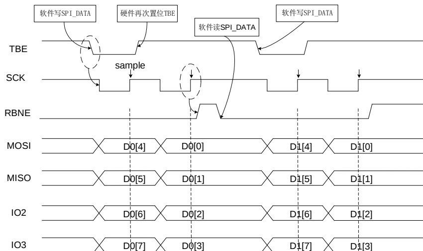
图 21-12. 四线模式读操作时序图
