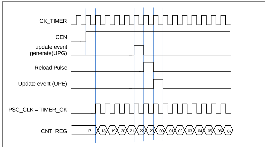
图 18-81. 内部时钟分频为 1 时，计数器的时序图
