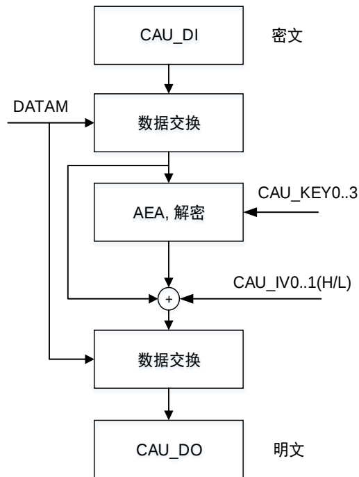
图 28-11. AES CBC 解密
