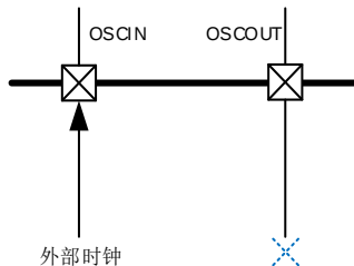
图 6-5. 旁路模式下 HXTAL 时钟源
