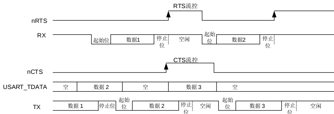
图 19-8. 硬件流控制
