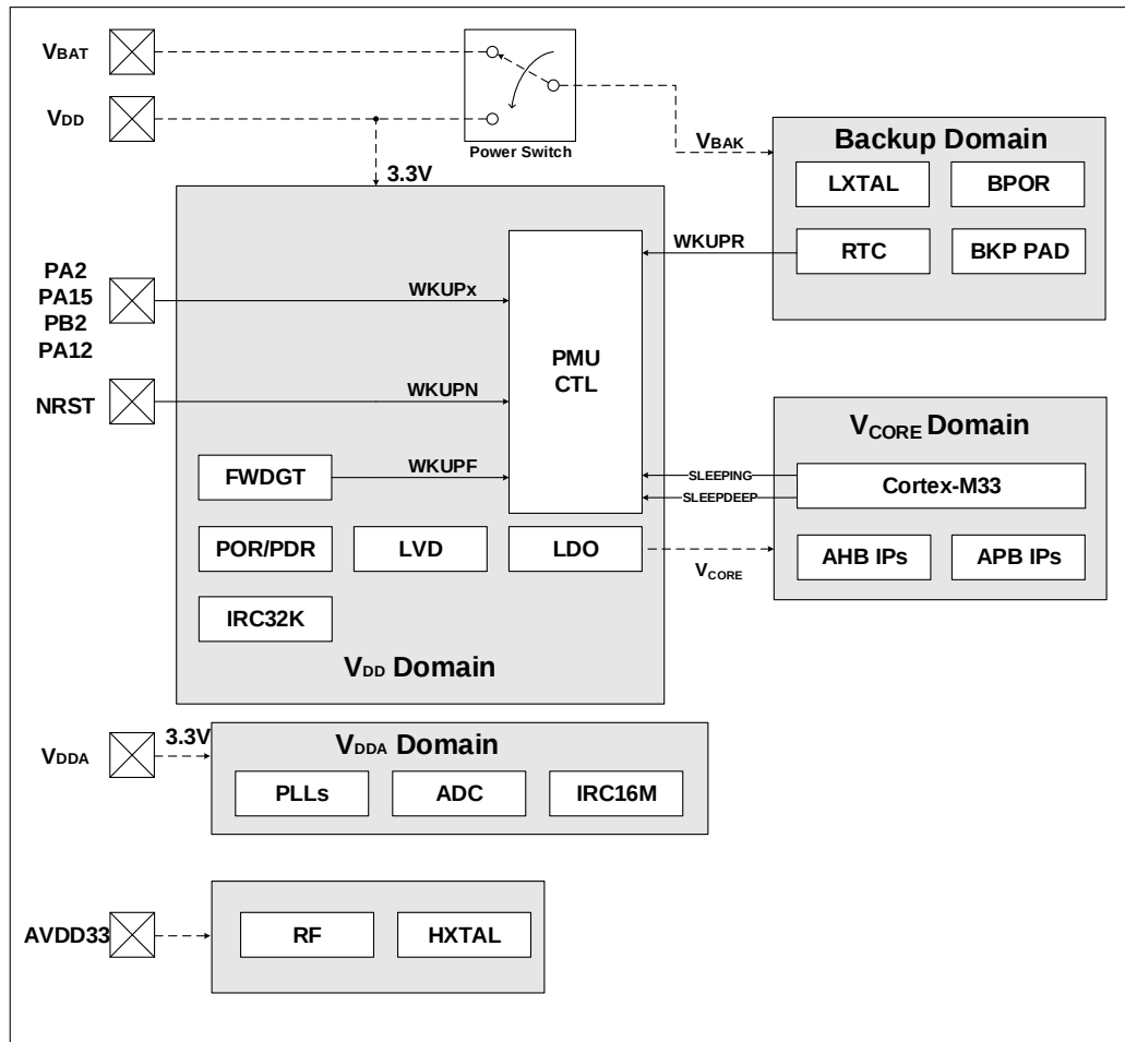
图 5-1. 电源域概览（适用于 GD32W515xx 系列）
