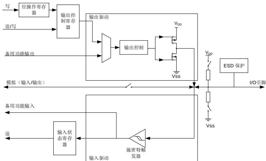
图 9-1. GPIO 端口位的基本结构
