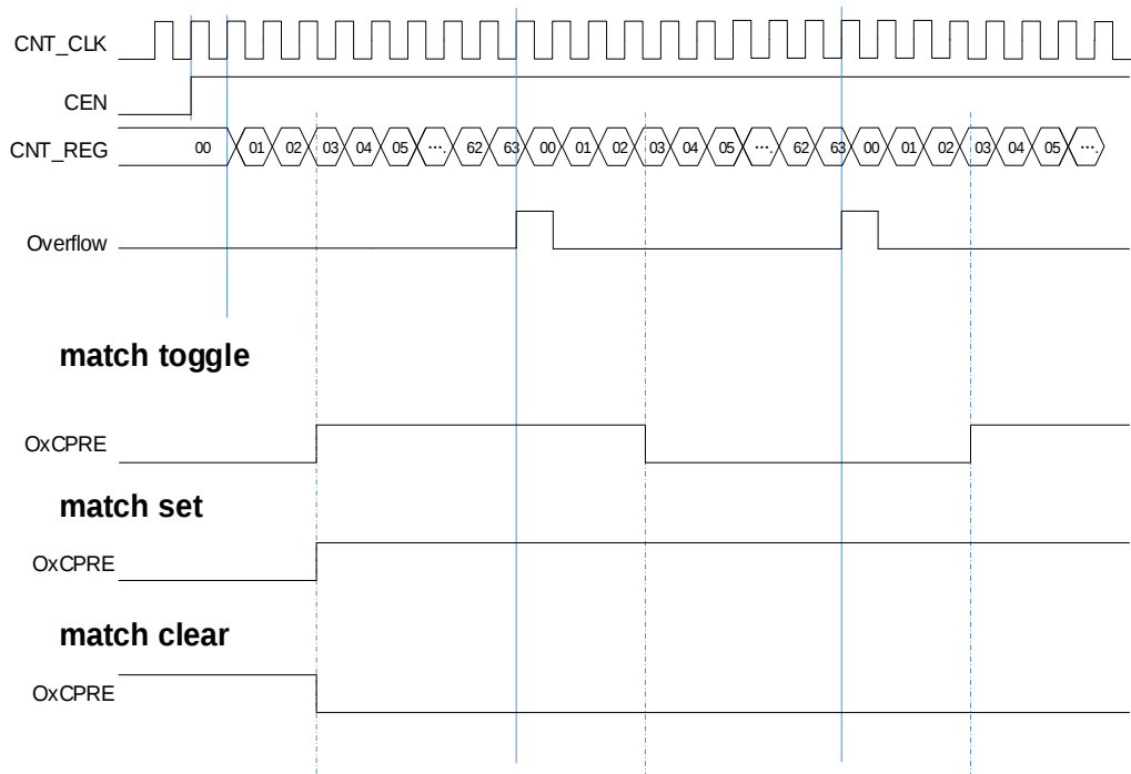
图 18-17. 三种输出比较模式
