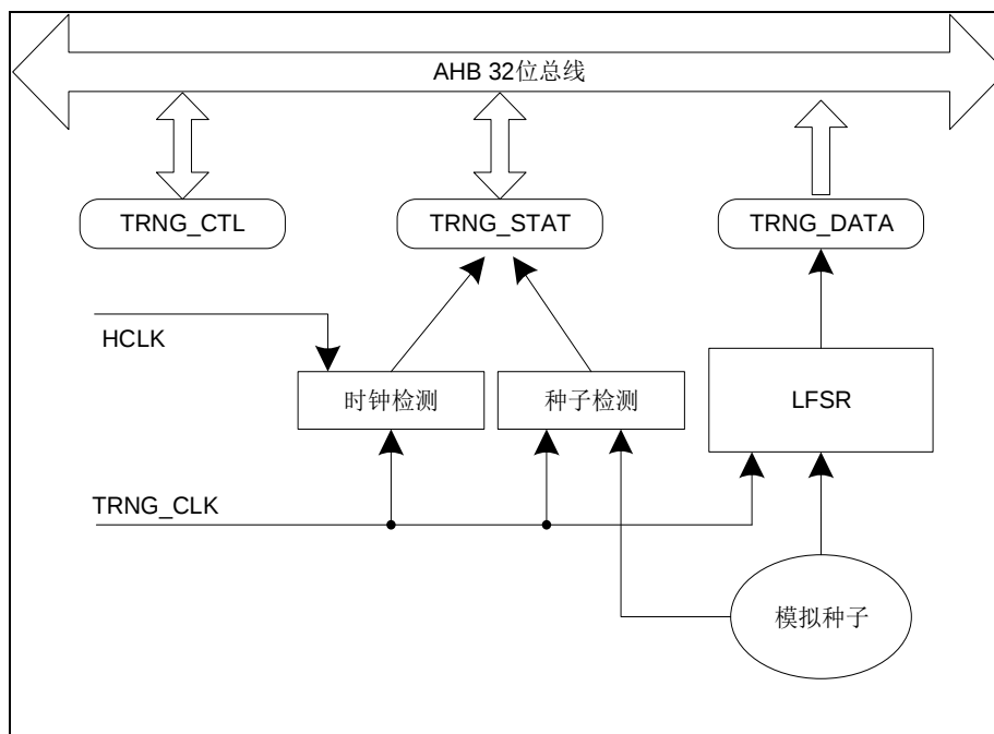
图 13-1. TRNG 模块框图
