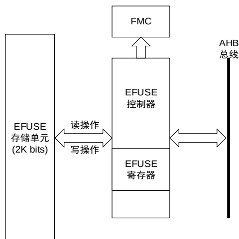
图 3-1. 熔丝控制器结构框图
