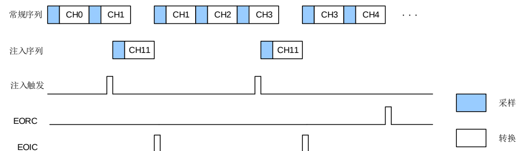
图 15-17. 触发注入
