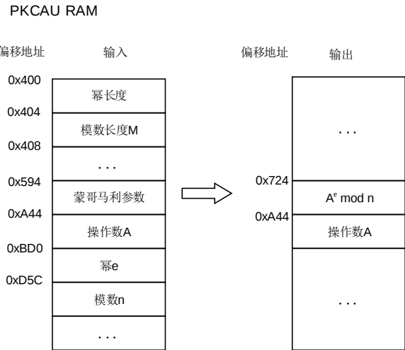
图 30-16. 快速模式模幂运算
