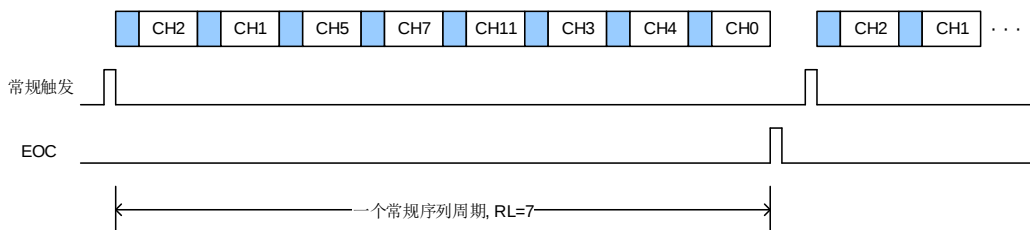
图 15-4. 扫描运行模式, 且连续运行模式禁能
