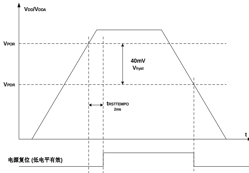
图 5-5. 上电/掉电复位波形图
