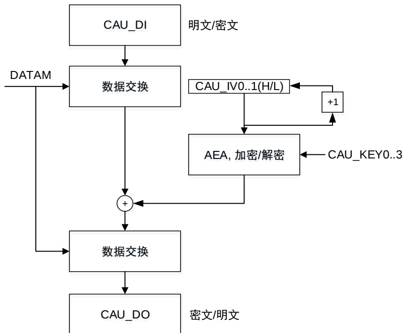
图 28-13. AES CTR 加密/解密
