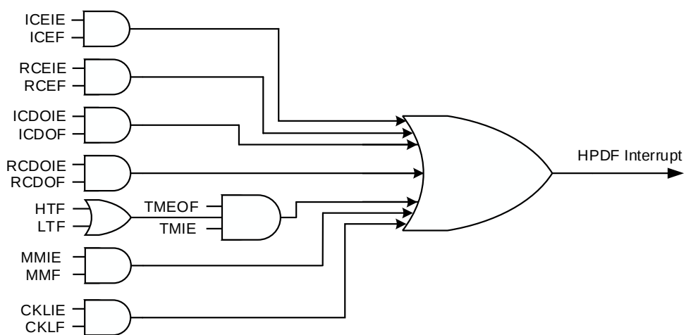
图 31-8. HPDF 中断逻辑图
