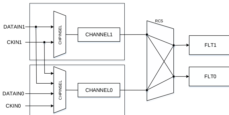
图 31-6. 通道引脚重定向
