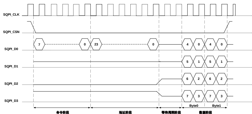
图 22-7. SQPI SQQ 模式时序(SQPI)
