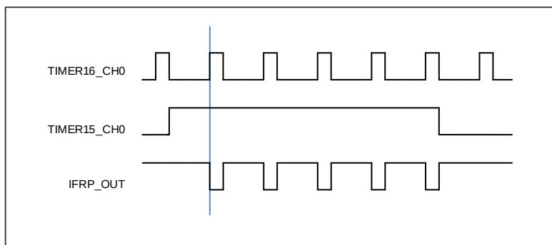
图 32-2. IFRP 输出时序图 3
