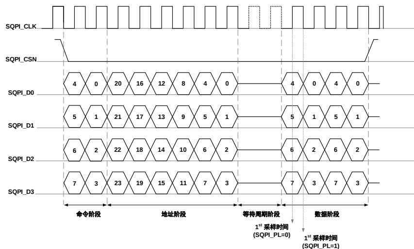
图 22-1. SQPI 采样极性
