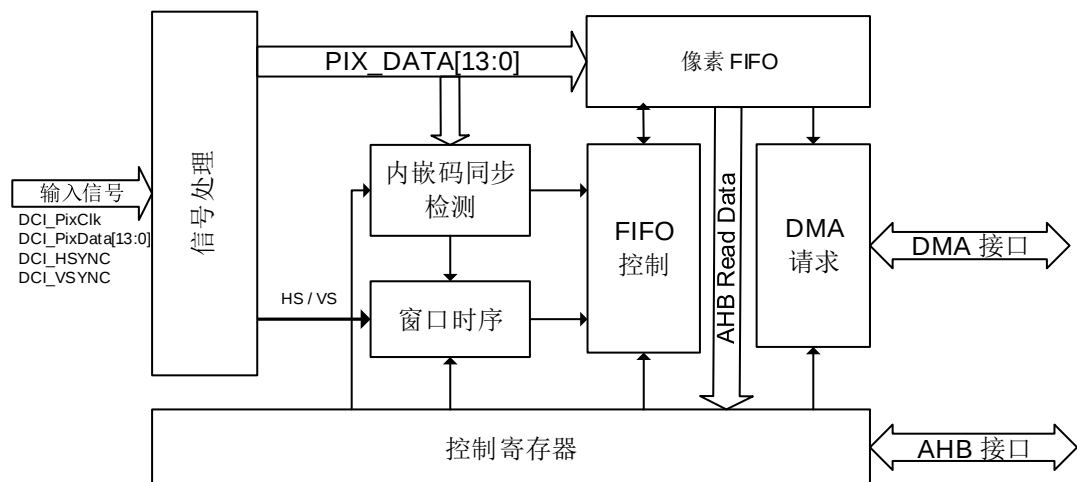
图 26-1. DCI 模块示意图
