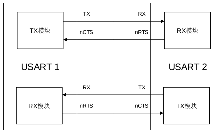
图 19-7. 两个 USART 之间的硬件流控制
