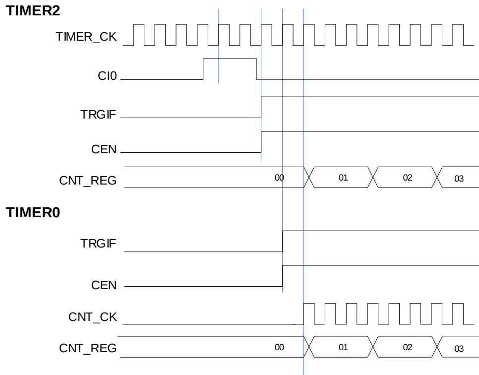
图 18-44. 用定时器 2 的 CI0 信号来触发定时器 0 和定时器 2 (仅适用于 GD32F5HCxx 系列)
