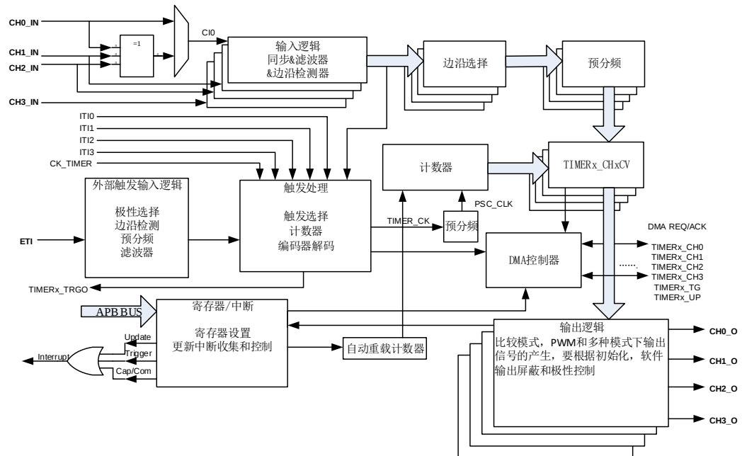
图 18-46. 通用定时器 L0 结构框图（仅适用于 GD32F5HCxx 系列）
