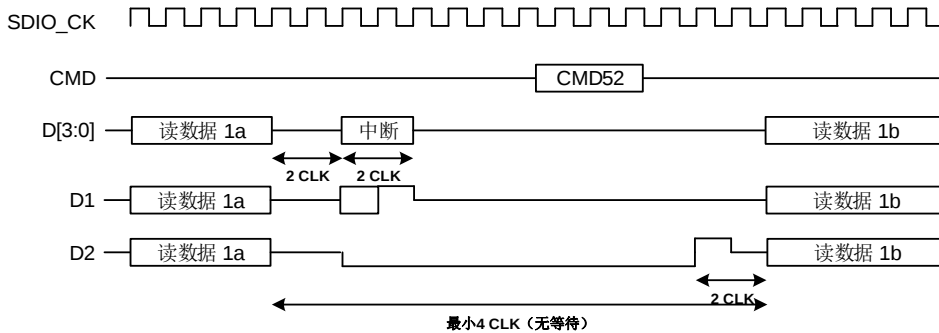
图 24-13. 使用 SDIO_D[2]信号线的读等待操作
