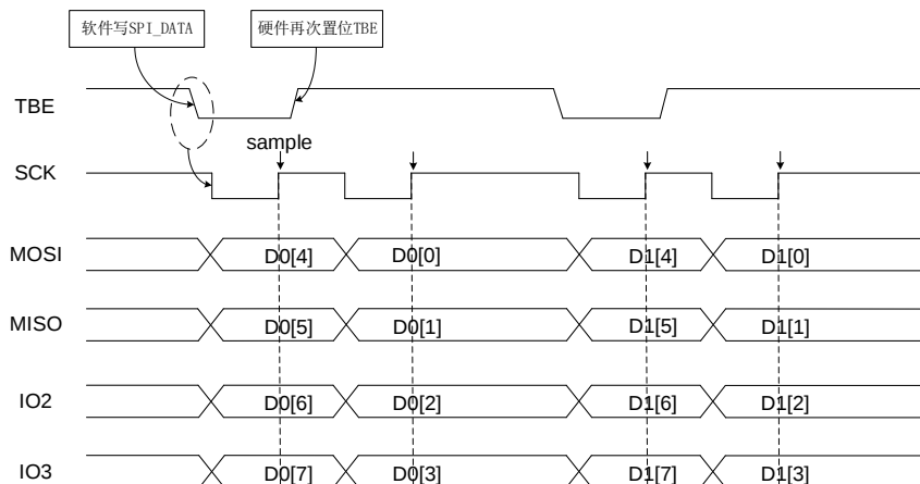
图 21-11. SPI 四线模式四线写操作时序图
