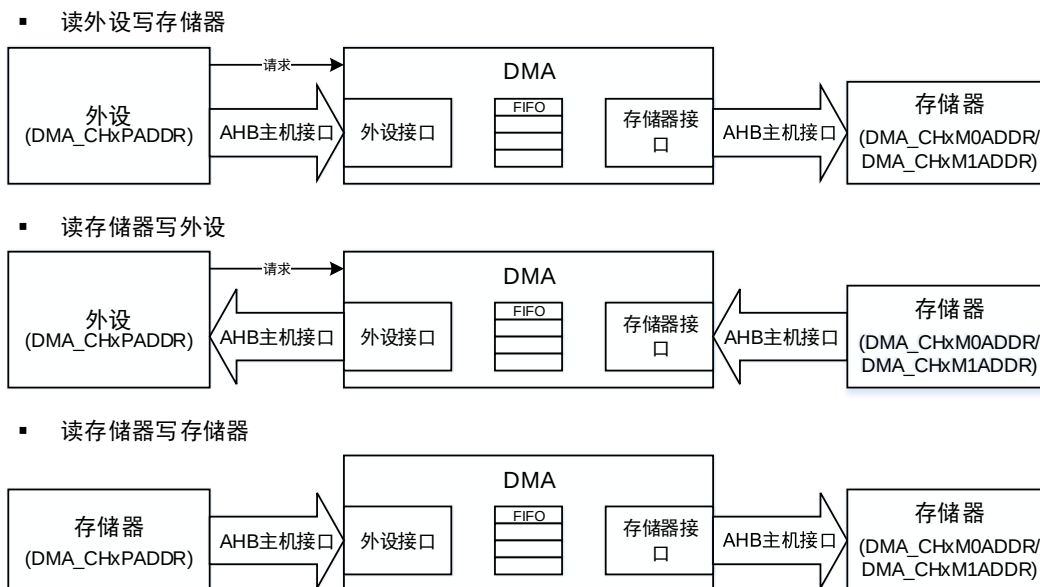
图 14-2. 三种传输模式的数据流
