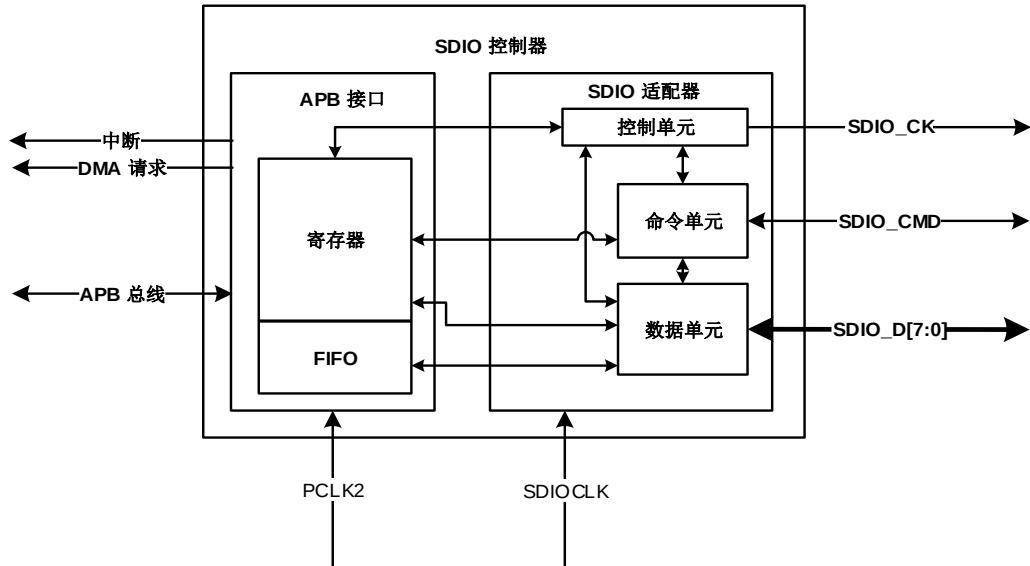
图 24-6. SDIO 框图
