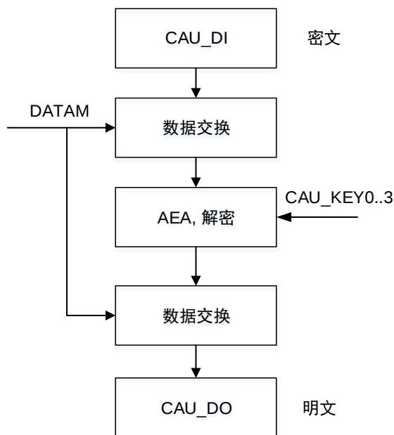
图 28-9. AES ECB 解密
