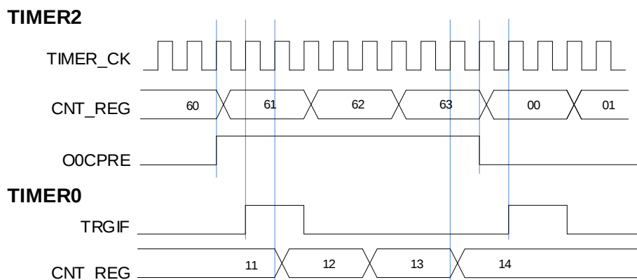
图 18-43. 用定时器 2 的 O0CPRE 信号控制定时器 0 的暂停模式（仅适用于 GD32F5HCxx 系列）
