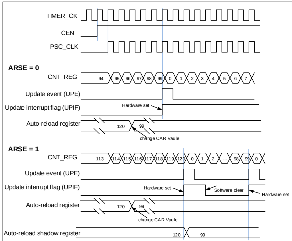
图 18-7. 向上计数时序图，在运行时改变 TIMERx_CAR 寄存器的值
