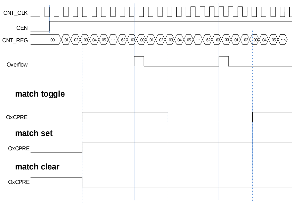
图 18-57. 三种输出比较模式
