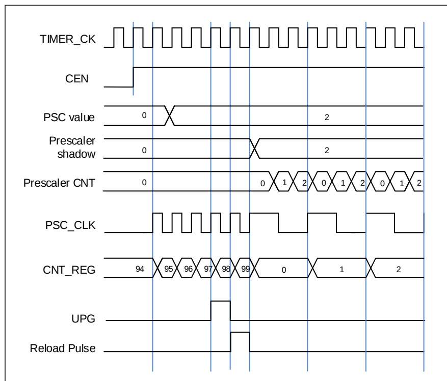
图 18-5. 当 PSC 数值从 0 变到 2 时，计数器的时序图
