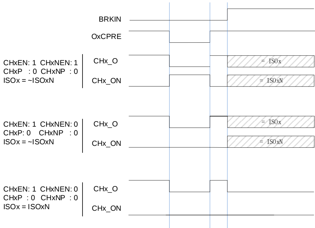
图 18-21. 通道响应中止输入（高电平有效）时，输出信号的行为
