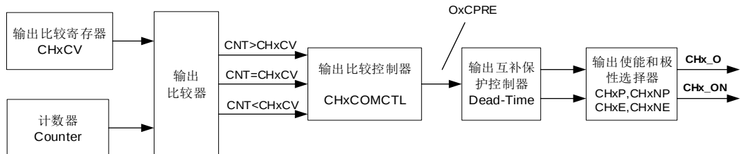
图 18-74. 通道输出比较原理（带有互补输出的通道，x=0）
