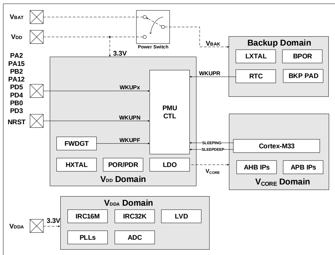
图 5-2. 电源域概览（适用于 GD32F5HCxx 系列）
