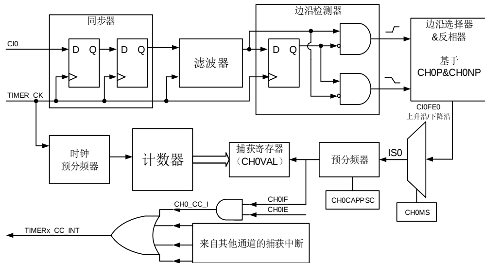
图 18-73. 通道输入捕获原理
