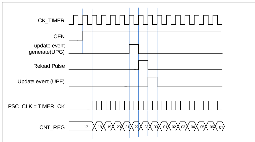
图 18-4. 内部时钟分频为 1 时，计数器的时序图（仅适用于 GD32F5HCxx 系列）
