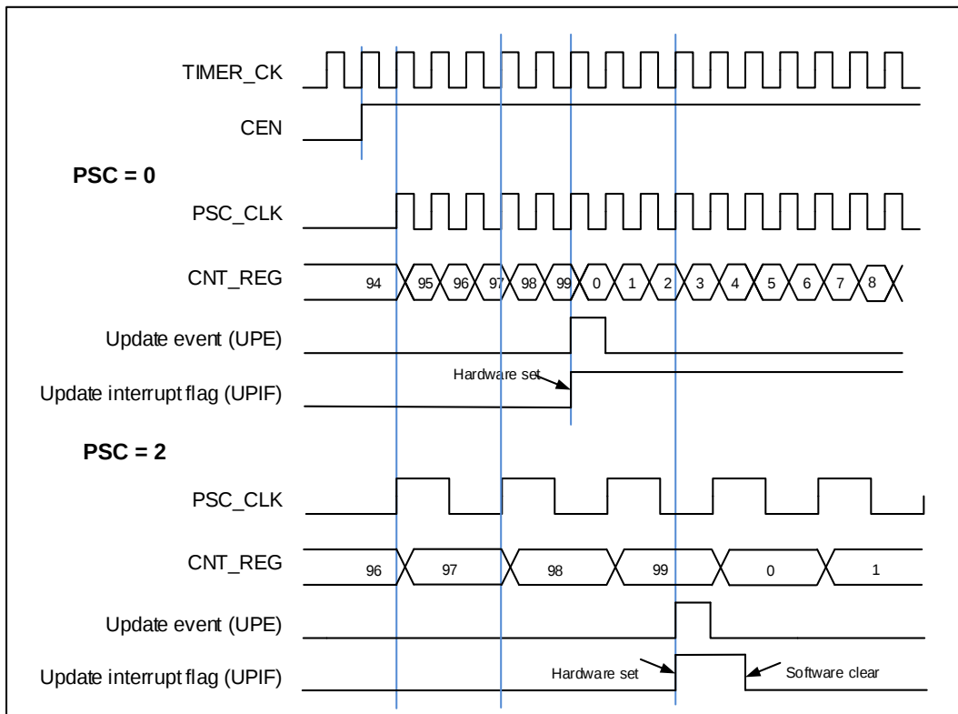
图 18-50. 向上计数时序图, PSC=0/2
