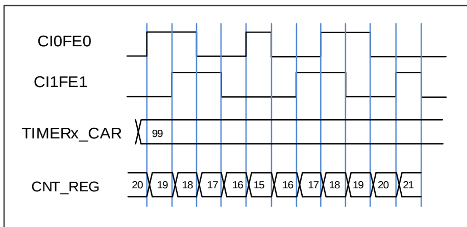
图 18-23.在编码器模式 2 且 CI0FE0 极性反相时计数器行为
