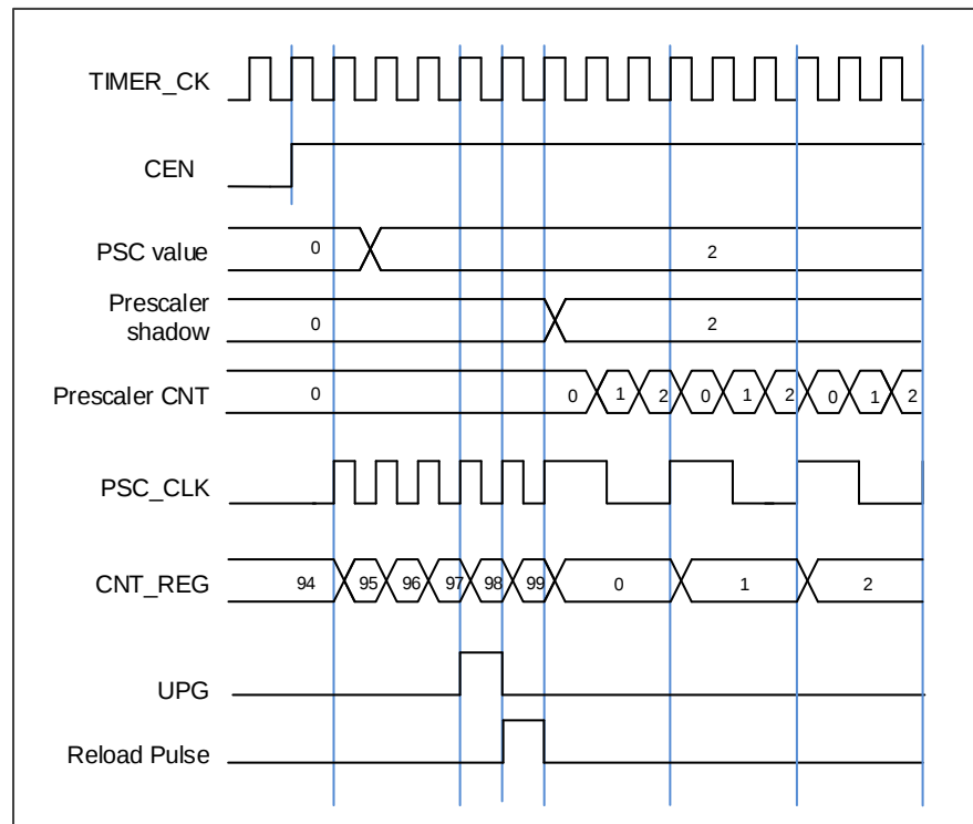
图 18-82. 当 PSC 数值从 0 变到 2 时，计数器的时序图
