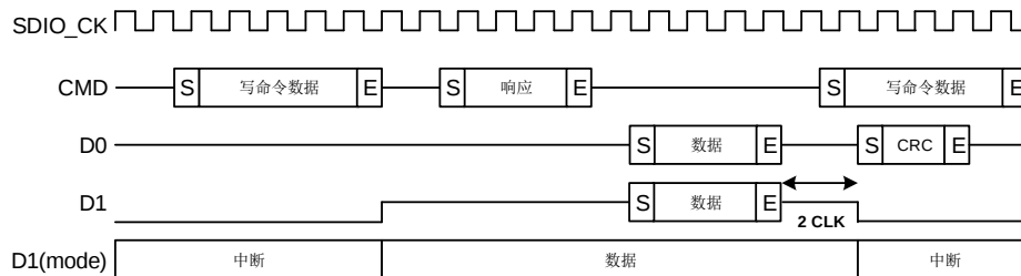
图 24-16. 写中断周期时序
