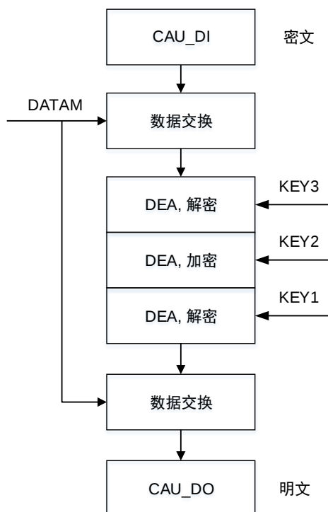
图 28-5. DES / TDES ECB 解密
