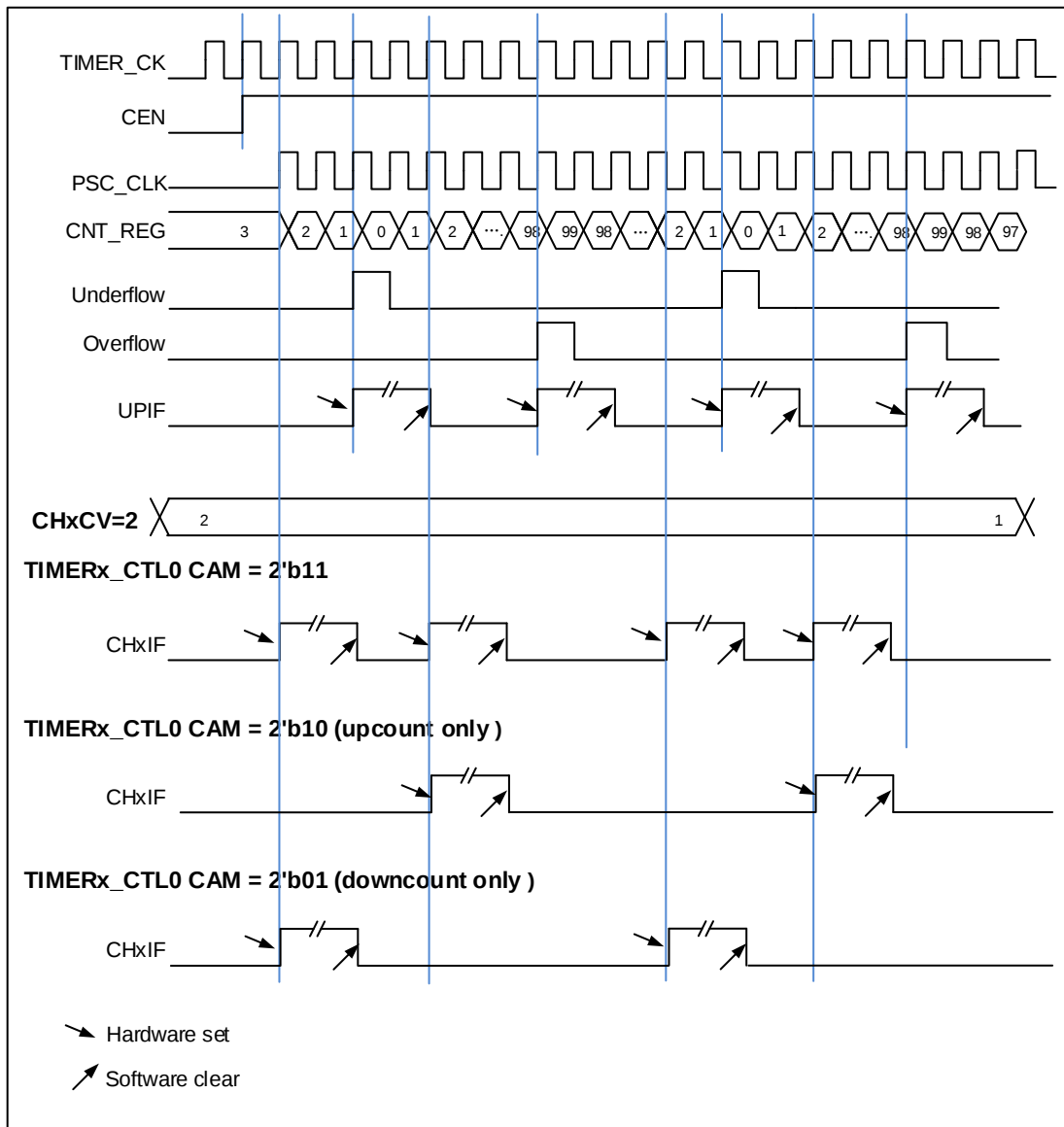
图 18-54. 中央计数模式计数器时序图
