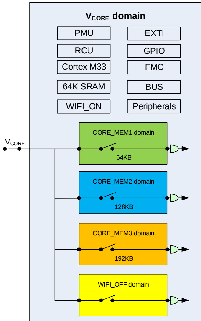
图 5-3. V CORE 电源域概览（适用于 GD32W515xx 系列）
