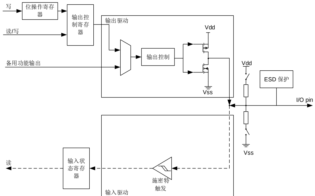
图 9-3. 输出配置的基本结构
