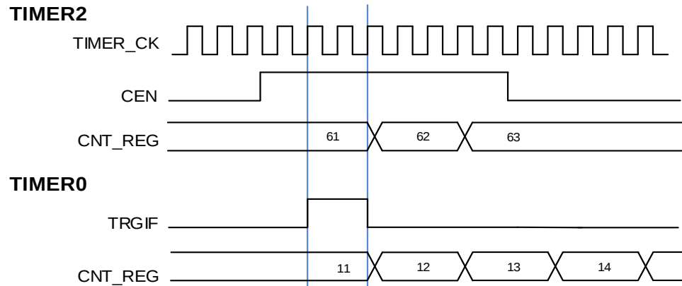
图 18-40. 用定时器 2 的使能信号触发定时器 0（仅适用于 GD32F5HCxx 系列）
