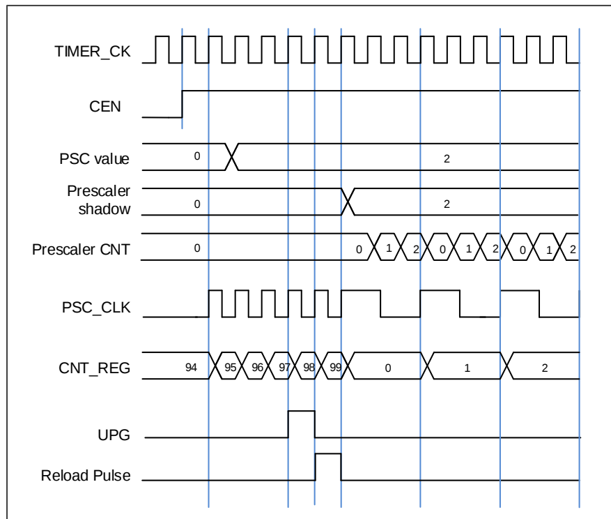
图 18-69. 当 PSC 数值从 0 变到 2 时，计数器的时序图
