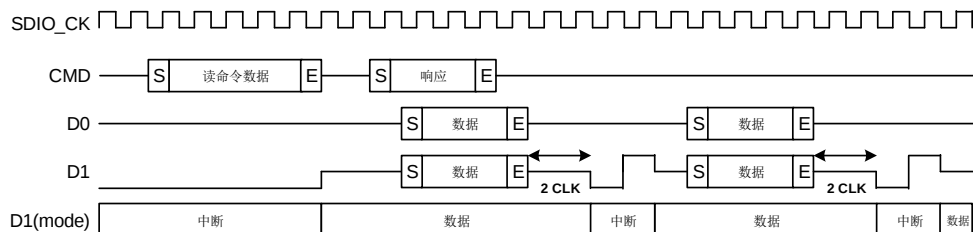
图 24-17. 4 位模式下多块读中断周期时序
