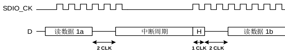
图 24-12. 通过停止 SDIO_CK 的读等待操作
