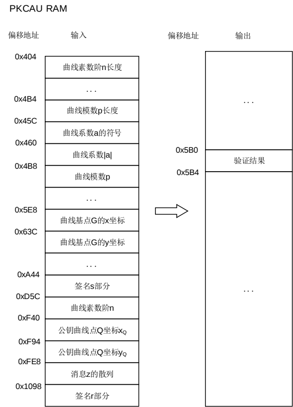
图 30-23. ECDSA 验证
