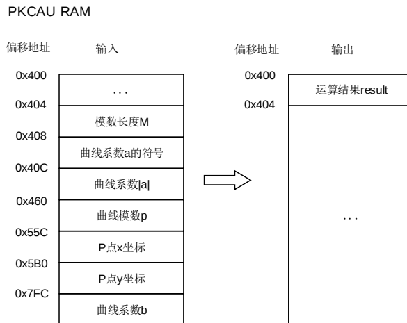
图 30-19. 椭圆曲线在 F_p 域上点的检查
