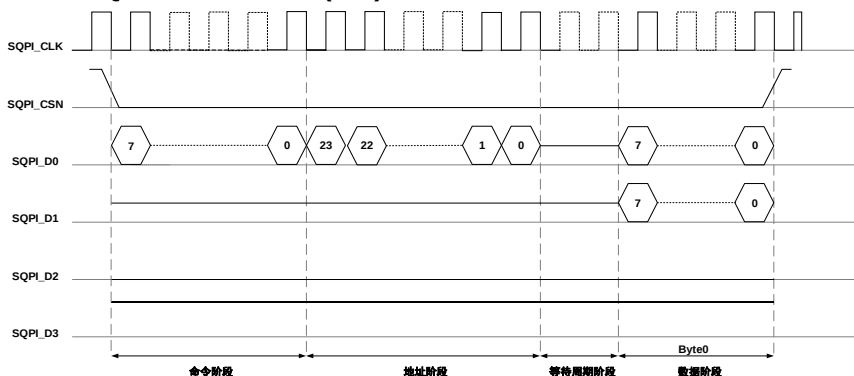
图 22-5. SQPI SSS 模式时序(SPI)
