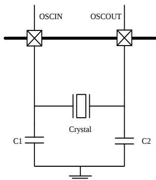
图 6-4. HXTAL 时钟源
