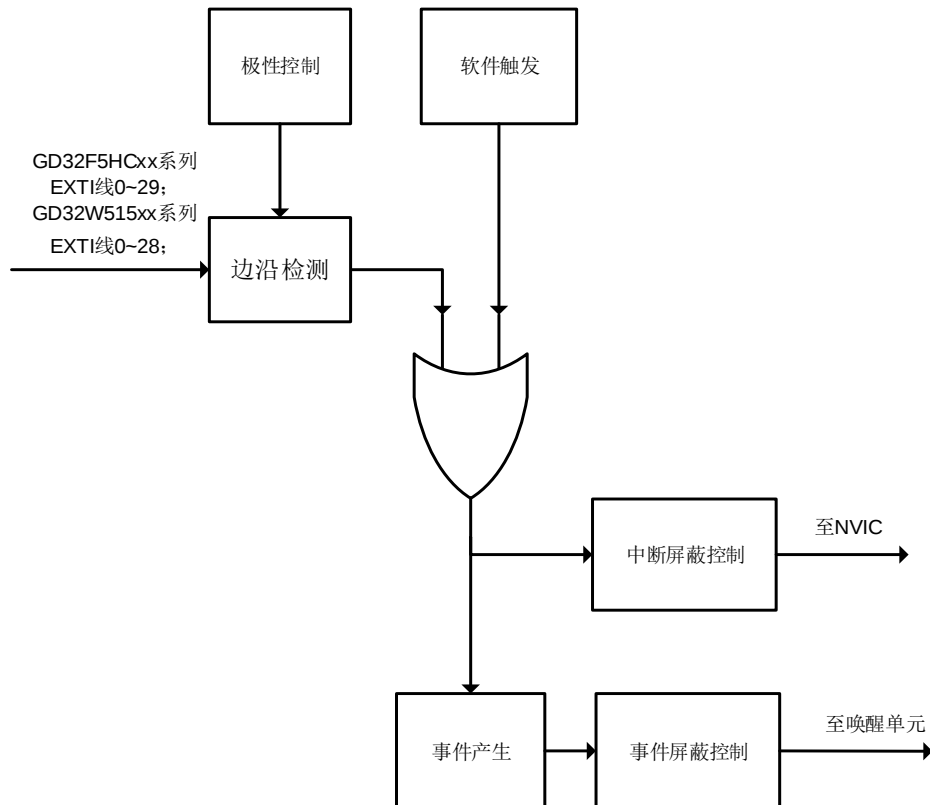
图 8-1. EXTI 结构框图
