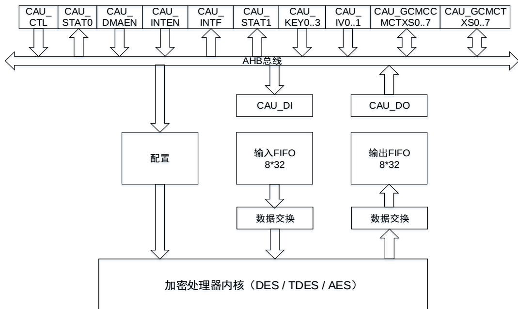
图 28-3. CAU 框图
