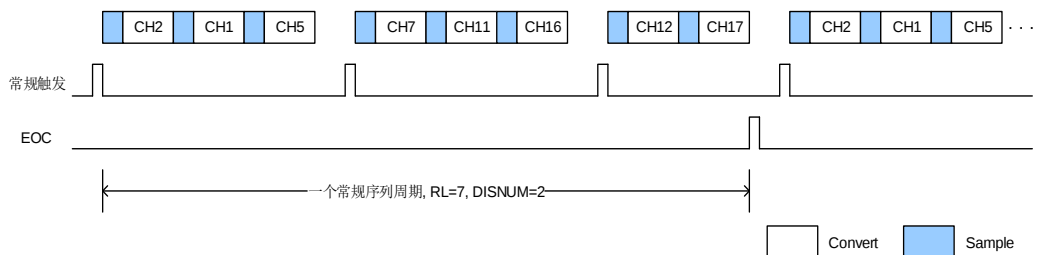
图 15-6. 间断运行模式
