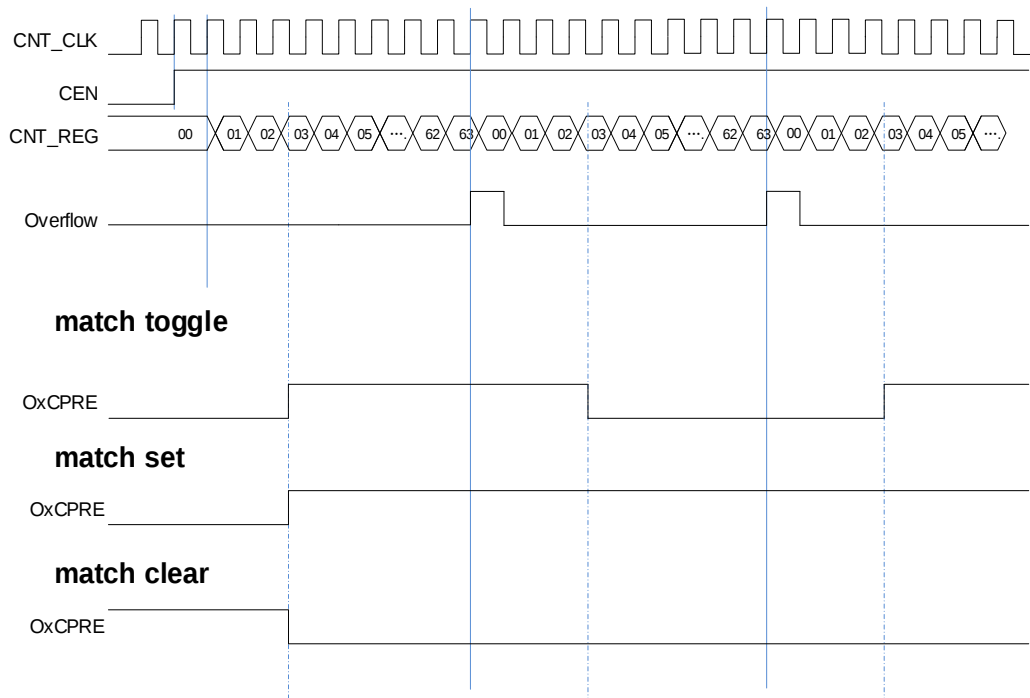
图 18-75. 三种输出比较模式
