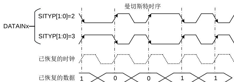
图 31-3. 曼切斯特数据传输时序图
