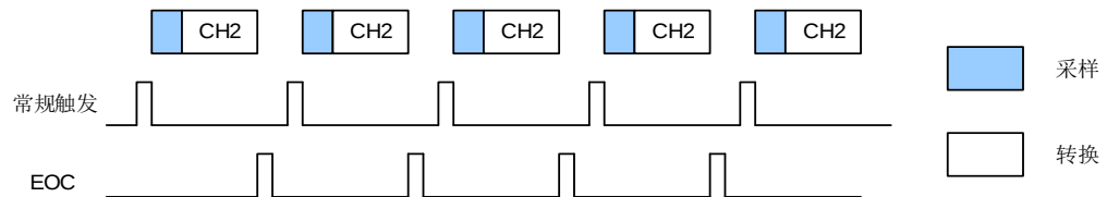
图 15-2. 单次运行模式
