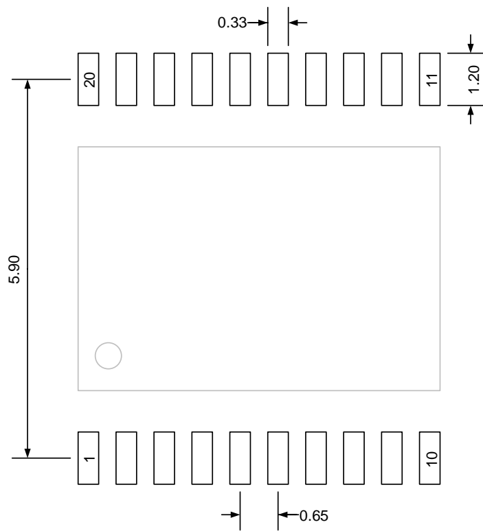
图5-12. 推荐的TSSOP20焊盘尺寸
