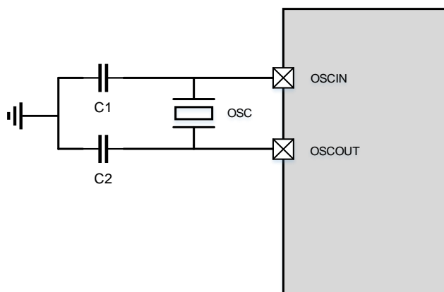
图4-4. 推荐用于外部无源晶振的OSCIN和OSCOUT引脚电路
