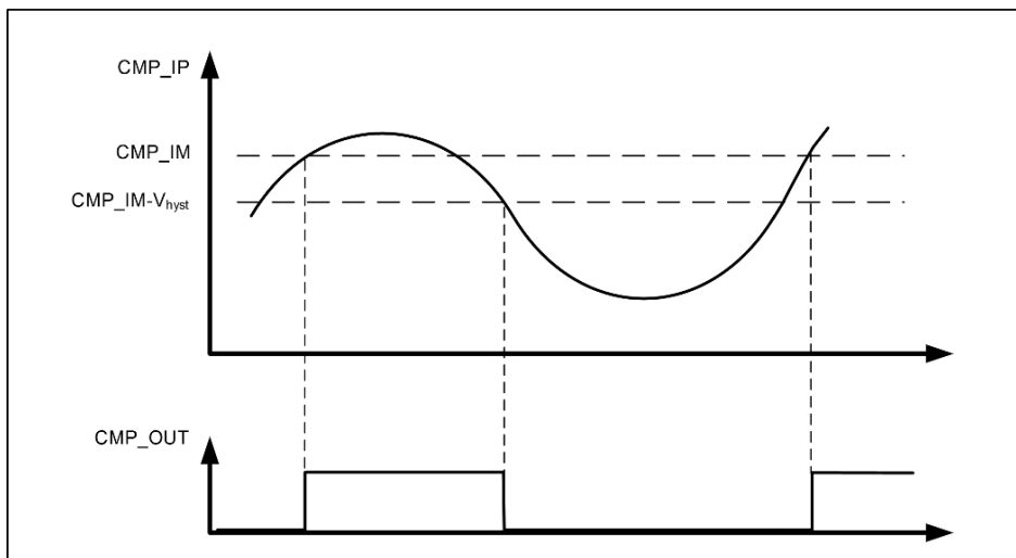
图4-9. CMP滞后
