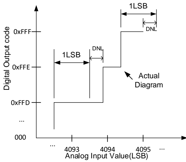
图4-7. 微分线性误差
