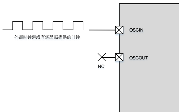
图4-5. 推荐用于外部时钟源或有源晶振的OSCIN和OSCOUT引脚电路
