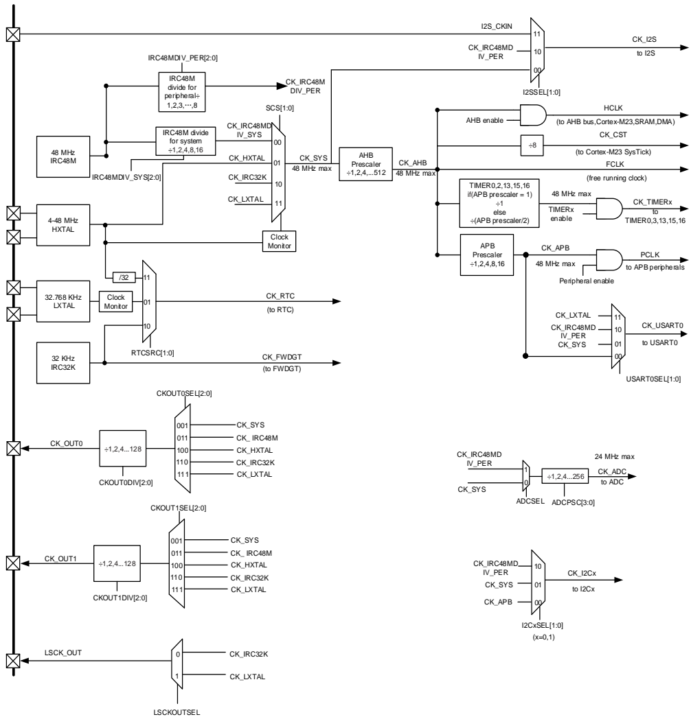
图2-9. GD32C231xx时钟树
