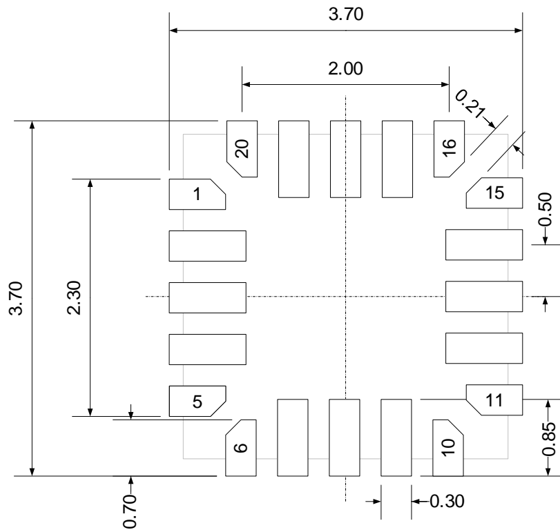
图5-14. 推荐的LGA20焊盘尺寸
