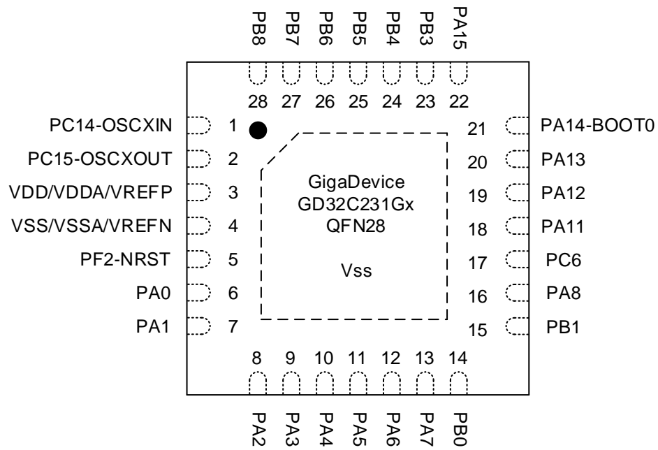
图2-6. GD32C231Gx QFN28引脚排列
